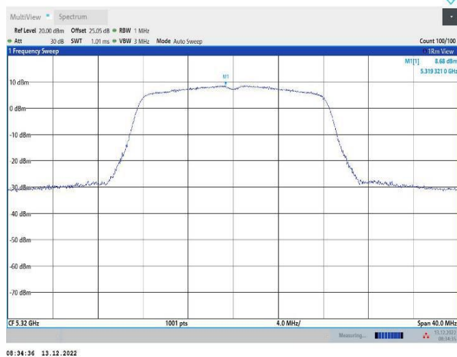
11A_Ant2_5320
