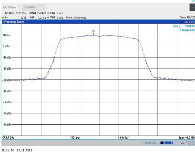
11A_Ant2_5700
