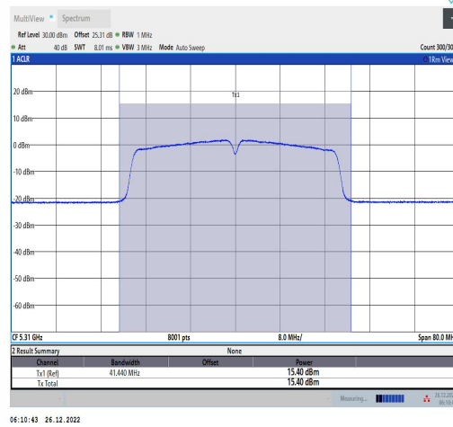
11N40MIMO-Ant1-5310-TPC L-----15.08-92.86-0.32
