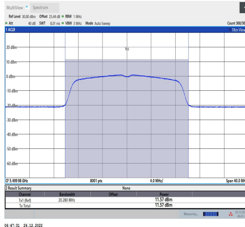
11AC20MIMO-Ant1-5500-TPC L-----11.20-91.89-0.37
