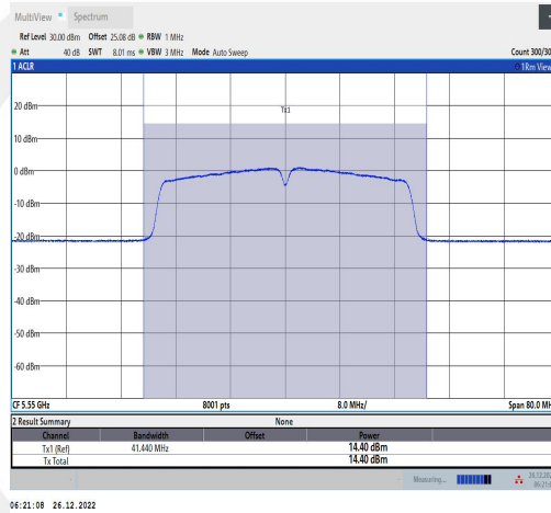
11N40MIMO-Ant1-5550-TPC L-----14.08-92.86-0.32
