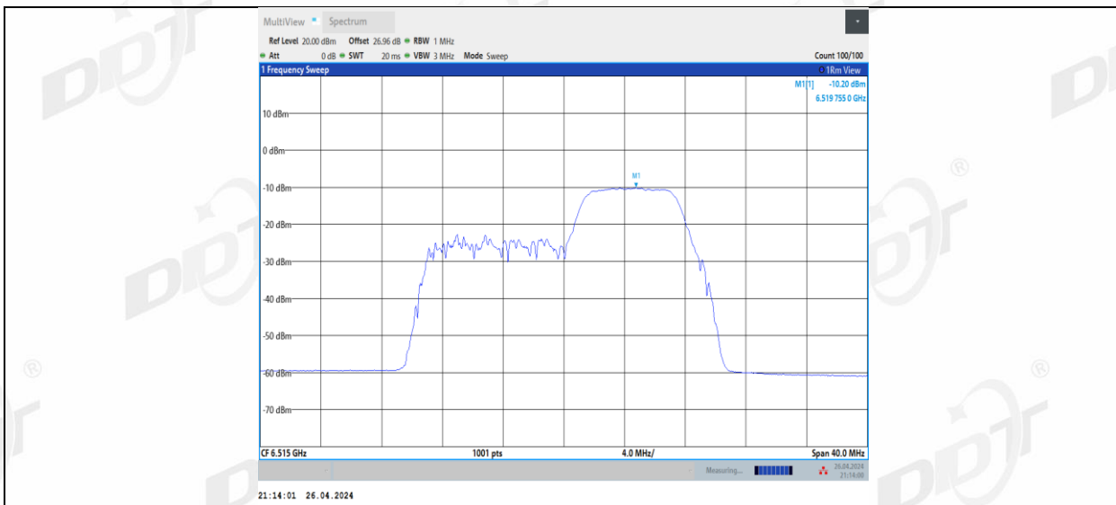
11BE20MIMO_Ant3_6515_106+26_1
