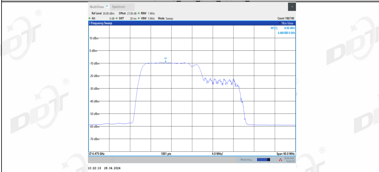
11BE20MIMO_Ant3_6475_106+26_2
