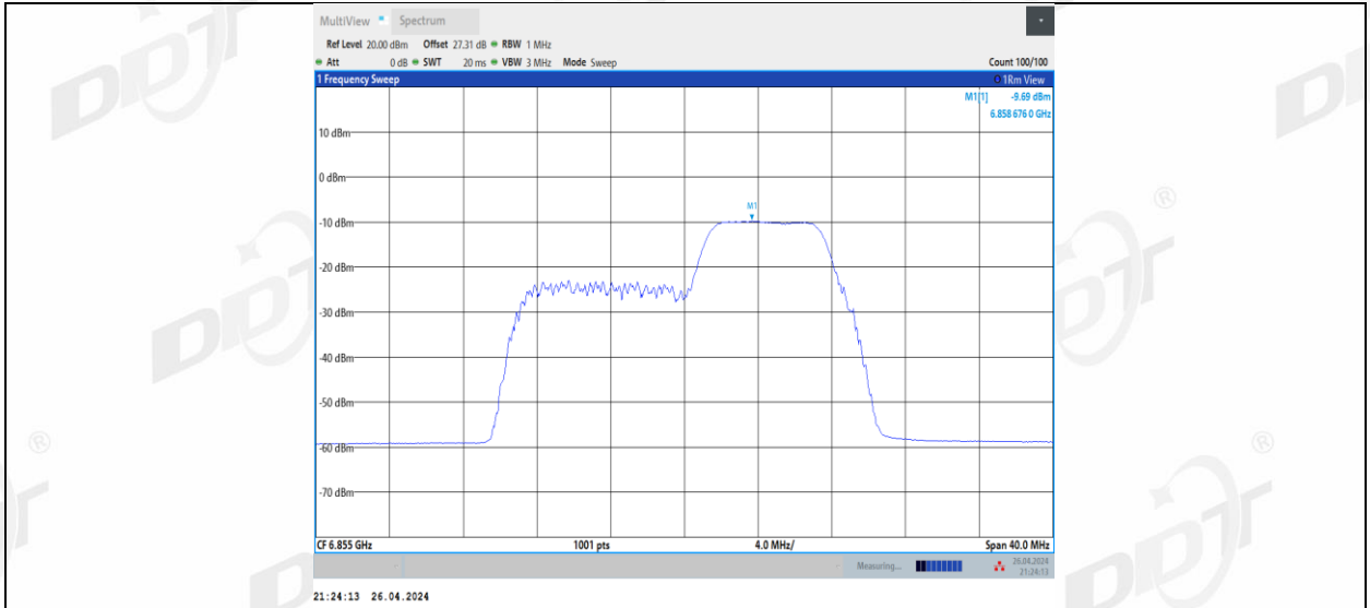
11BE20MIMO_Ant3_6855_106+26_1
