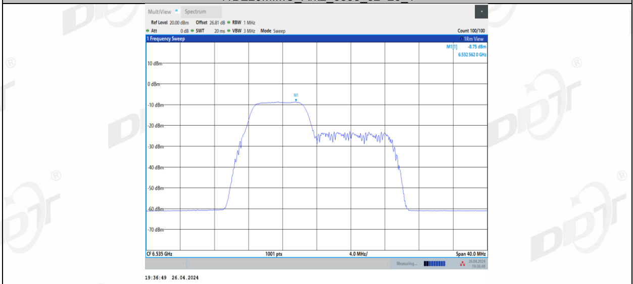
11BE20MIMO_Ant2_6535_52+26_2
