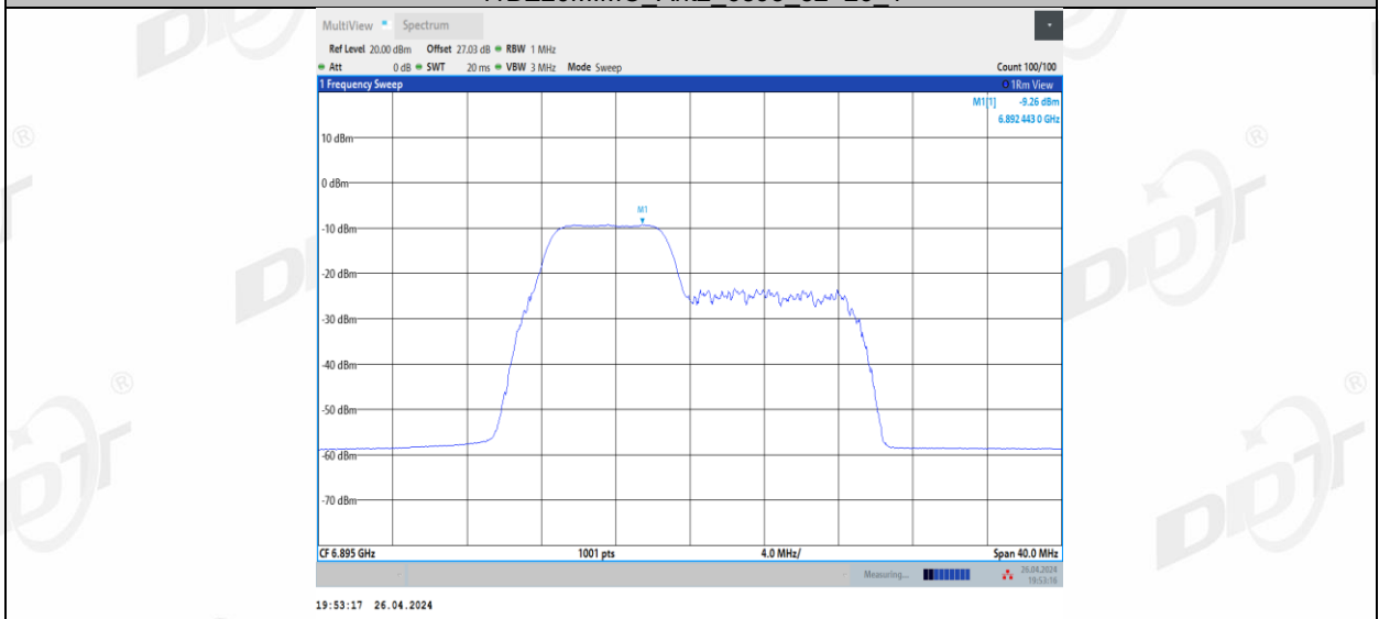
11BE20MIMO_Ant2_6895_52+26_2
