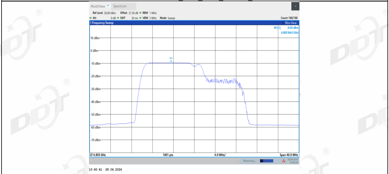
11BE20MIMO_Ant3_6855_106+26_2
