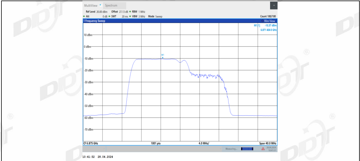
11BE20MIMO_Ant1_6875_106+26_2
