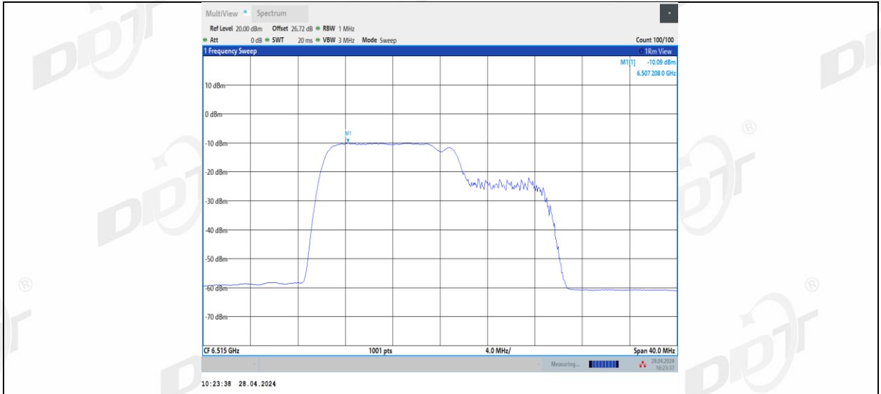
11BE20MIMO_Ant1_6515_106+26_2
