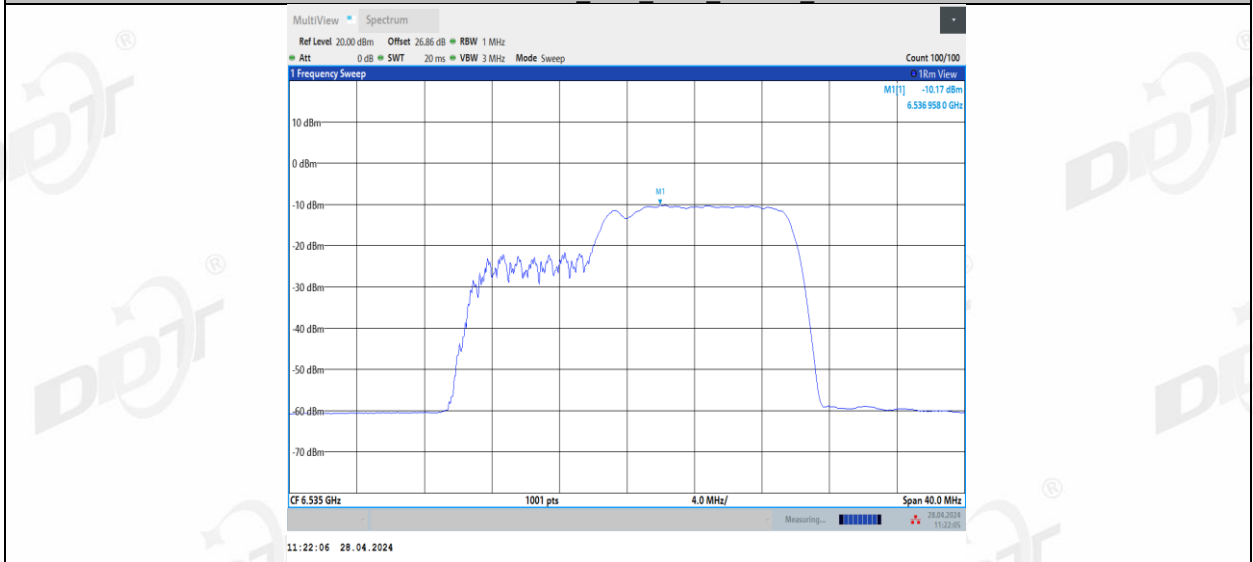
11BE20MIMO_Ant2_6535_52+26_1
