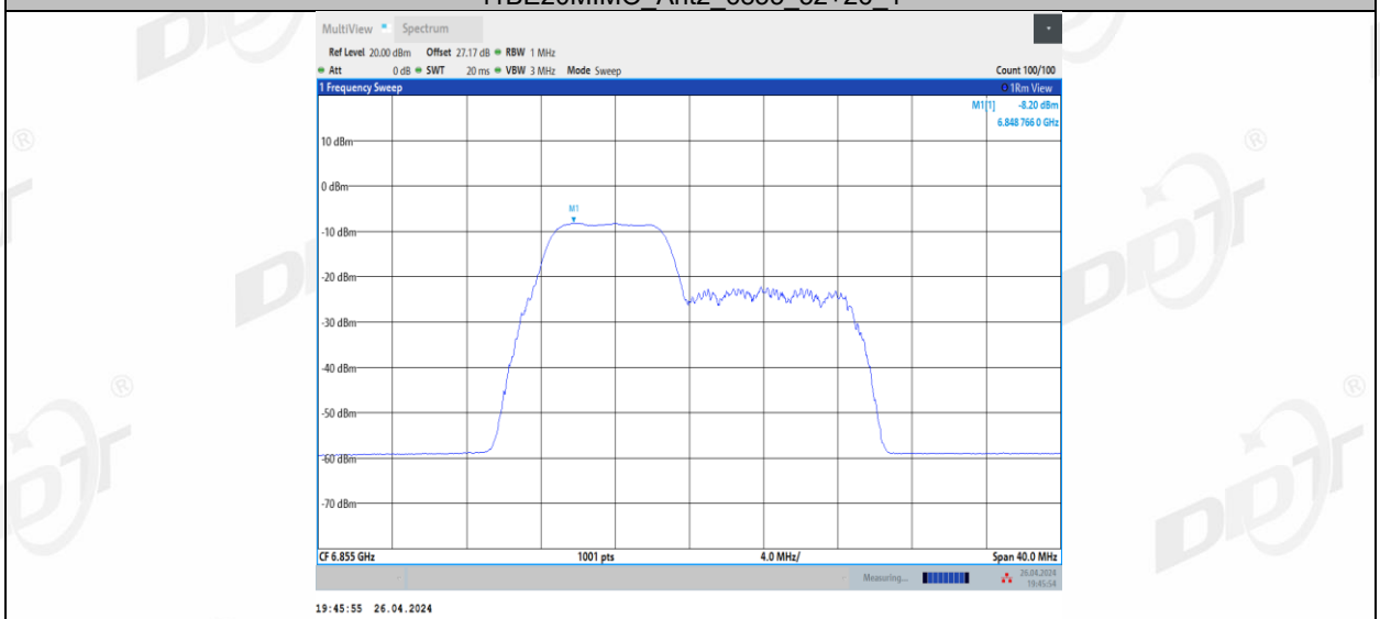
11BE20MIMO_Ant2_6855_52+26_2
