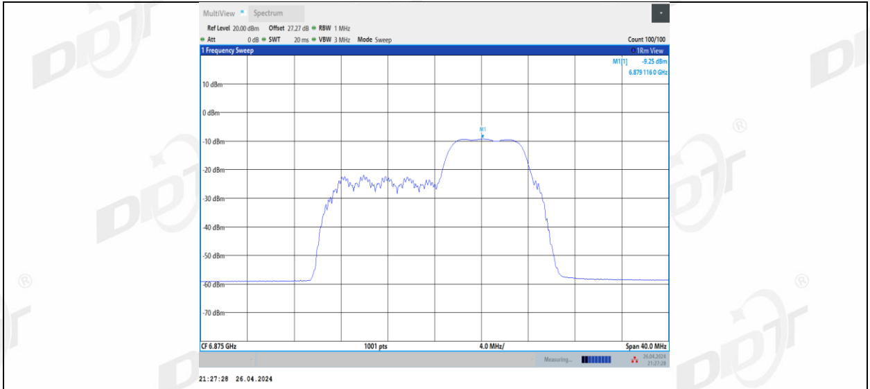
11BE20MIMO_Ant3_6875_106+26_1
