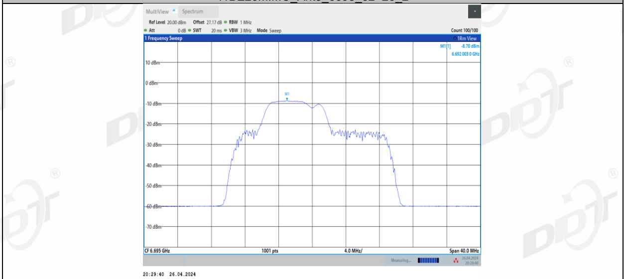
11BE20MIMO Ant3 6695 52+26_3
