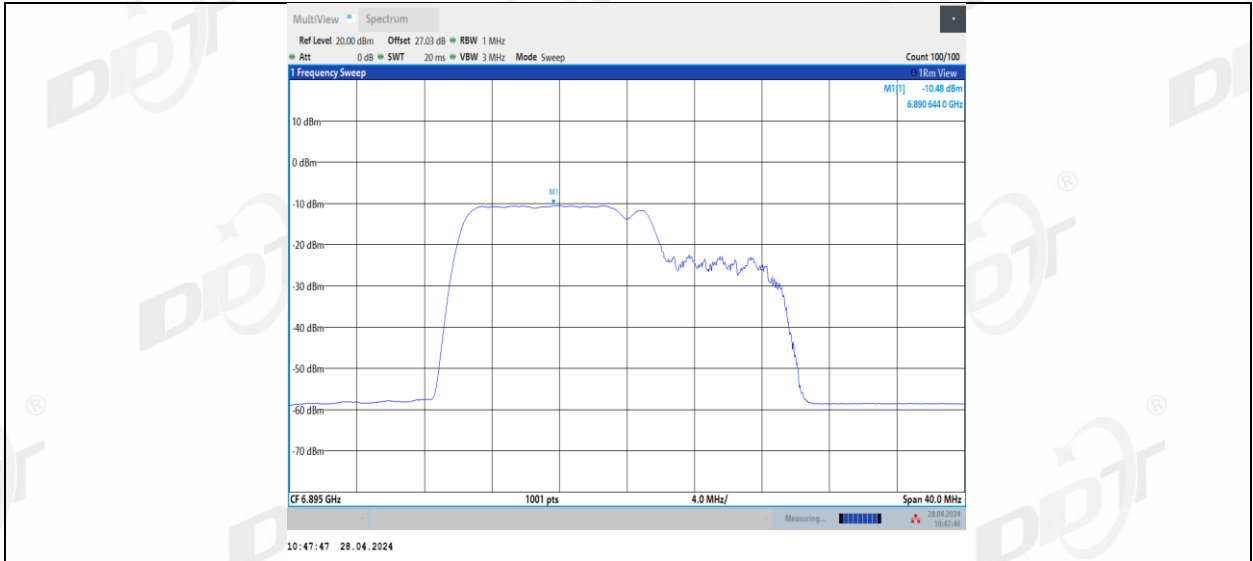
11BE20MIMO_Ant1_6895_106+26_2
