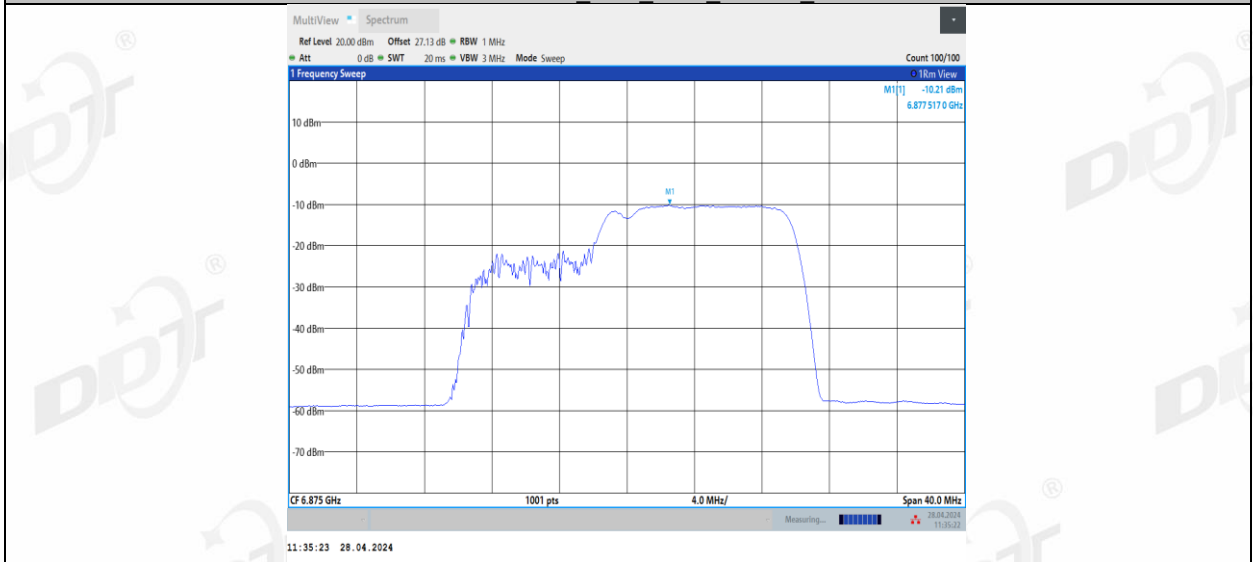
11BE20MIMO_Ant2_6875_52+26_1
