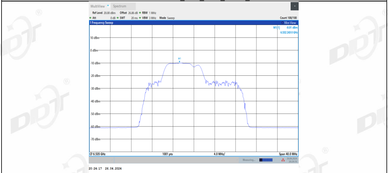
11BE20MIMO Ant1_6535_52+26_3
