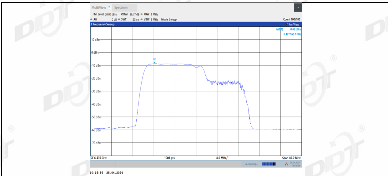
11BE20MIMO_Ant1_6435_106+26_2
