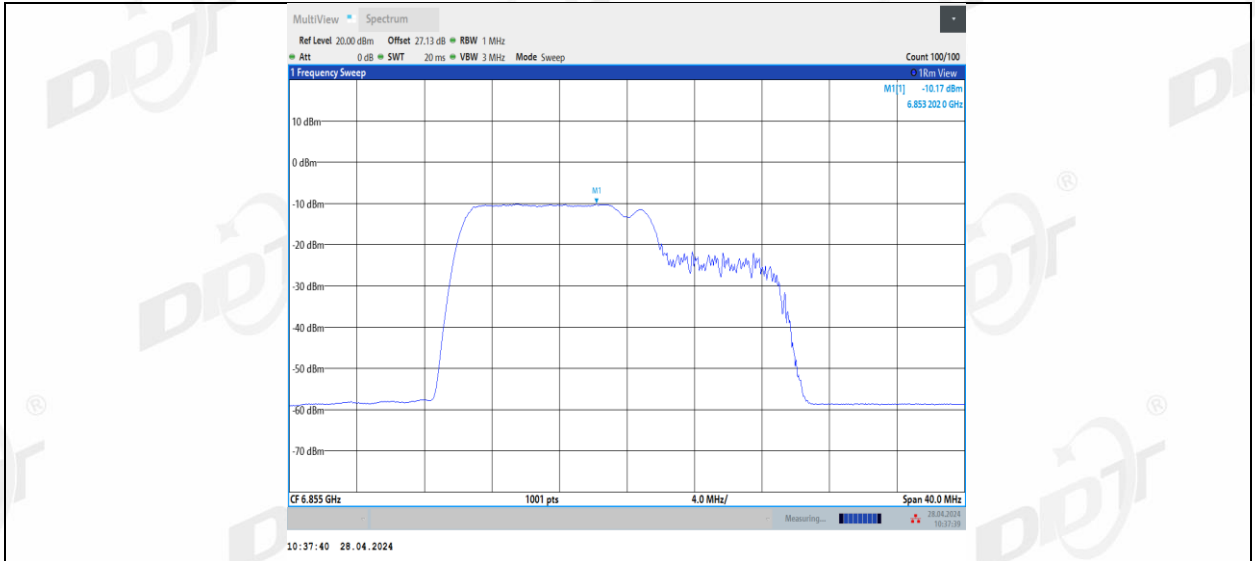
11BE20MIMO_Ant1_6855_106+26_2
