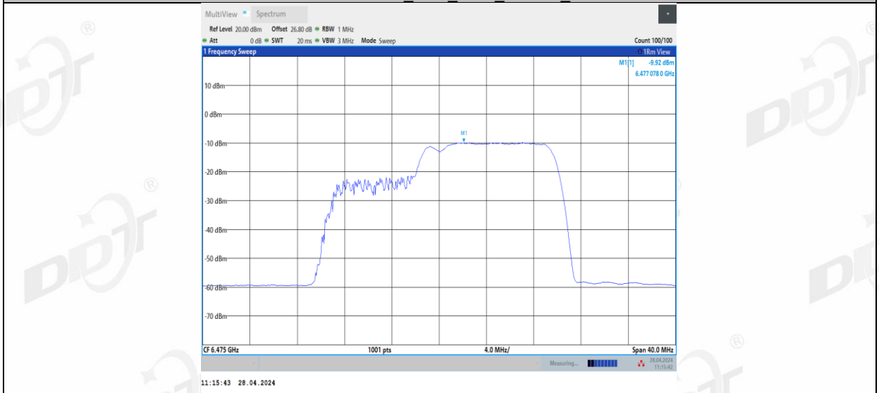
11BE20MIMO_Ant2_6475_52+26_1
