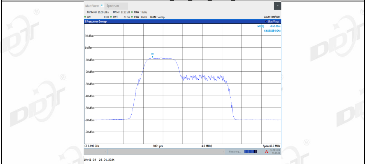
11BE20MIMO Ant3 6695 52+26_2
