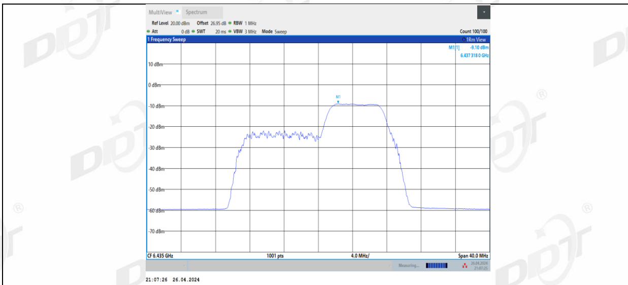
11BE20MIMO_Ant3_6435_106+26_1
