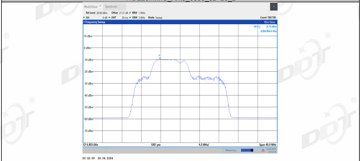
11BE20MIMO Ant3 6855 52+26_3
