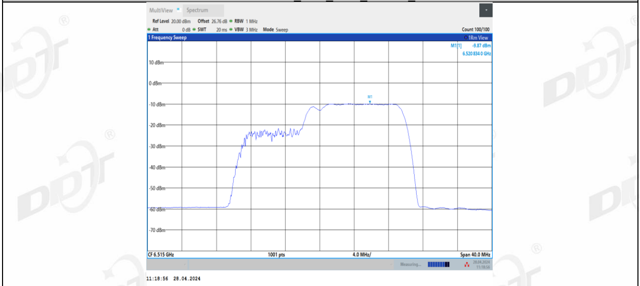
11BE20MIMO_Ant2_6515_52+26_1
