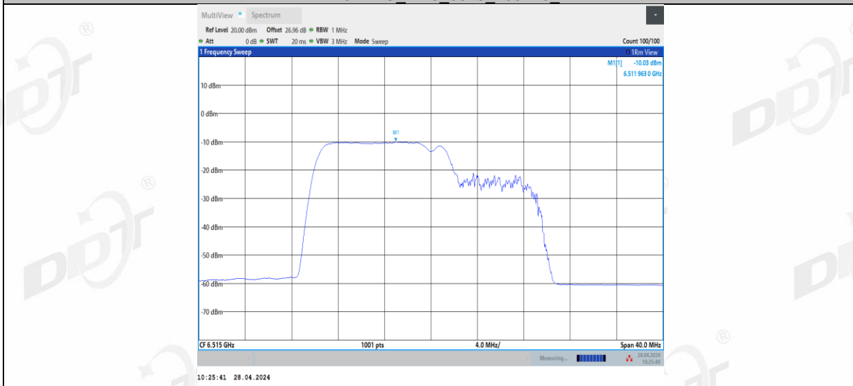
11BE20MIMO_Ant3_6515_106+26_2
