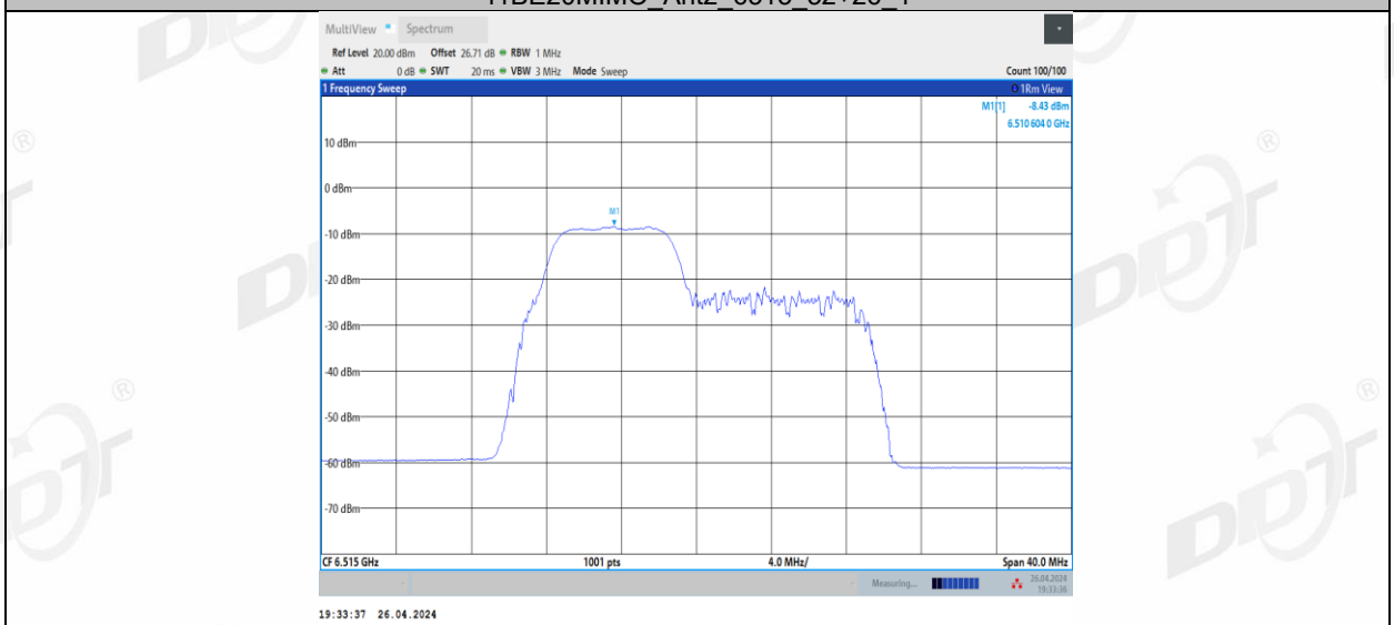
11BE20MIMO_Ant2_6515_52+26_2
