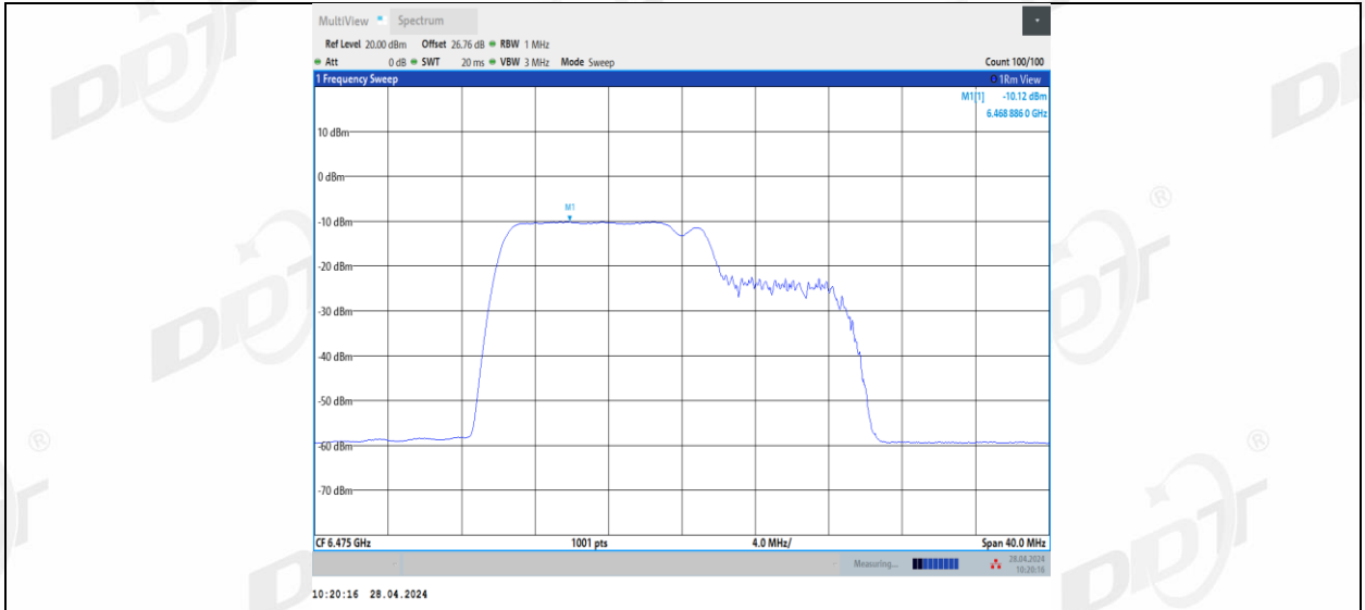
11BE20MIMO_Ant1_6475_106+26_2
