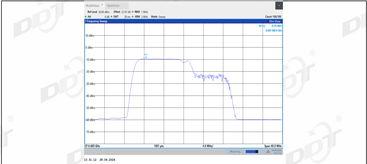
11BE20MIMO_Ant1_6695_106+26_2
