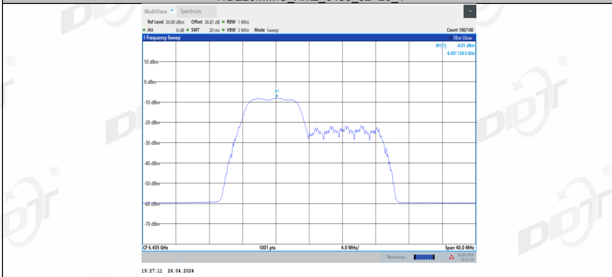
11BE20MIMO_Ant2_6435_52+26_2
