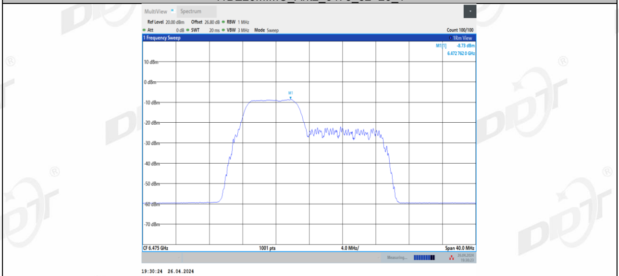
11BE20MIMO_Ant2_6475_52+26_2
