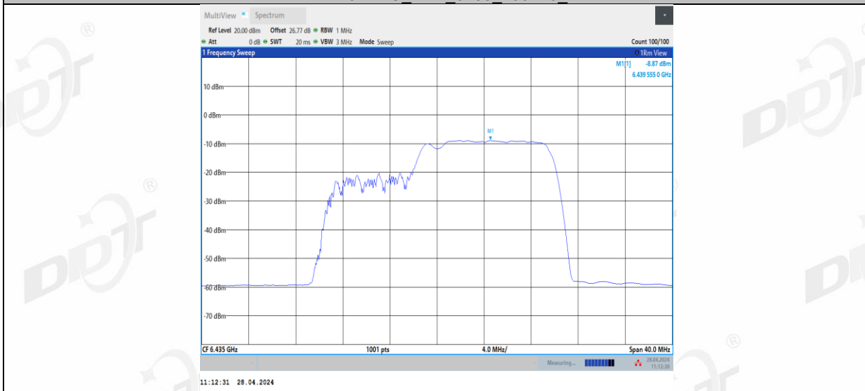
11BE20MIMO_Ant2_6435_52+26_1
