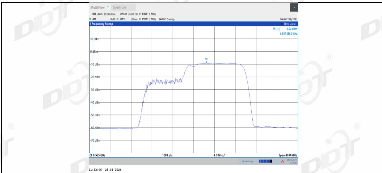
11BE20MIMO Ant3 6535 52+26_1
