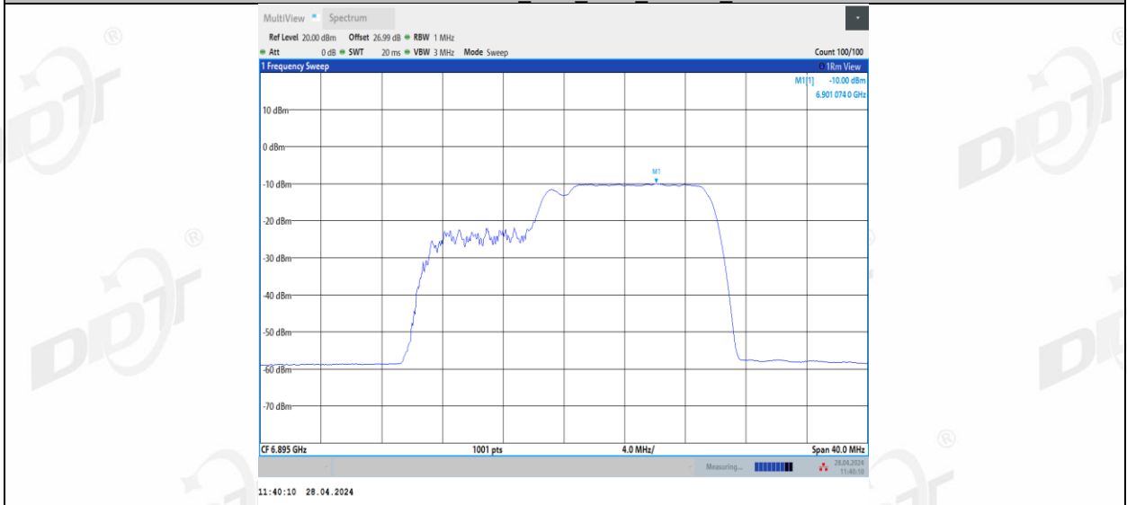
11BE20MIMO_Ant2_6895_52+26_1
