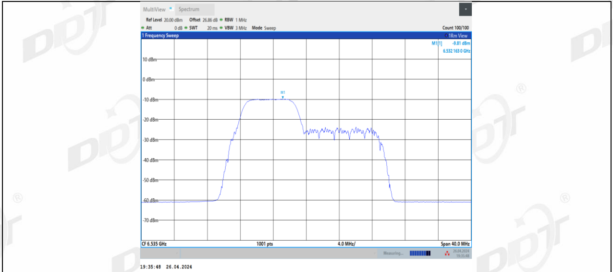
11BE20MIMO Ant1_6535_52+26_2
