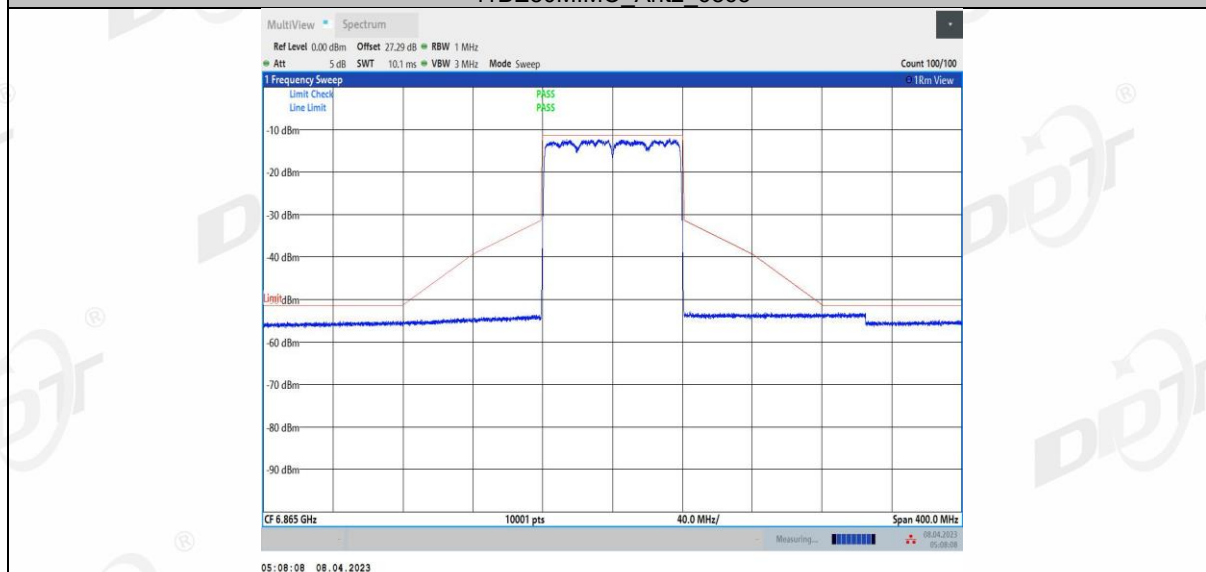
11BE80MIMO_Ant3_6865
