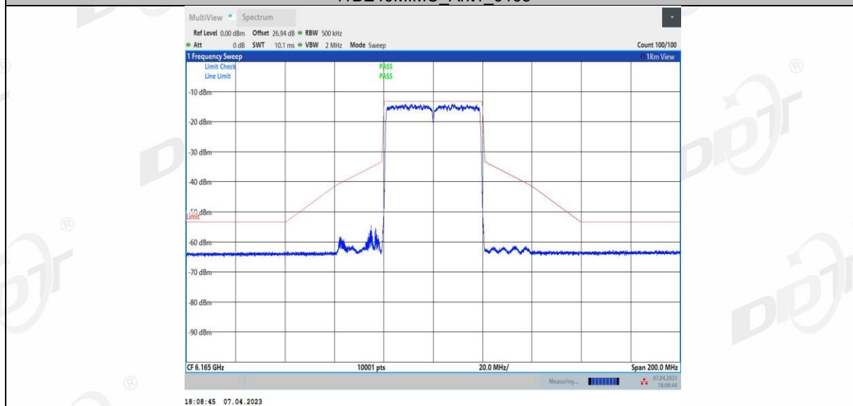
11BE40MIMO_Ant2_6165
