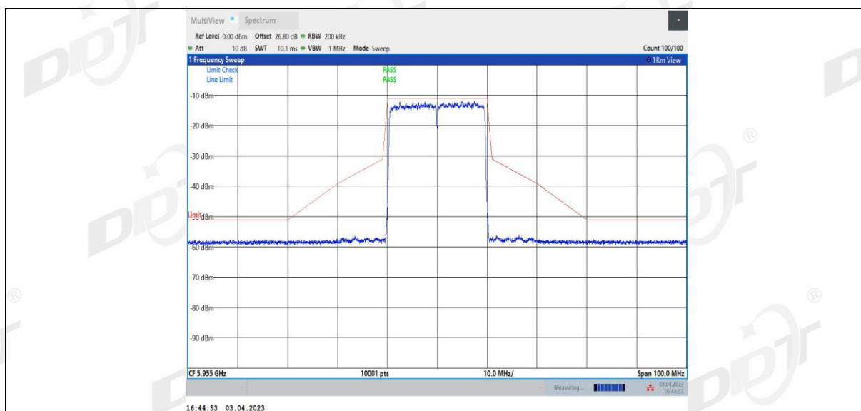
11BE20MIMO_Ant2_5955
