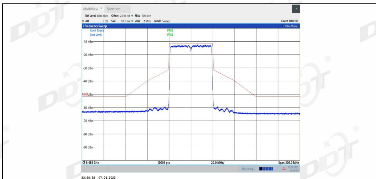
11BE40MIMO_Ant3_6485
