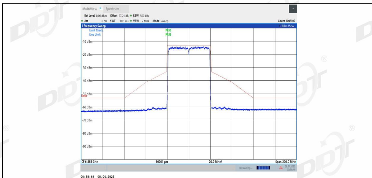
11BE40MIMO_Ant4_6885
