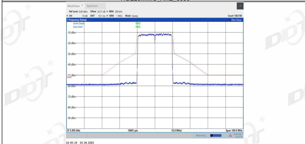
11BE20MIMO_Ant3_5955
