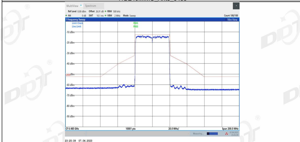
11BE40MIMO_Ant4_6485
