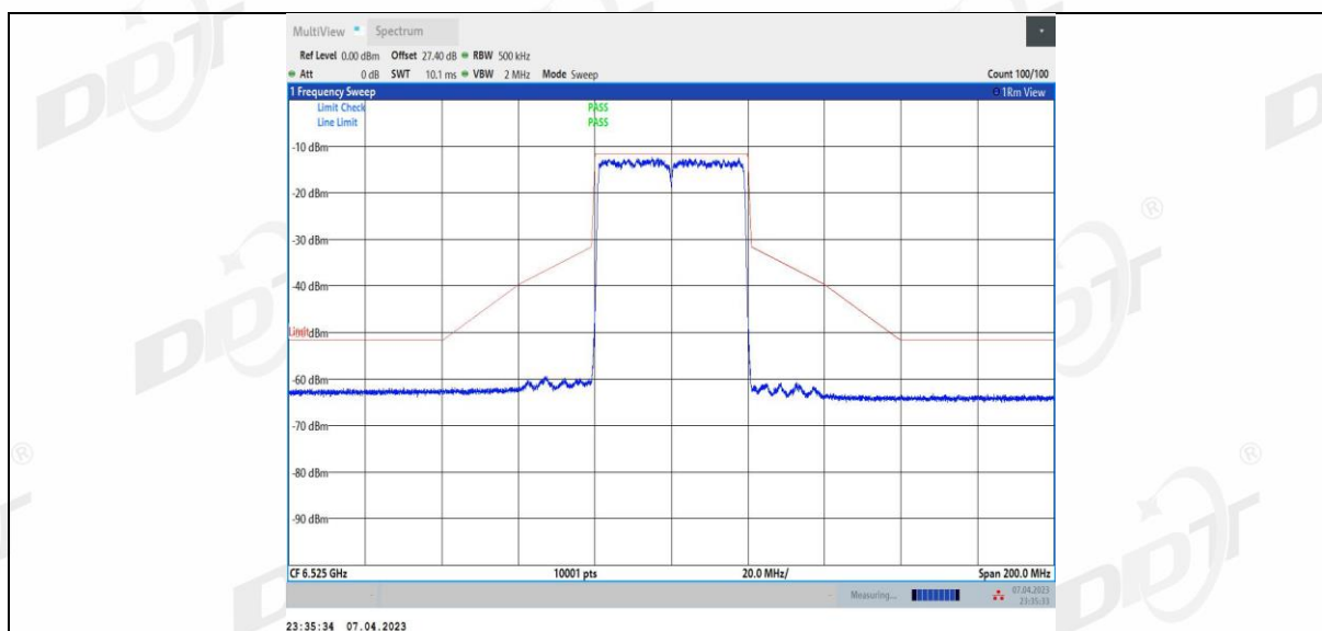
11BE40MIMO_Ant2_6525
