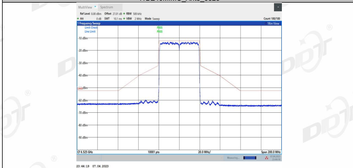
11BE40MIMO_Ant4_6525
