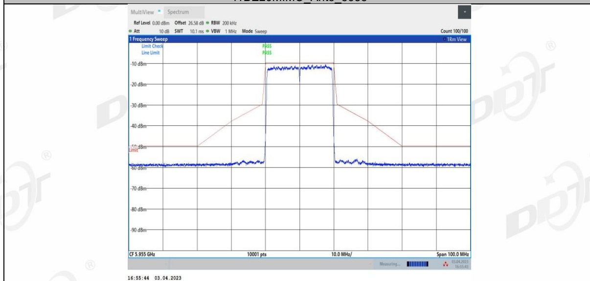
11BE20MIMO_Ant4_5955
