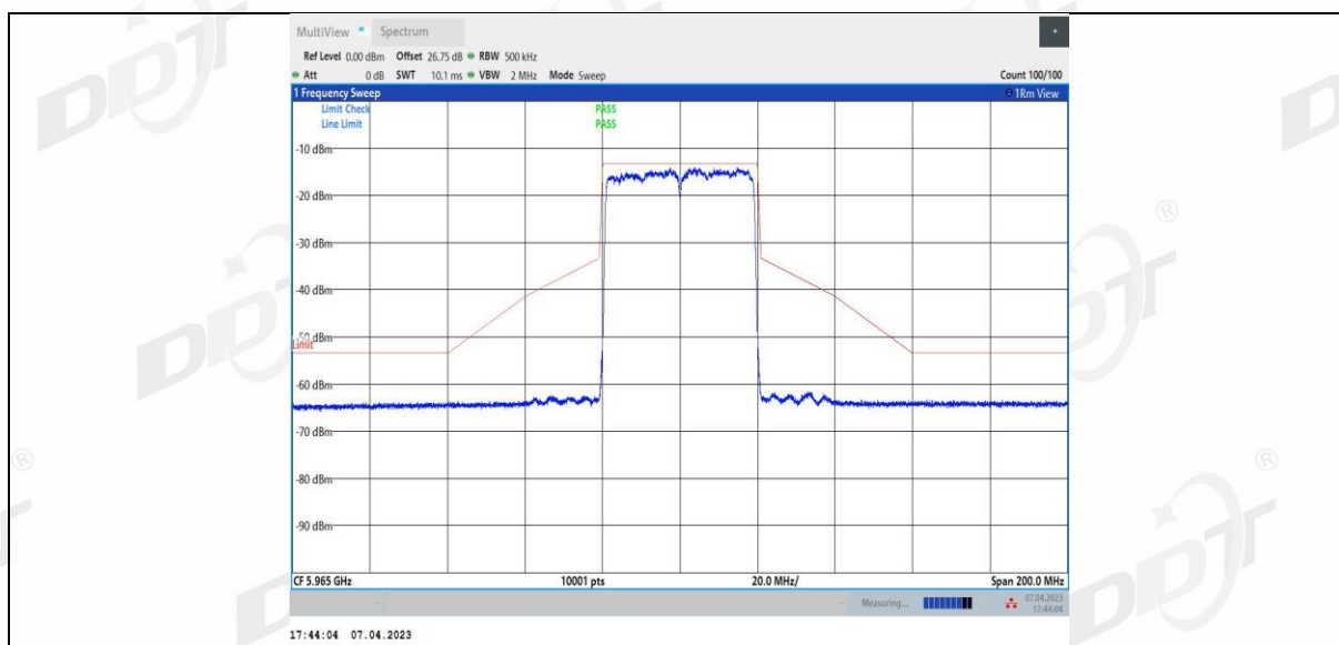
11BE40MIMO_Ant4_5965
