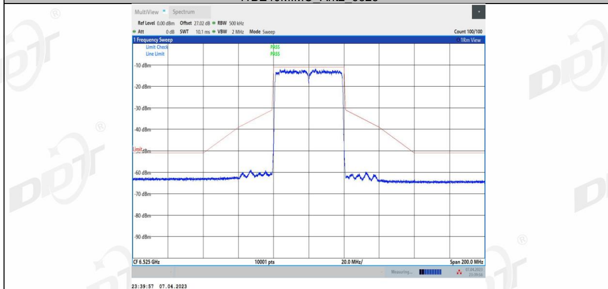
11BE40MIMO_Ant3_6525
