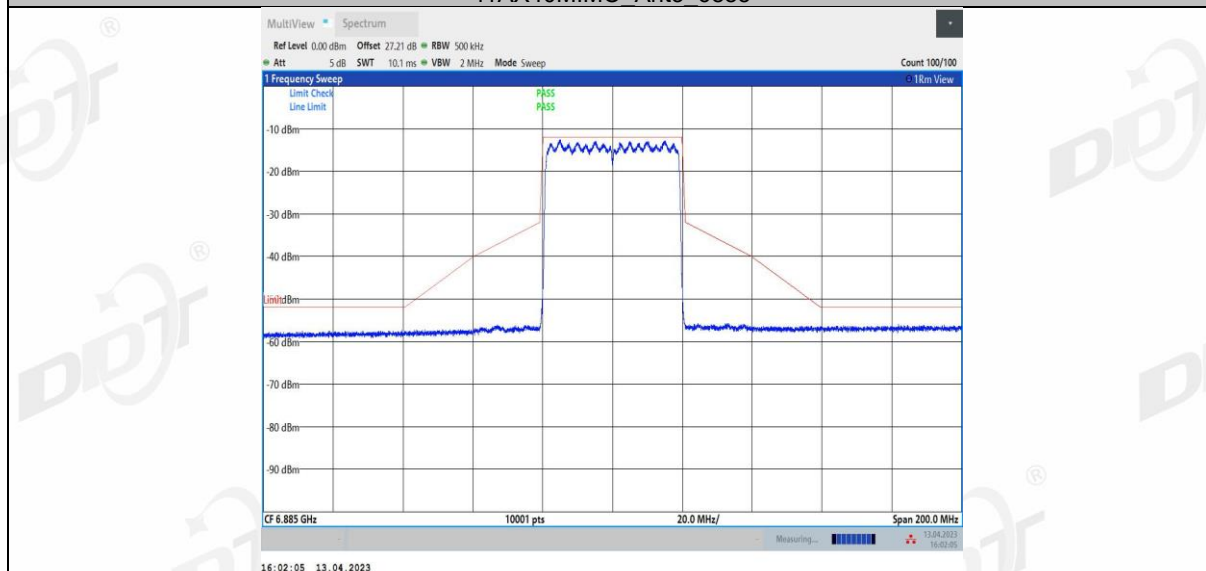
11AX40MIMO_Ant4_6885
