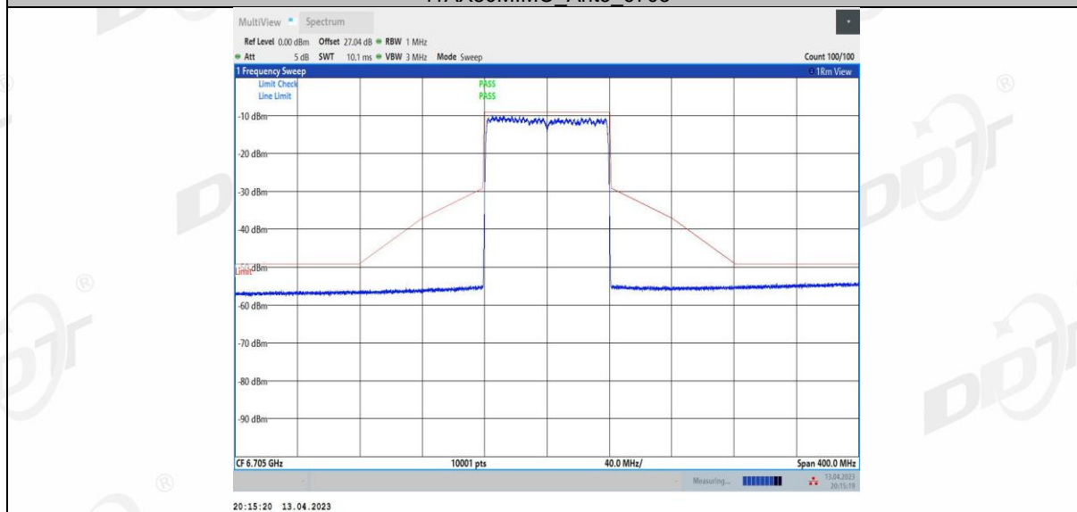
11AX80MIMO_Ant4_6705
