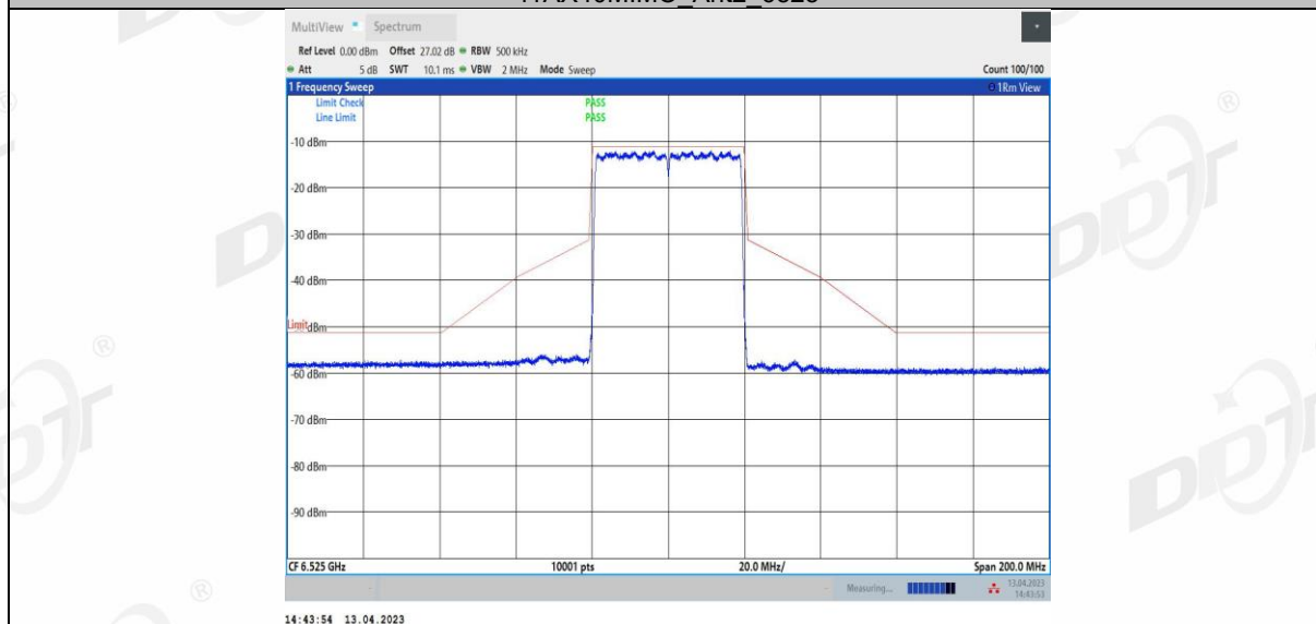
11AX40MIMO_Ant3_6525
