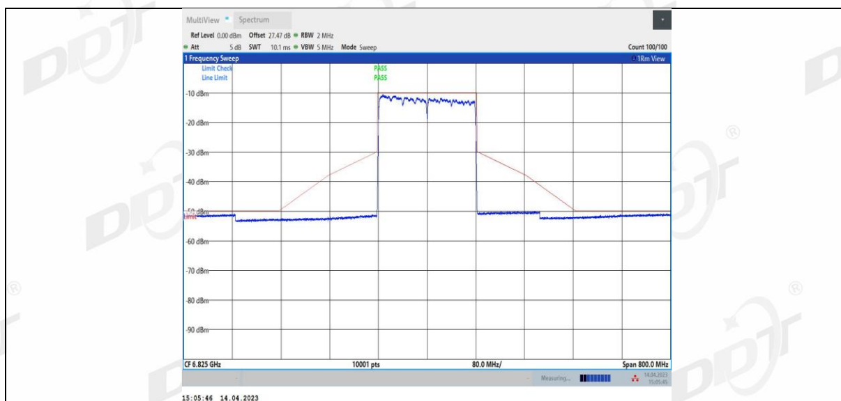
11AX160MIMO Ant4 6825
