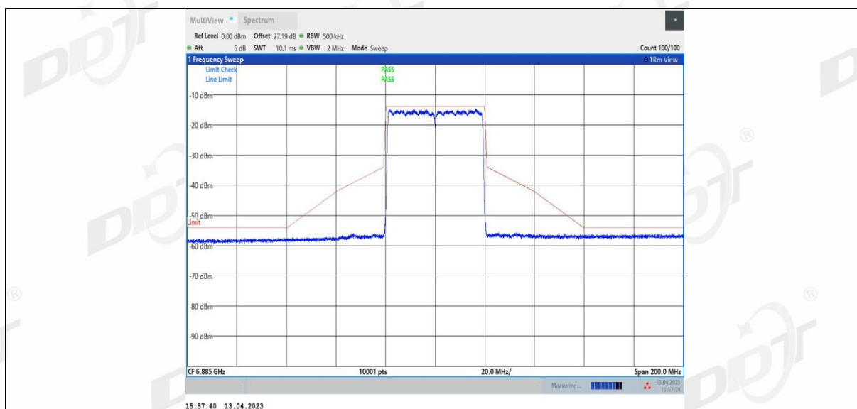
11AX40MIMO_Ant3_6885
