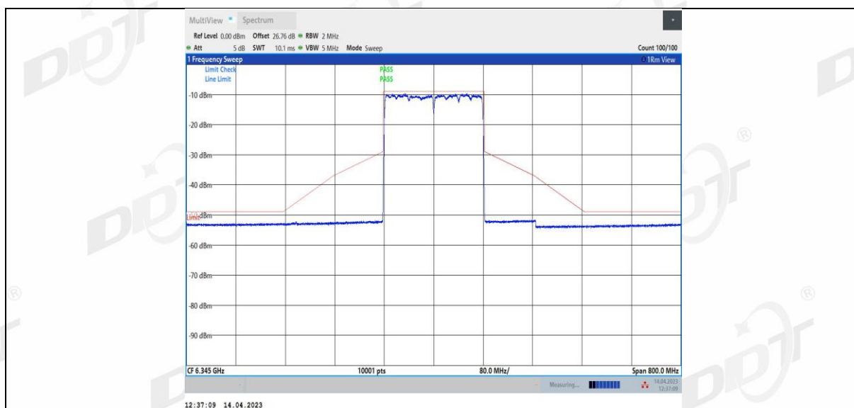
11AX160MIMO Ant4 6345
