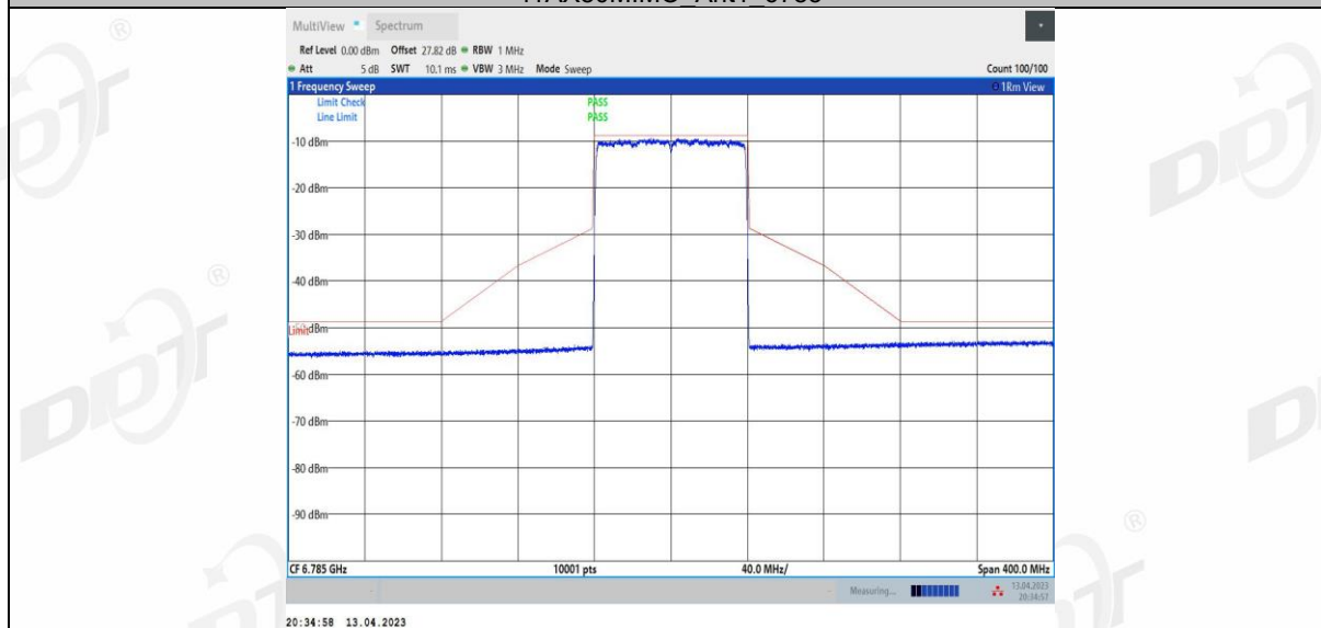
11AX80MIMO_Ant2_6785
