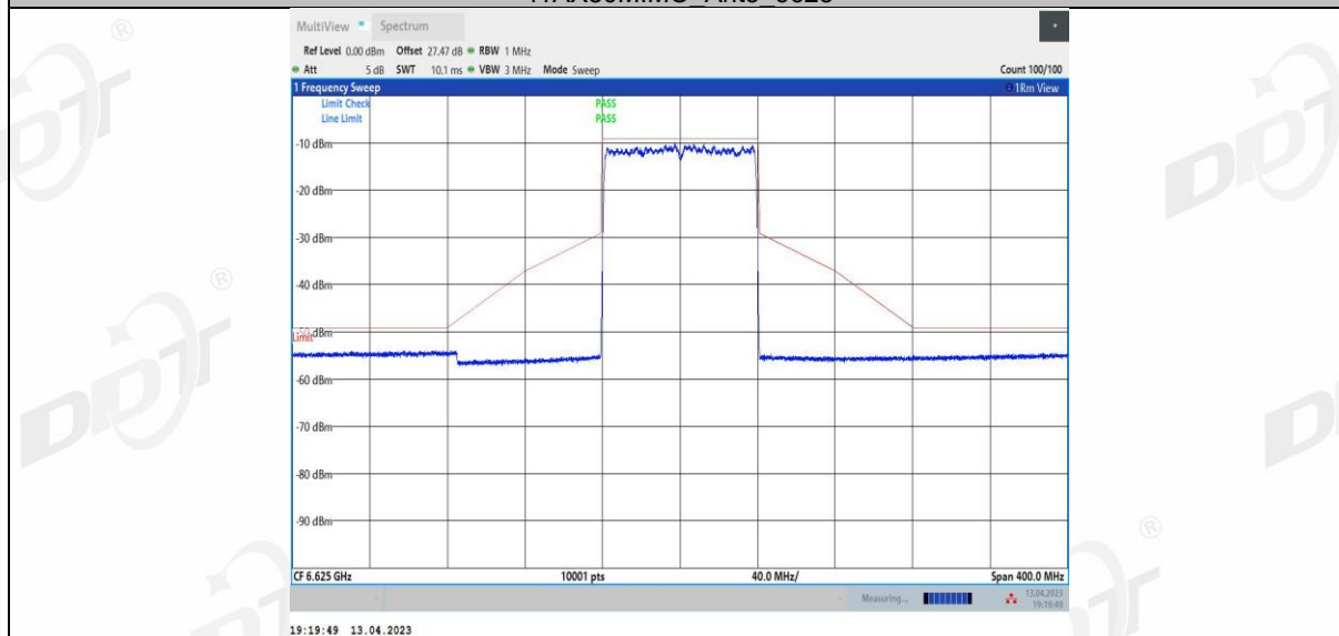
11AX80MIMO_Ant4_6625
