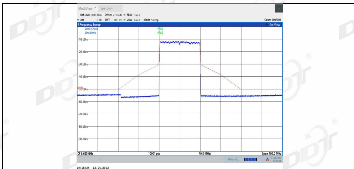
11AX80MIMO_Ant3_6625
