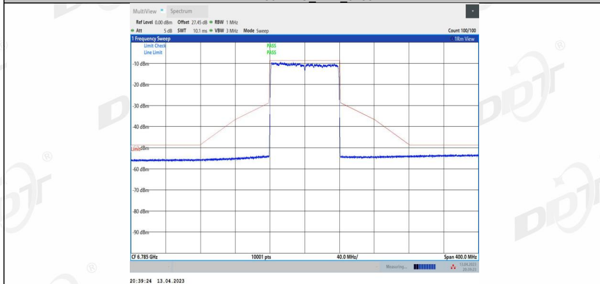
11AX80MIMO_Ant3_6785
