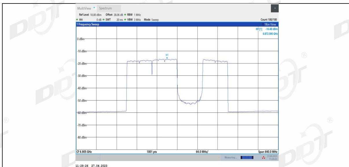
11BE320MIMO Ant1 6905 3*996 4
