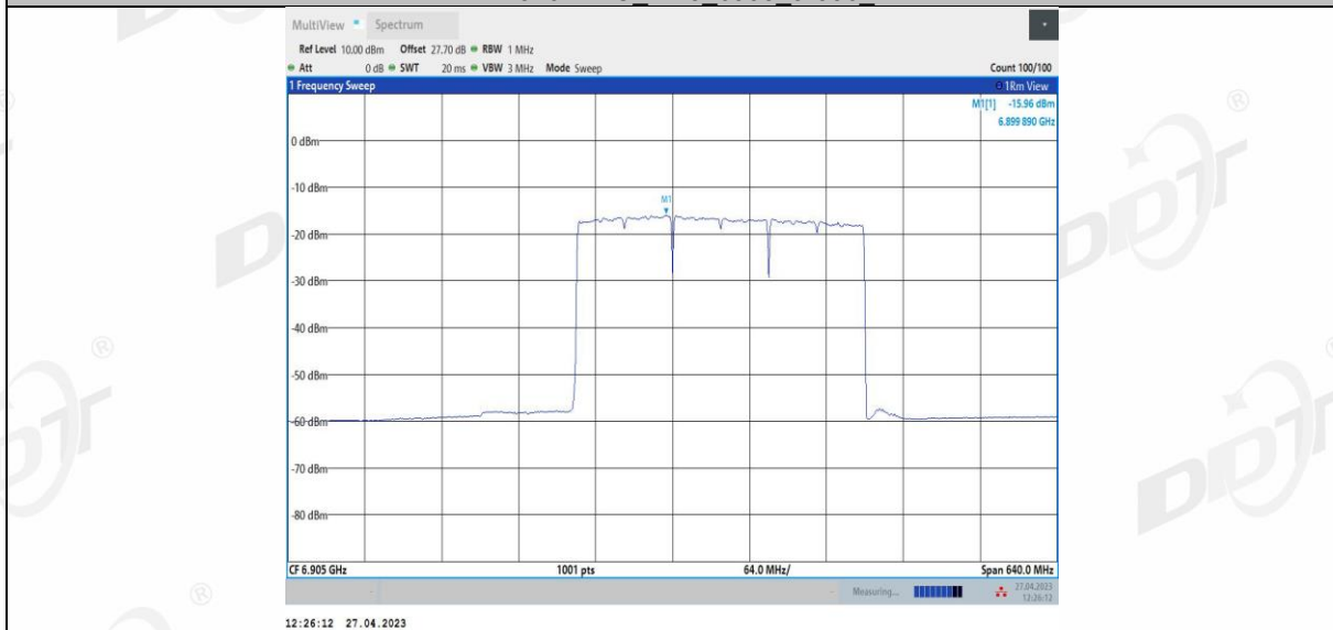
11BE320MIMO_Ant3_6905_3*996_2
