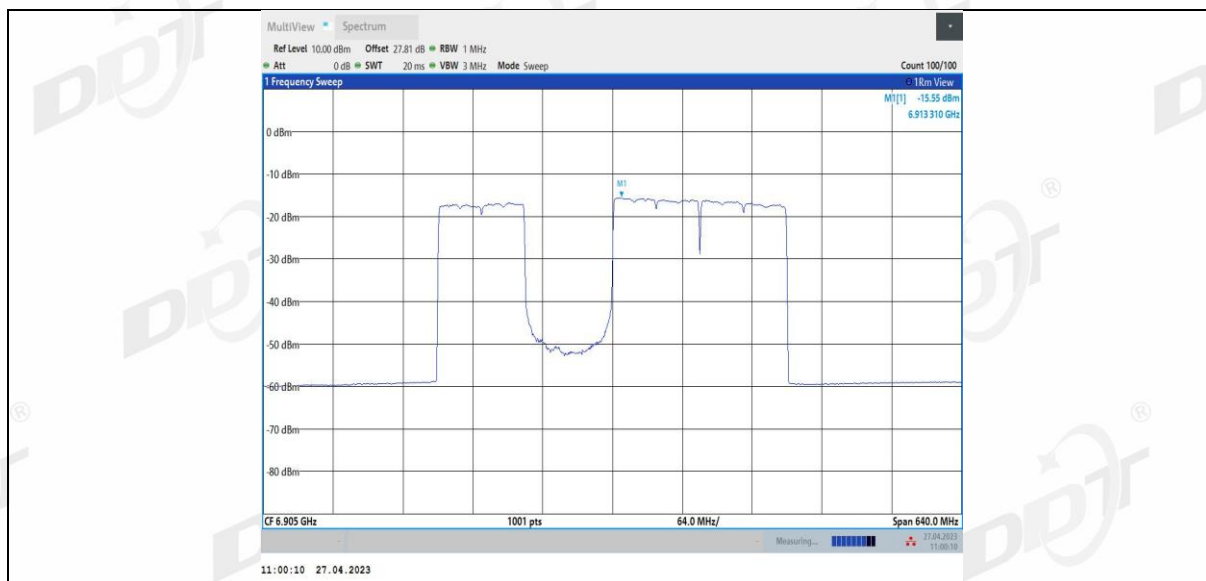
11BE320MIMO Ant3 6905 3*996 3
