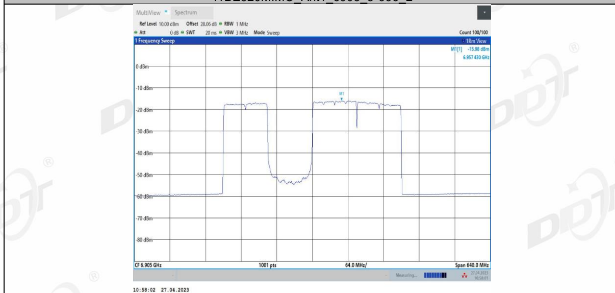
11BE320MIMO_Ant1_6905_3*996_3
