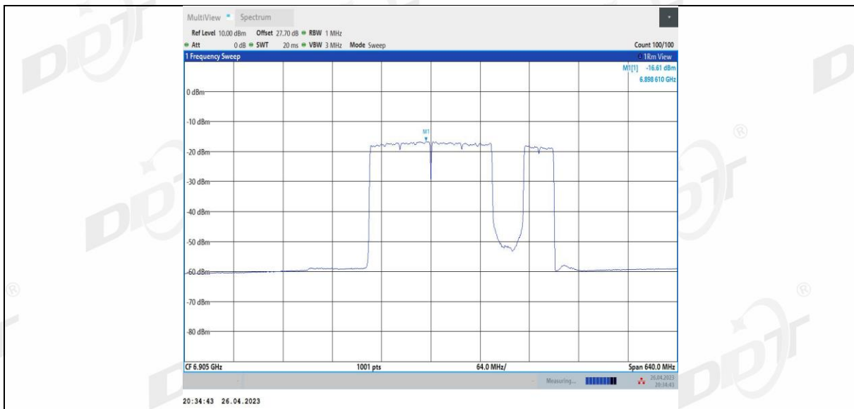
11BE320MIMO_Ant3_6905_2*996+484_12
