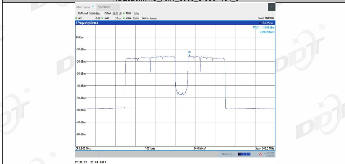
11BE320MIMO Ant1 6905 3*996+484 6
