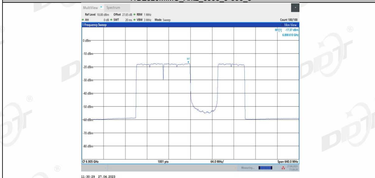
11BE320MIMO Ant2_6905_3*996_4
