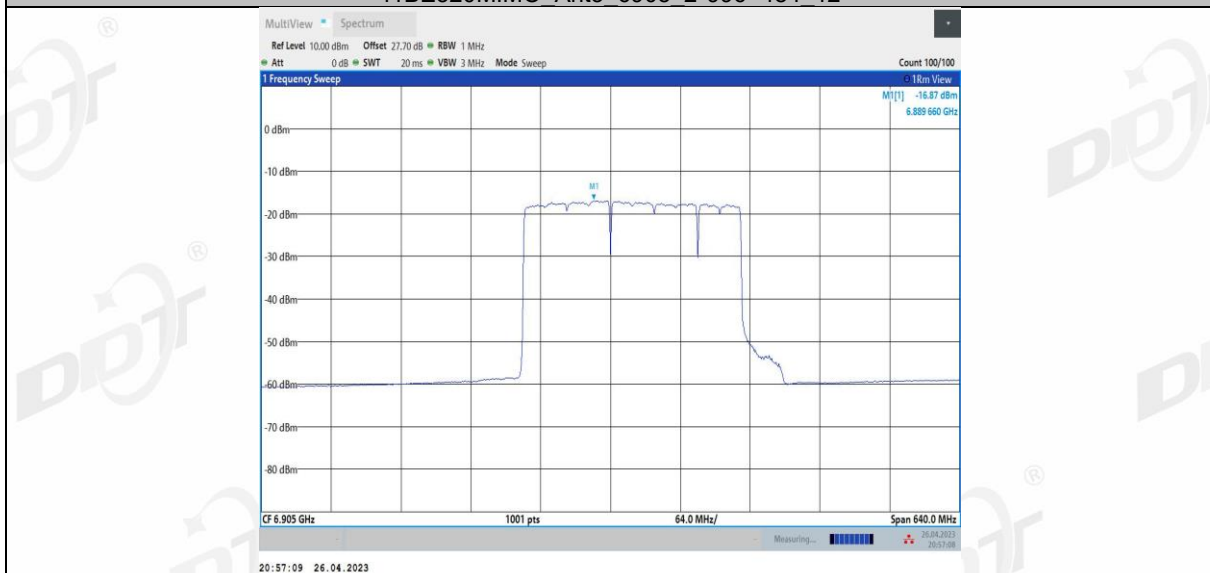
11BE320MIMO_Ant3_6905_3*996_1
