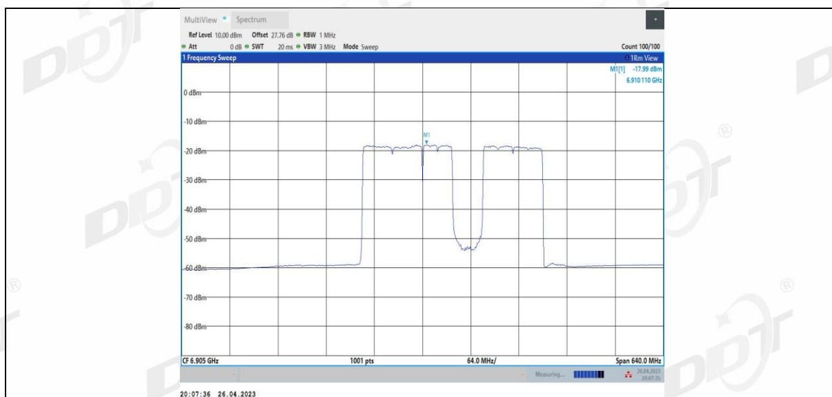
11BE320MIMO_Ant2_6905_2*996+484_11
