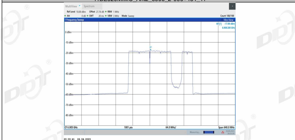
11BE320MIMO_Ant2_6905_2*996+484_12
