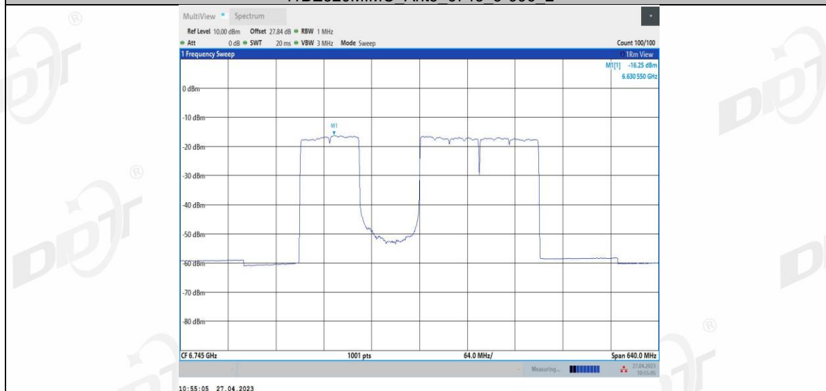
11BE320MIMO_Ant3_6745_3*996_3
