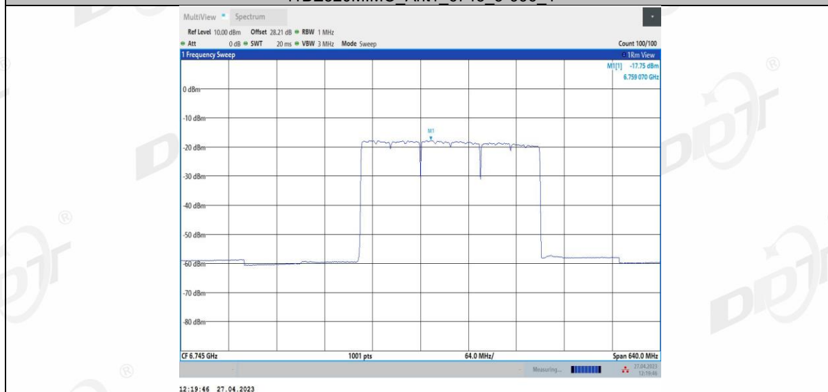
11BE320MIMO_Ant1_6745_3*996_2
