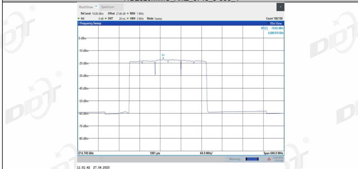
11BE320MIMO Ant2 6745 3*996+484 5
