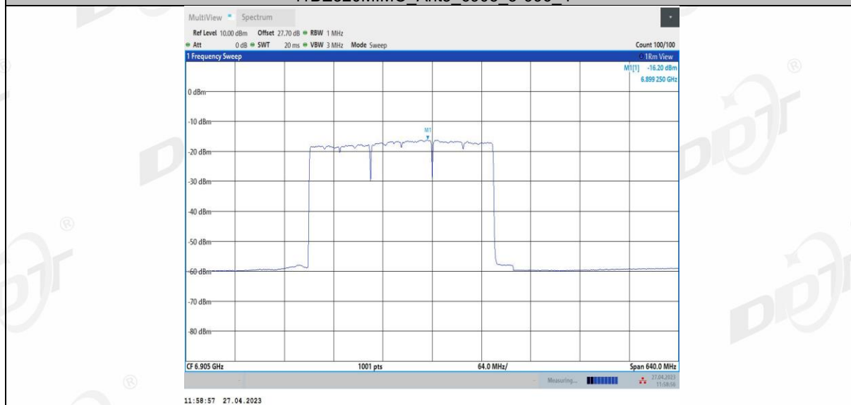
11BE320MIMO Ant3 6905 3*996+484 5
