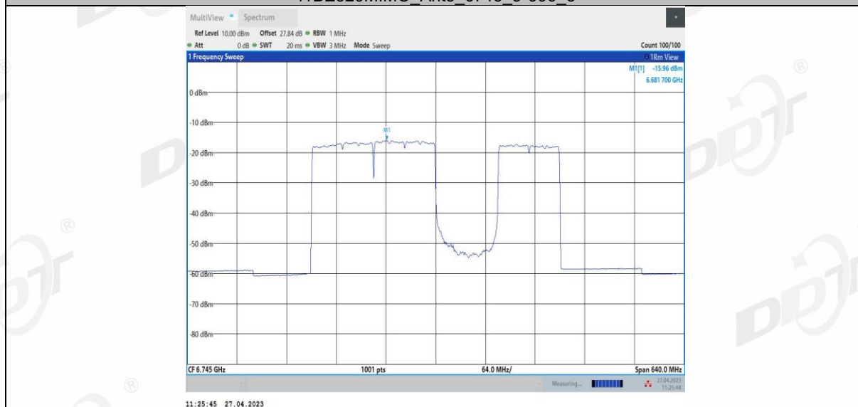
11BE320MIMO_Ant3_6745_3*996_4
