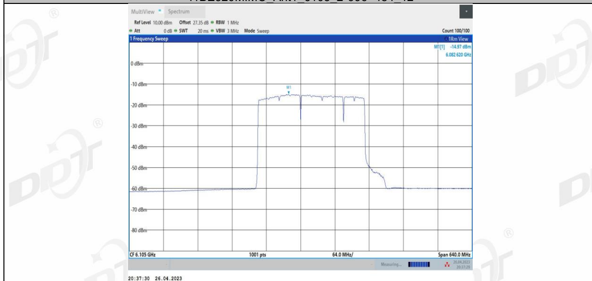
11BE320MIMO_Ant1_6105_3*996_1
