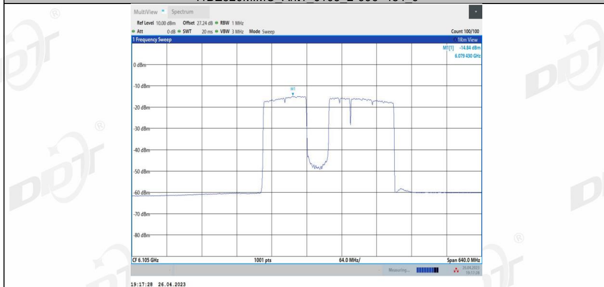
11BE320MIMO Ant1 6105 2*996+484 10
