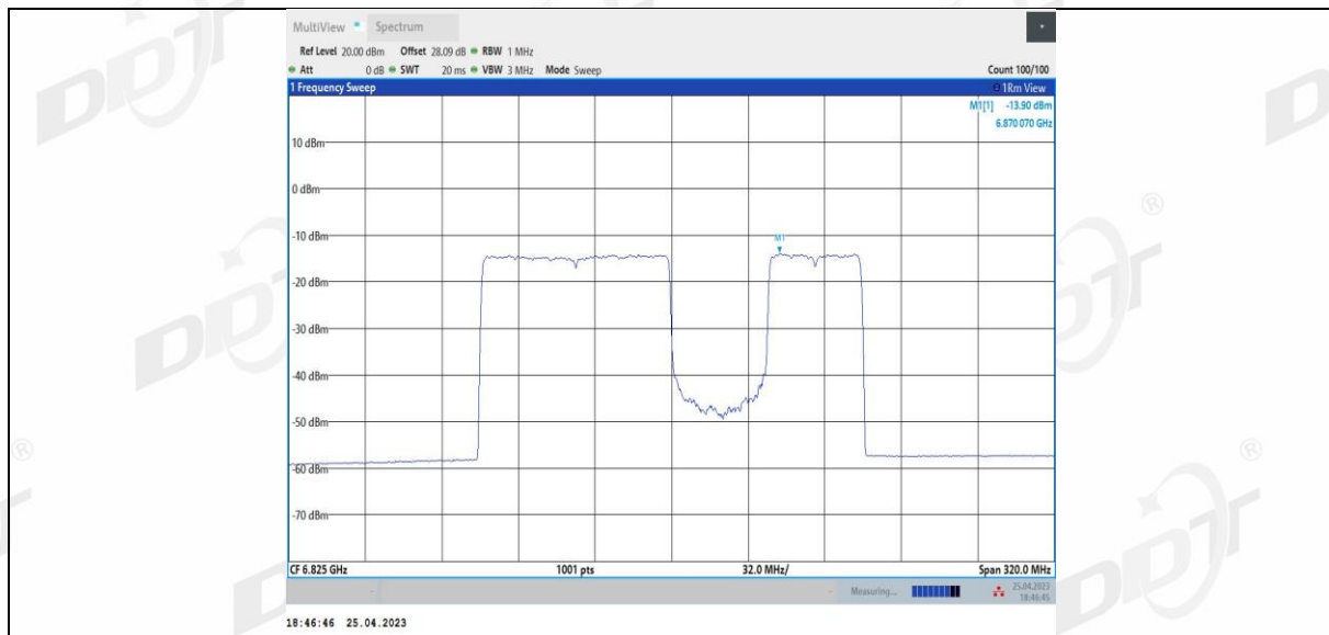
11BE160MIMO Ant4 6825_996+484_4
