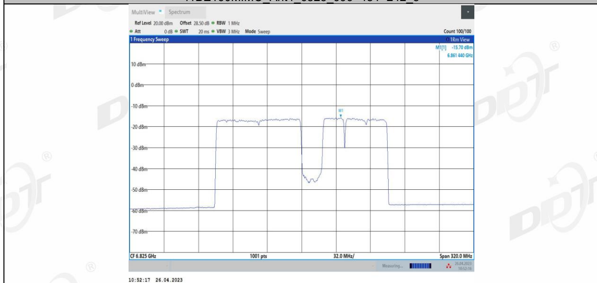
11BE160MIMO Ant4 6825_996+484+242_6
