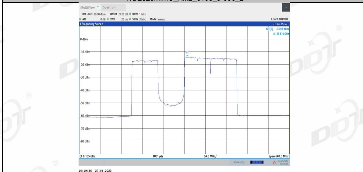
11BE320MIMO_Ant2_6105_3*996_3
