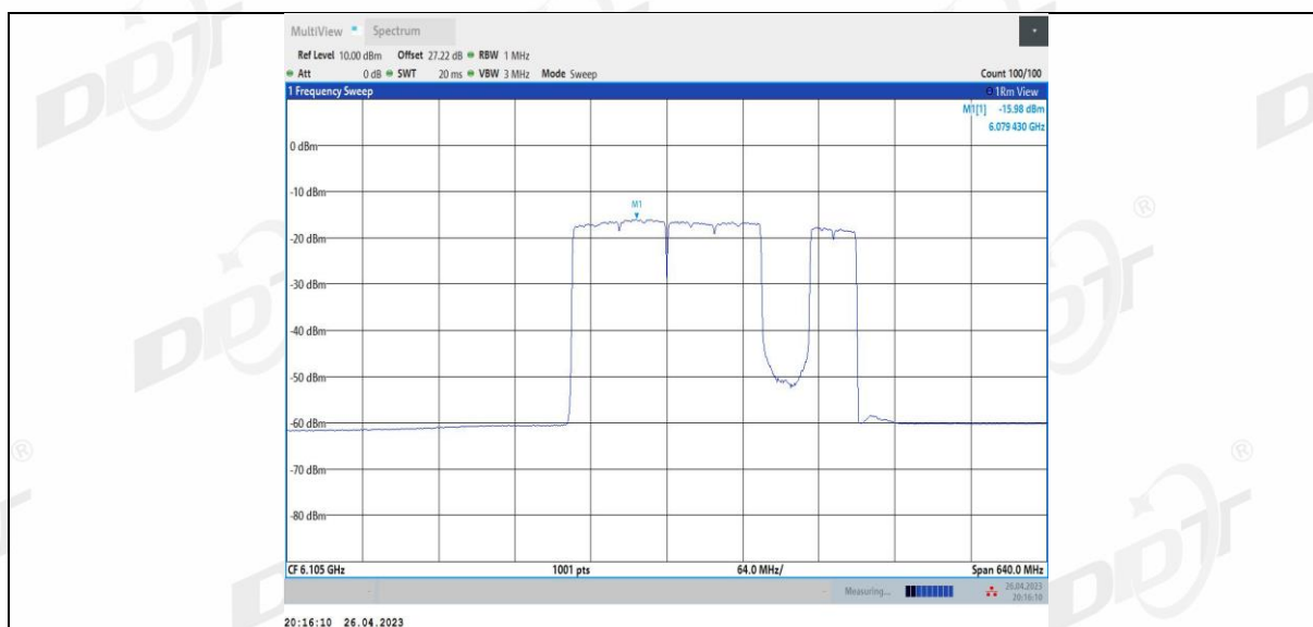
11BE320MIMO_Ant4_6105_2*996+484_12
