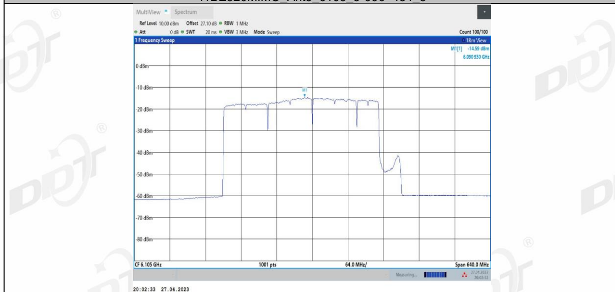
11BE320MIMO Ant4 6105 2*996+484 7
