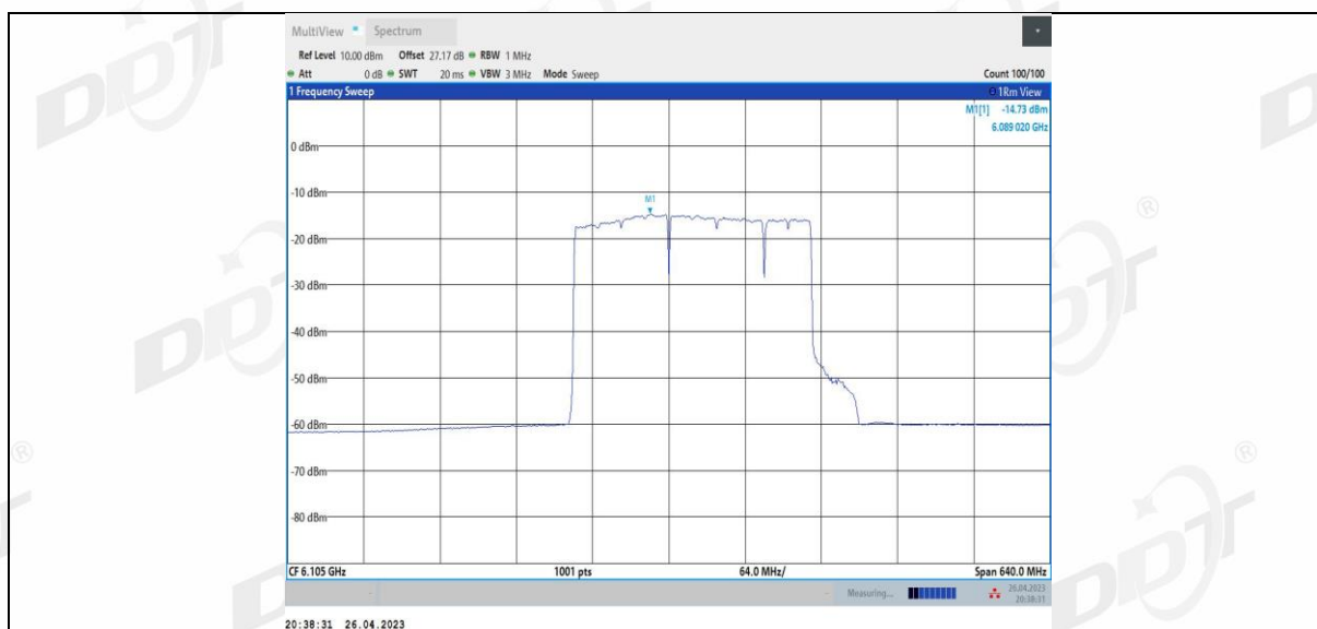
11BE320MIMO_Ant2_6105_3*996_1
