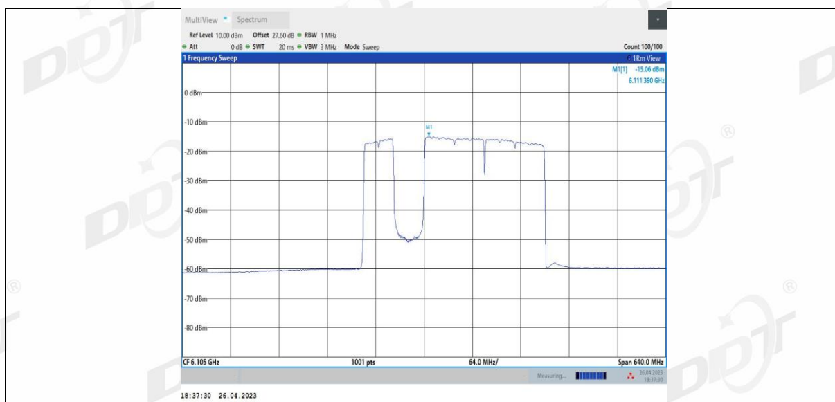
11BE320MIMO Ant1 6105 2*996+484 9
