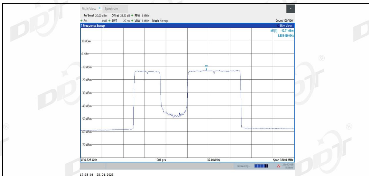
11BE160MIMO Ant3 6825 996+484_3
