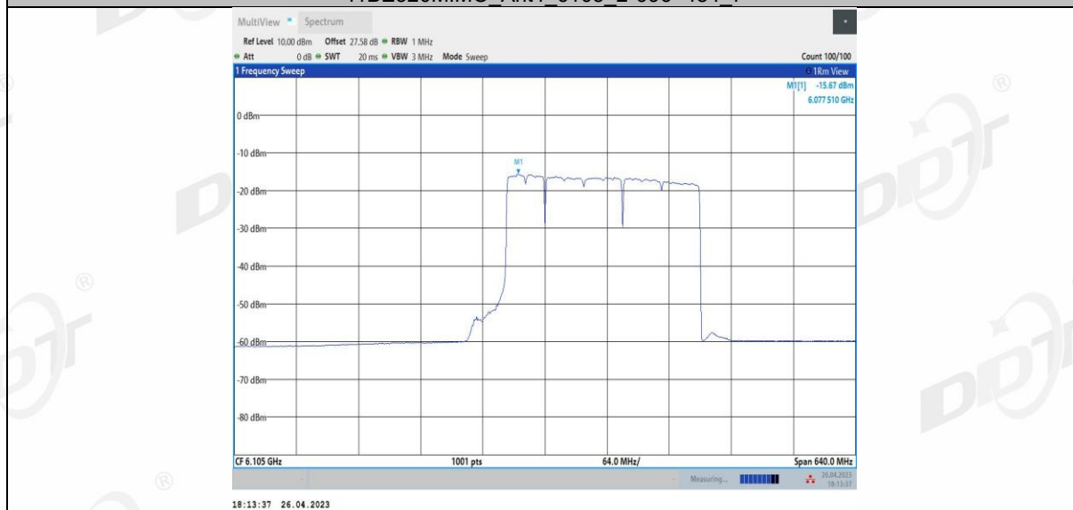
11BE320MIMO Ant4 6105 2*996+484 8
