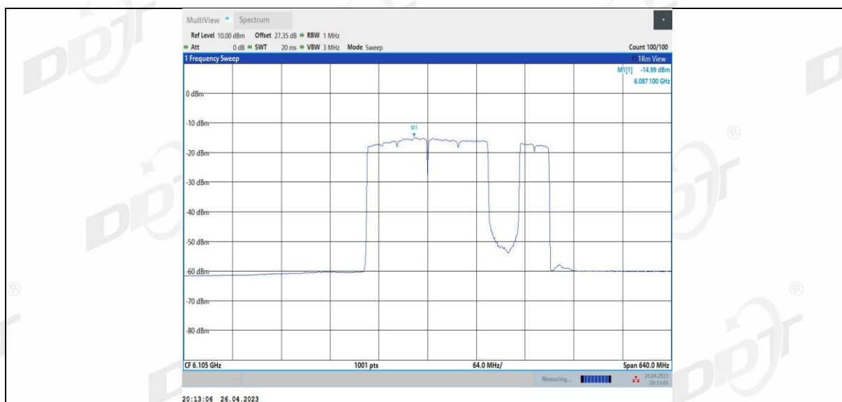
11BE320MIMO_Ant1_6105_2*996+484_12
