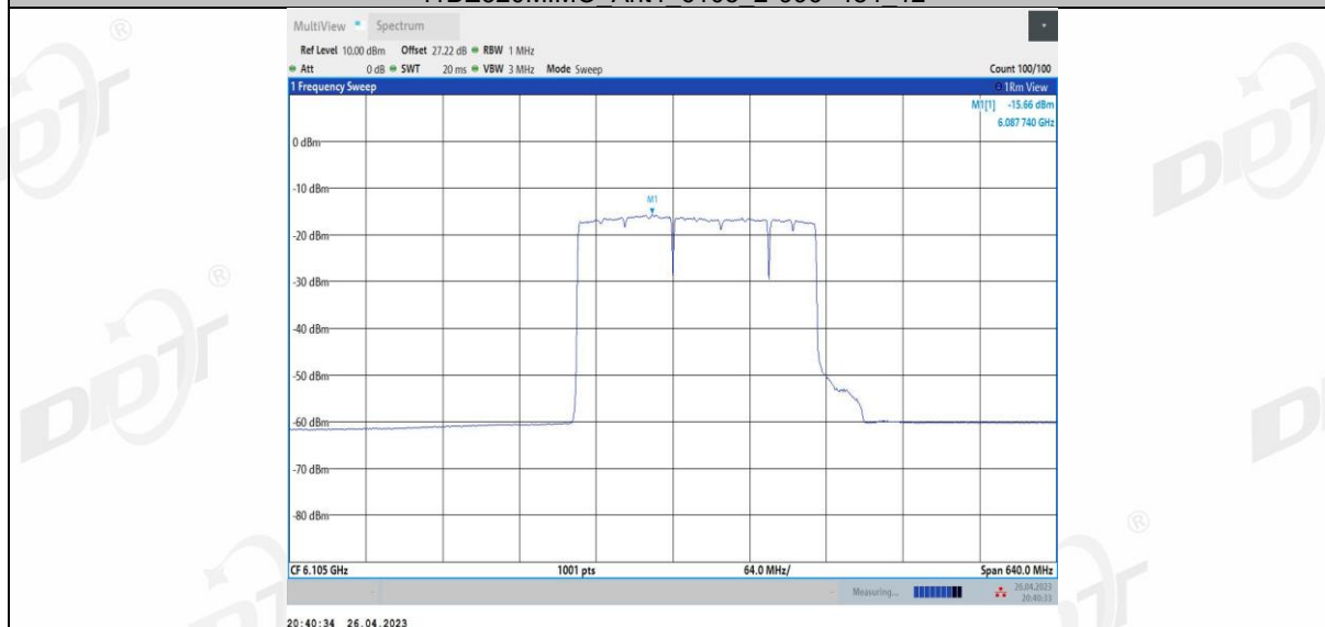
11BE320MIMO_Ant4_6105_3*996_1
