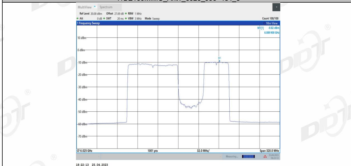
11BE160MIMO Ant1_6025_996+484_4
