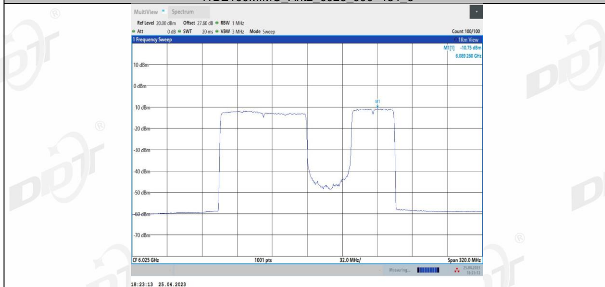
11BE160MIMO Ant2 6025 996+484_4
