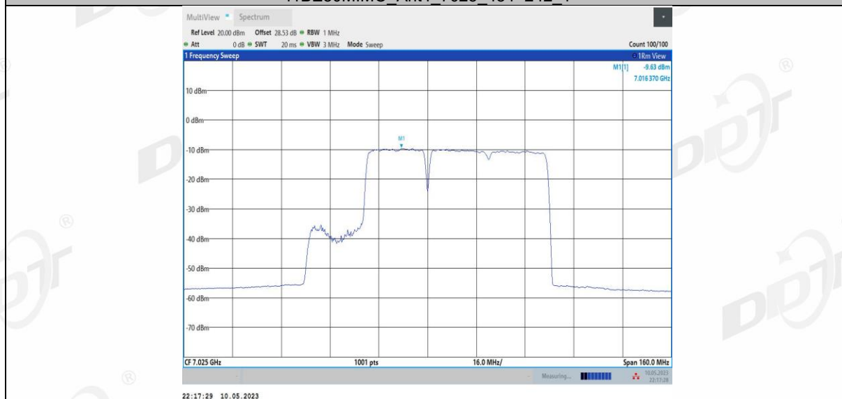
11BE80MIMO Ant4 7025 484+242 2
