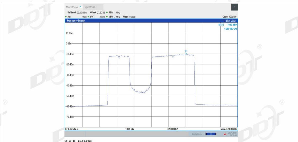
11BE160MIMO Ant2 6025 996+484_3
