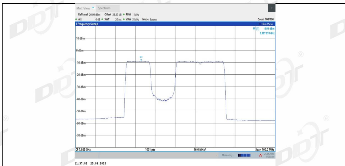
11BE80MIMO Ant1 7025 484+242_3
