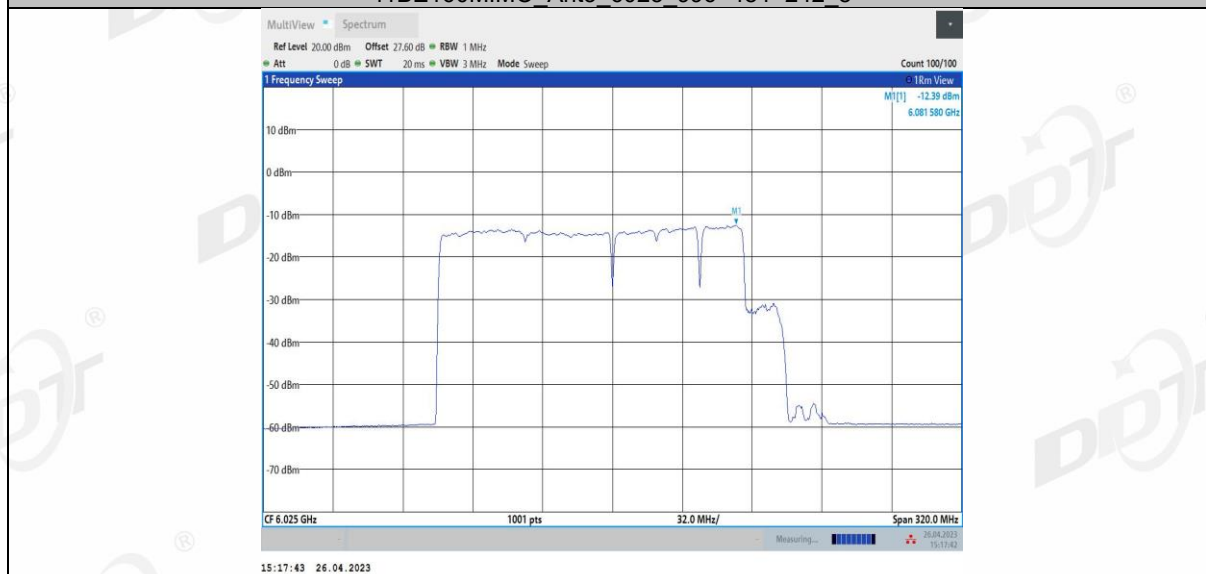
11BE160MIMO Ant4 6025_996+484_1
