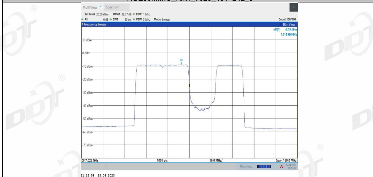
11BE80MIMO Ant1 7025 484+242_4
