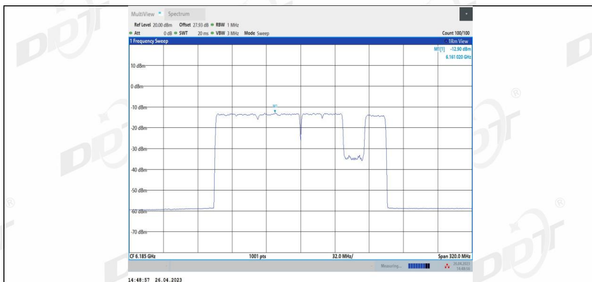
11BE160MIMO Ant3 6185 996+484+242 8
