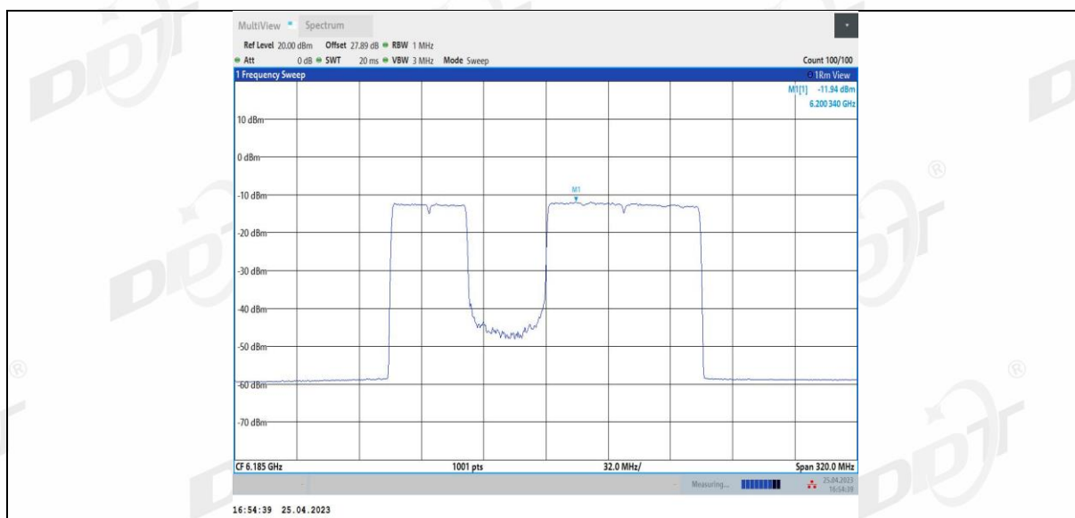
11BE160MIMO Ant1_6185_996+484_3
