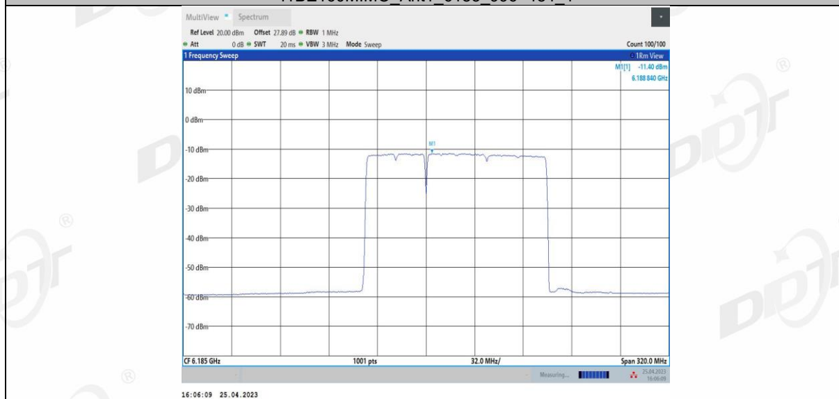
11BE160MIMO Ant1_6185 996+484_2
