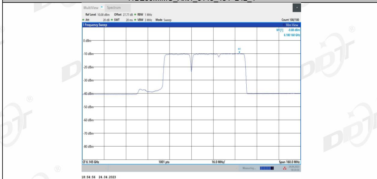
11BE80MIMO_Ant4_6145_484+242_2
