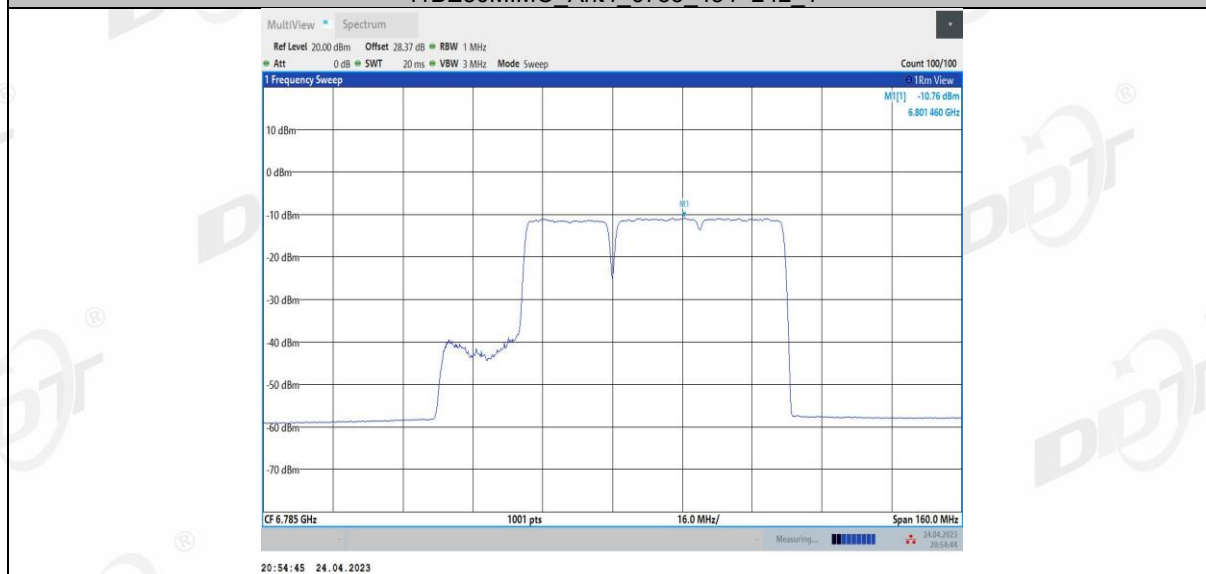
11BE80MIMO Ant4 6785 484+242 2
