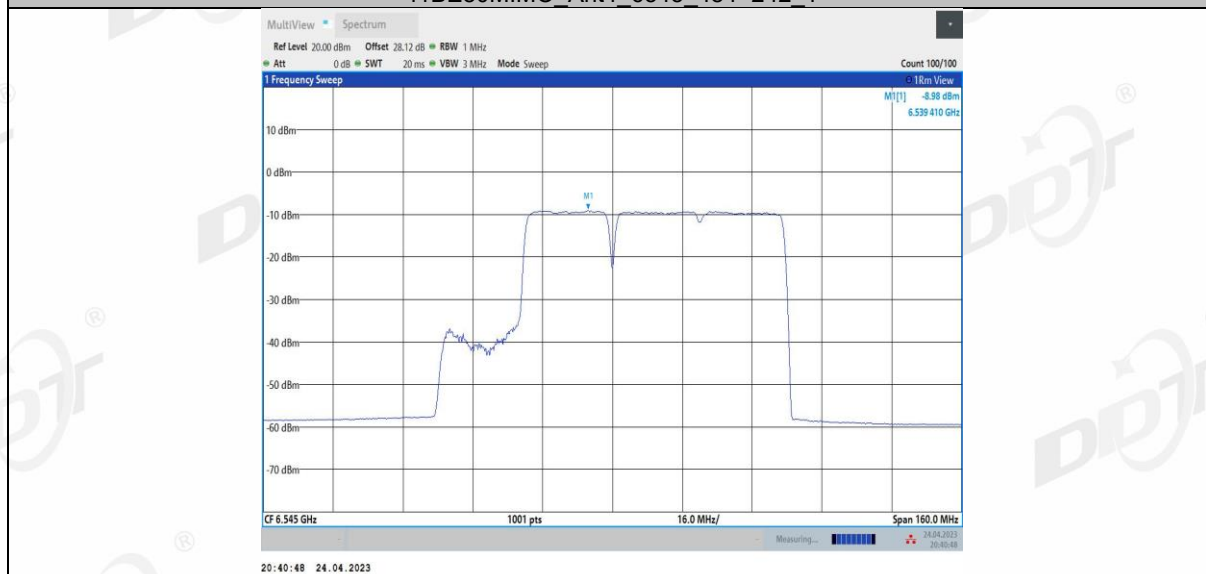
11BE80MIMO_Ant4_6545_484+242_2
