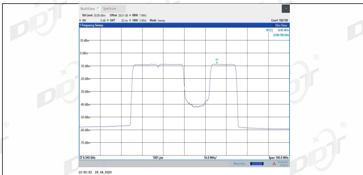
11BE80MIMO_Ant3_6545_484+242_4
