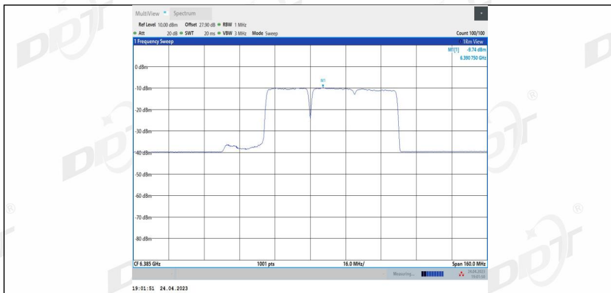
11BE80MIMO Ant4 6385 484+242 2
