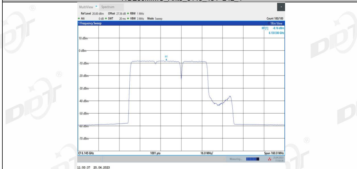
11BE80MIMO_Ant4_6145_484+242_1
