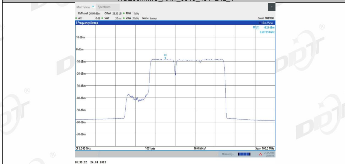
11BE80MIMO Ant1 6545 484+242 2
