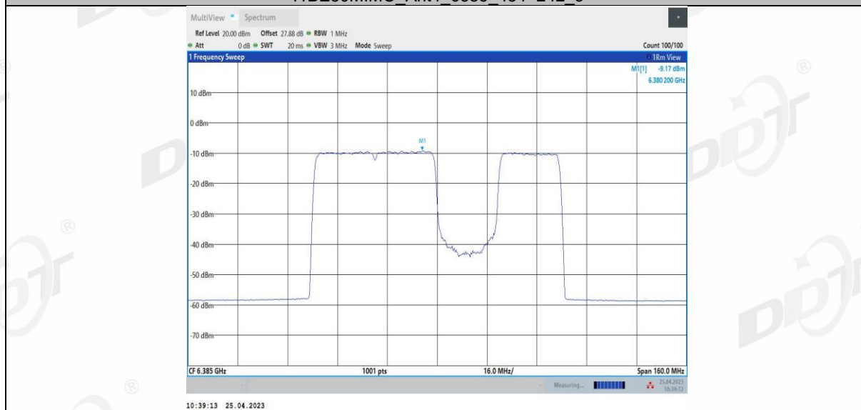
11BE80MIMO Ant4 6385 484+242 4
