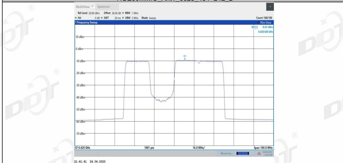
11BE80MIMO Ant1 6625 484+242 3
