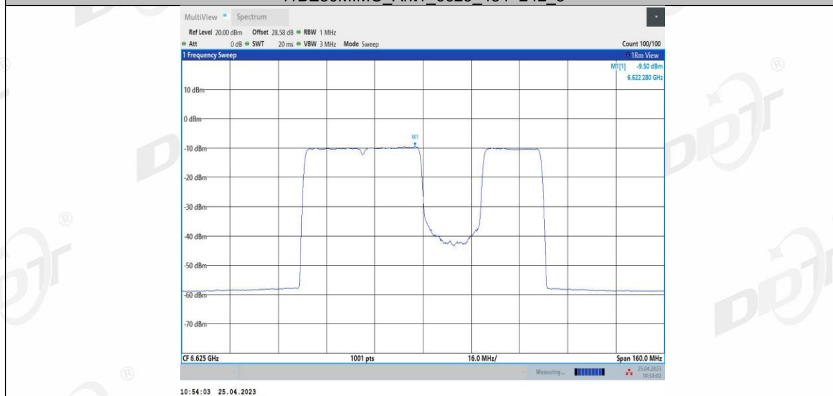
11BE80MIMO Ant1 6625 484+242 4
