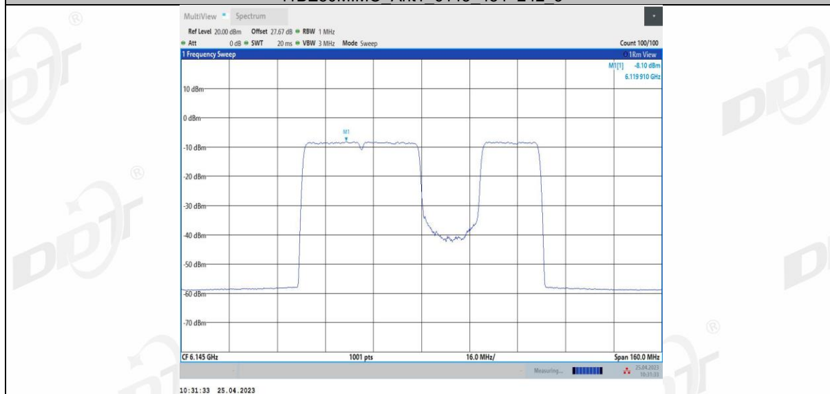
11BE80MIMO Ant1 6145 484+242_4
