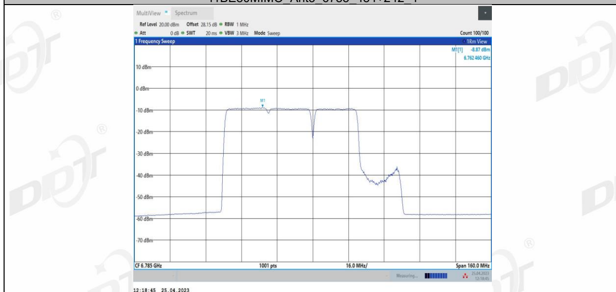
11BE80MIMO Ant4 6785 484+242 1
