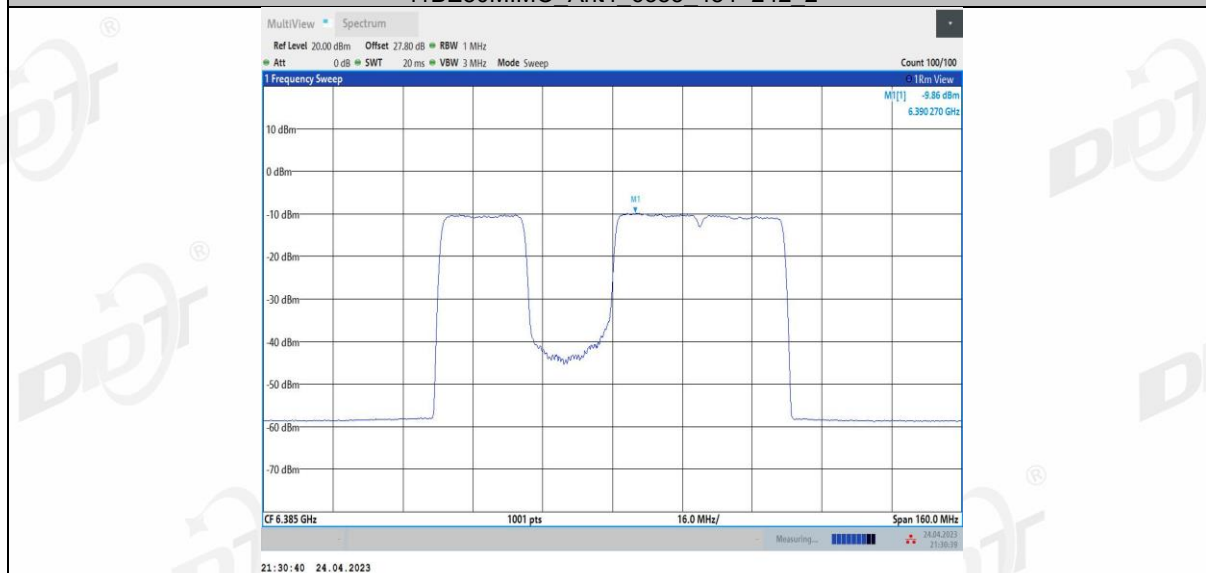
11BE80MIMO Ant4 6385 484+242 3
