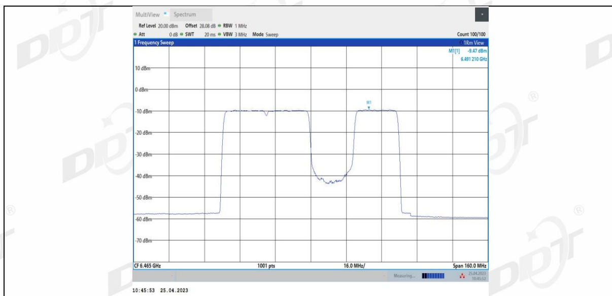
11BE80MIMO Ant4 6465 484+242 4
