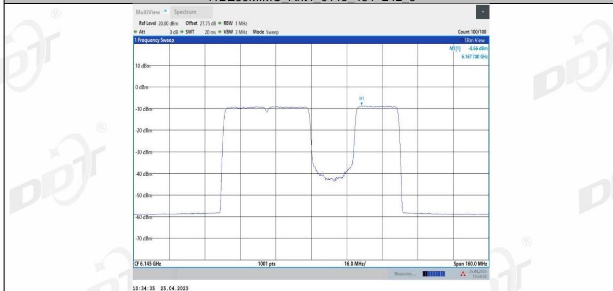
11BE80MIMO Ant4 6145 484+242_4
