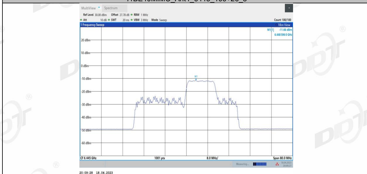
11BE40MIMO Ant4 6445 106+26 4
