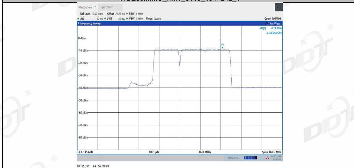
11BE80MIMO Ant1 6145 484+242 2
