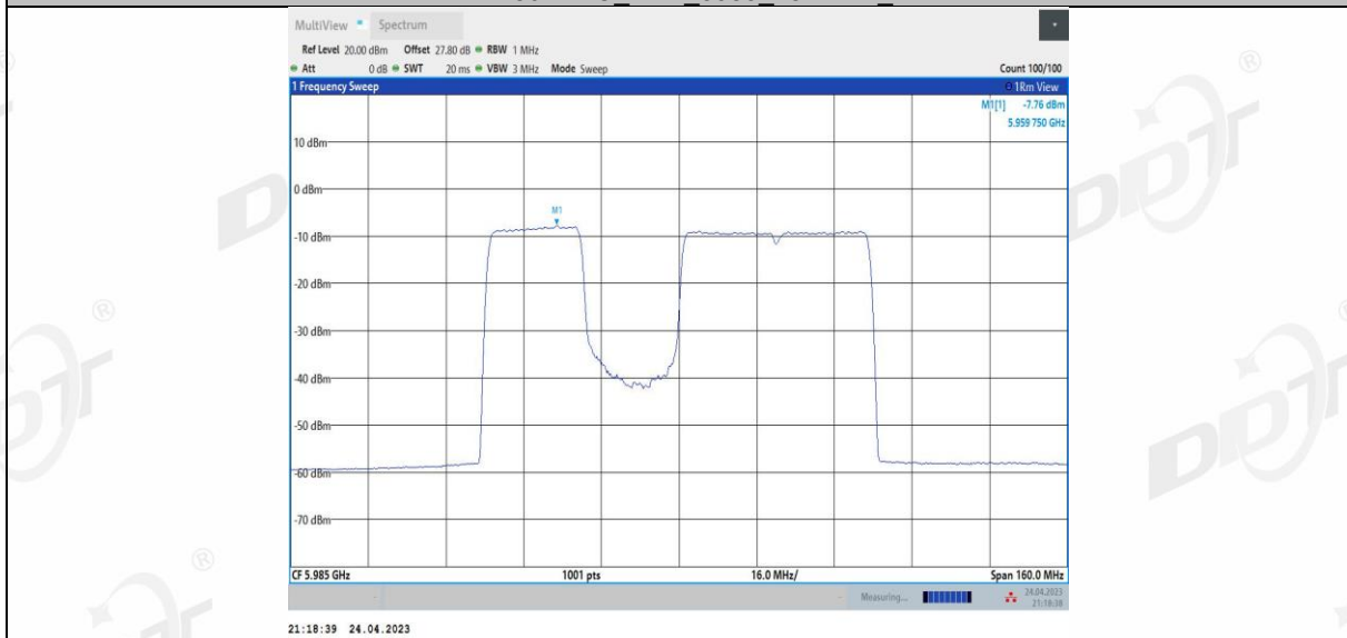
11BE80MIMO_Ant1_5985_484+242_3
