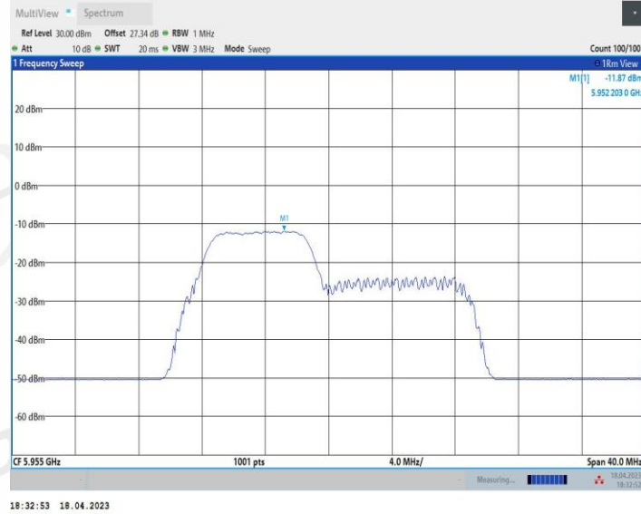
11BE20MIMO Ant1 5955 52+26 2
