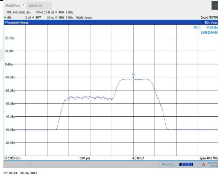
11BE20MIMO Ant1 5955 106+26 1
