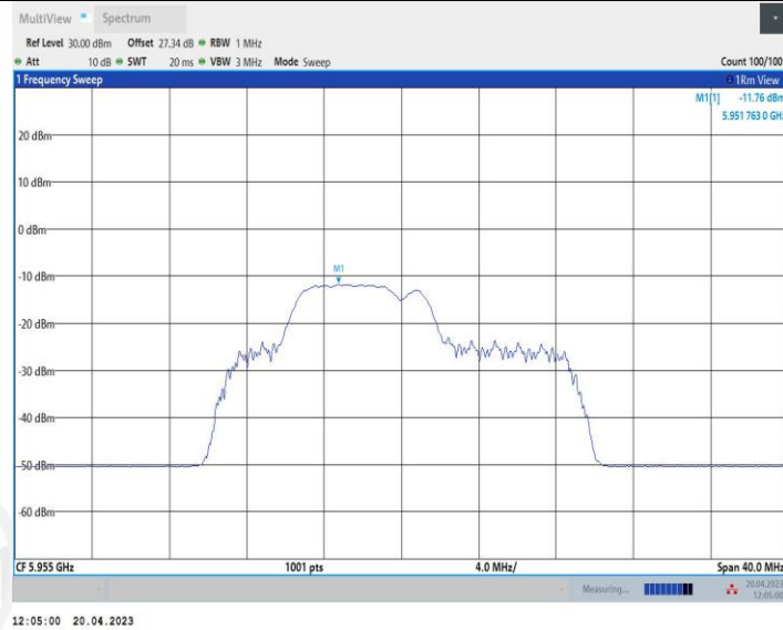
11BE20MIMO Ant1 5955 52+26 3
