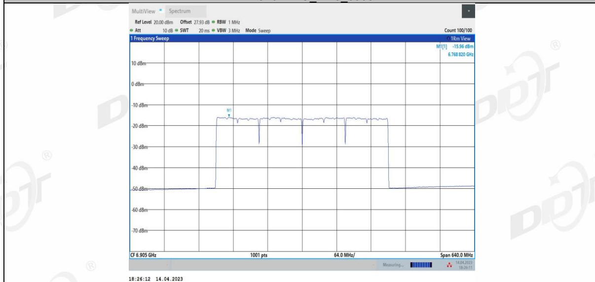
11BE320MIMO Ant4 6905
