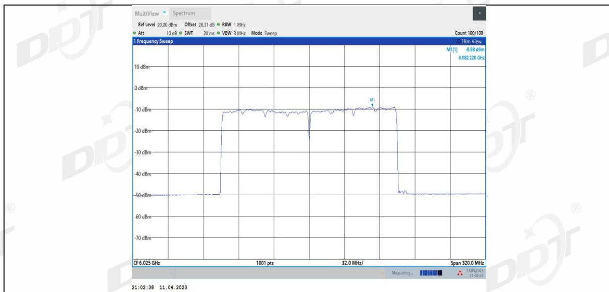
11BE160MIMO Ant4 6025
