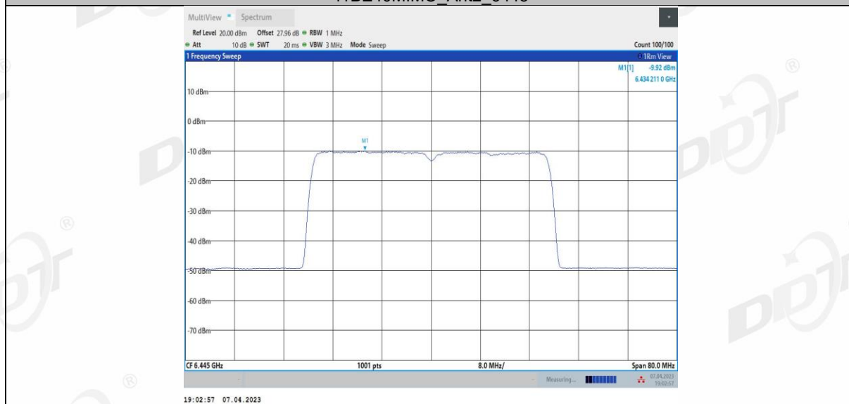
11BE40MIMO_Ant3_6445
