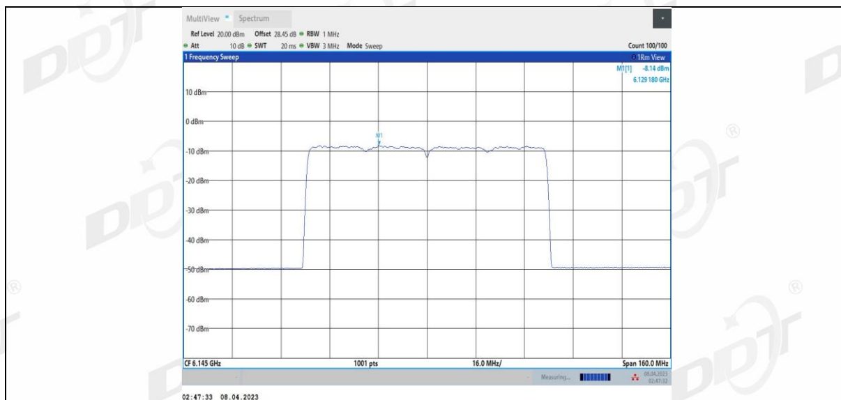
11BE80MIMO_Ant2_6145
