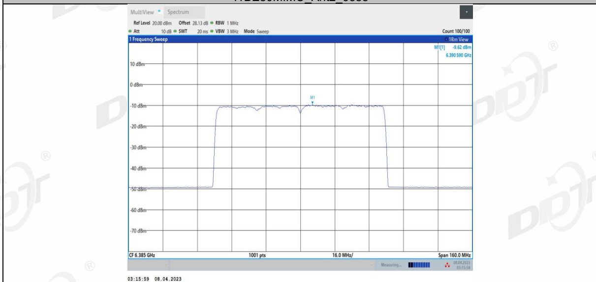
11BE80MIMO_Ant3_6385
