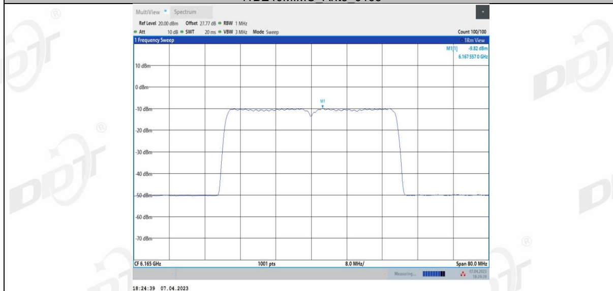
11BE40MIMO_Ant4_6165
