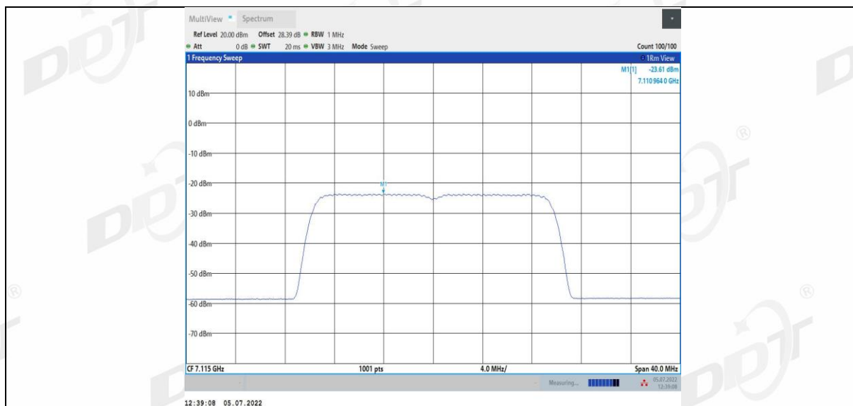
11BE20MIMO_Ant2_7115
