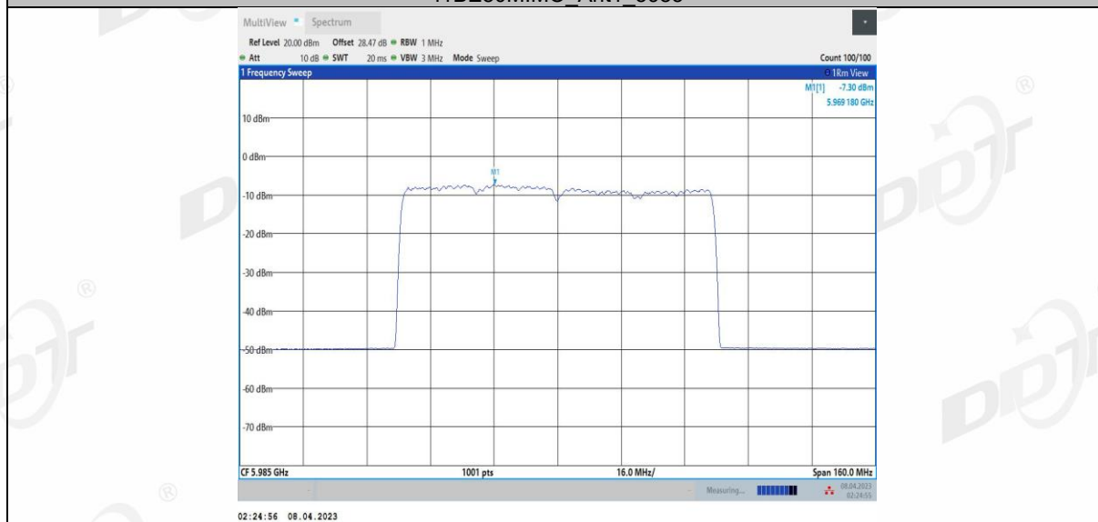
11BE80MIMO_Ant2_5985
