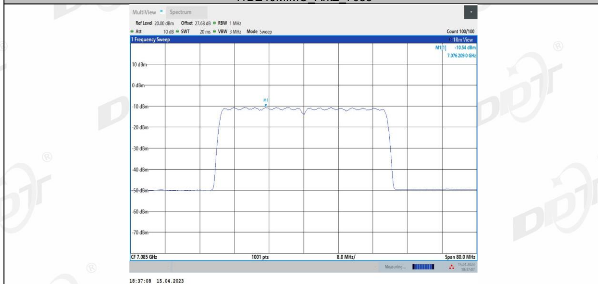
11BE40MIMO_Ant3_7085
