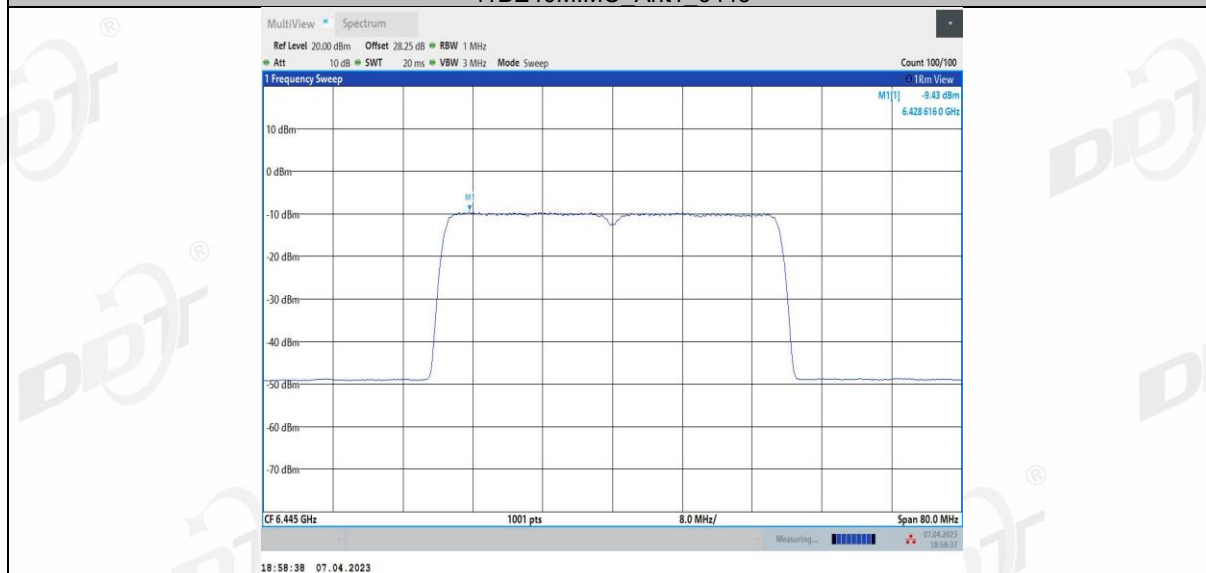
11BE40MIMO_Ant2_6445
