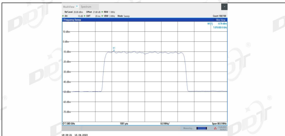
11BE40MIMO_Ant4_7085
