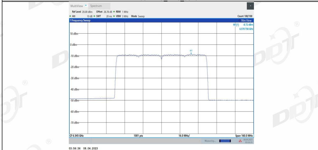
11BE80MIMO_Ant4_6545
