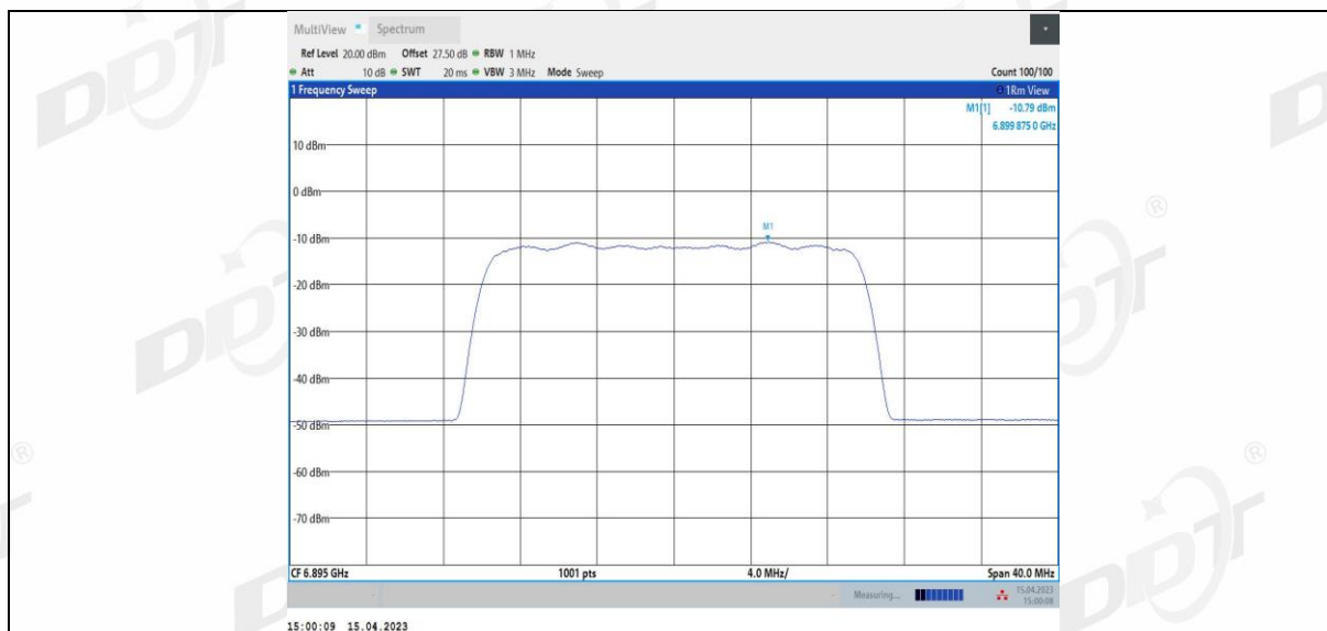
11BE20MIMO_Ant4_6895
