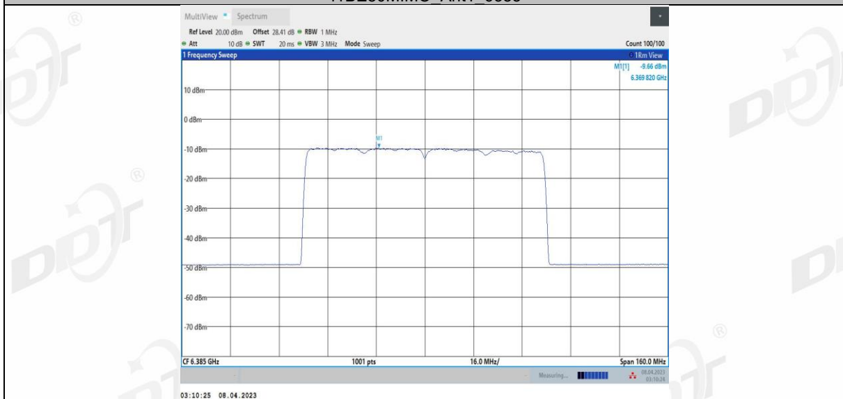
11BE80MIMO_Ant2_6385
