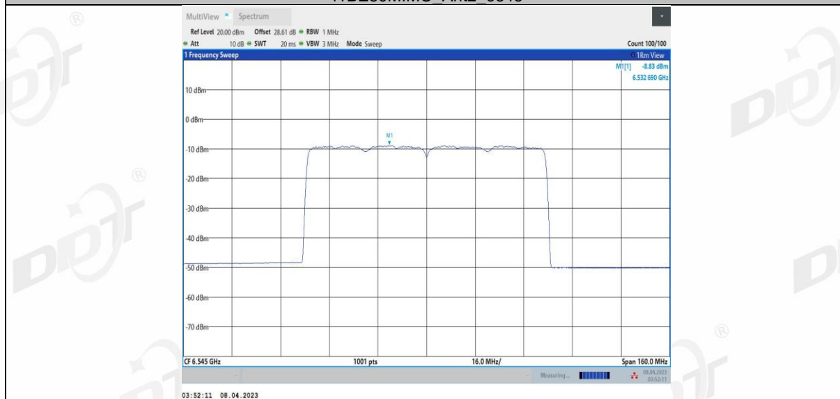
11BE80MIMO_Ant3_6545
