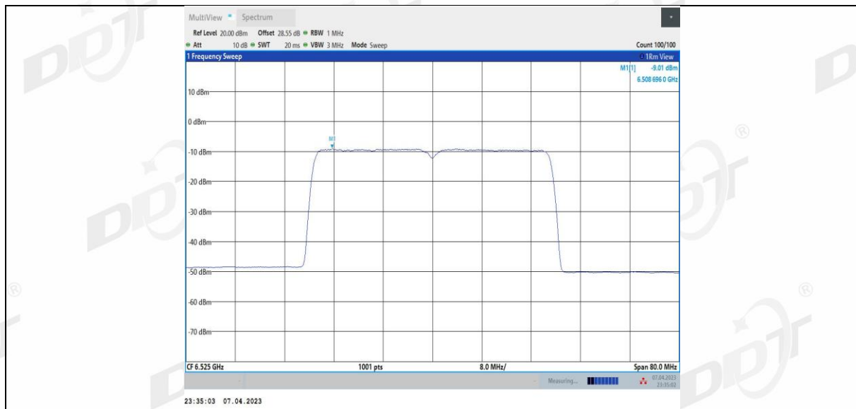
11BE40MIMO_Ant2_6525
