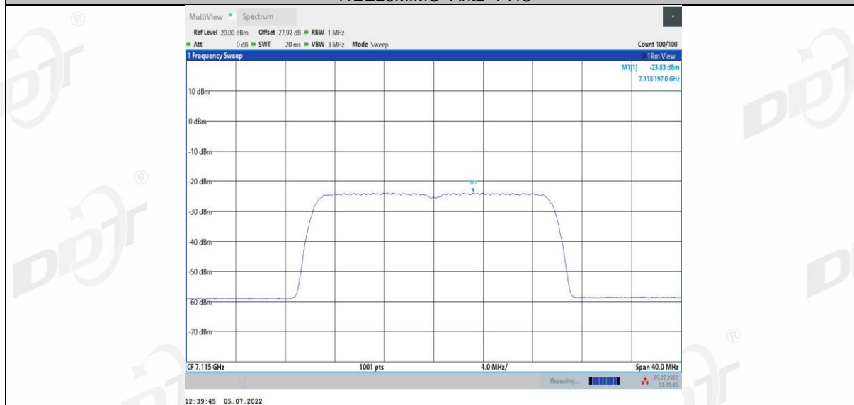
11BE20MIMO_Ant3_7115
