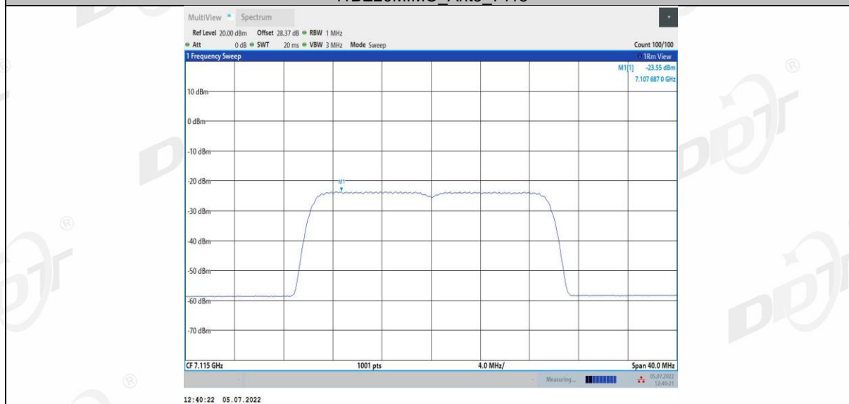
11BE20MIMO_Ant4_7115
