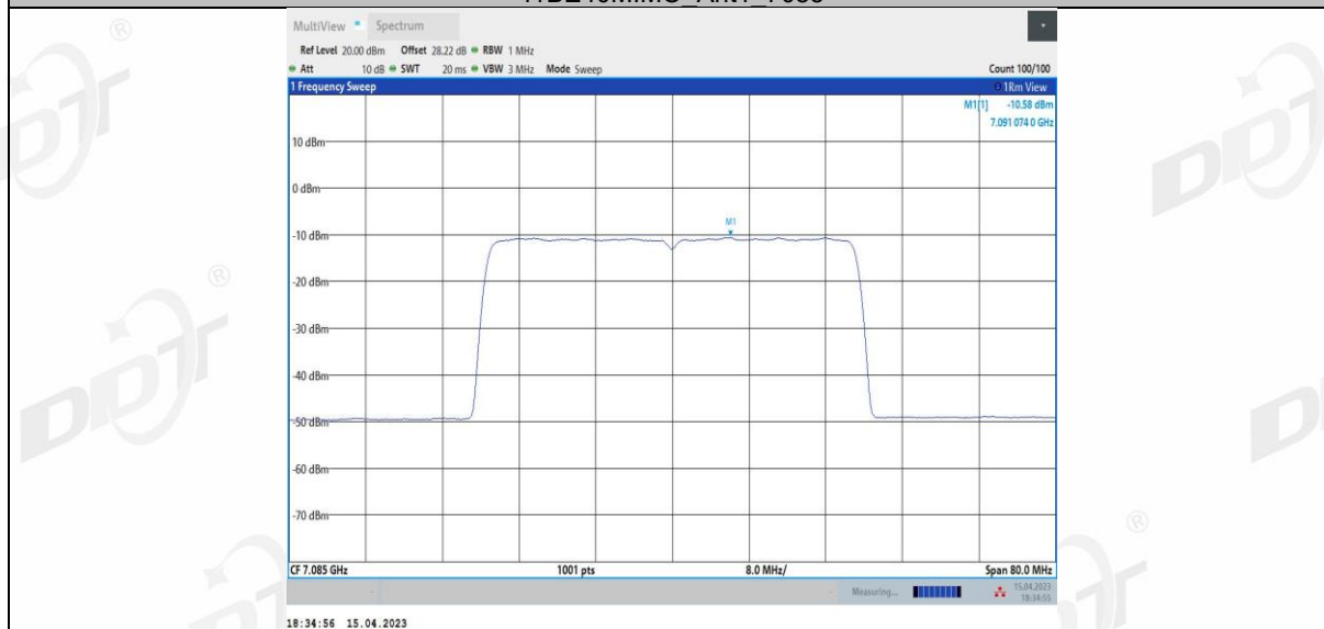
11BE40MIMO_Ant2_7085
