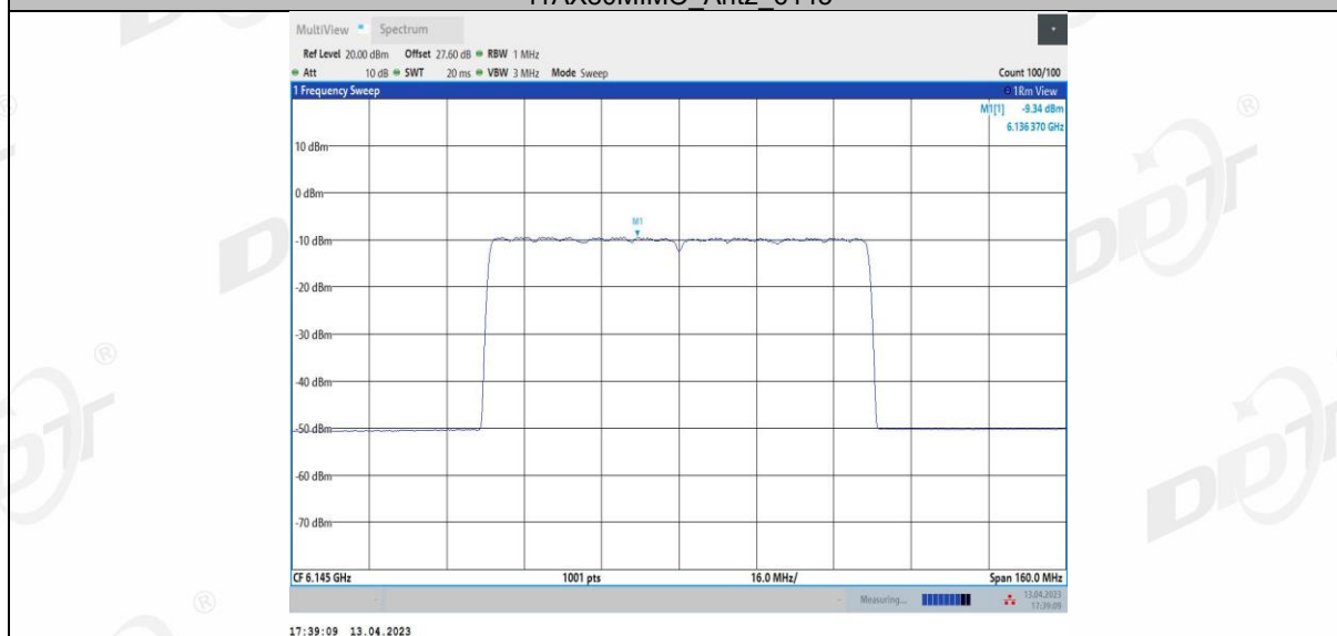
11AX80MIMO_Ant3_6145
