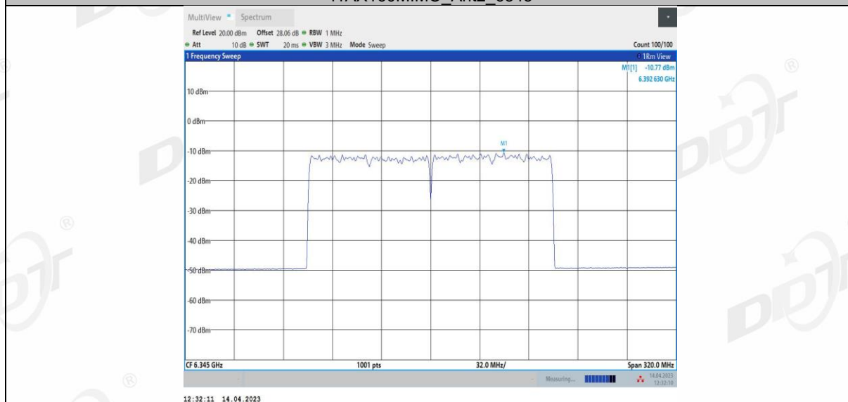
11AX160MIMO Ant3 6345
