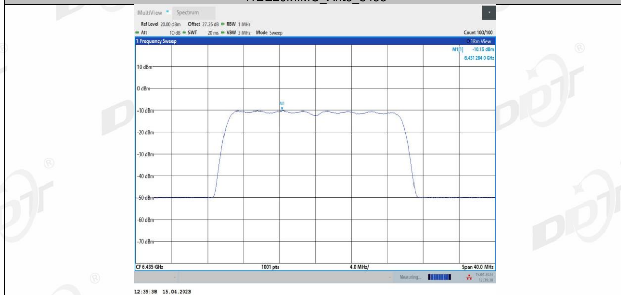
11BE20MIMO_Ant4_6435
