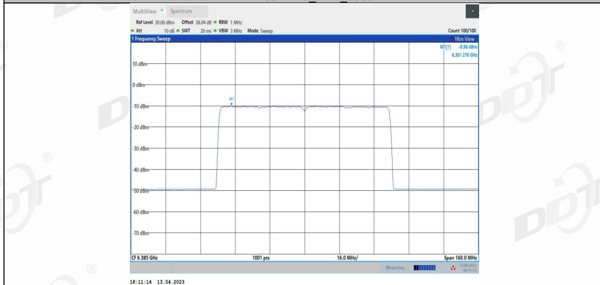
11AX80MIMO_Ant2_6385
