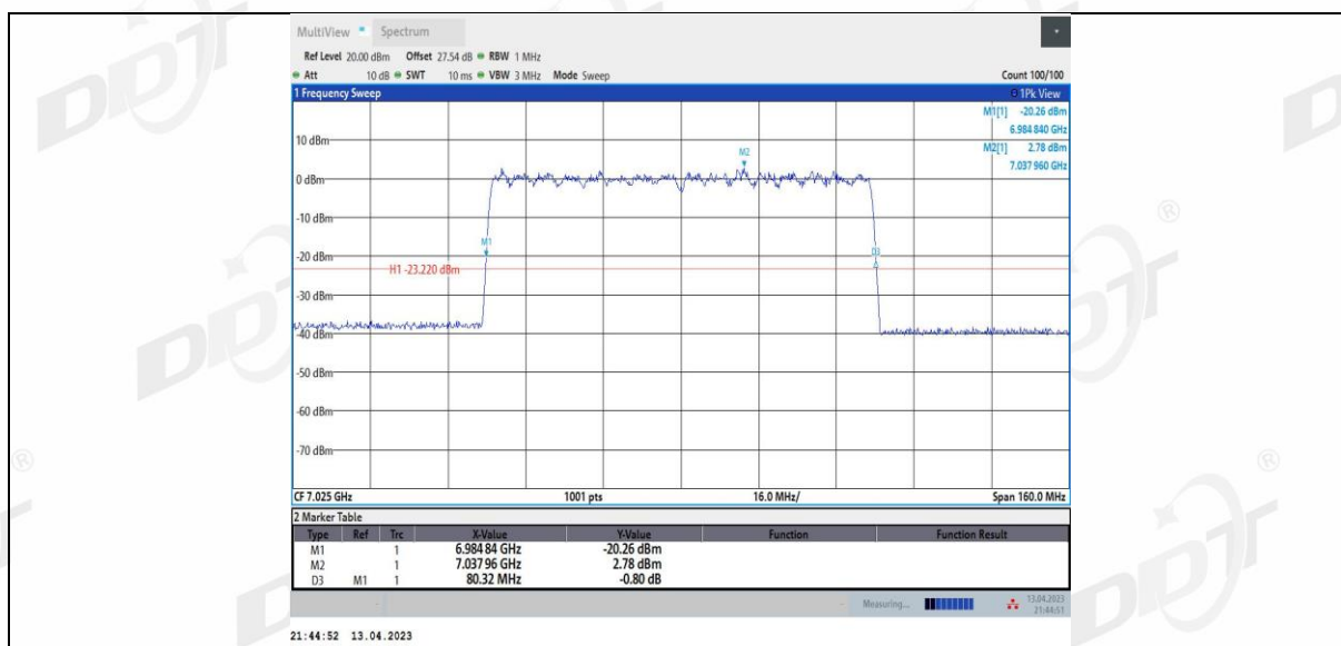
11AX80MIMO Ant4 7025
