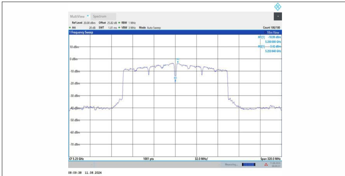
11AC160MIMO_Ant2_5250_UNII-2A
