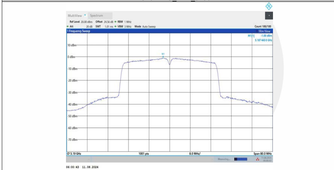
11AC40MIMO_Ant2_5190
