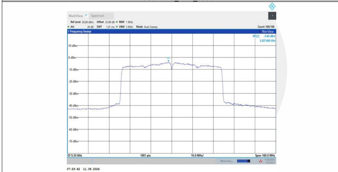
11AC80MIMO_Ant3_5530
