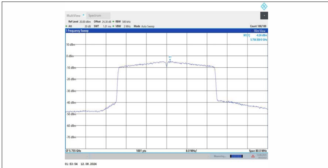
11AX40MIMO_Ant3_5755
