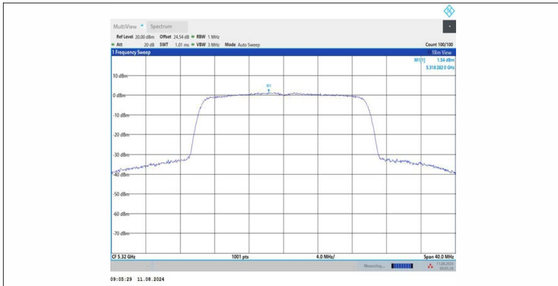
11AX20MIMO_Ant3_5320
