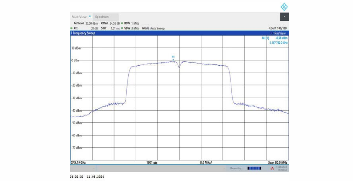
11AC40MIMO_Ant3_5190
