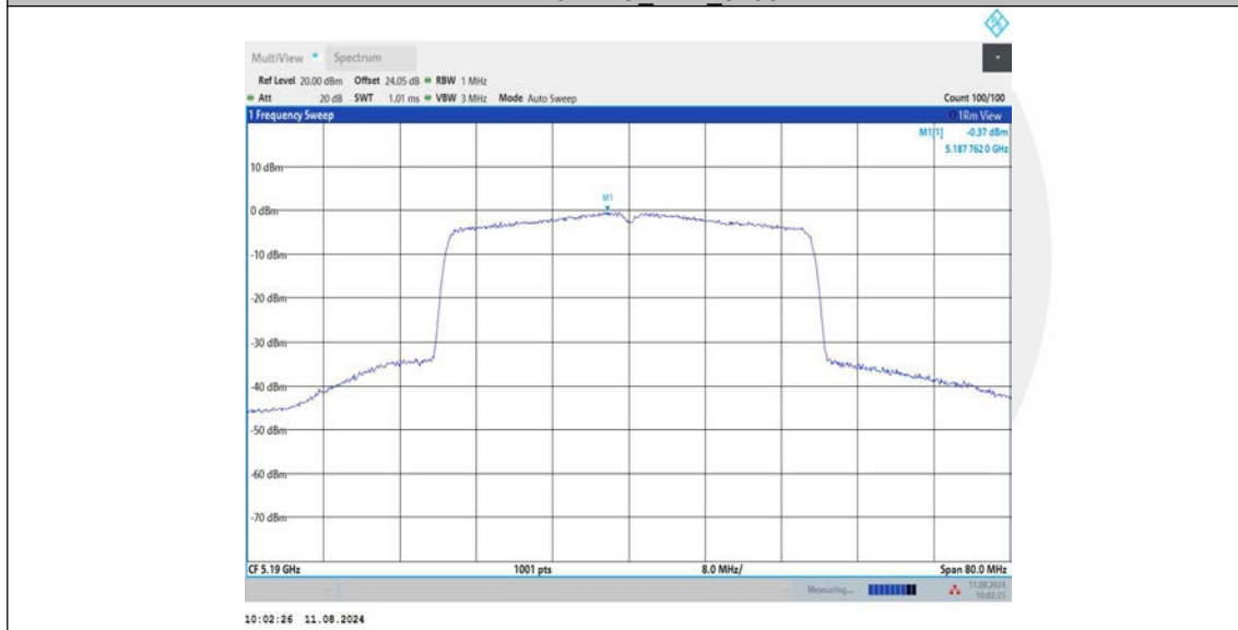
11AX40MIMO_Ant3_5190
