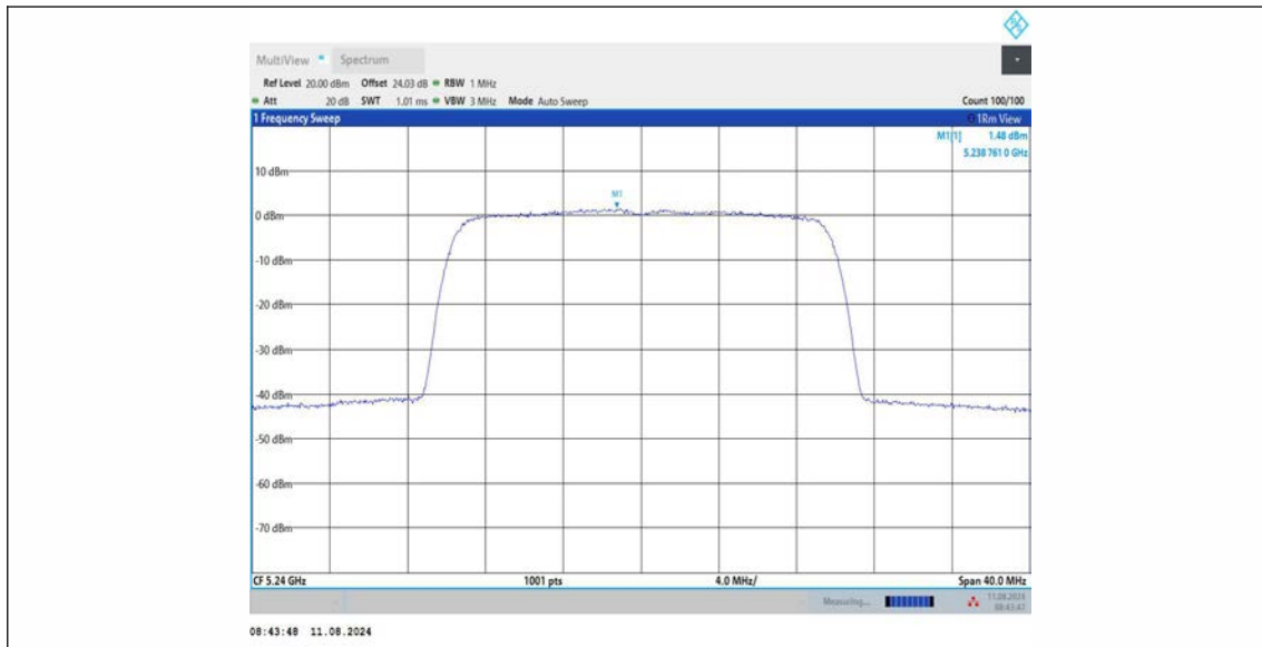
11AX20MIMO_Ant2_5240
