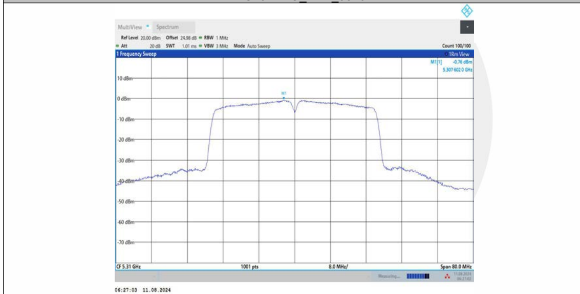
11AC40MIMO_Ant3_5310
