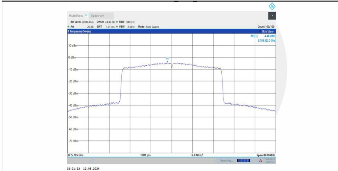
11AX40MIMO_Ant3_5795
