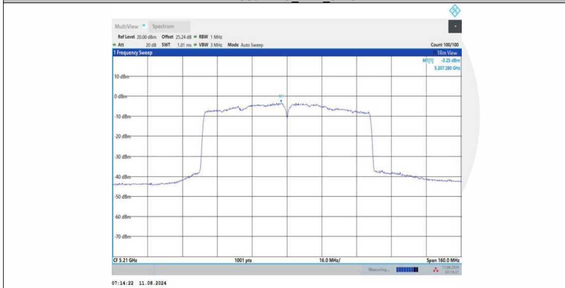
11AC80MIMO_Ant3_5210
