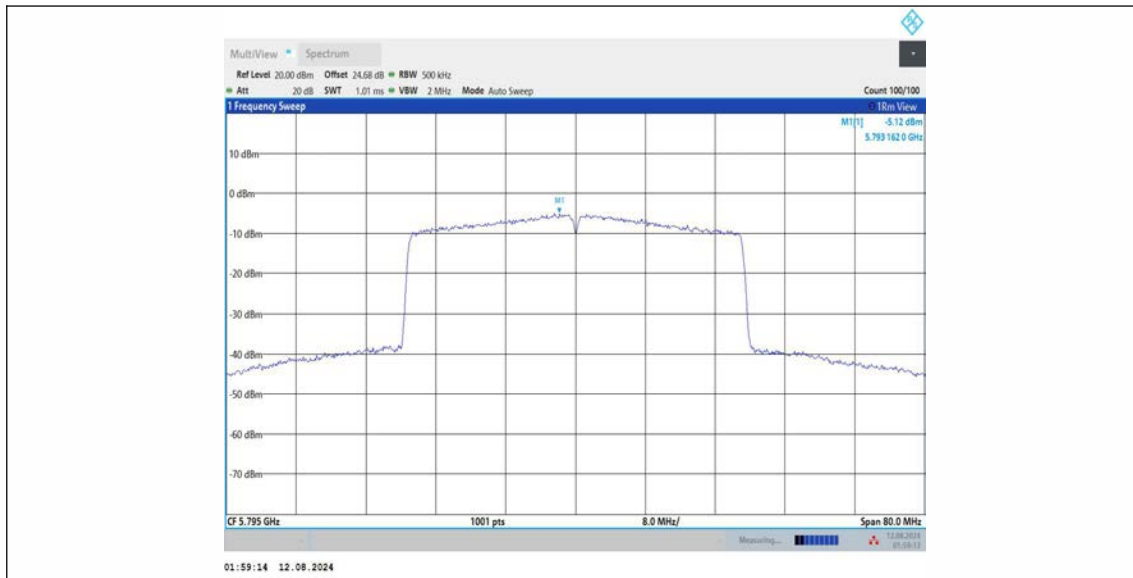
11AX40MIMO_Ant2_5795
