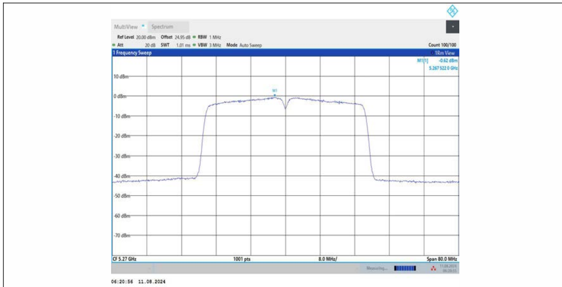
11AC40MIMO_Ant3_5270
