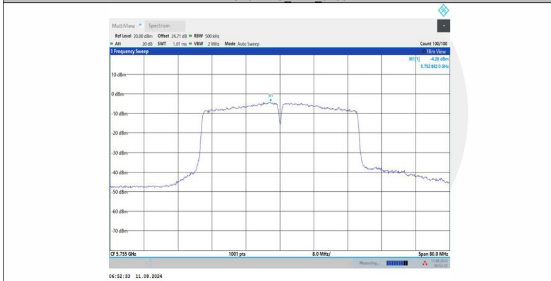
11AC40MIMO_Ant3_5755
