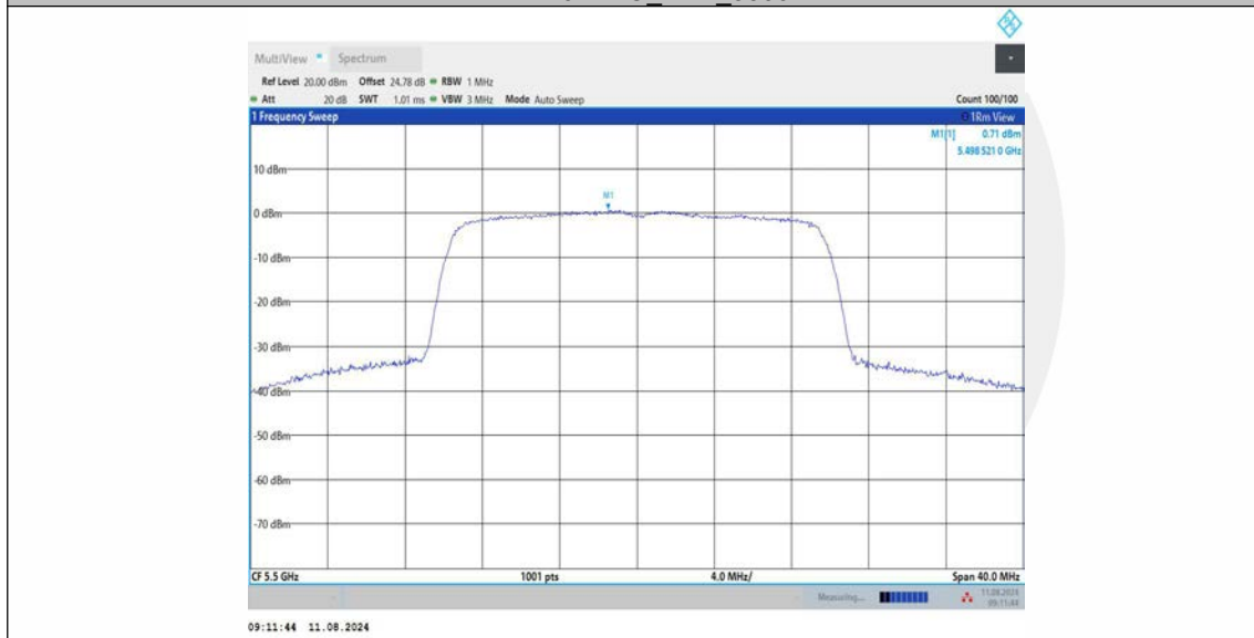
11AX20MIMO_Ant3_5500
