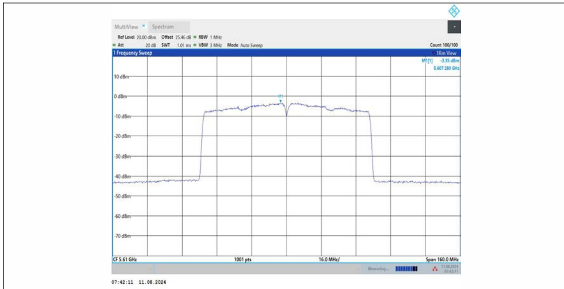
11AC80MIMO_Ant3_5610
