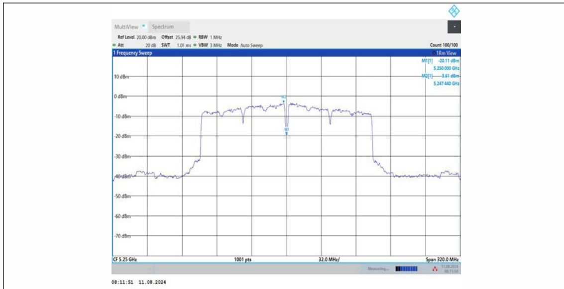
11AC160MIMO_Ant3_5250_UNII-1
