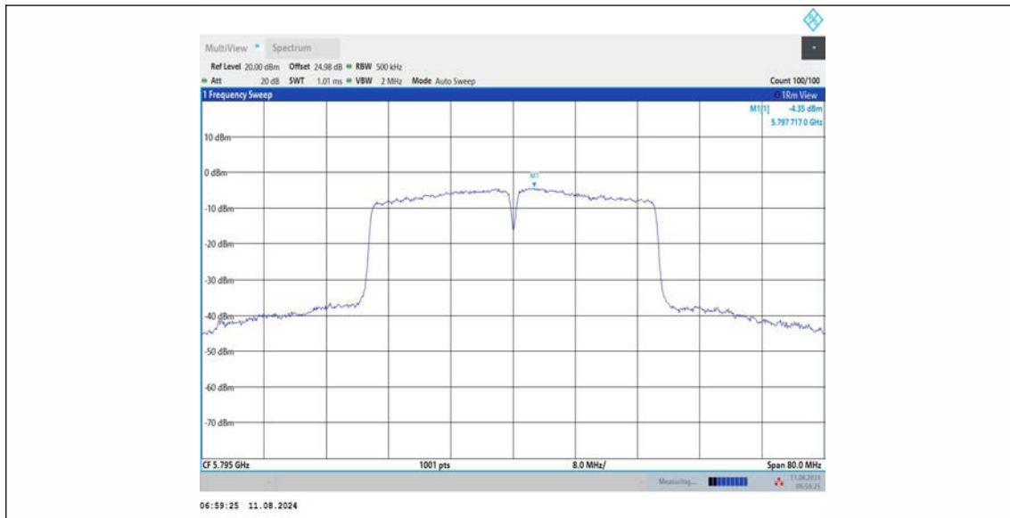
11AC40MIMO_Ant3_5795
