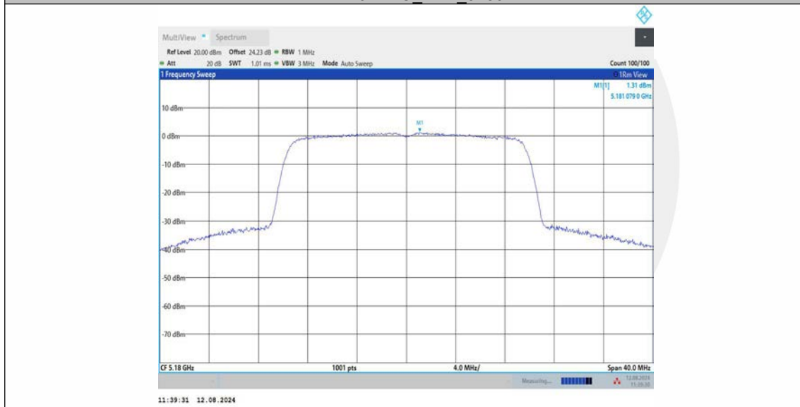
11BE20MIMO_Ant2_5180
