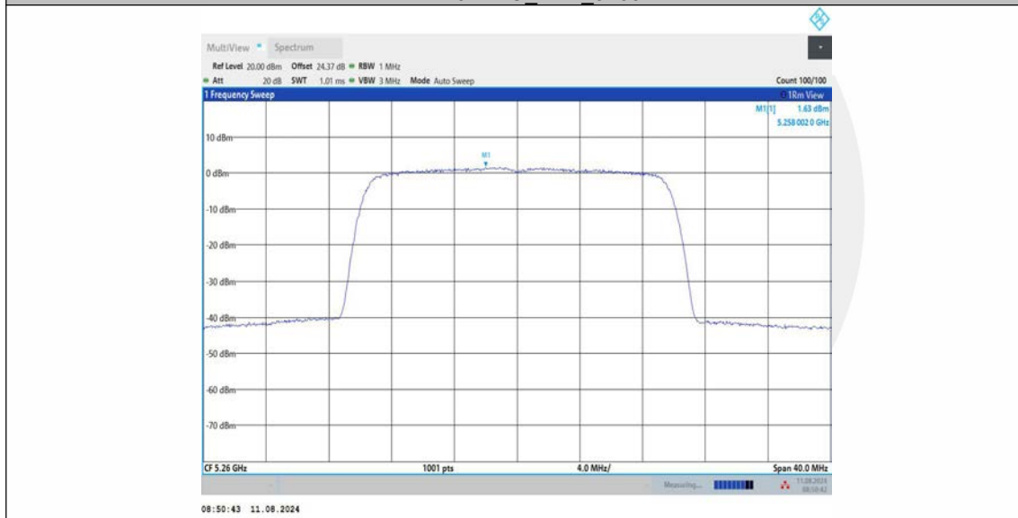
11AX20MIMO Ant2_5260
