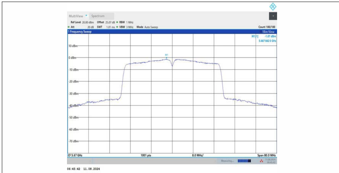
11AC40MIMO_Ant3_5670
