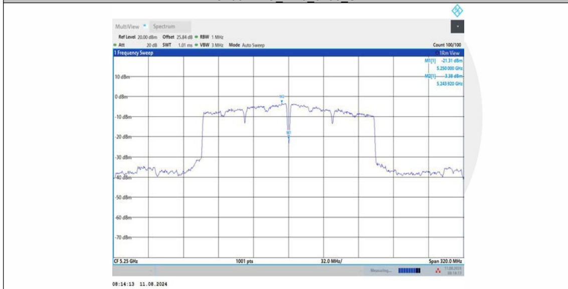
11AC160MIMO_Ant1_5250_UNII-2A
