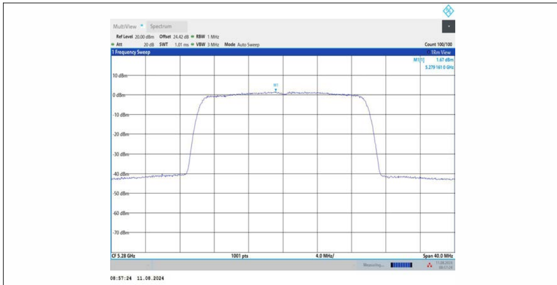
11AX20MIMO_Ant2_5280
