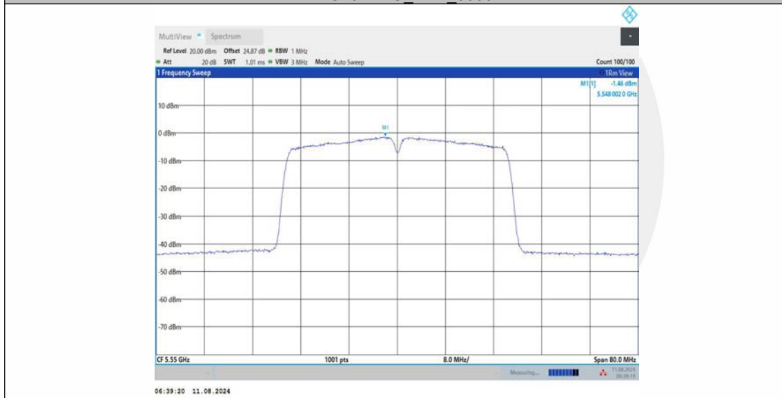
11AC40MIMO_Ant3_5550
