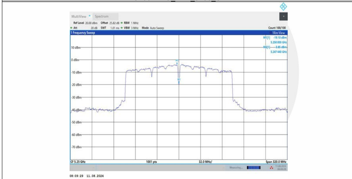
11AC160MIMO_Ant2_5250_UNII-1
