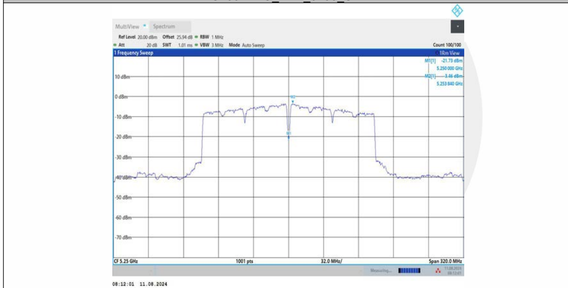
11AC160MIMO_Ant3_5250_UNII-2A
