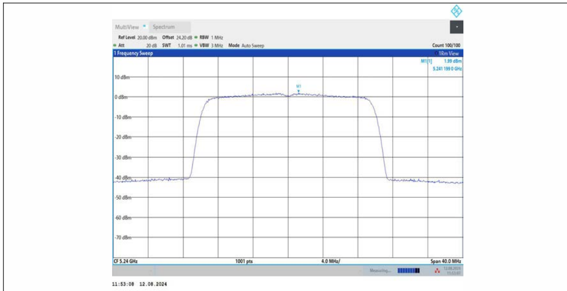
11BE20MIMO_Ant3_5240
