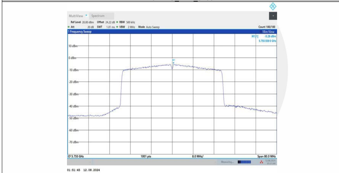
11AX40MIMO_Ant2_5755
