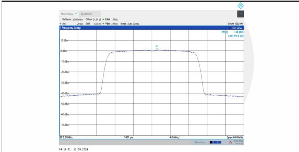
11AX20MIMO_Ant2_5580
