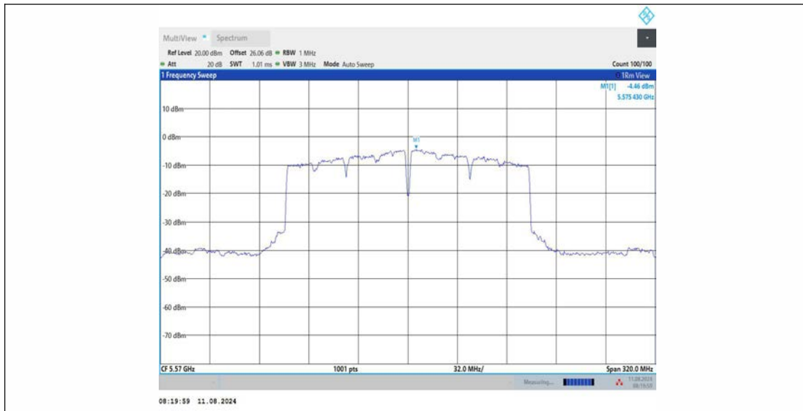
11AC160MIMO_Ant3_5570
