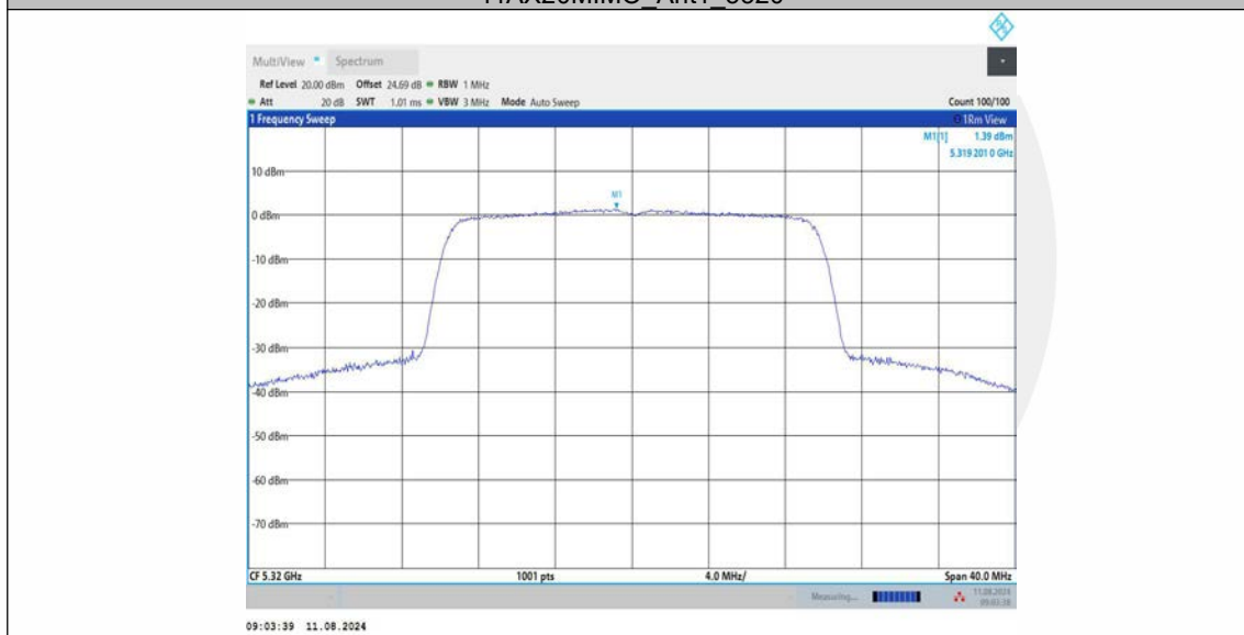
11AX20MIMO_Ant2_5320
