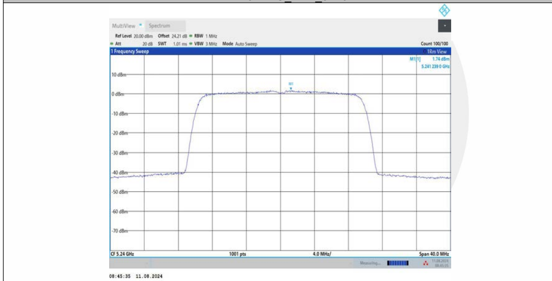
11AX20MIMO_Ant3_5240
