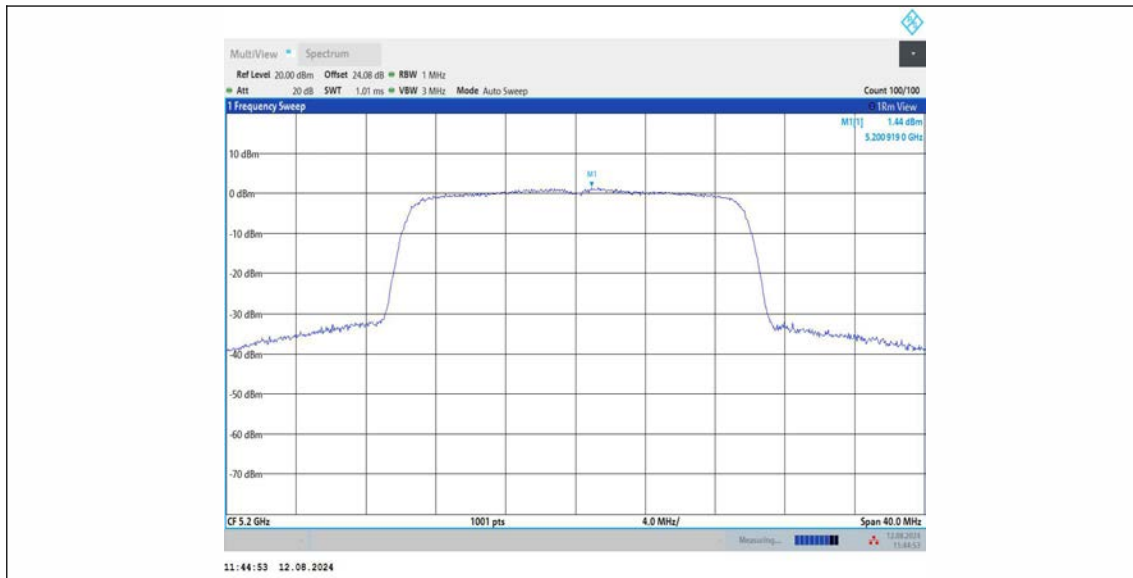
11BE20MIMO_Ant2_5200
