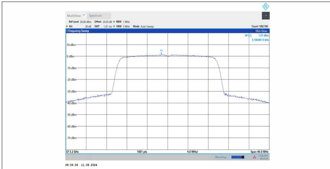
11AX20MIMO_Ant3_5200
