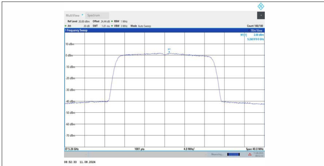
11AX20MIMO_Ant3_5260
