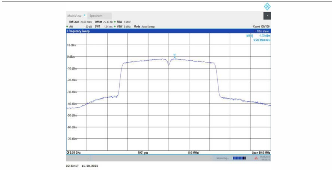
11AC40MIMO_Ant3_5510
