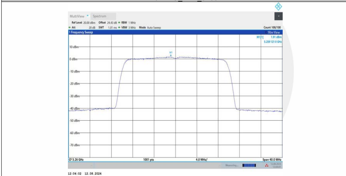
11BE20MIMO_Ant3_5260
