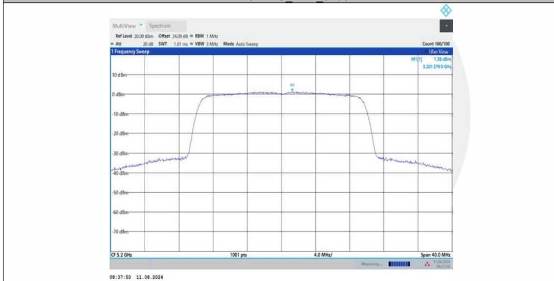
11AX20MIMO Ant2_5200
