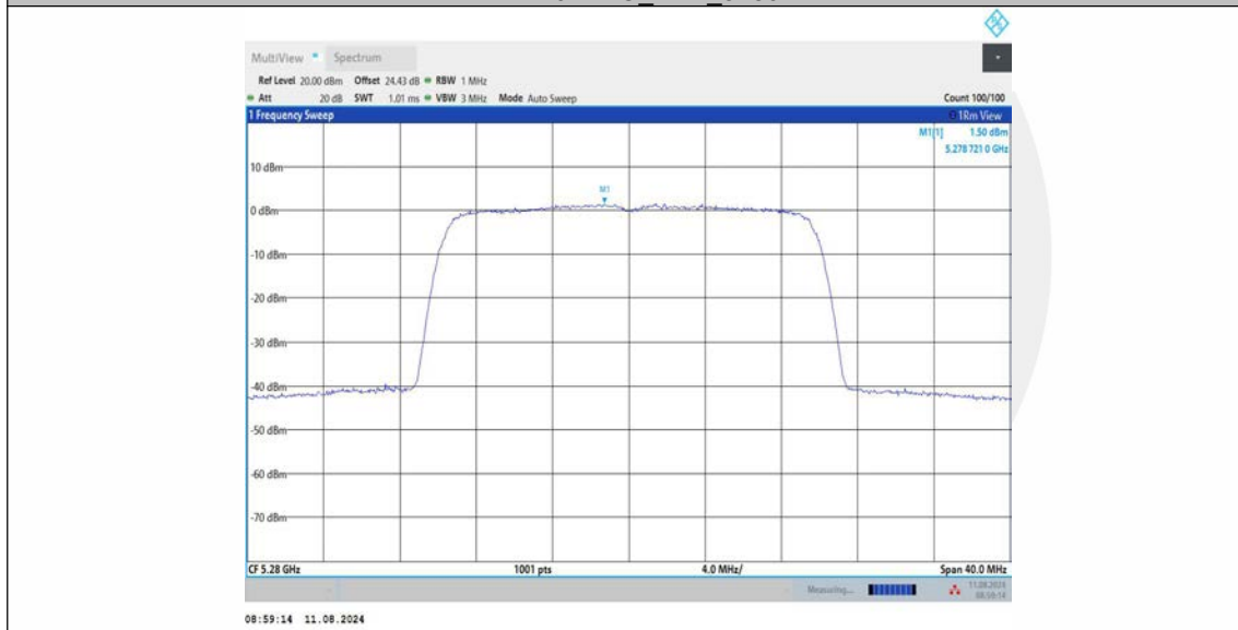
11AX20MIMO_Ant3_5280
