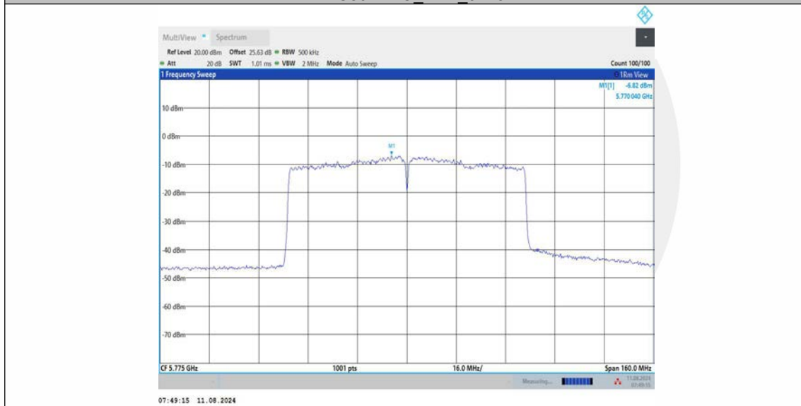
11AC80MIMO_Ant3_5775
