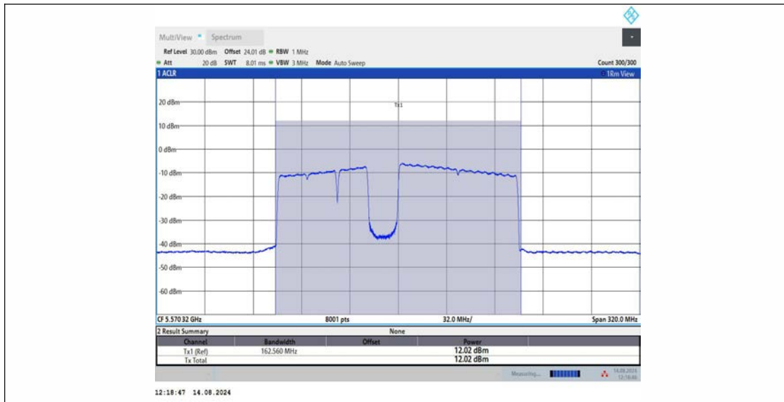
11BE160MIMO_Ant2_5570_996+484+242_OFDMA_4
