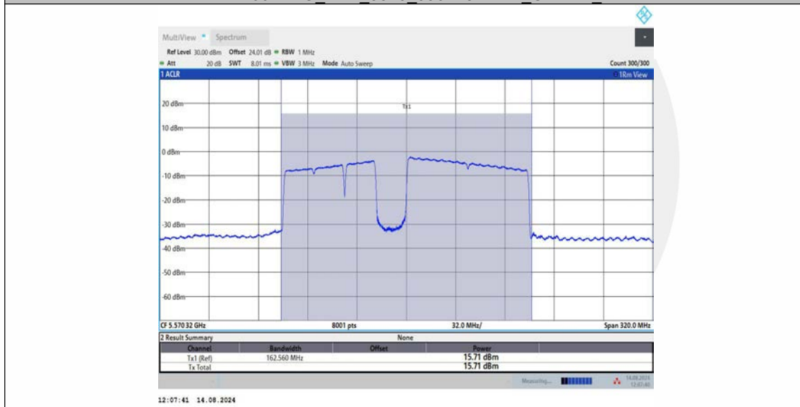
11BE160MIMO_Ant2_5570_996+484+242_OFDMA_5
