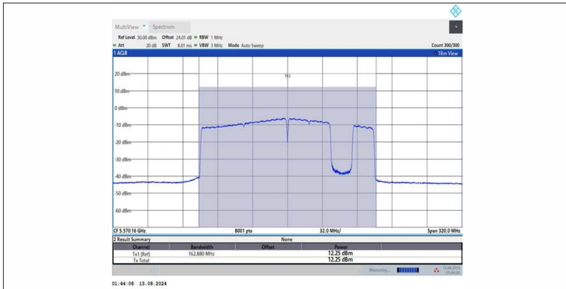
11BE160MIMO_Ant2_5570_996+484+242_OFDMA_7
