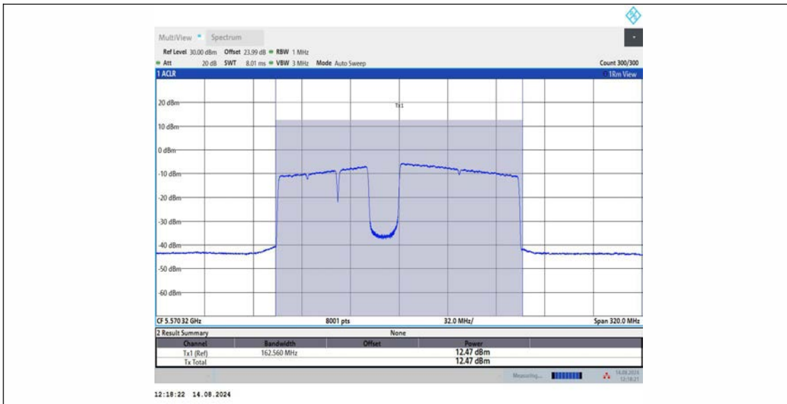
11BE160MIMO_Ant1_5570_996+484+242_OFDMA_4
