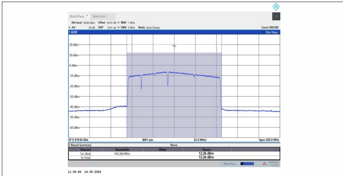
11BE160MIMO_Ant2_5570_996+484+242_OFDMA_1
