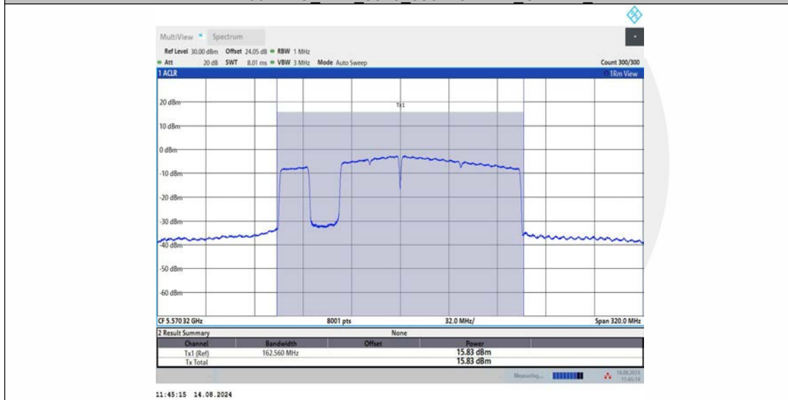
11BE160MIMO_Ant2_5570_996+484+242_OFDMA_3
