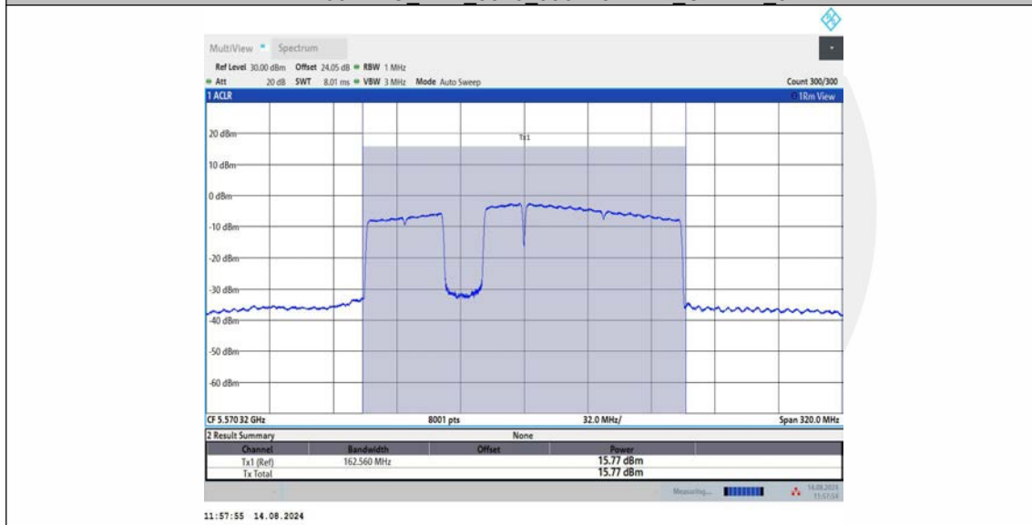
11BE160MIMO_Ant2_5570_996+484+242_OFDMA_4
