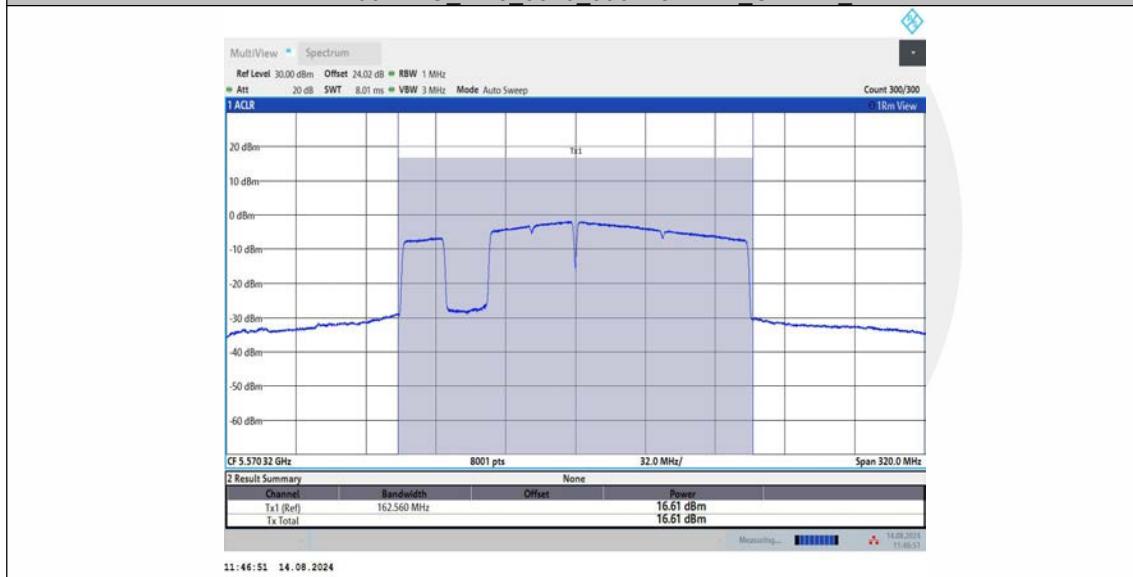
11BE160MIMO_Ant3_5570_996+484+242_OFDMA_3
