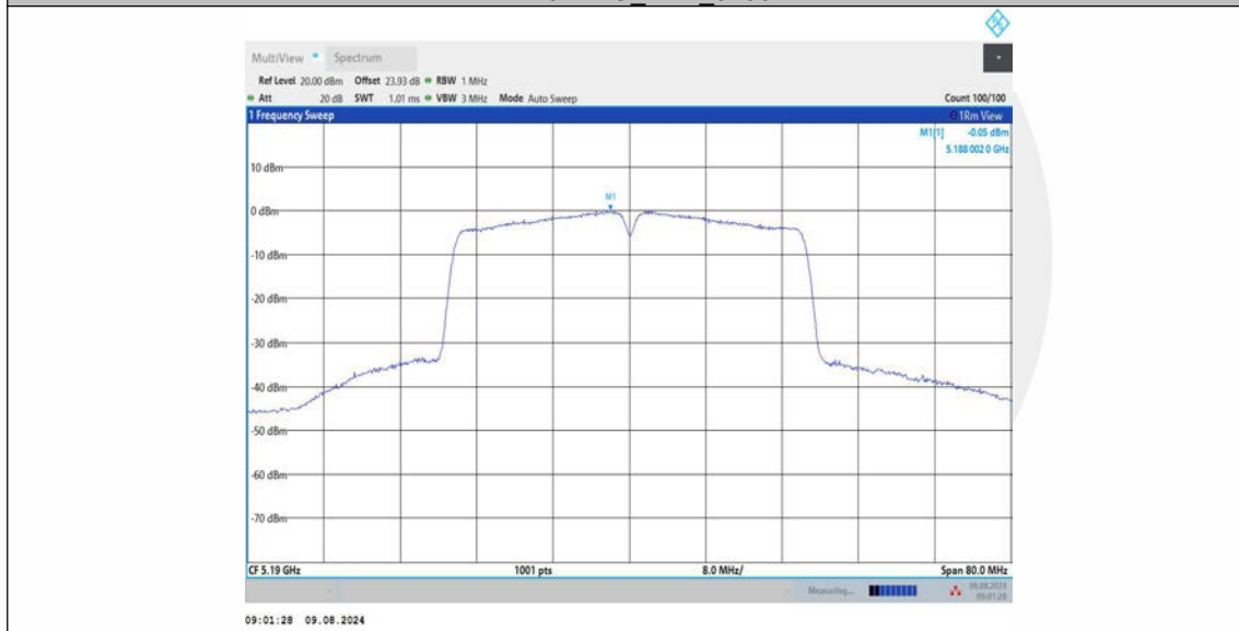
11N40MIMO_Ant3_5190
