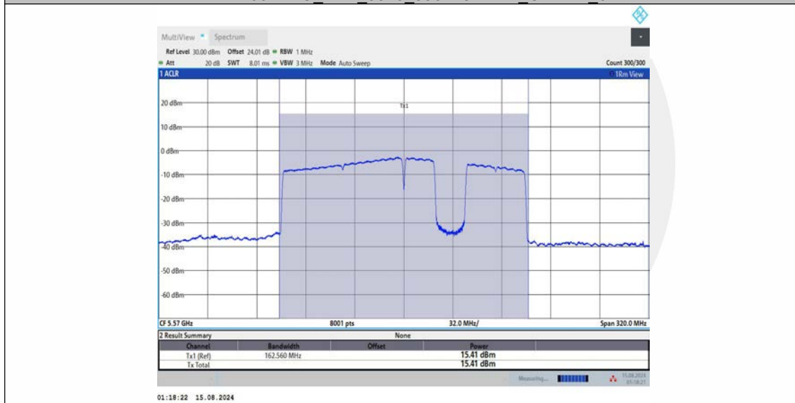
11BE160MIMO_Ant2_5570_996+484+242_OFDMA_7
