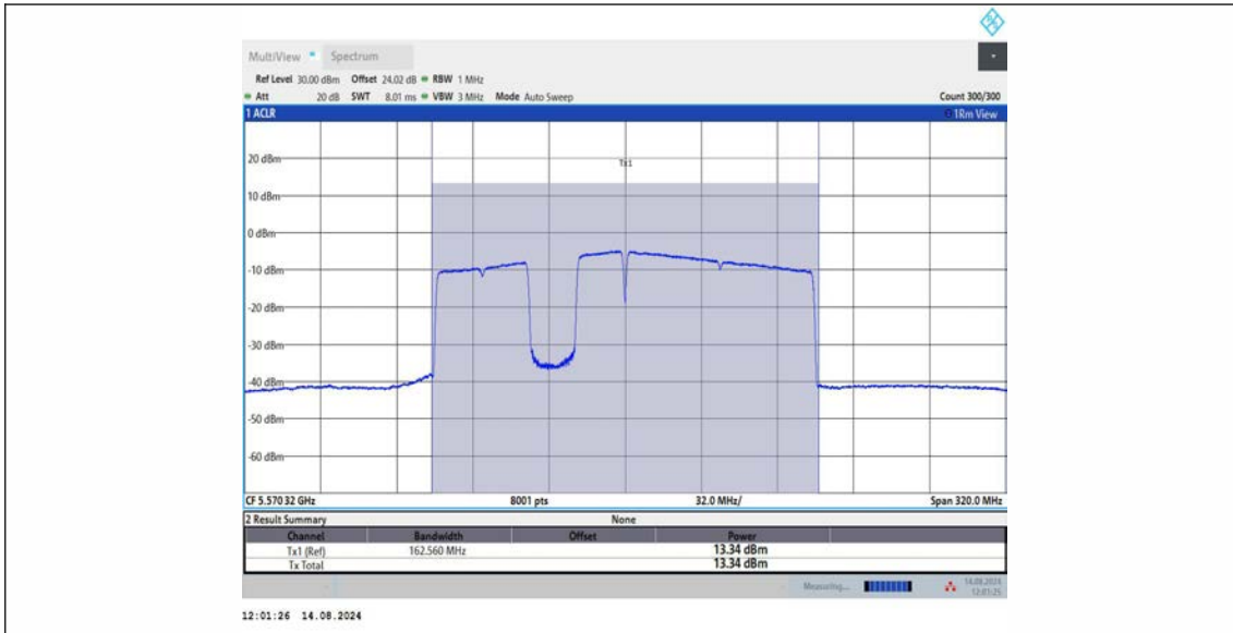
11BE160MIMO_Ant3_5570_996+484+242_OFDMA_3
