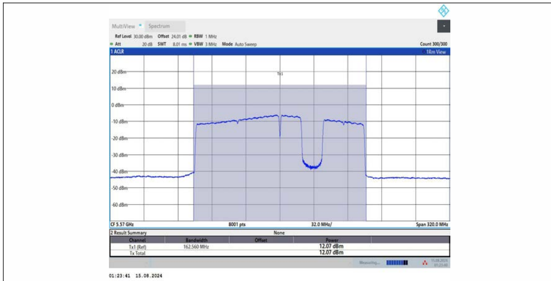
11BE160MIMO_Ant2_5570_996+484+242_OFDMA_6
