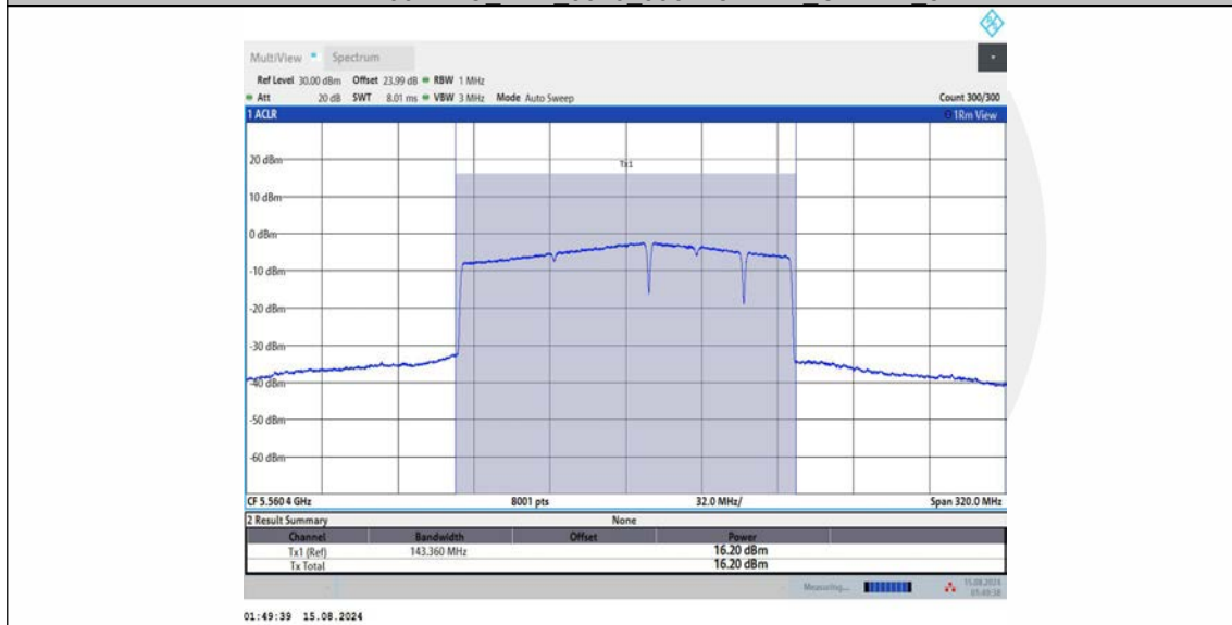
11BE160MIMO_Ant2_5570_996+484_OFDMA_1
