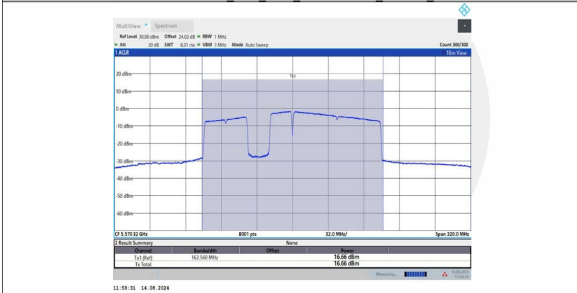
11BE160MIMO_Ant3_5570_996+484+242_OFDMA_4
