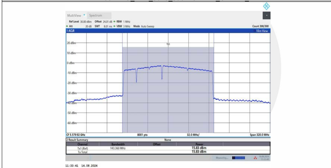
11BE160MIMO_Ant2_5570_996+484+242_OFDMA_2
