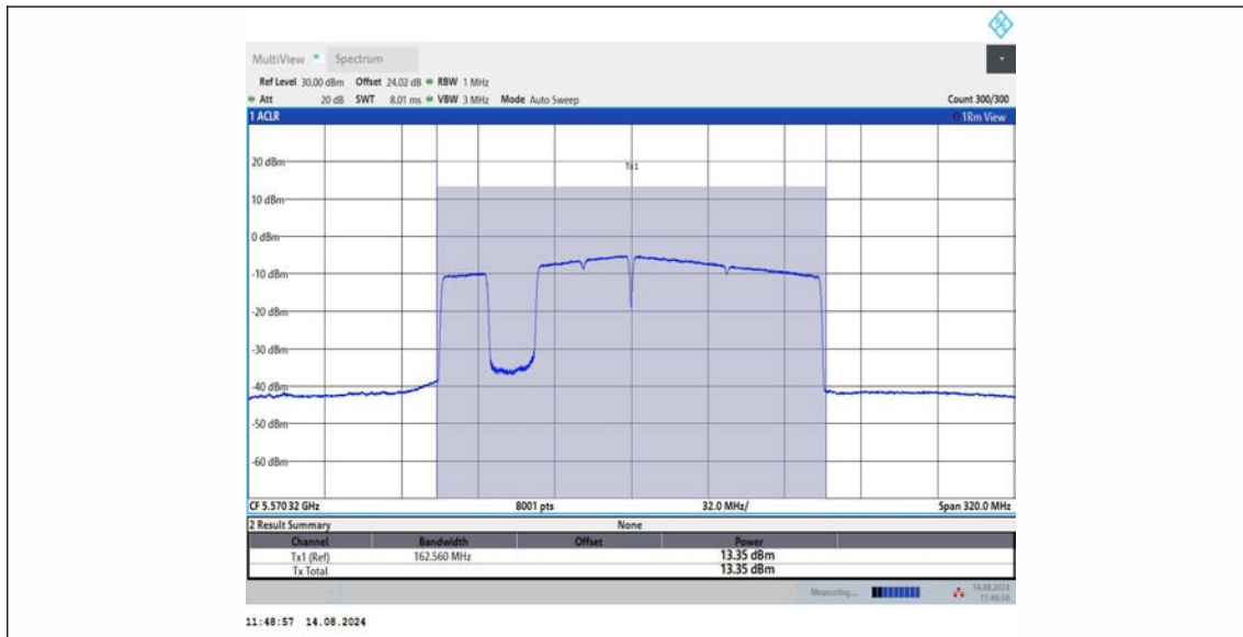
11BE160MIMO_Ant3_5570_996+484+242_OFDMA_2
