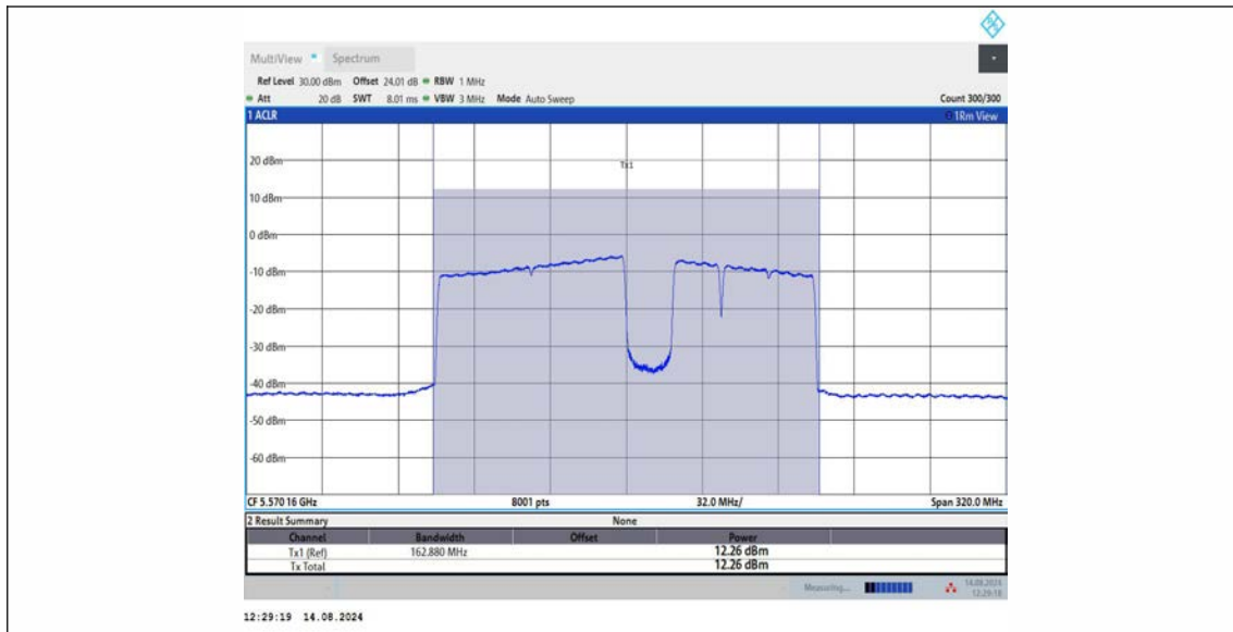
11BE160MIMO_Ant2_5570_996+484+242_OFDMA_5
