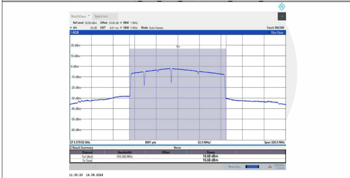
11BE160MIMO_Ant3_5570_996+484+242_OFDMA_2
