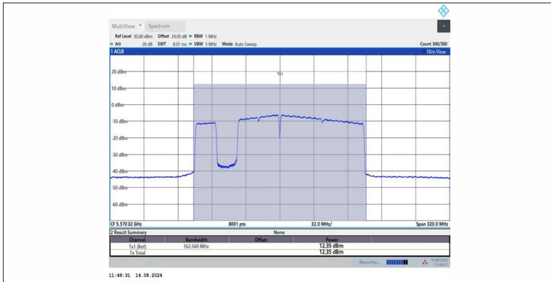
11BE160MIMO_Ant2_5570_996+484+242_OFDMA_2
