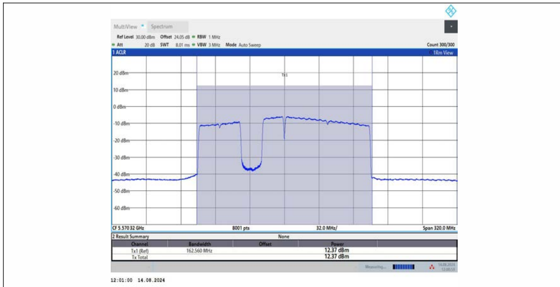
11BE160MIMO_Ant2_5570_996+484+242_OFDMA_3
