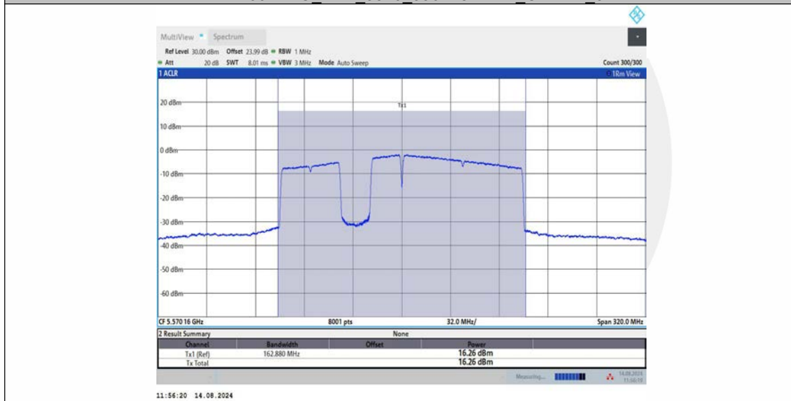
11BE160MIMO_Ant1_5570_996+484+242_OFDMA_4
