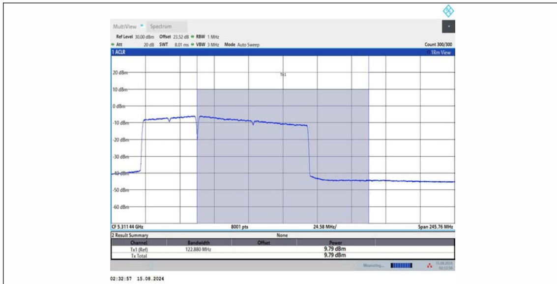
11BE160MIMO Ant1 5250 UNII-2A 996+484 OFDMA 1
