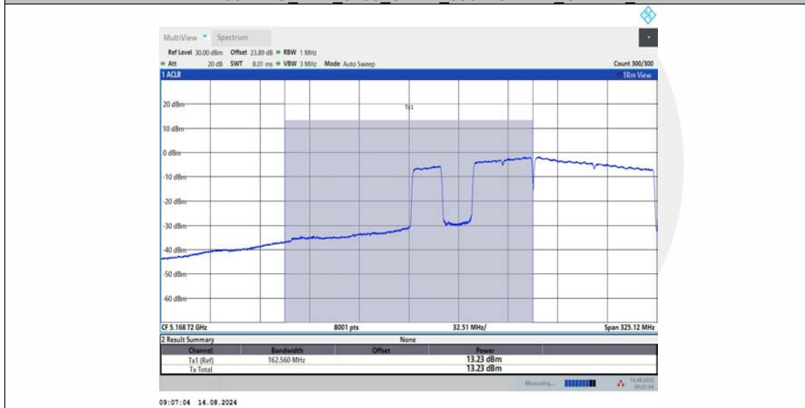
11BE160MIMO_Ant2_5250_UNII-1_996+484+242_OFDMA_3
