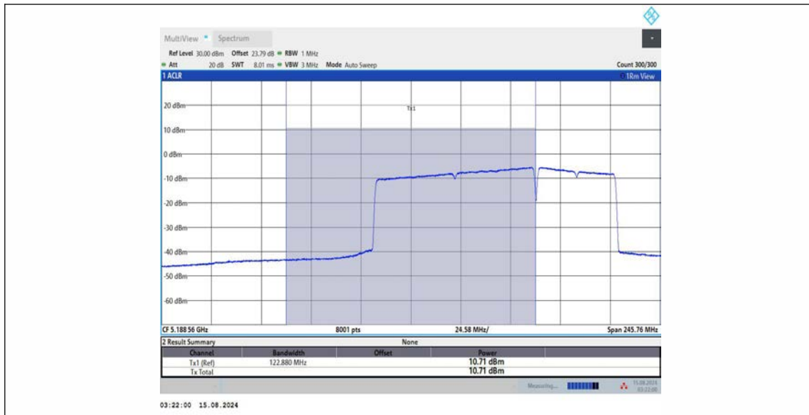
11BE160MIMO_Ant3_5250_UNII-1_996+484_OFDMA_4
