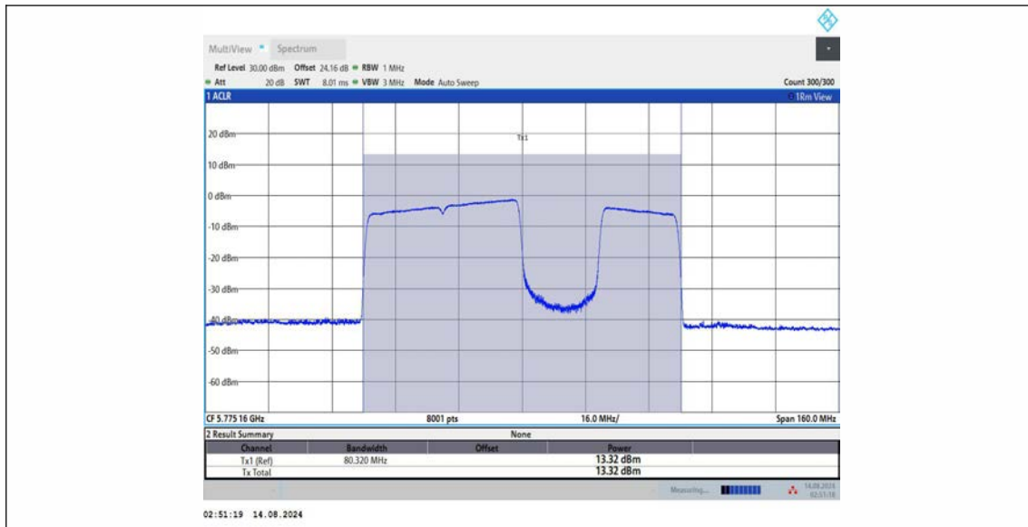
11BE80MIMO_Ant3_5775_484+242_OFDMA_4
