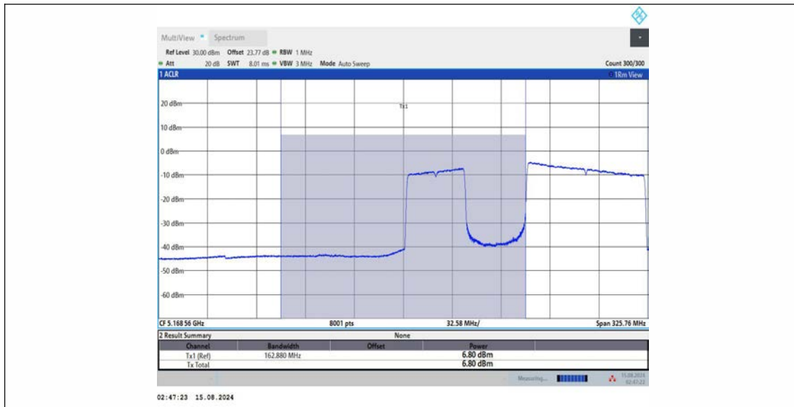
11BE160MIMO Ant1 5250 UNII-1 996+484 OFDMA 2
