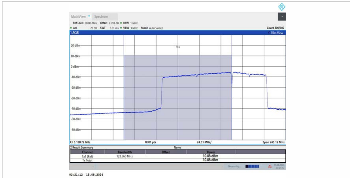
11BE160MIMO_Ant2_5250_UNII-1_996+484_OFDMA_4
