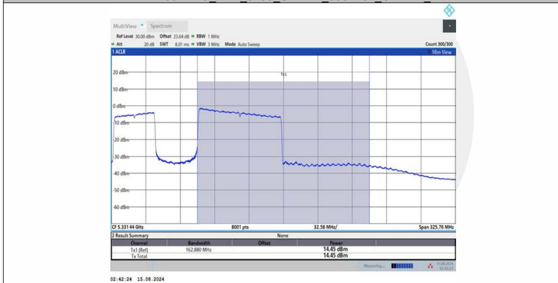
11BE160MIMO Ant2 5250 UNII-2A 996+484 OFDMA 3
