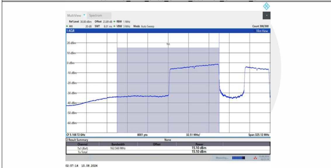
11BE160MIMO_Ant2_5250_UNII-1_996+484_OFDMA_4
