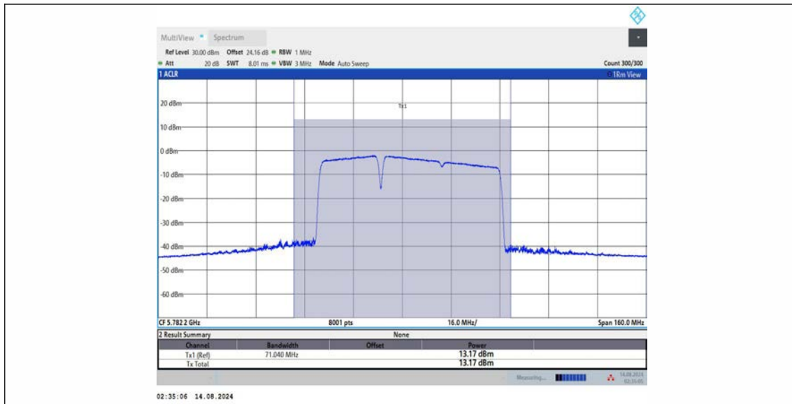
11BE80MIMO_Ant3_5775_484+242_OFDMA_2
