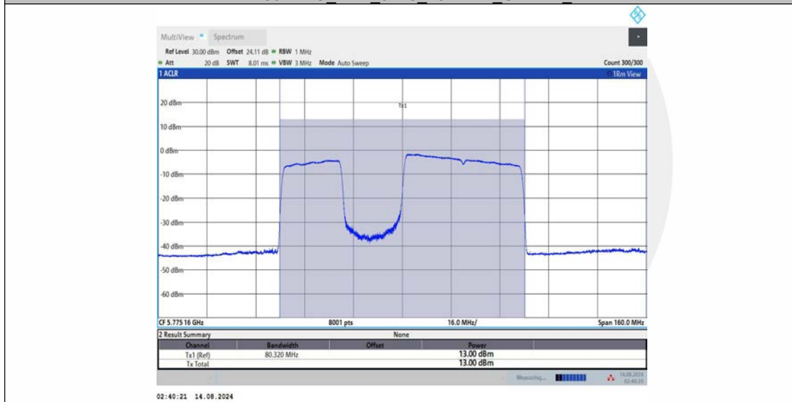
11BE80MIMO_Ant2_5775_484+242_OFDMA_3
