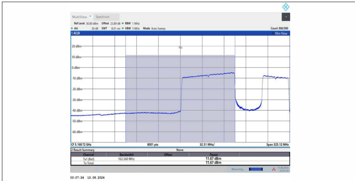
11BE160MIMO_Ant2_5250_UNII-1_996+484_OFDMA_3
