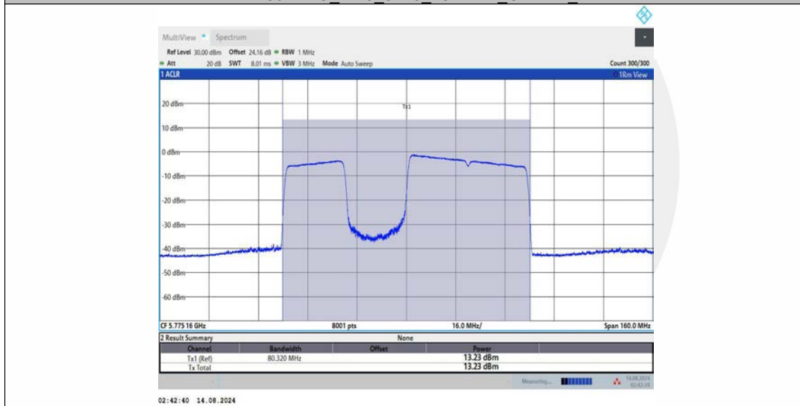
11BE80MIMO_Ant3_5775_484+242_OFDMA_3
