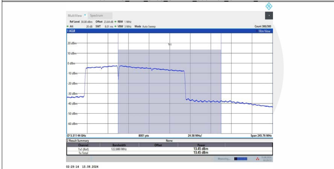
11BE160MIMO Ant2 5250 UNII-2A 996+484 OFDMA 2
