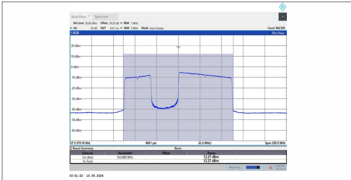
11BE160MIMO Ant1 5570 996+484 OFDMA 2
