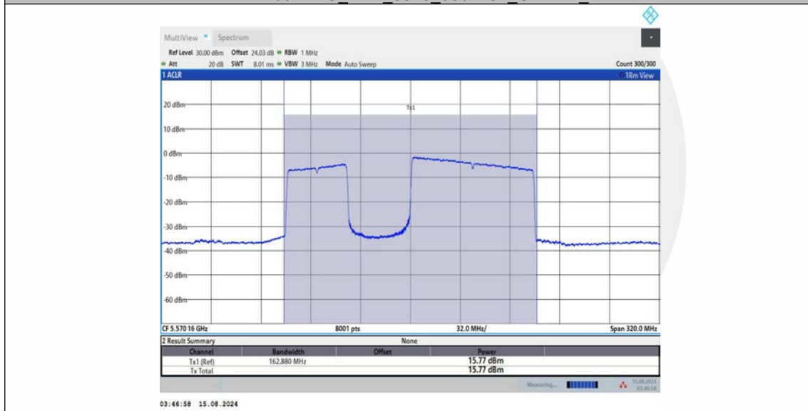
11BE160MIMO Ant1 5570 996+484 OFDMA 3
