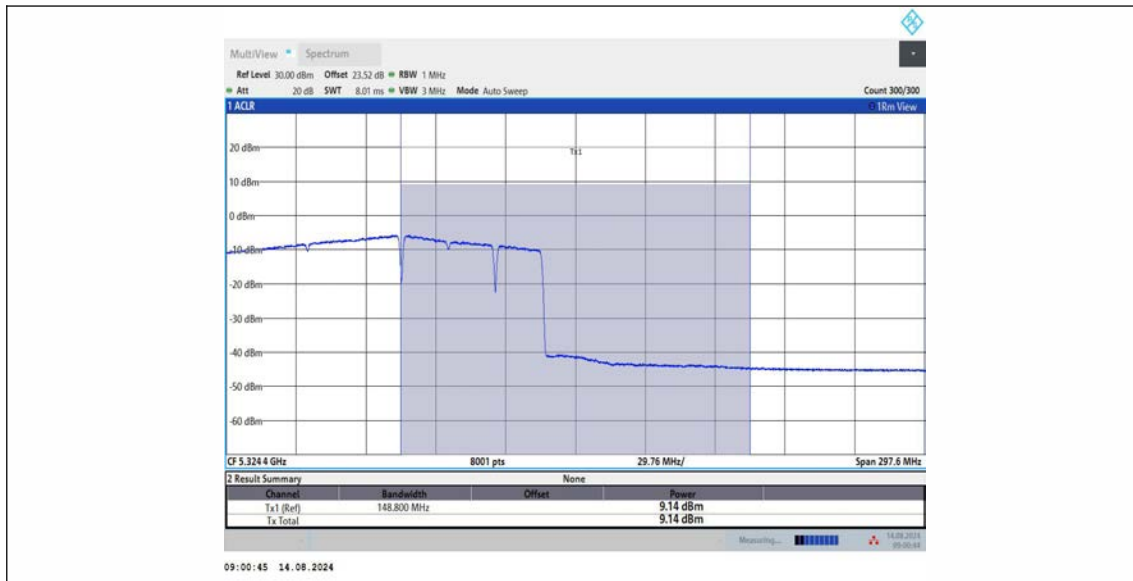
11BE160MIMO_Ant1 5250 UNII-2A 996+484+242 OFDMA 8
