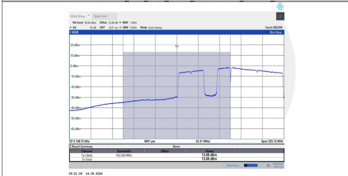
11BE160MIMO_Ant2_5250_UNII-1_996+484+242_OFDMA_4
