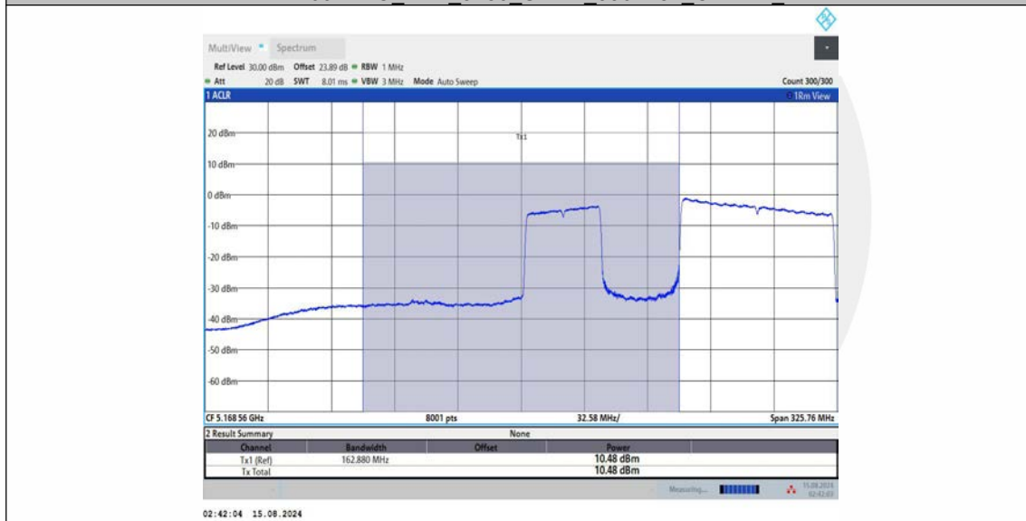
11BE160MIMO_Ant2_5250_UNII-1_996+484_OFDMA_3
