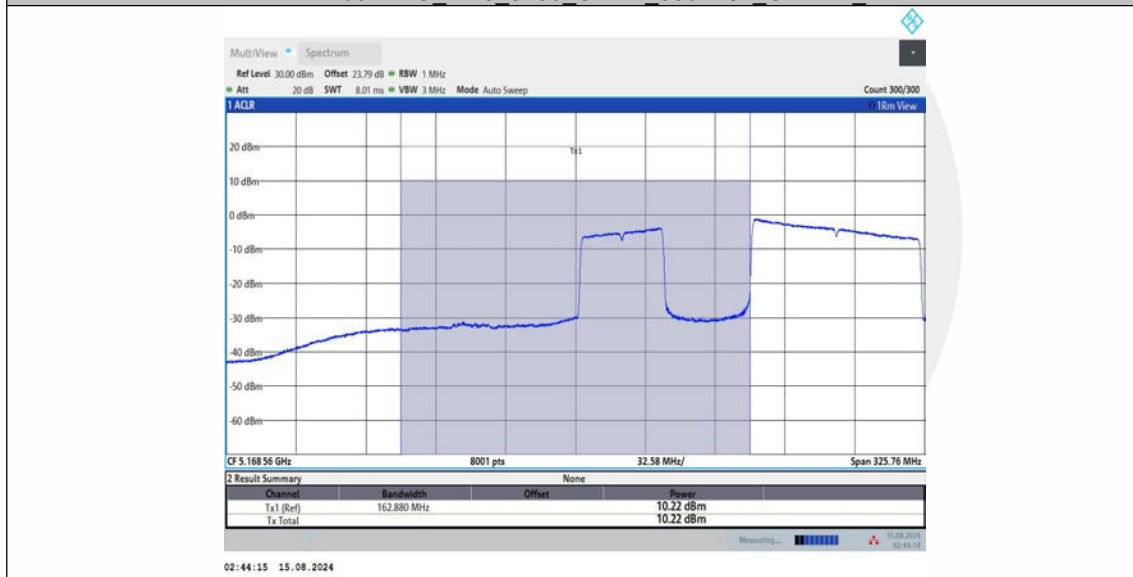
11BE160MIMO_Ant3_5250_UNII-1_996+484_OFDMA_3
