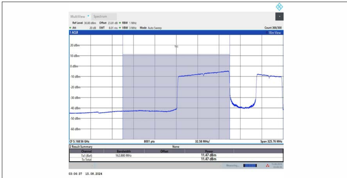
11BE160MIMO Ant1 5250 UNII-1 996+484 OFDMA 3
