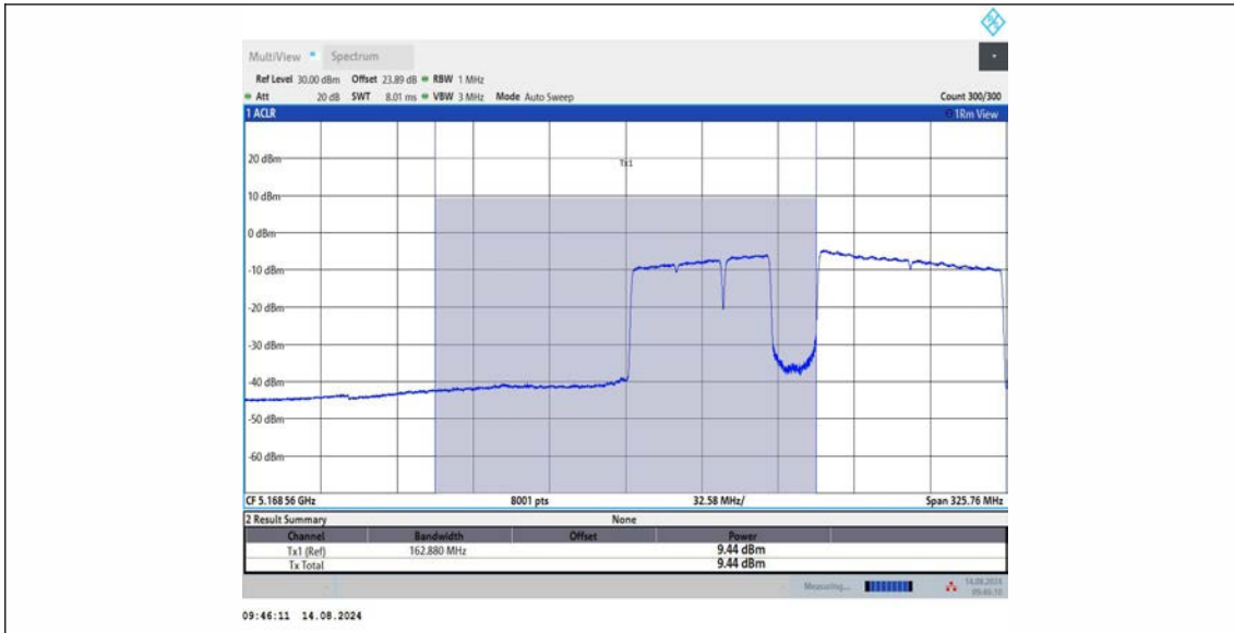
11BE160MIMO_Ant2_5250_UNII-1_996+484+242_OFDMA_4
