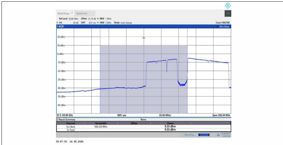
11BE160MIMO_Ant3_5250_UNII-1_996+484+242_OFDMA_4
