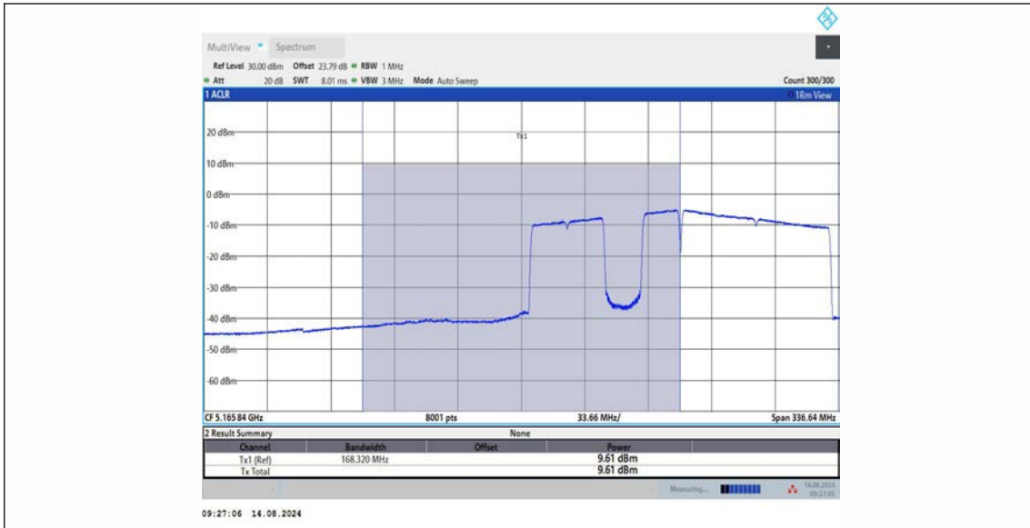
11BE160MIMO_Ant3_5250_UNII-1_996+484+242_OFDMA_3
