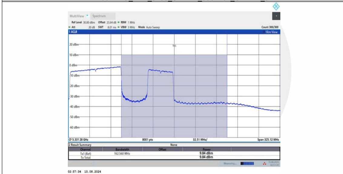
11BE160MIMO_Ant2_5250_UNII-2A_996+484_OFDMA_4
