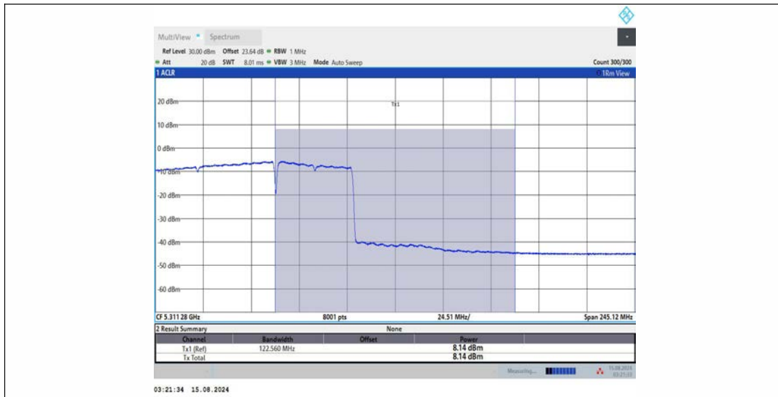
11BE160MIMO Ant2 5250 UNII-2A 996+484 OFDMA 4
