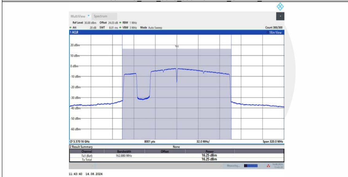
11BE160MIMO_Ant1 5570_996+484+242_OFDMA 3
