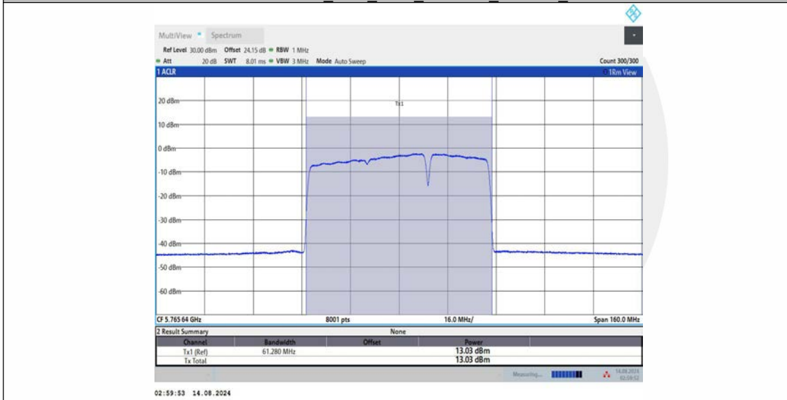
11BE80MIMO_Ant3_5775_484+242_OFDMA_1
