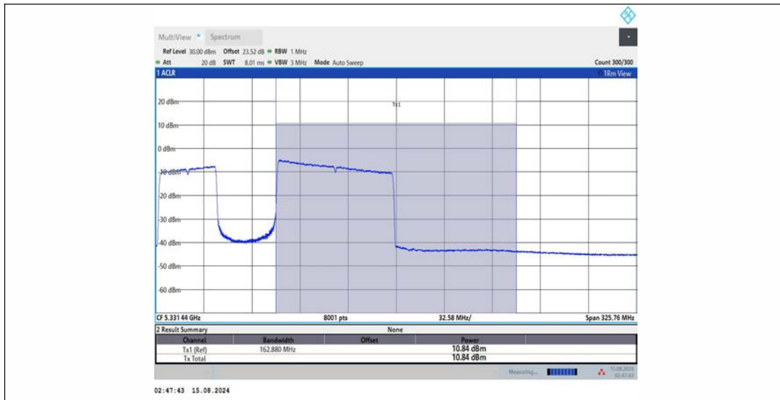
11BE160MIMO Ant1_5250_UNII-2A_996+484_OFDMA_2
