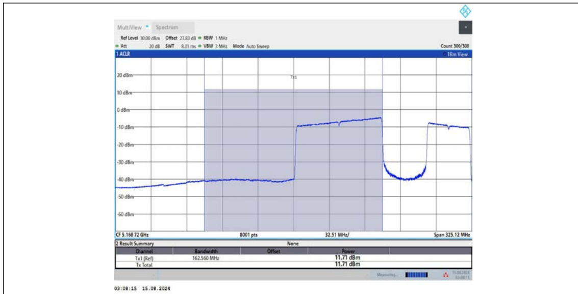
11BE160MIMO_Ant3_5250_UNII-1_996+484_OFDMA_3
