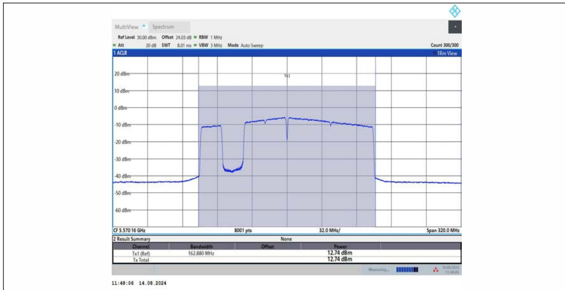
11BE160MIMO_Ant1 5570_996+484+242_OFDMA 2
