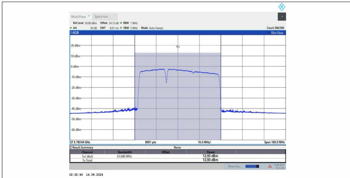
11BE80MIMO_Ant2_5775_484+242_OFDMA_2
