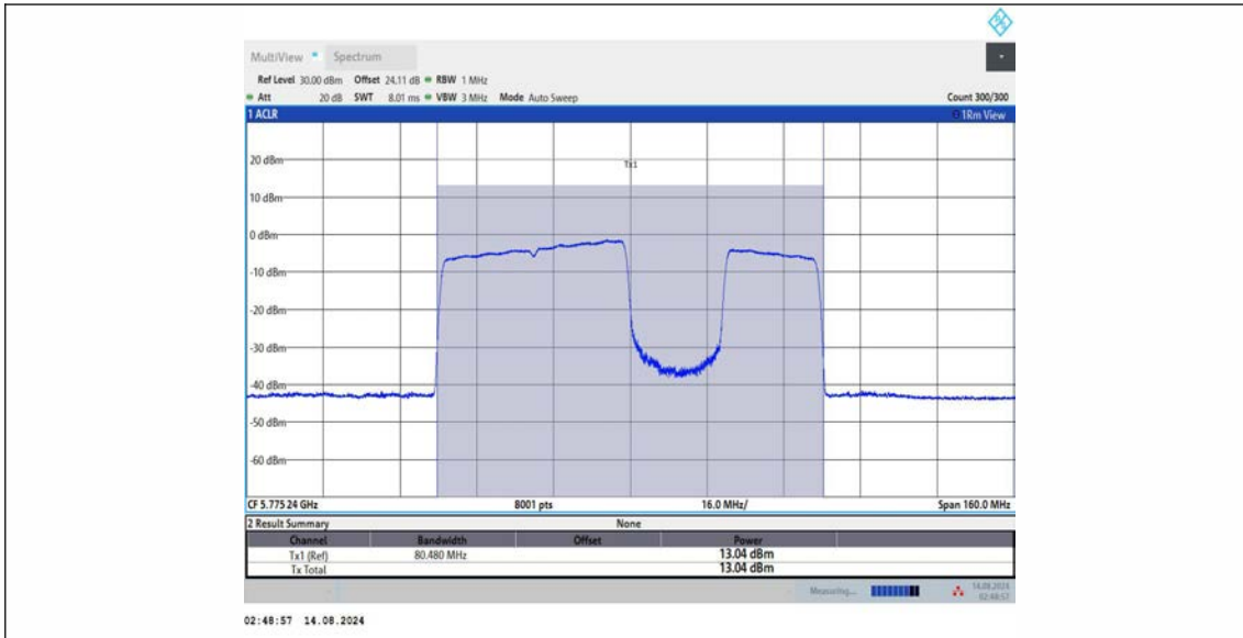
11BE80MIMO_Ant2_5775_484+242_OFDMA_4
