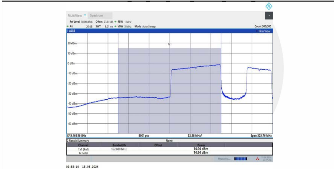
11BE160MIMO Ant1 5250 UNII-1 996+484 OFDMA 4
