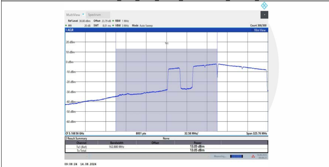
11BE160MIMO_Ant3_5250_UNII-1_996+484+242_OFDMA_3
