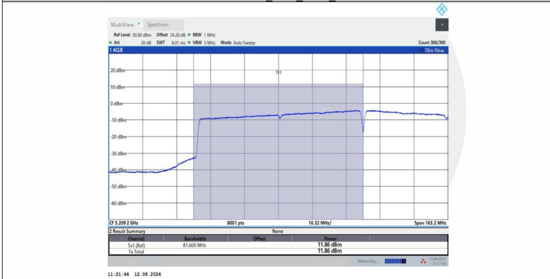
11AX160MIMO_Ant2_5250_UNII-1
