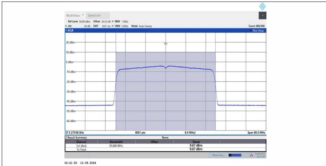
11BE40MIMO_Ant2_5270
