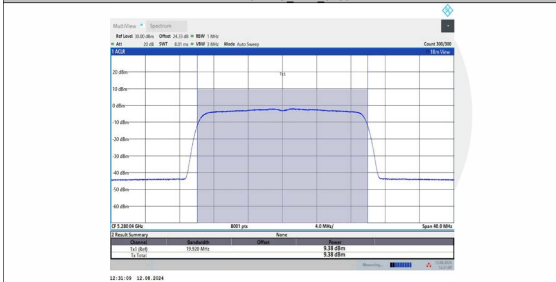
11BE20MIMO Ant2_5280
