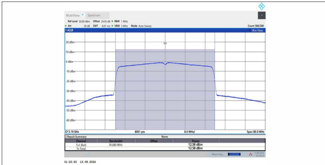
11BE40MIMO_Ant2_5190
