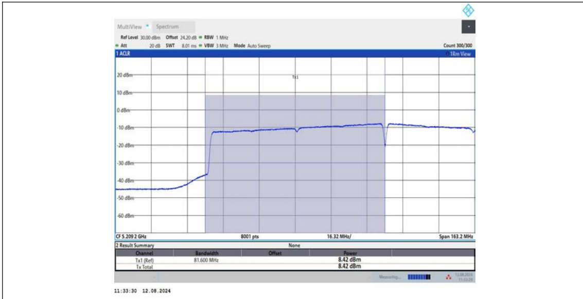
11AX160MIMO_Ant1_5250_UNII-1
