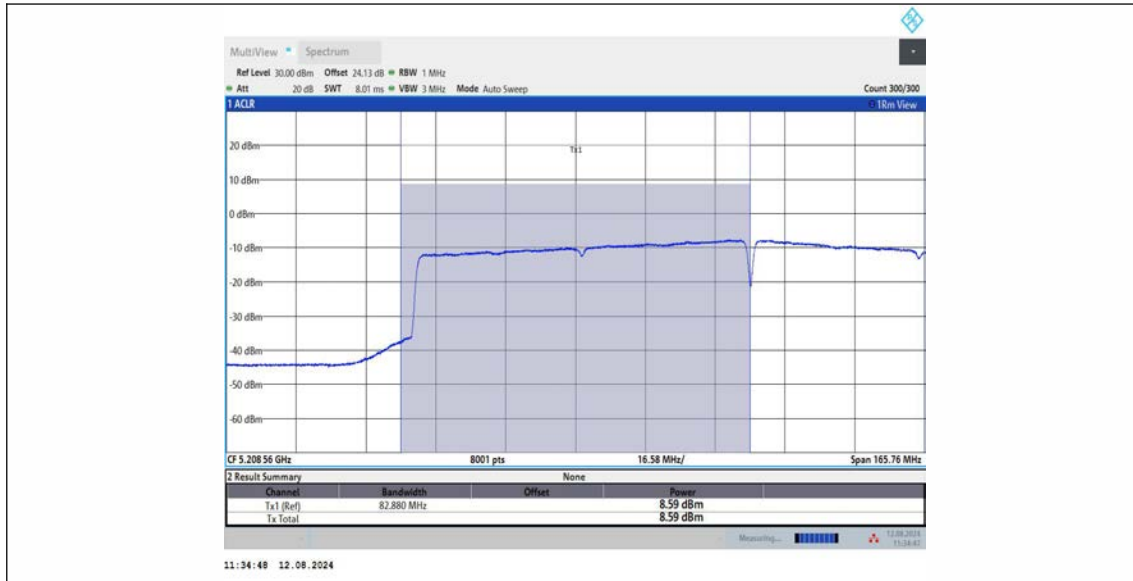
11AX160MIMO_Ant3_5250_UNII-1
