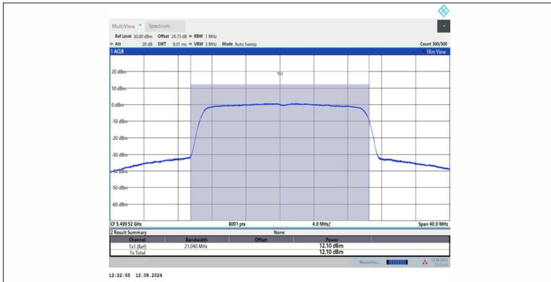
11BE20MIMO Ant2_5500
