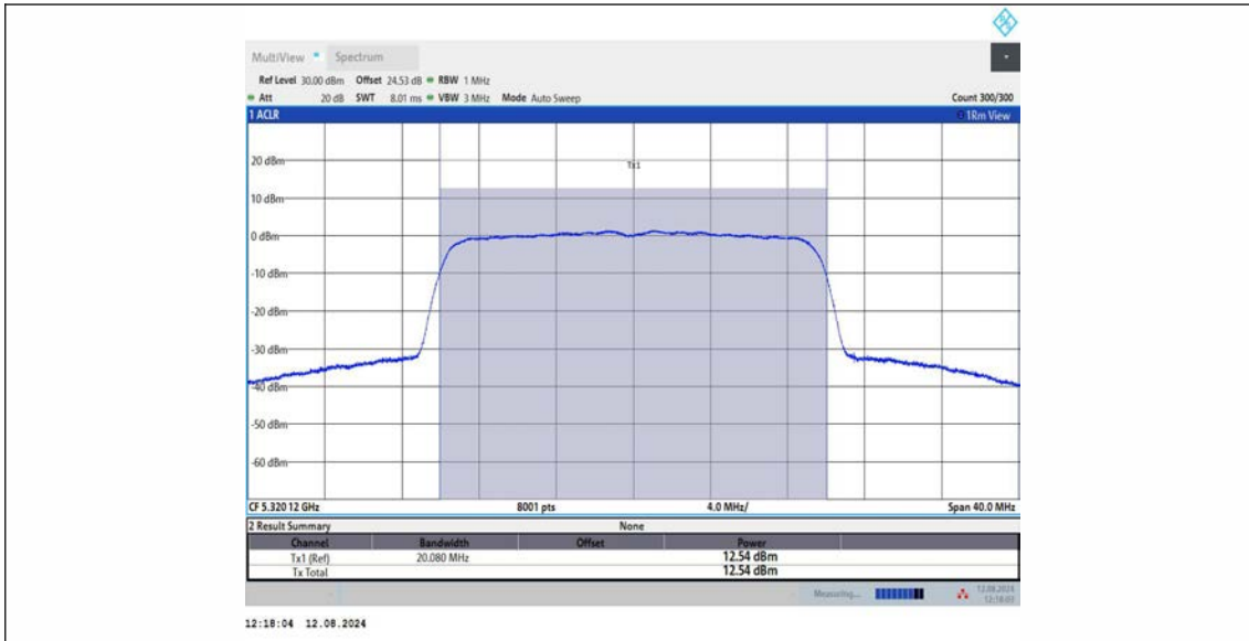
11BE20MIMO Ant3 5320
