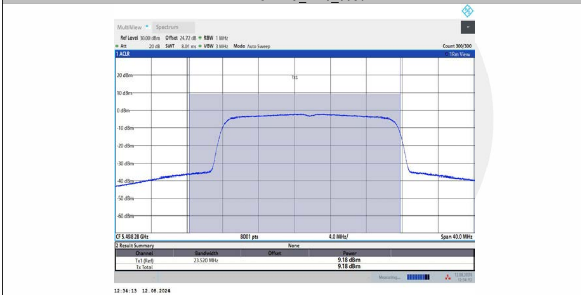
11BE20MIMO Ant3 5500
