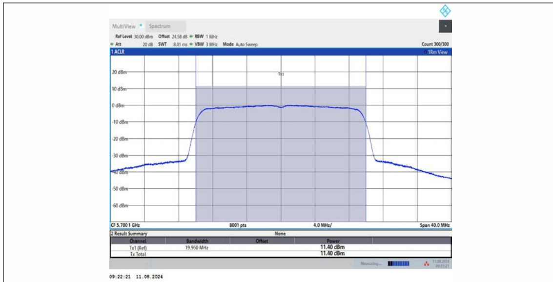
11AX20MIMO Ant2_5700
