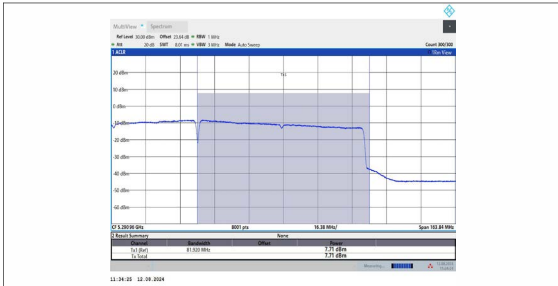
11AX160MIMO_Ant2_5250_UNII-2A
