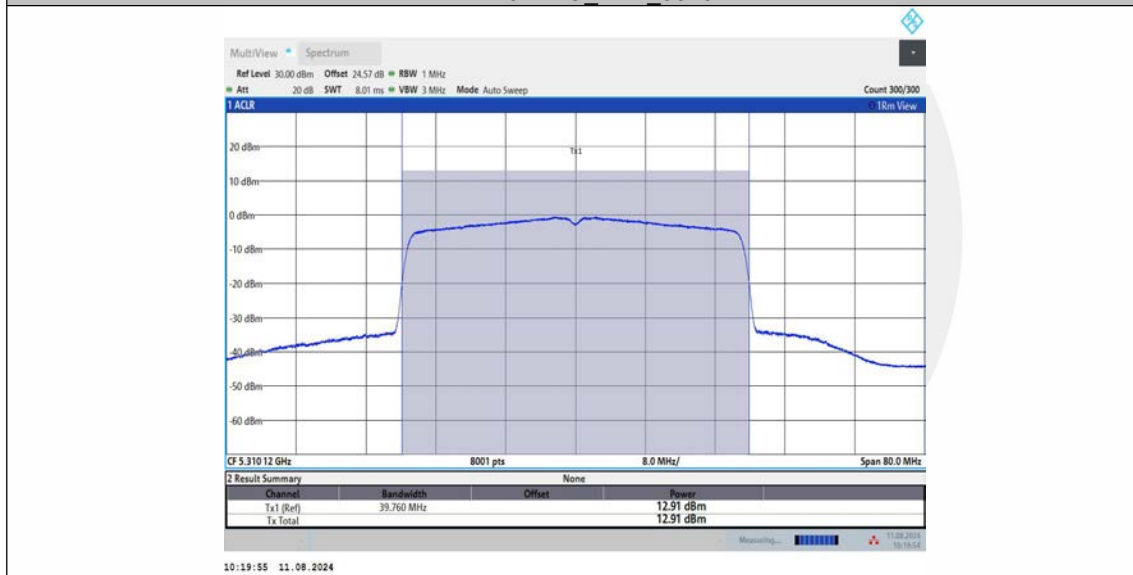
11AX40MIMO_Ant3_5310
