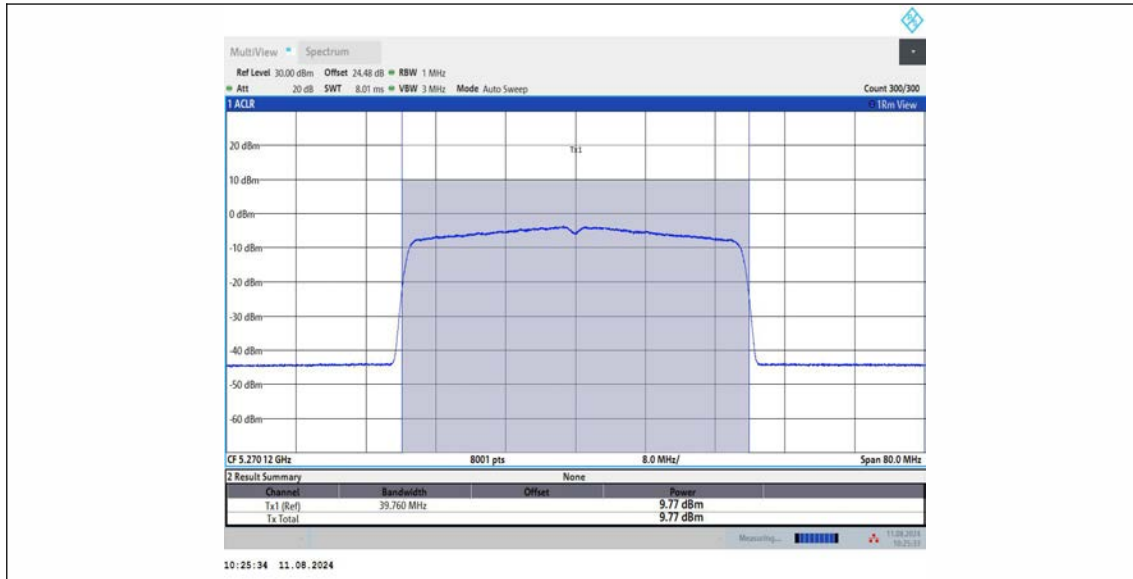
11AX40MIMO_Ant1_5270
