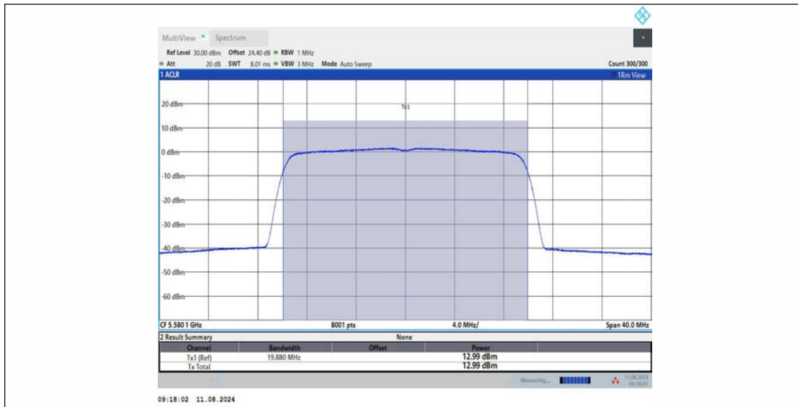
11AX20MIMO Ant3 5580
