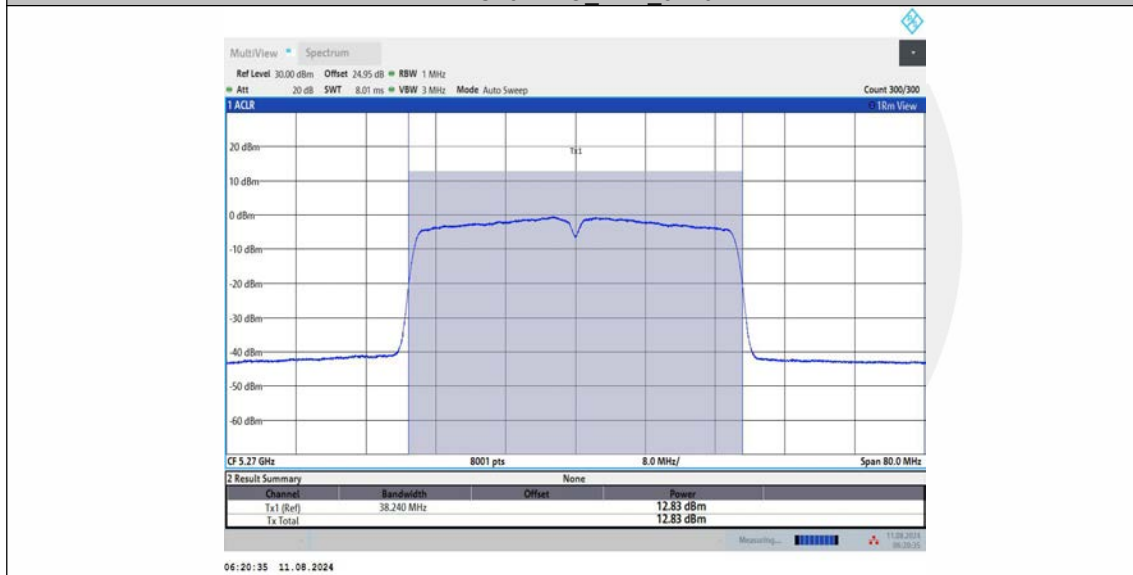
11AC40MIMO_Ant3_5270
