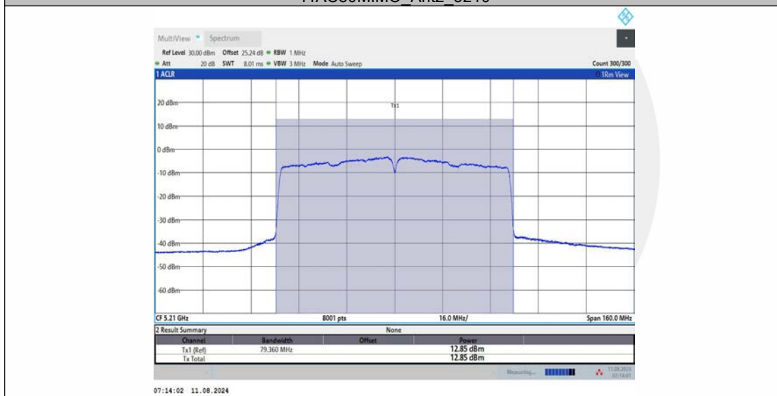
11AC80MIMO_Ant3_5210
