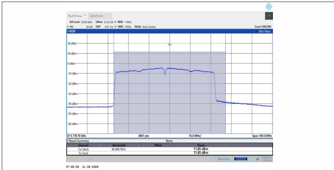
11AC80MIMO_Ant3_5775
