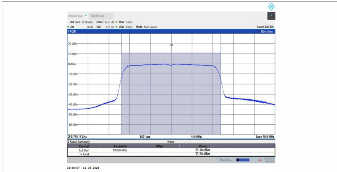
11AC20MIMO_Ant3_5745
