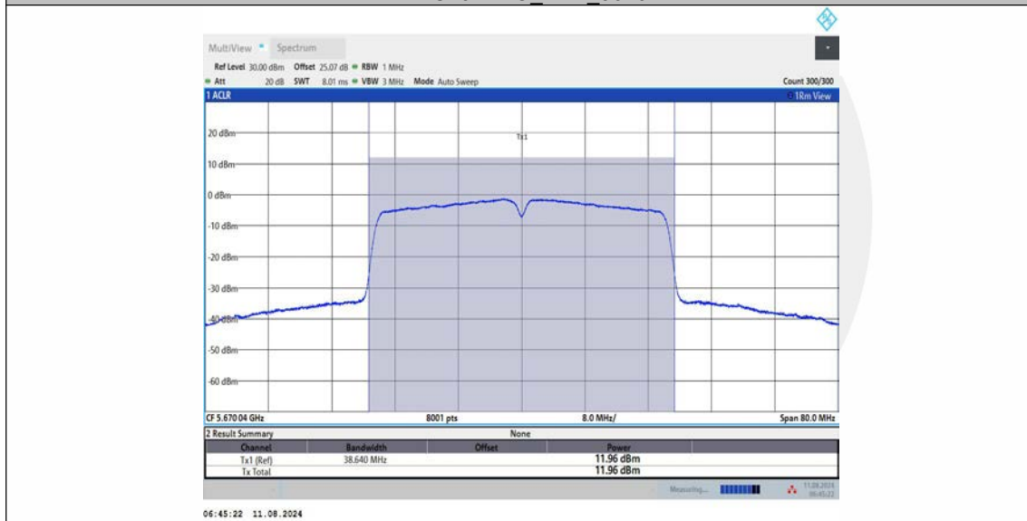
11AC40MIMO_Ant3_5670
