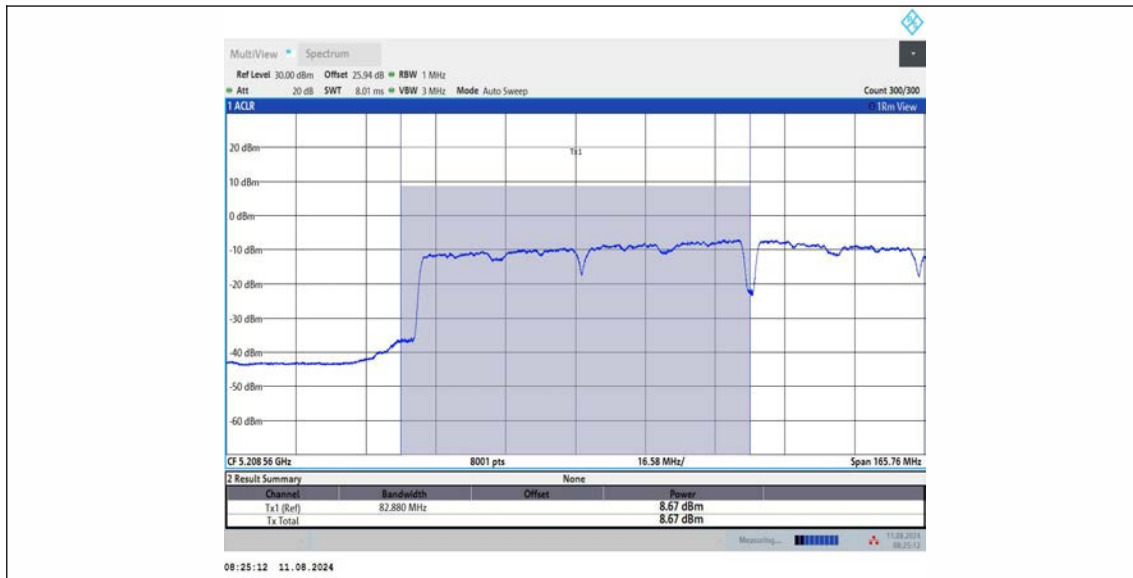
11AC160MIMO_Ant2_5250_UNII-1
