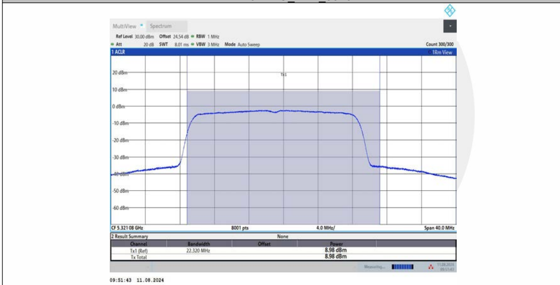
11AX20MIMO Ant2_5320
