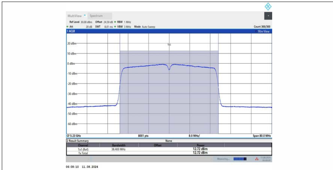
11AC40MIMO_Ant3_5230
