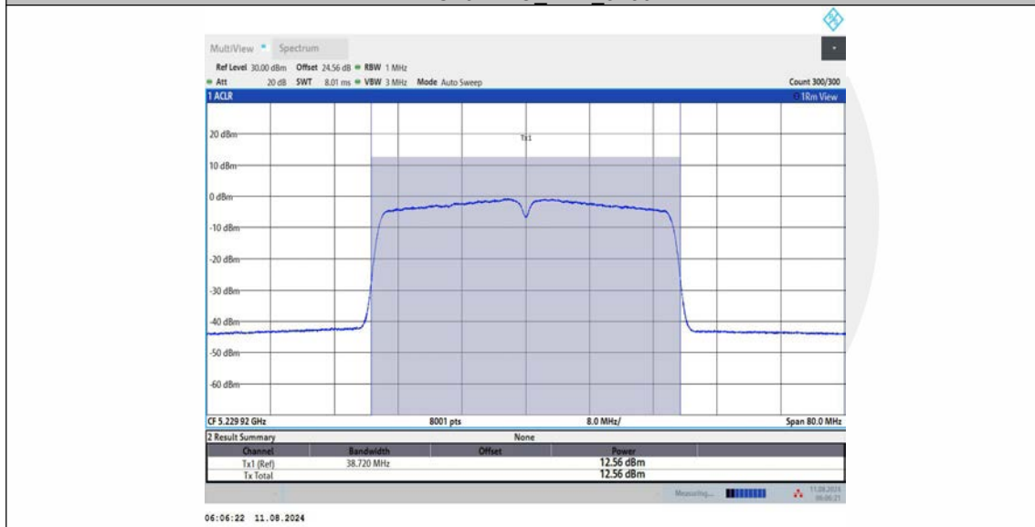
11AC40MIMO_Ant2_5230
