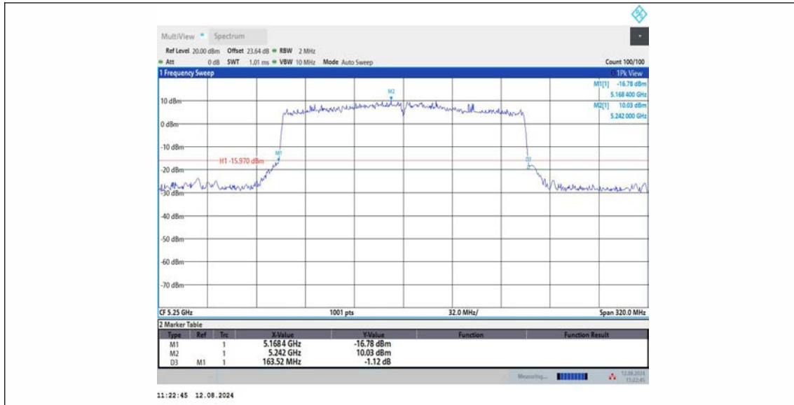
11AX160MIMO_Ant3_5250
