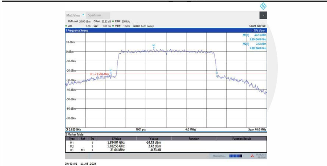
11AX20MIMO_Ant3_5825
