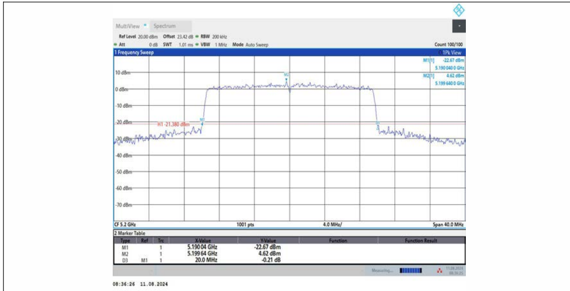
11AX20MIMO_Ant2_5200
