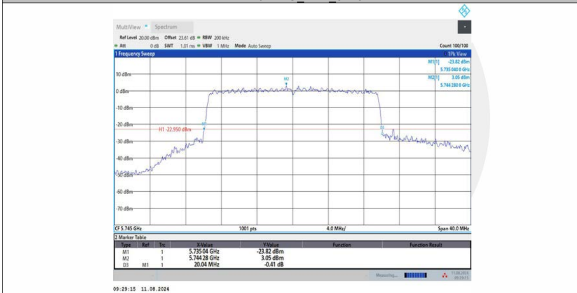
11AX20MIMO_Ant3_5745
