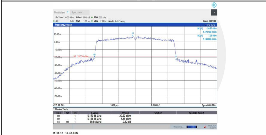
11AX40MIMO_Ant2_5190
