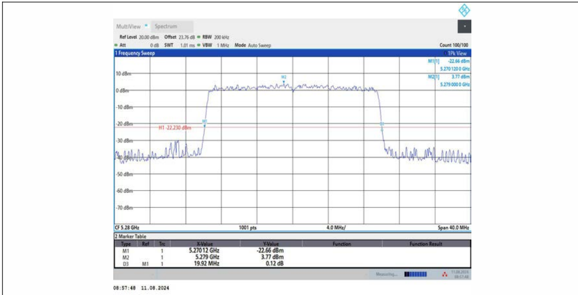
11AX20MIMO_Ant3_5280
