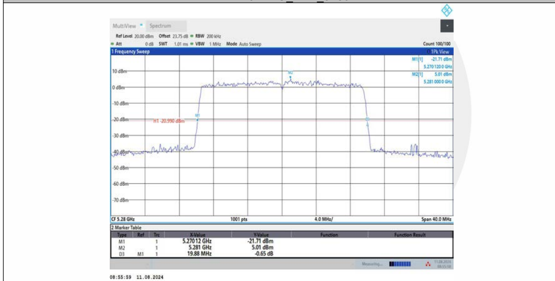
11AX20MIMO_Ant2_5280
