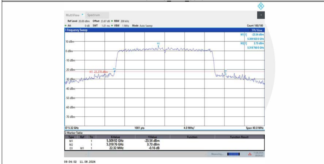
11AX20MIMO_Ant3_5320
