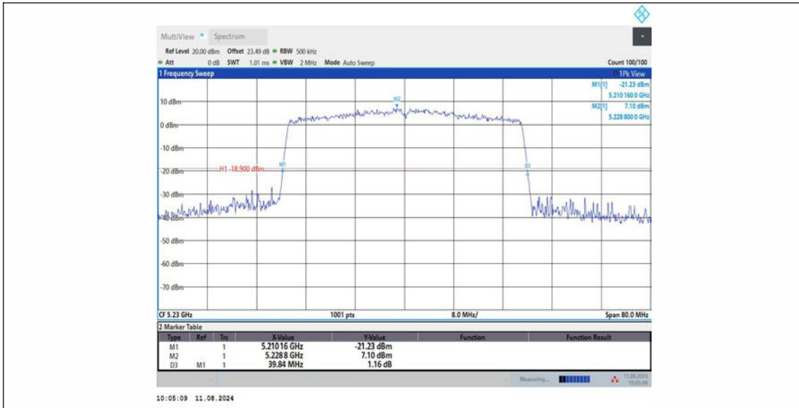
11AX40MIMO_Ant2_5230
