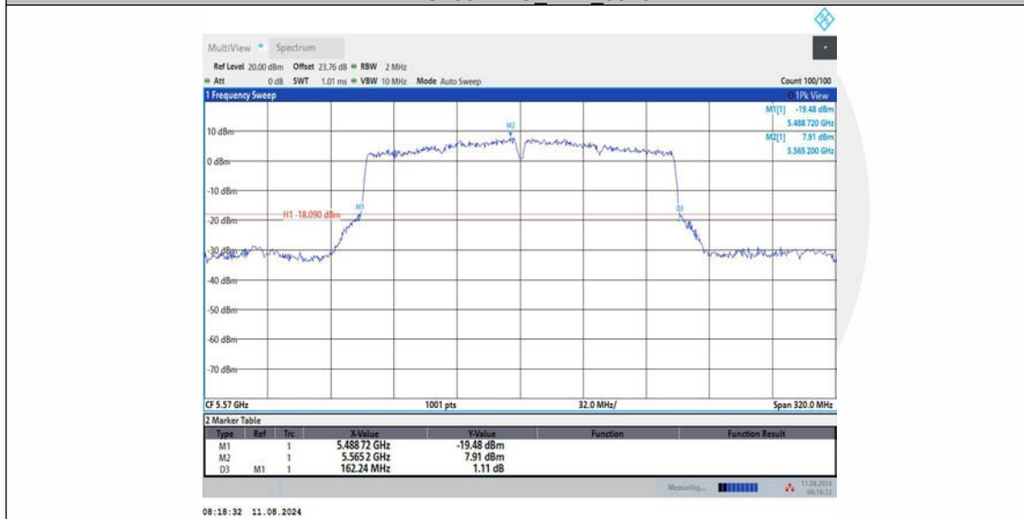
11AC160MIMO_Ant3_5570
