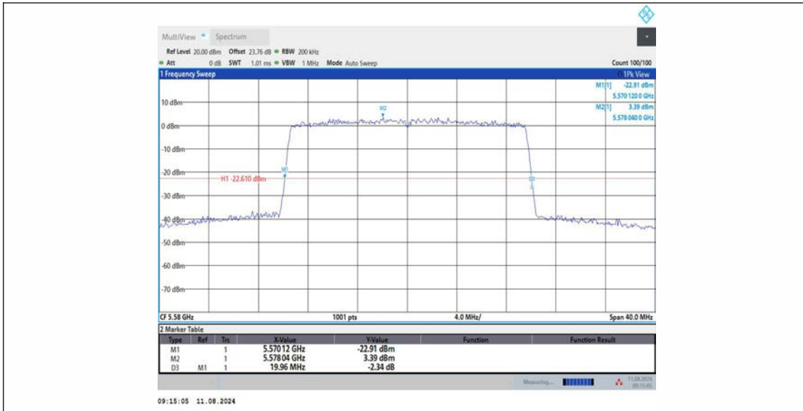
11AX20MIMO_Ant2_5580
