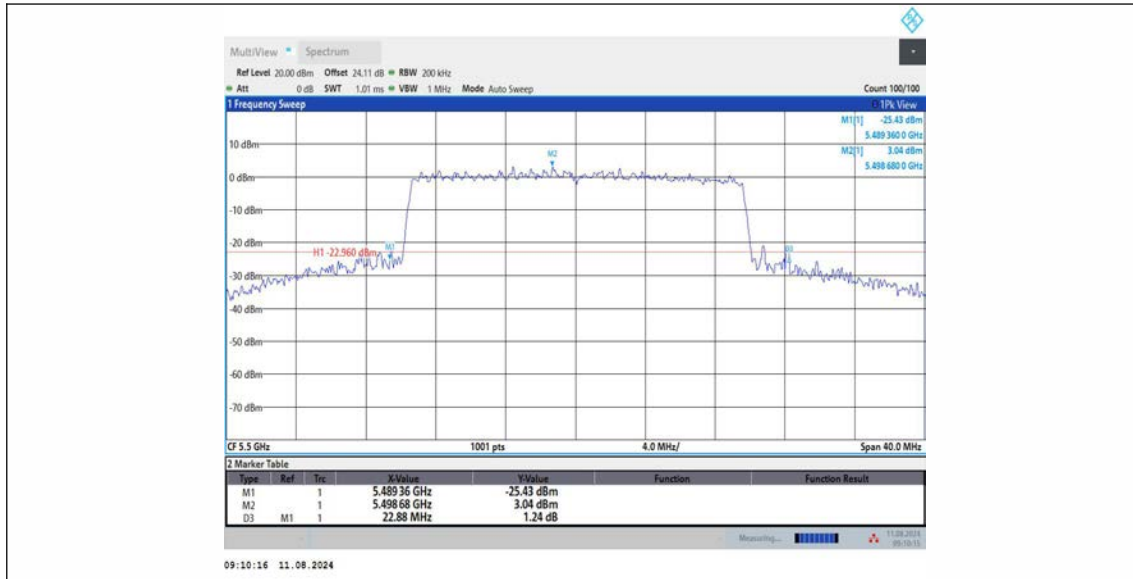
11AX20MIMO_Ant3_5500
