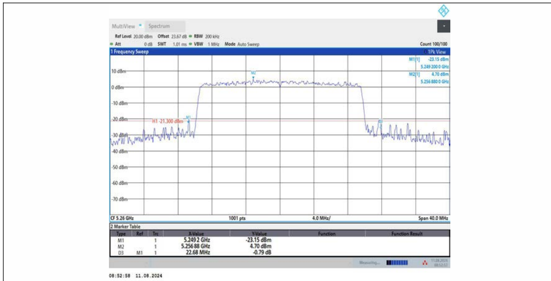
11AX20MIMO_Ant1_5280
