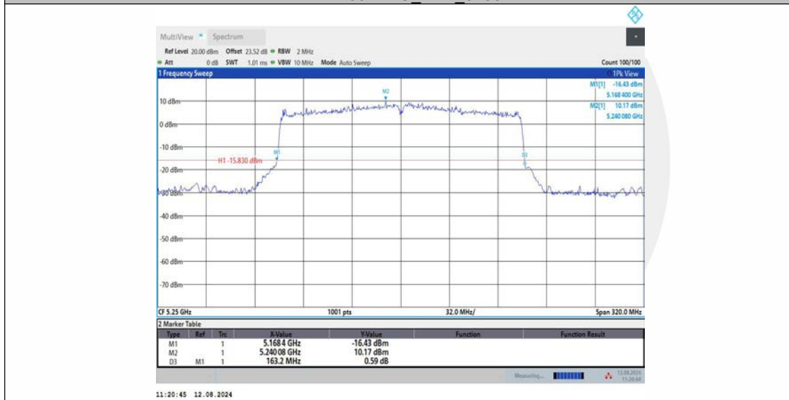
11AX160MIMO_Ant2_5250
