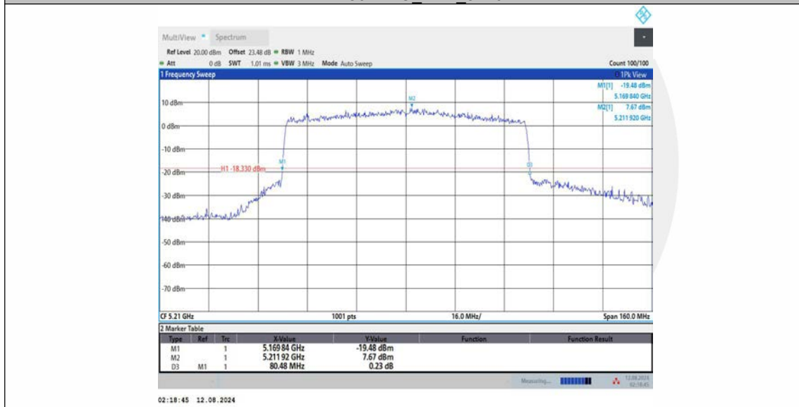
11AX80MIMO_Ant3_5210
