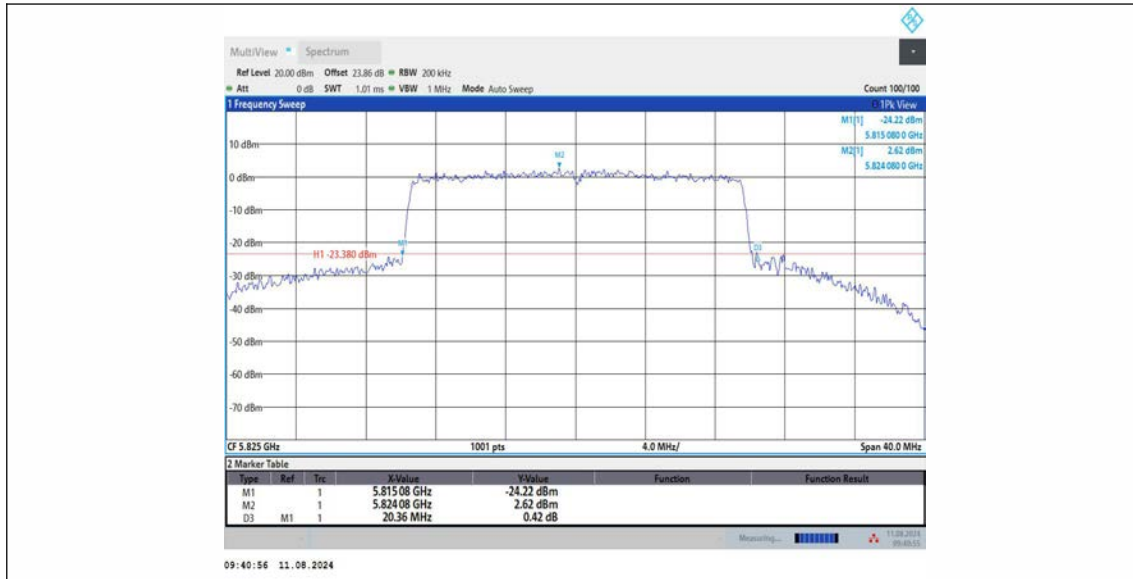
11AX20MIMO_Ant2_5825
