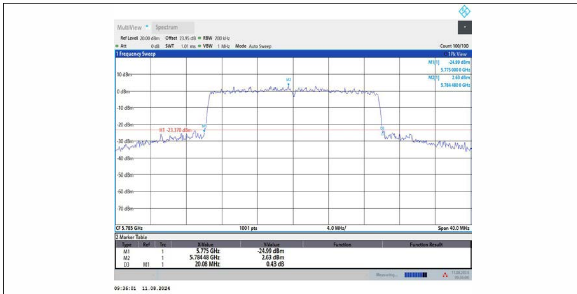
11AX20MIMO_Ant3_5785
