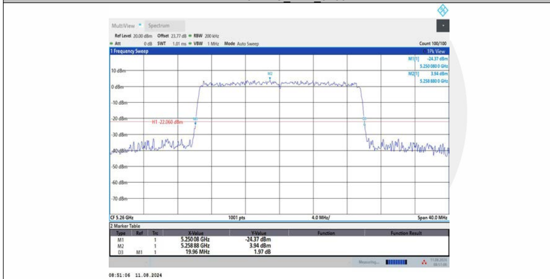
11AX20MIMO_Ant3_5260
