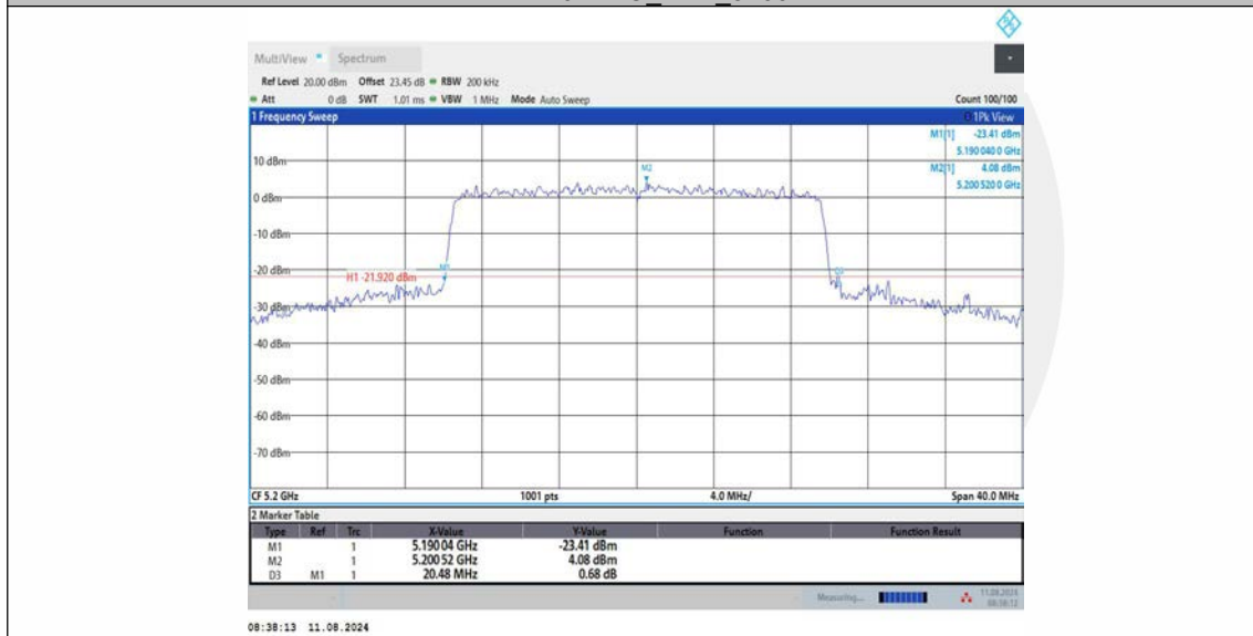
11AX20MIMO_Ant3_5200
