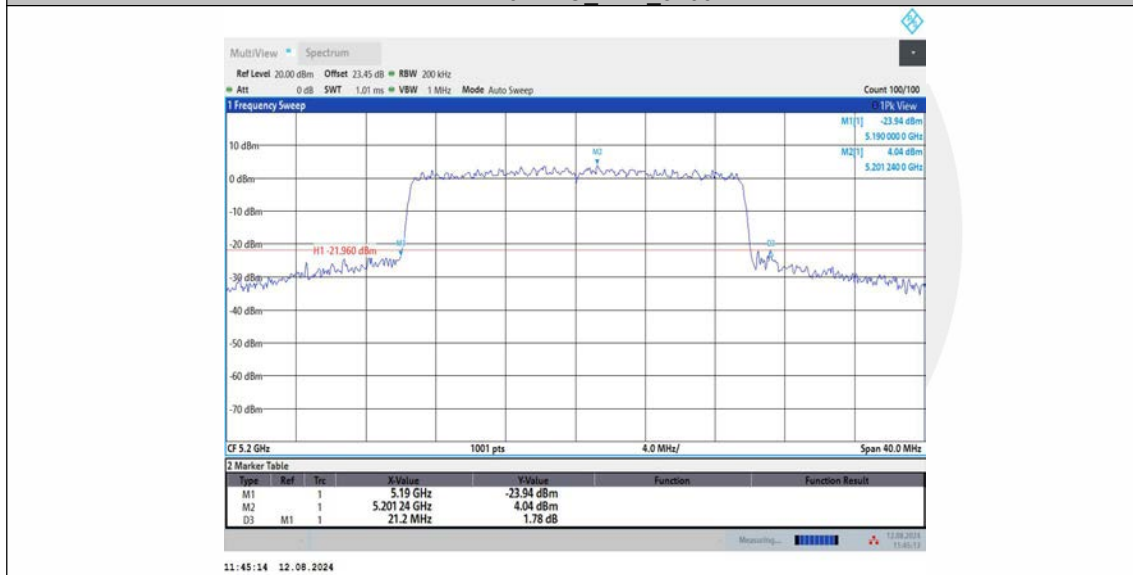
11BE20MIMO_Ant3_5200
