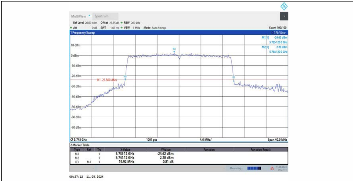
11AX20MIMO_Ant2_5745
