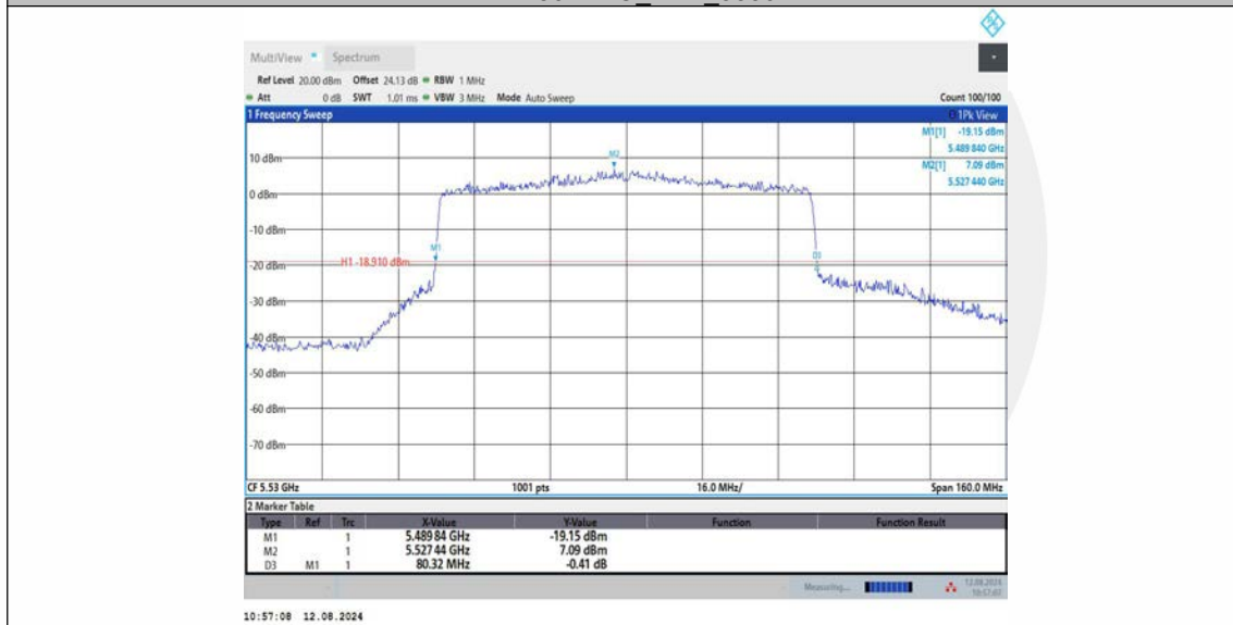
11AX80MIMO_Ant3_5530
