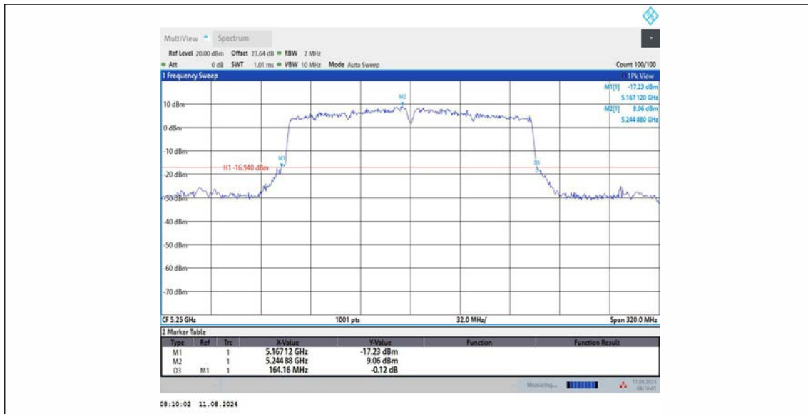
11AC160MIMO_Ant3_5250
