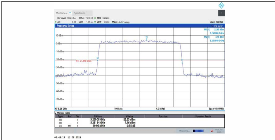
11AX20MIMO_Ant2_5260
