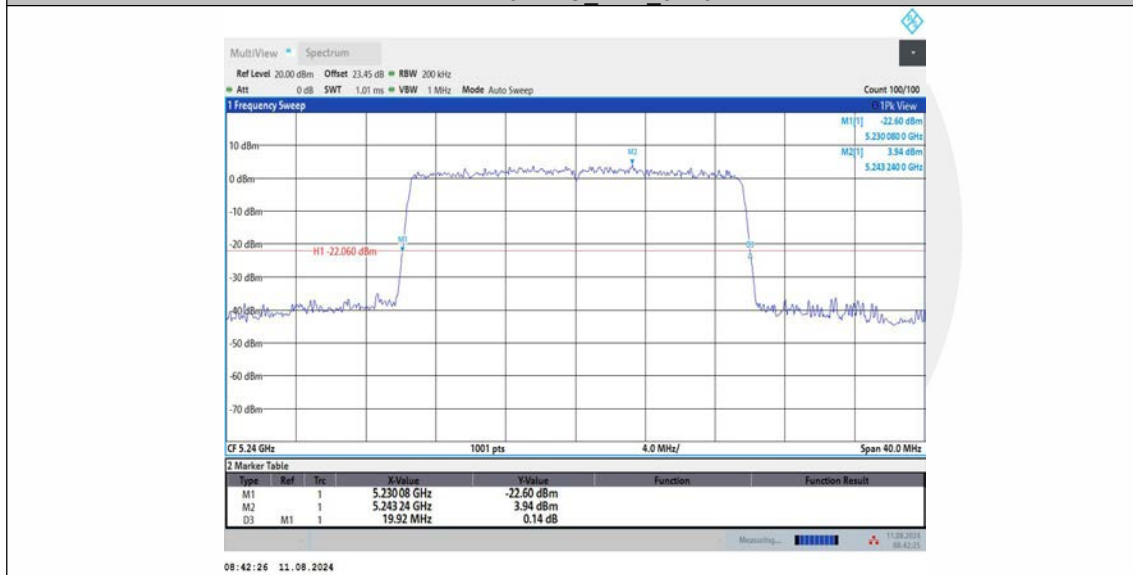
11AX20MIMO_Ant2_5240
