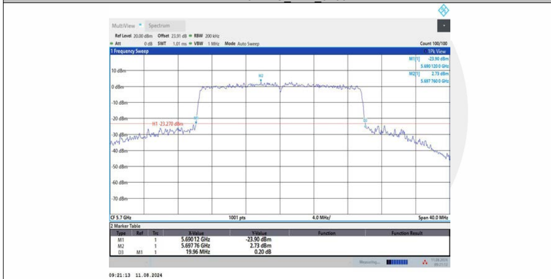
11AX20MIMO Ant2_5700
