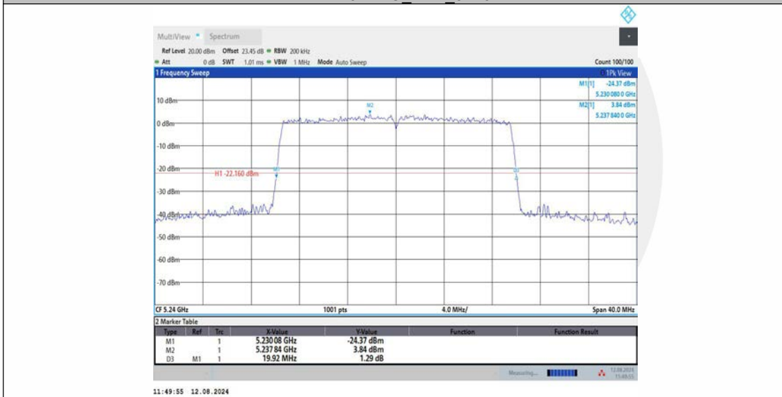
11BE20MIMO_Ant2_5240
