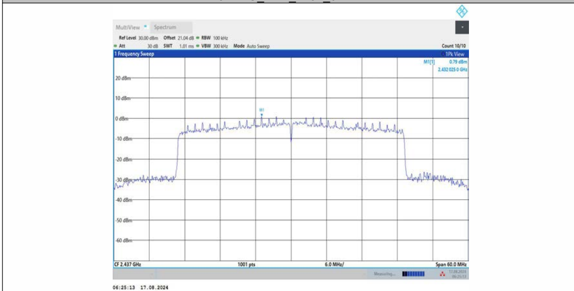
11AX40MIMO_Ant2_2437_0~Reference
