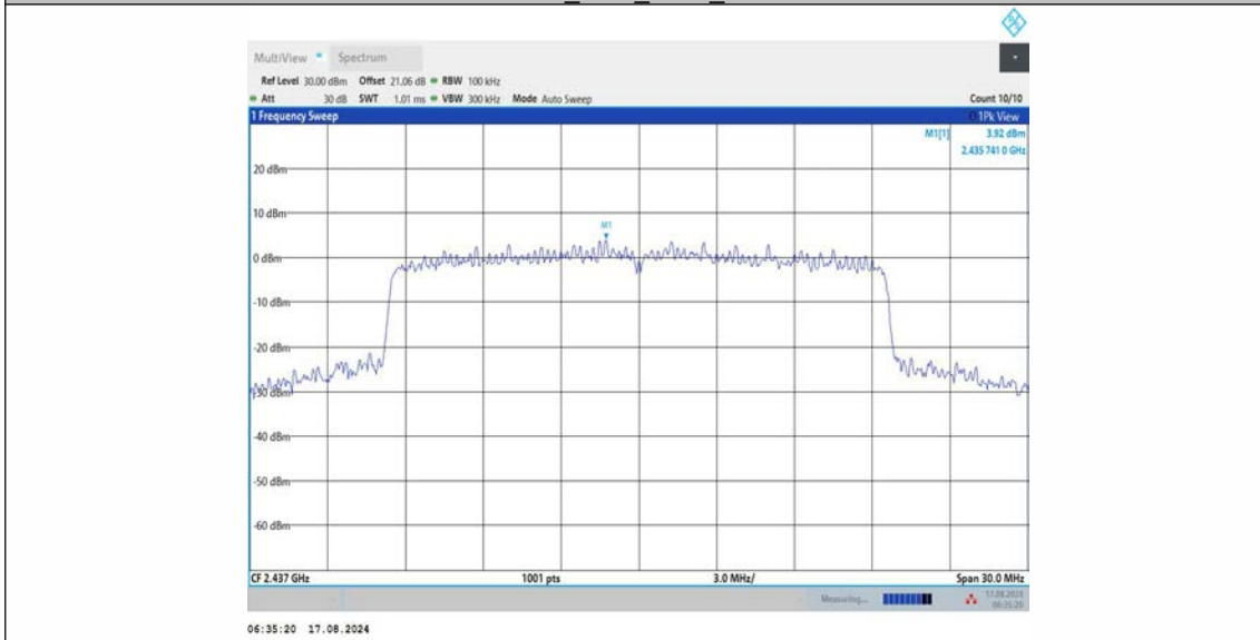
11BE20MIMO_Ant1_2437_0~Reference
