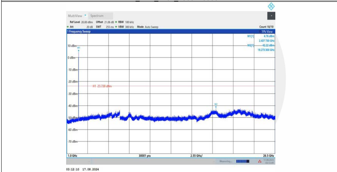
11B_Ant2_2437_0~Reference
