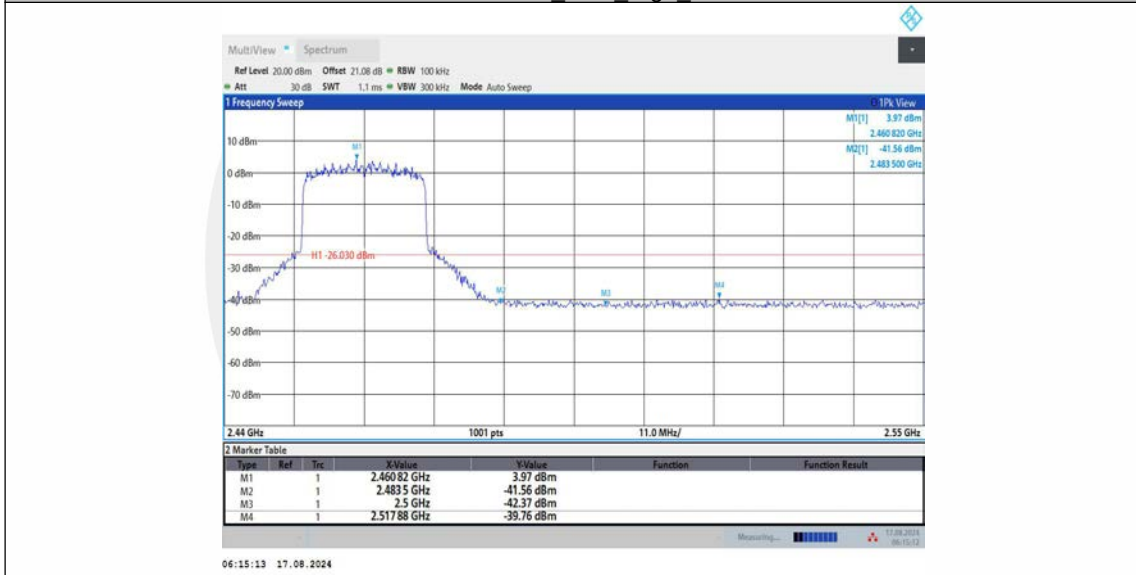
11AX20MIMO_Ant2_High_2462
