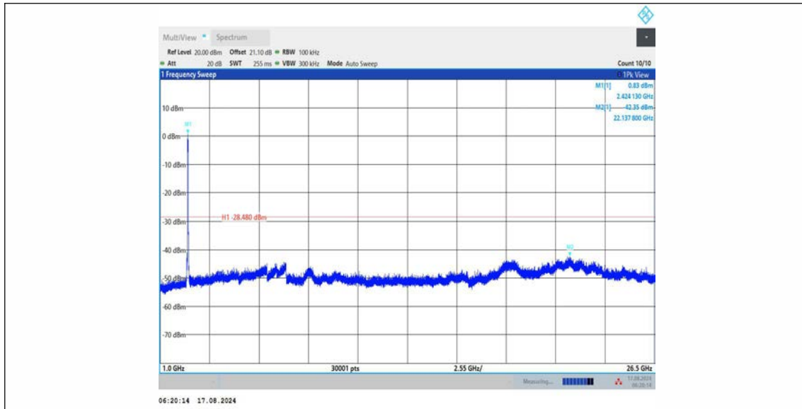
11AX40MIMO_Ant2_2422_0~Reference
