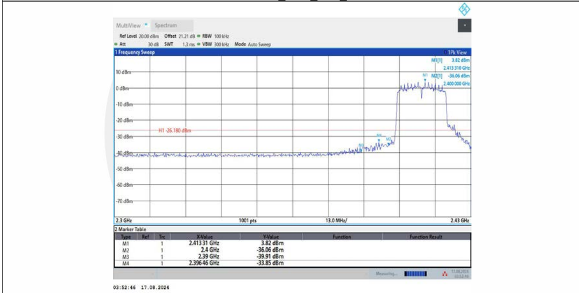
11N20MIMO_Ant2_Low_2412
