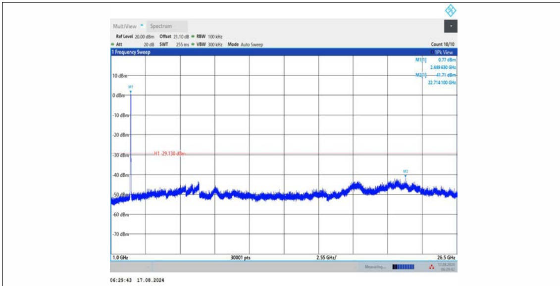
11BE20MIMO_Ant1_2412_0~Reference
