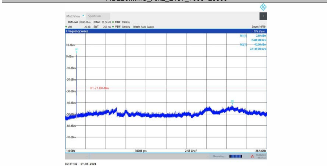
11BE20MIMO_Ant2_2437_1000~26500
