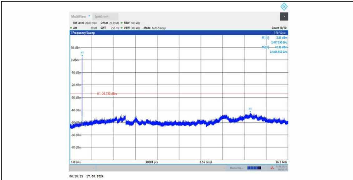
11AX20MIMO_Ant1_2437_0~Reference
