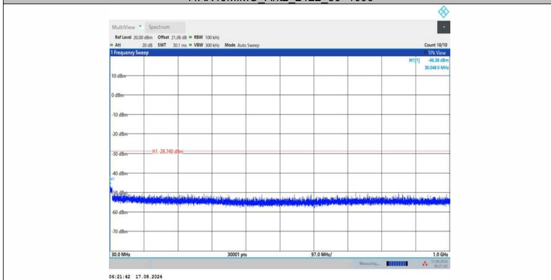
11AX40MIMO_Ant2_2422_30~1000
