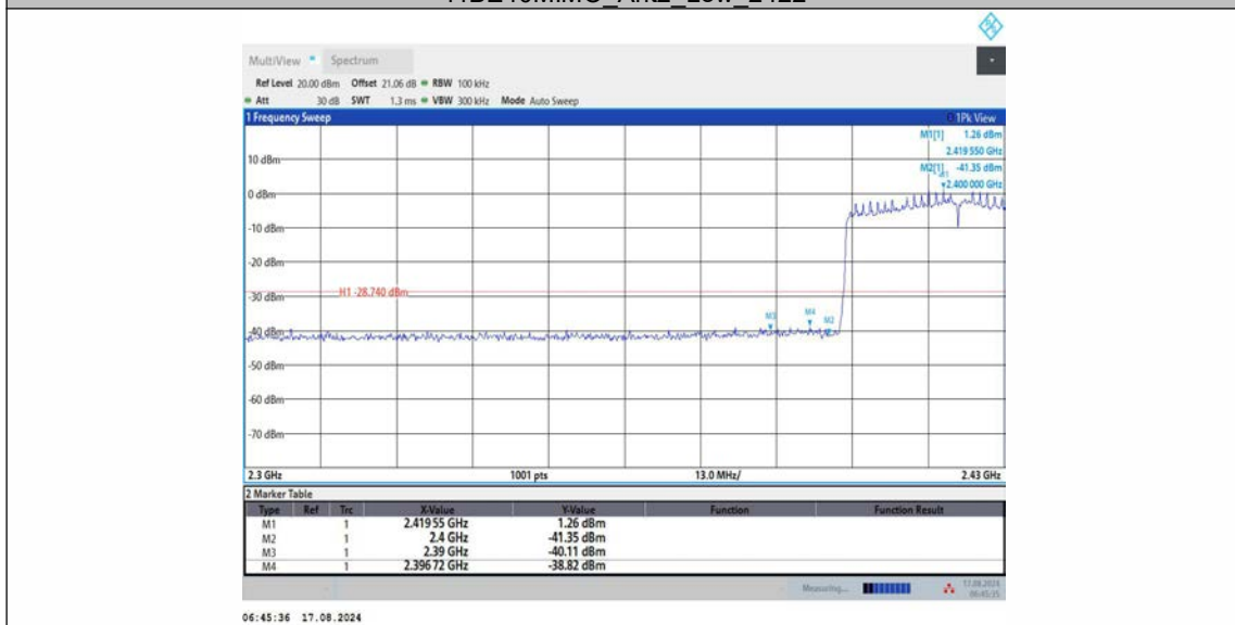
11BE40MIMO_Ant2_Low_2422
