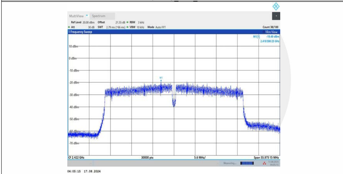
11N40MIMO_Ant2_2422
