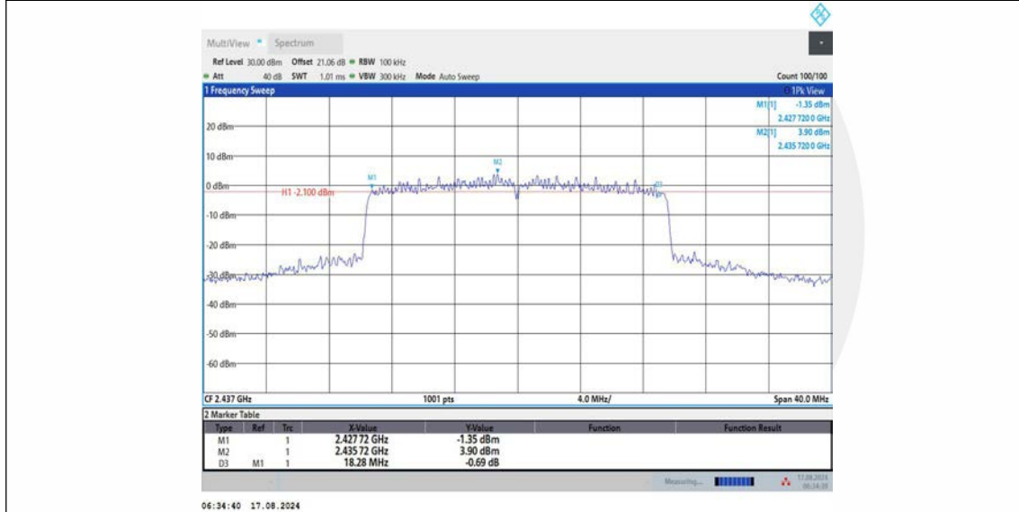
11BE20MIMO_Ant2_2437
