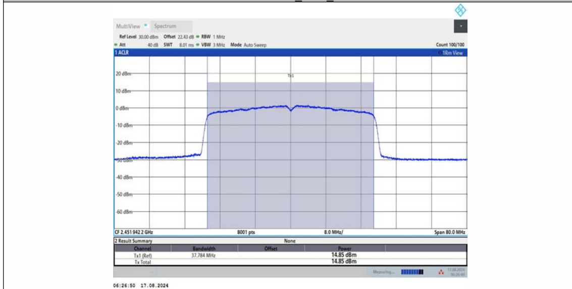
11AX40MIMO_Ant1_2452
