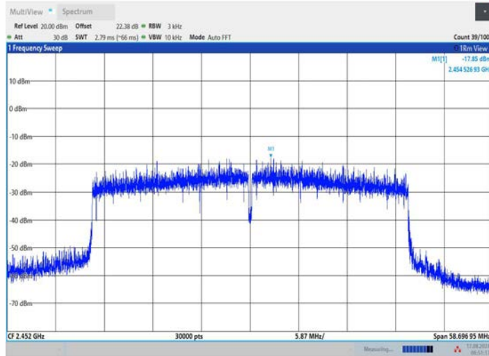
11BE40MIMO_Ant2_2452
