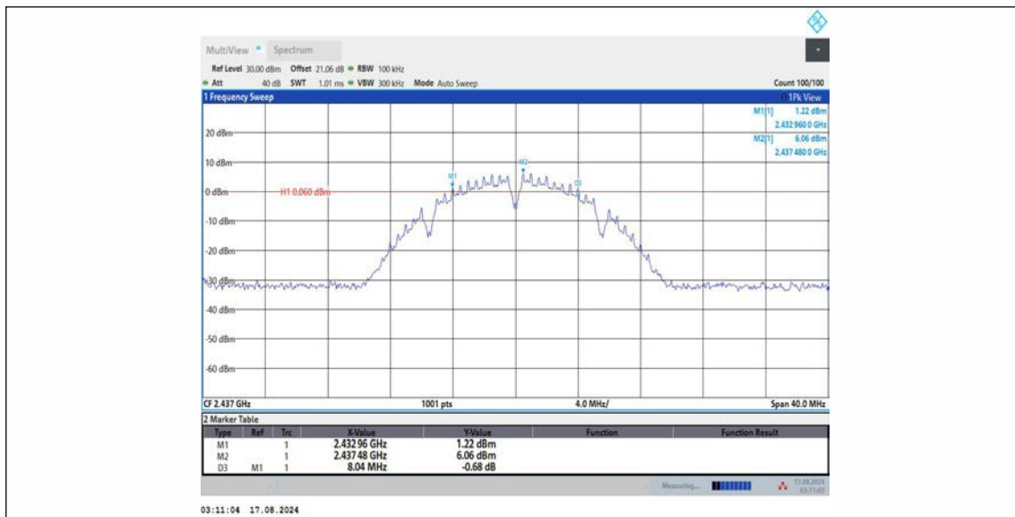
11B_Ant2_2437
