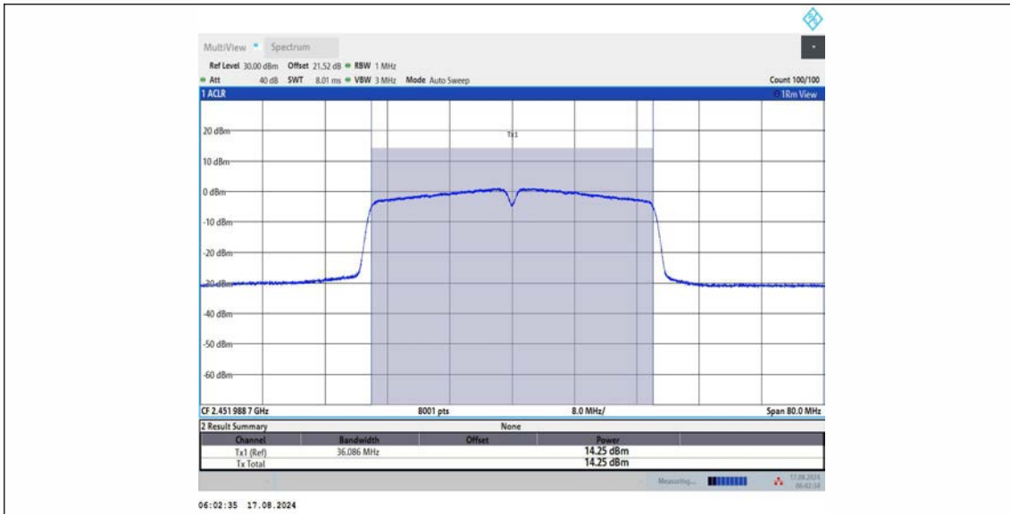
11N40MIMO Ant2_2452
