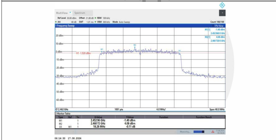
11AX20MIMO_Ant2_2462
