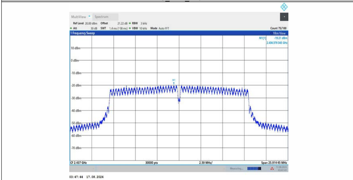
11G_Ant2_2437
