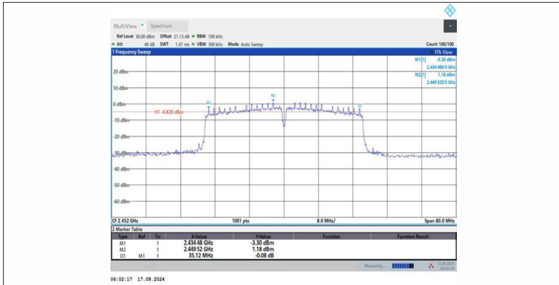
11N40MIMO_Ant2_2452
