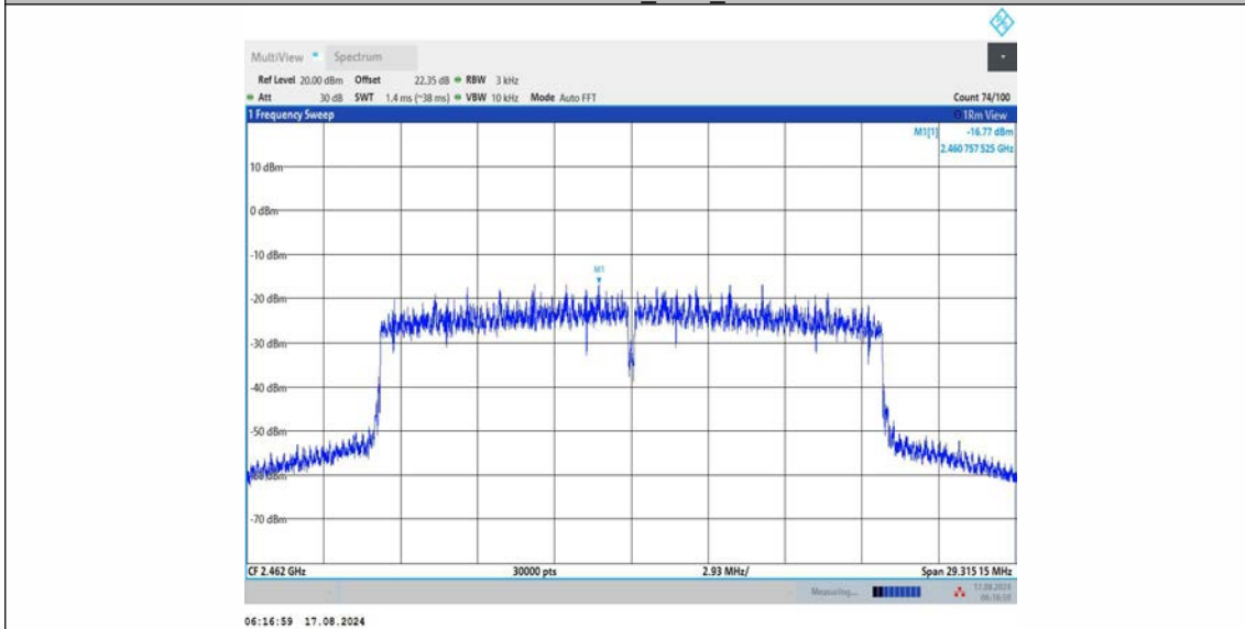
11AX20MIMO_Ant2_2462
