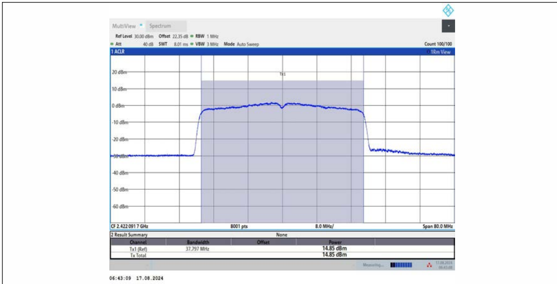
11BE40MIMO_Ant2_2422
