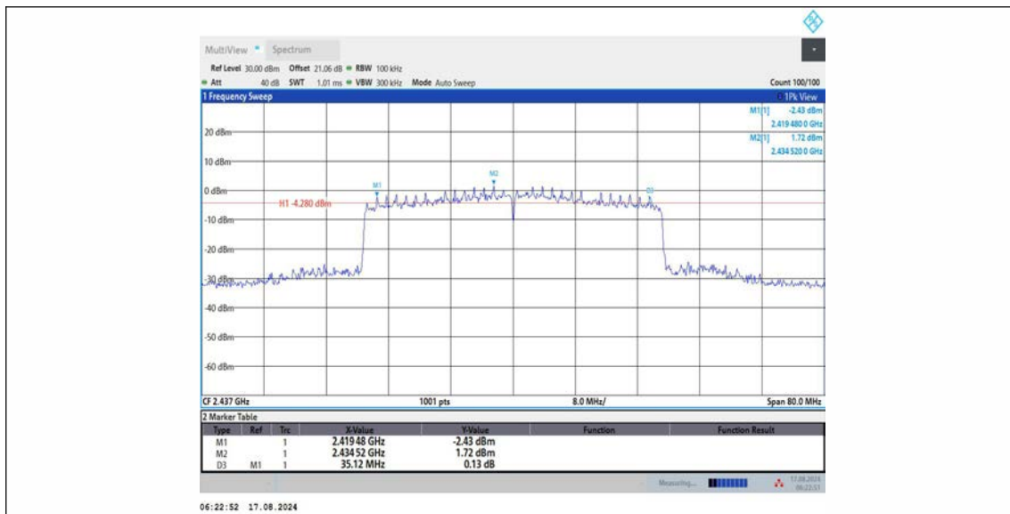
11AX40MIMO_Ant2_2437
