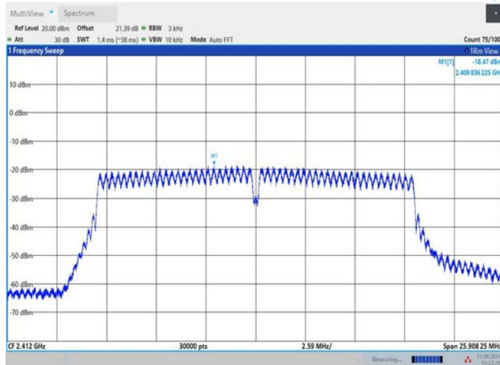
11G_Ant2_2412
