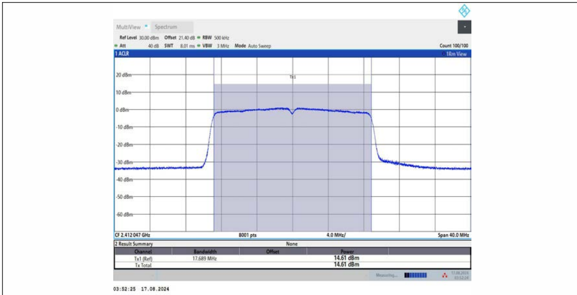
11N20MIMO_Ant2_2412
