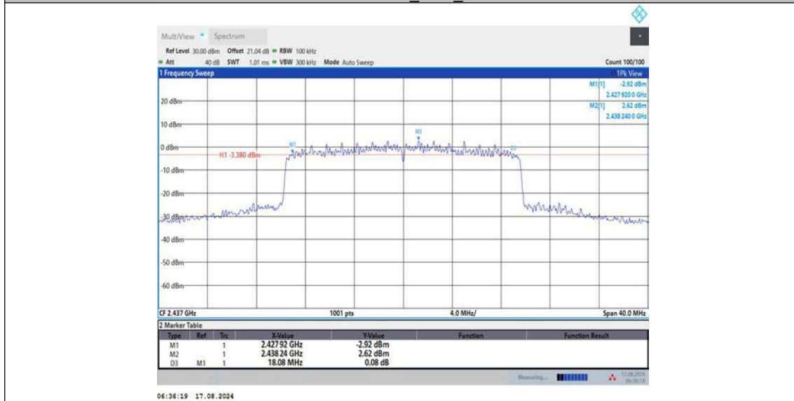
11BE20MIMO_Ant2_2437
