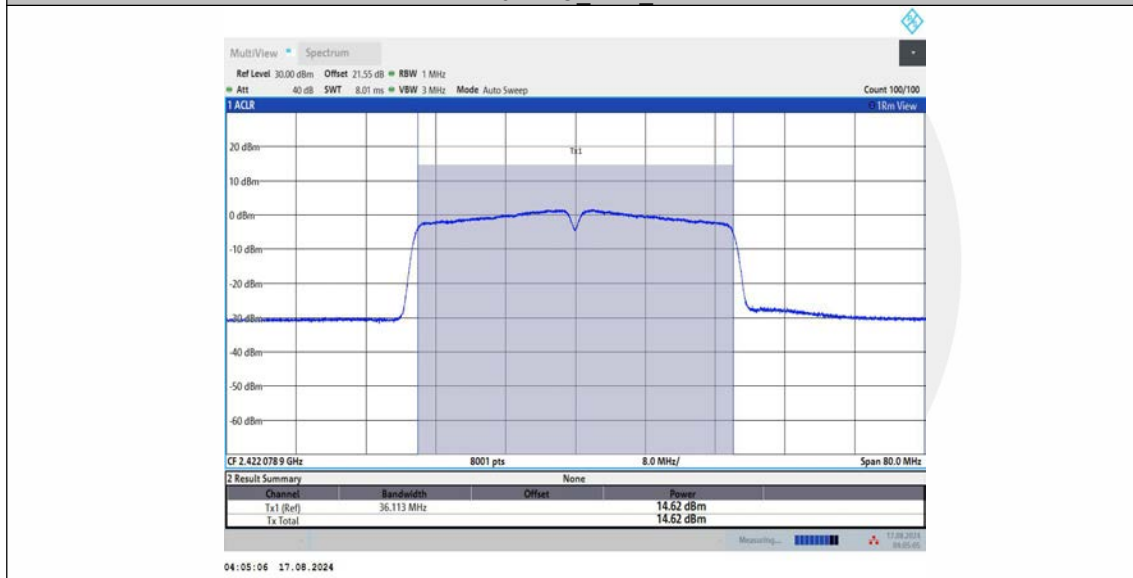
11N40MIMO_Ant2_2422
