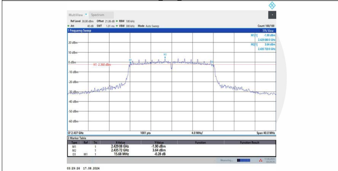
11G_Ant2_2437
