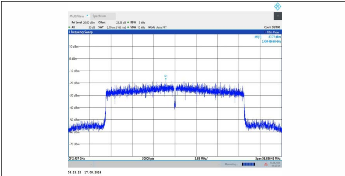
11AX40MIMO_Ant2_2437
