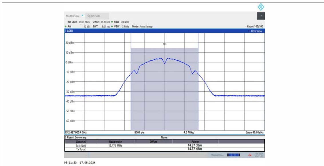
11B_Ant2_2437
