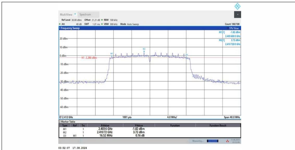
11N20MIMO_Ant2_2412
