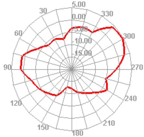
5500.000MHz E2
