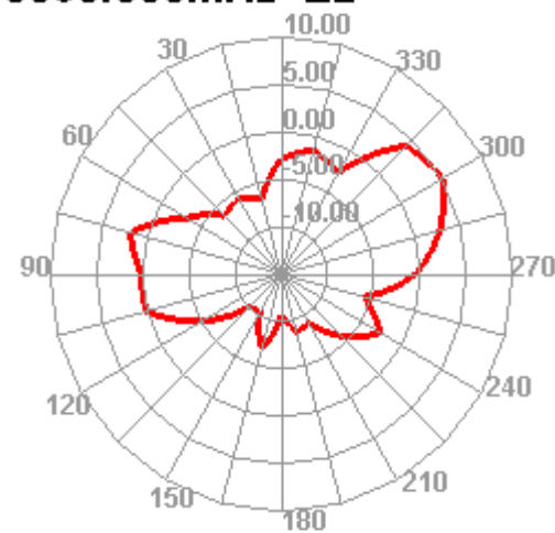
5560.000MHz E2
