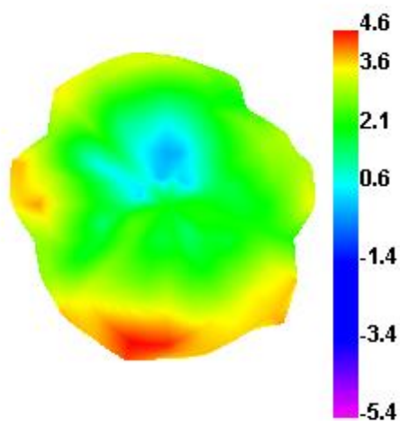
5750.000MHz E1
