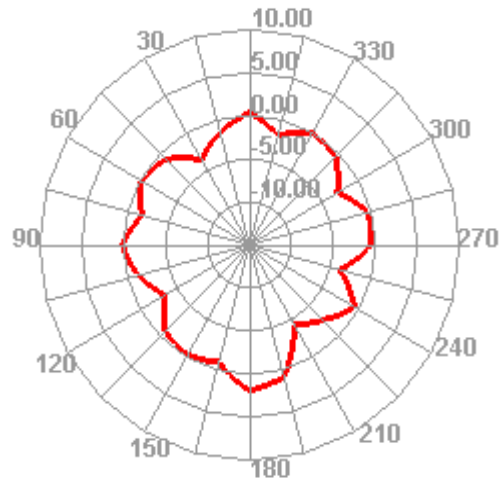
5560.000MHz H
