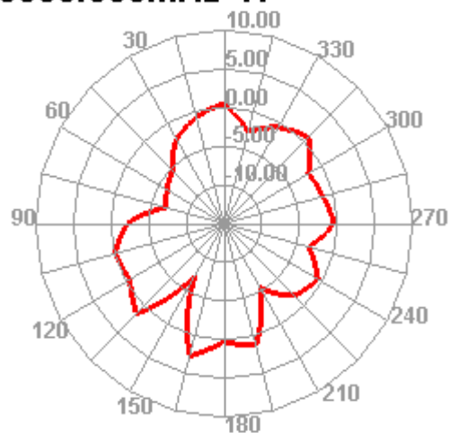
5850.000MHz H
