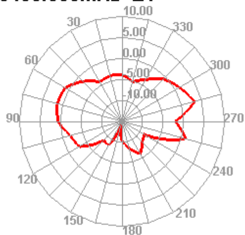
5450.000MHz E1
