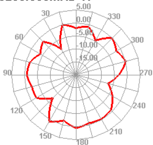
5250.000MHz H
