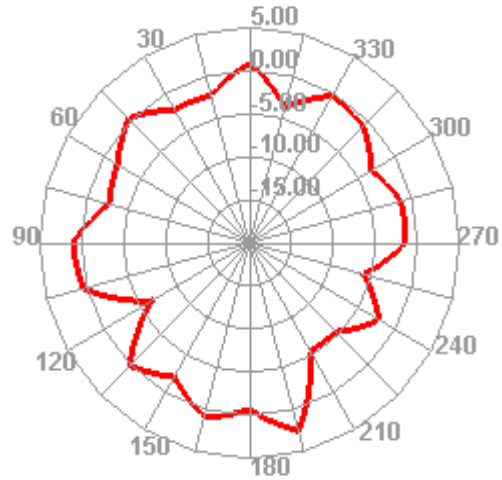
5500.000MHz H
