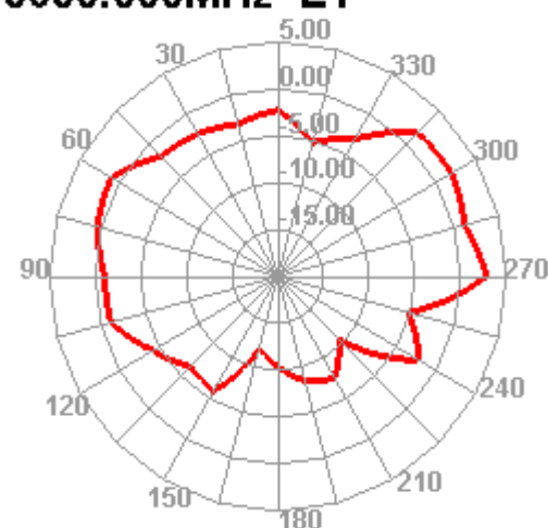
5650.000MHz E1
