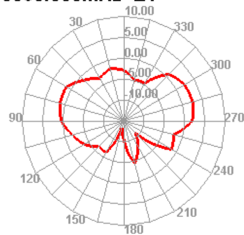
5560.000MHz E1
