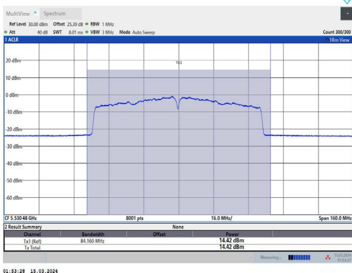
11AC80MIMO_Ant3_5530
