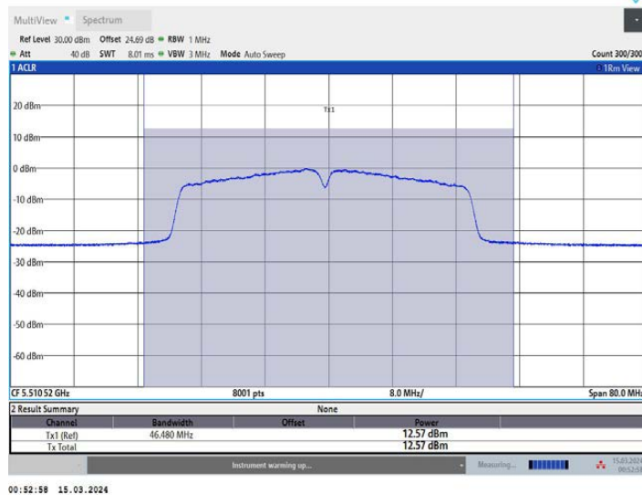
11AC40MIMO_Ant2_5510
