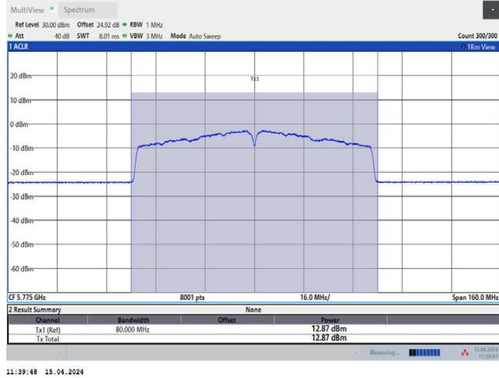
11AC80MIMO_Ant2_5775
