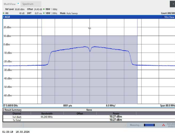
11AC40MIMO_Ant2_5670
