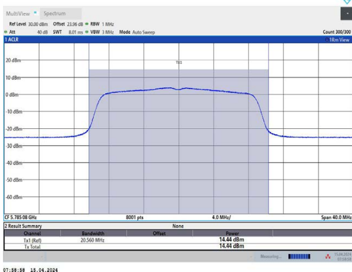
11AC20MIMO_Ant3_5785
