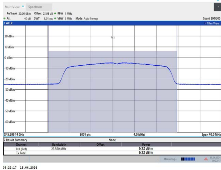
11AX20MIMO_Ant1_5700
