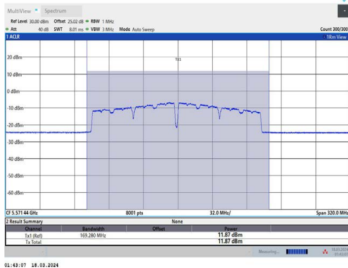
11AC160MIMO_Ant2_5570
