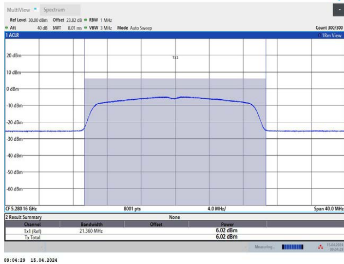
11AX20MIMO Ant1_5280
