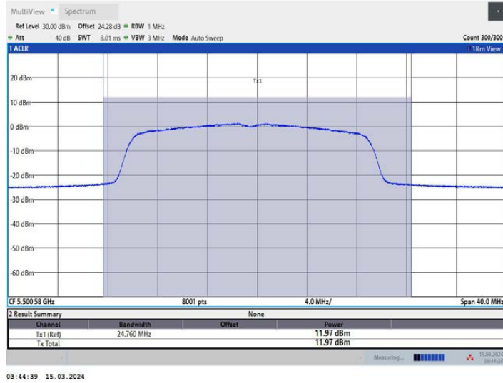
11AX20MIMO_Ant3_5500
