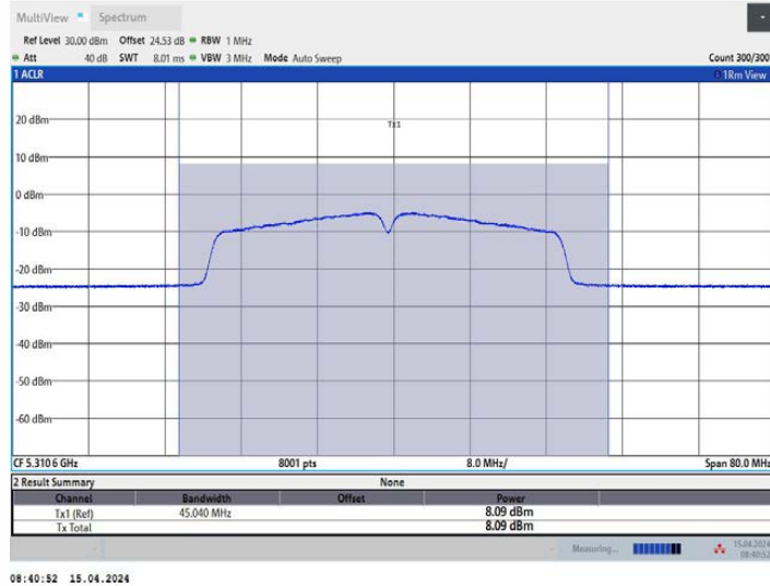
11AC40MIMO_Ant1_5310
