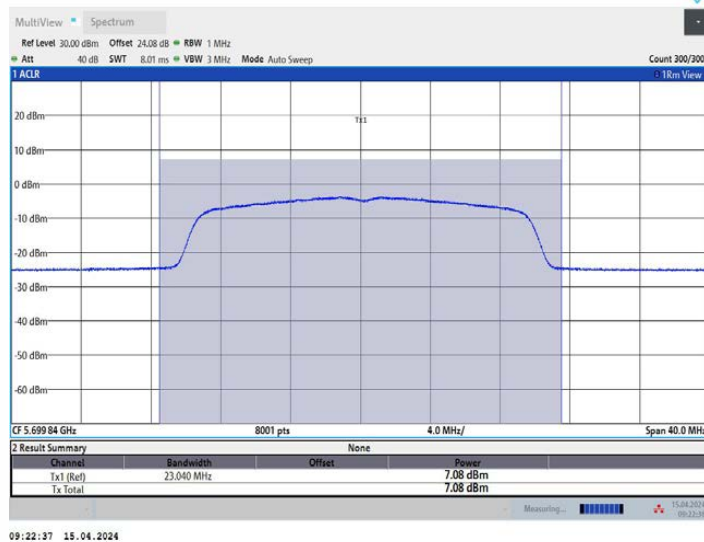
11AX20MIMO_Ant2_5700
