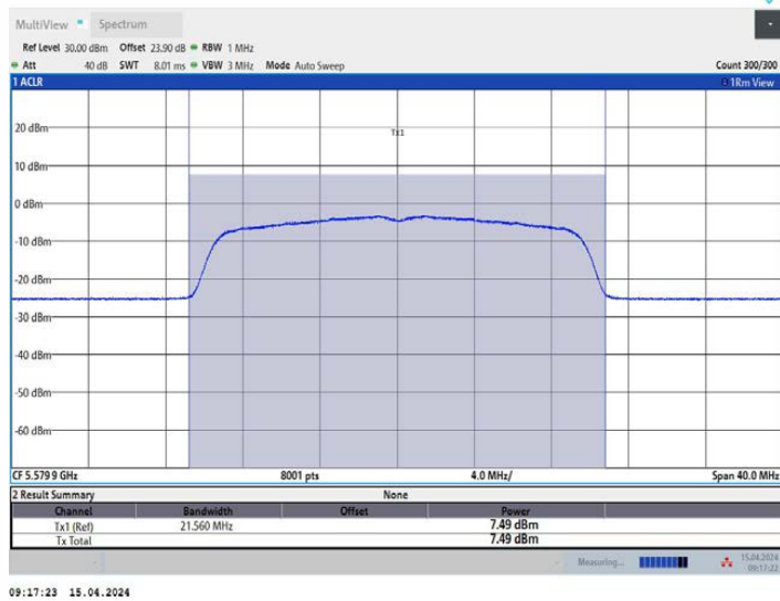
11AX20MIMO_Ant2_5580
