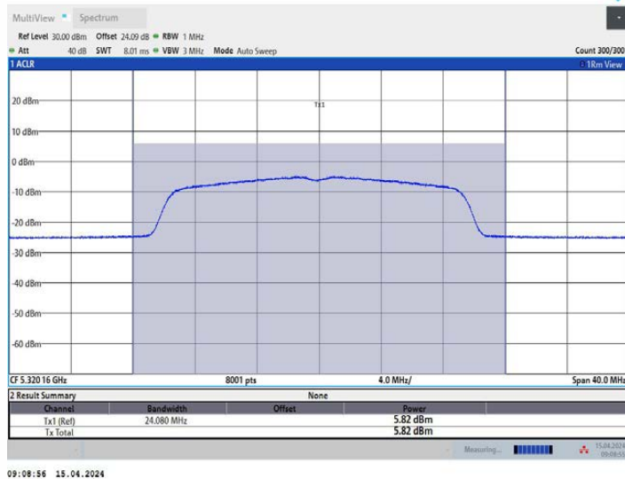
11AX20MIMO_Ant1_5320
