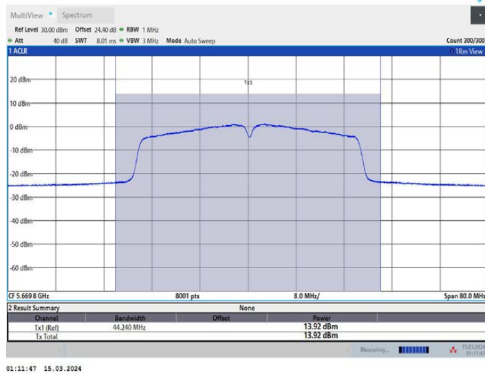
11AC40MIMO_Ant3_5670
