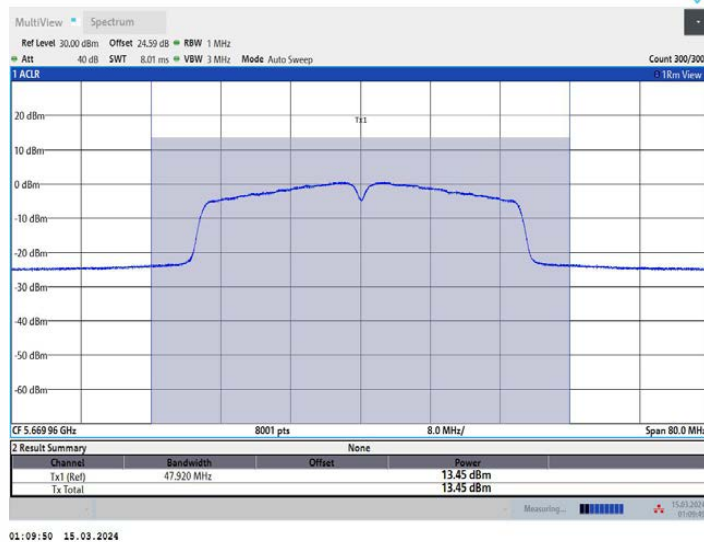
11AC40MIMO_Ant2_5670
