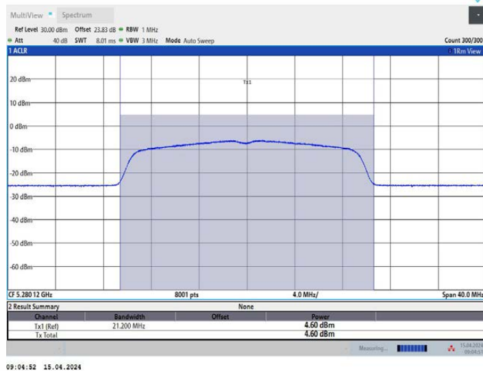
11AX20MIMO_Ant2_5280
