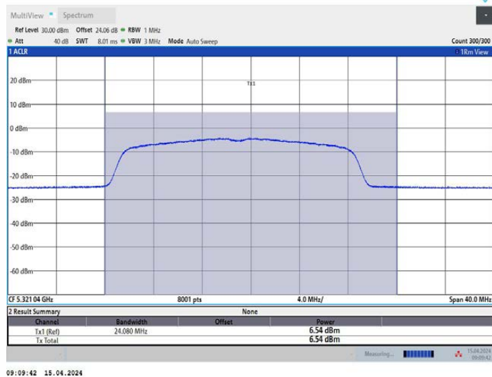
11AX20MIMO_Ant3_5320
