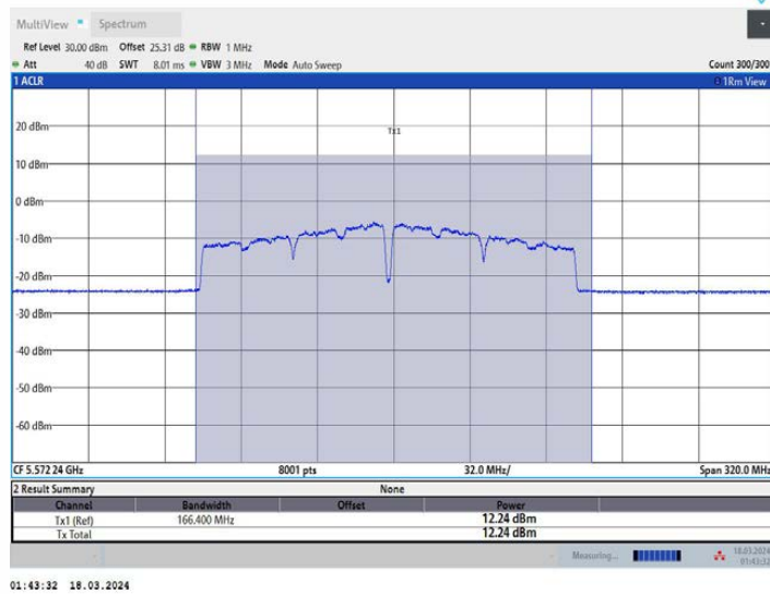
11AC160MIMO_Ant3_5570
