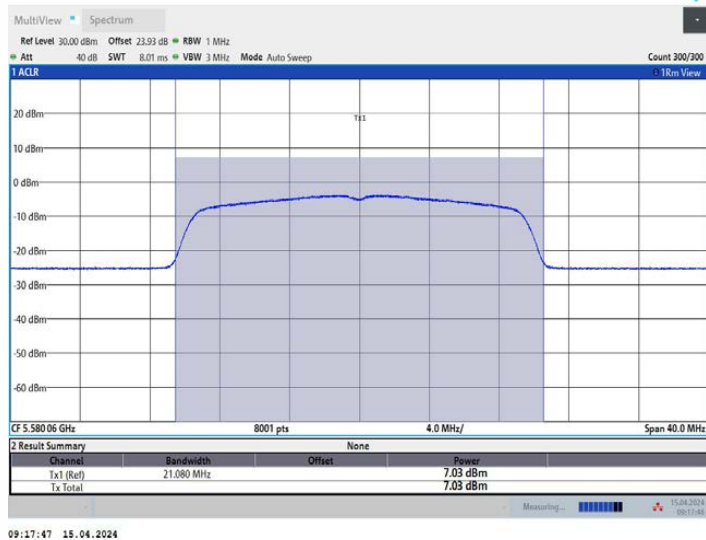
11AX20MIMO_Ant3_5580
