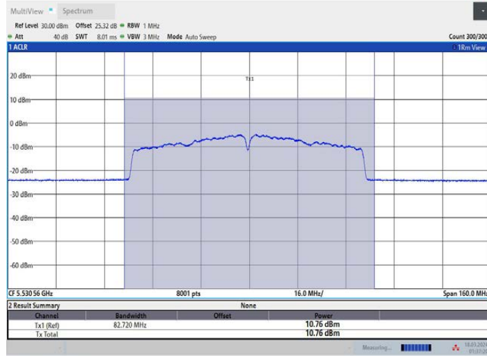
11AC80MIMO_Ant3_5530
