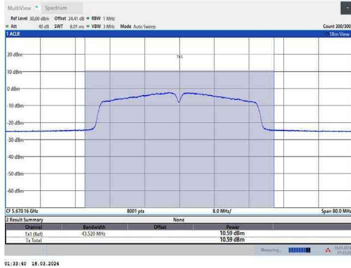
11AC40MIMO_Ant3_5670
