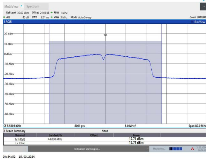
11AC40MIMO_Ant3_5510
