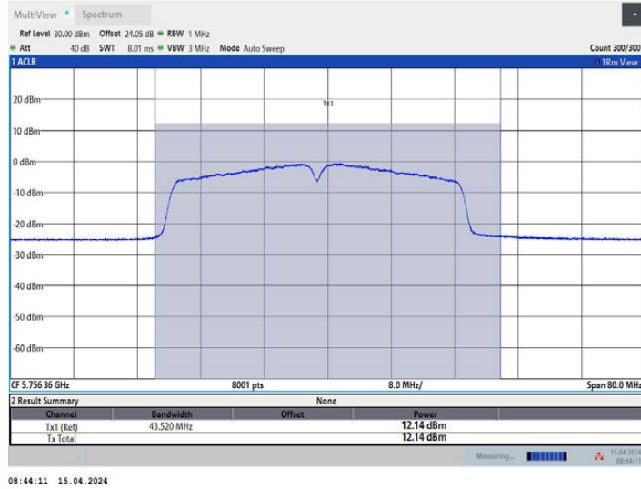
11AC40MIMO_Ant2_5755
