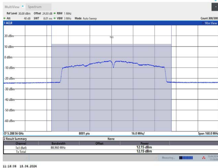
11AC80MIMO_Ant3_5290
