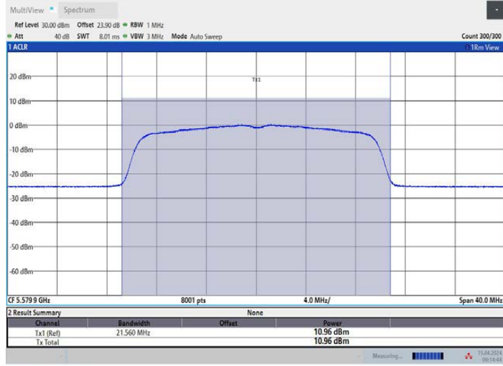
11AX20MIMO_Ant3_5580
