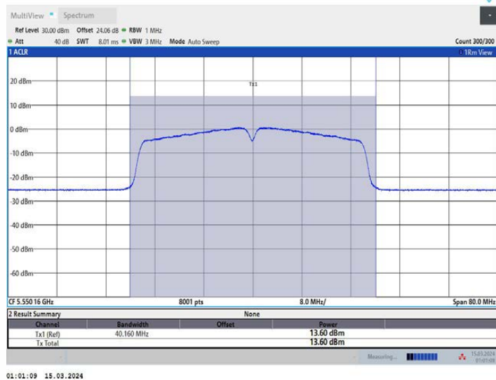
11AC40MIMO_Ant3_5550
