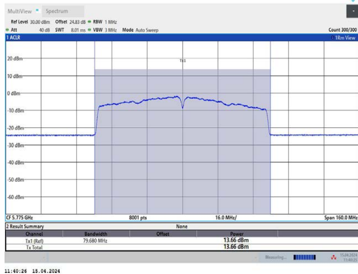
11AC80MIMO_Ant3_5775
