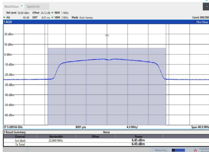
11AX20MIMO_Ant3_5700
