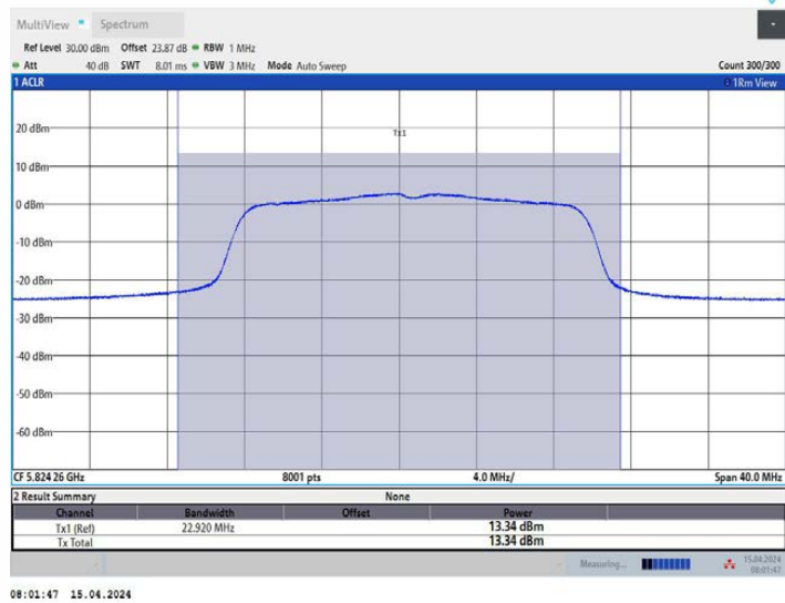
11AC20MIMO_Ant2_5825
