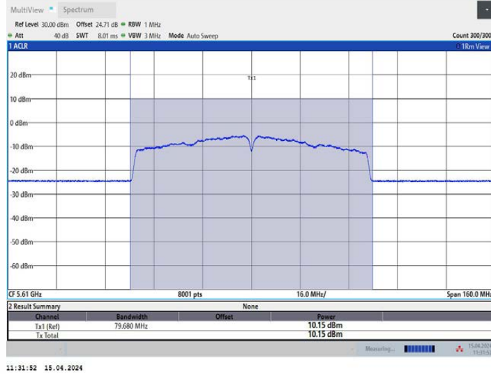
11AC80MIMO_Ant3_5610
