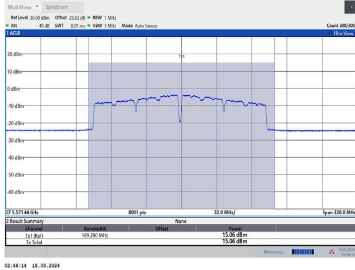
11AC160MIMO_Ant3_5570
