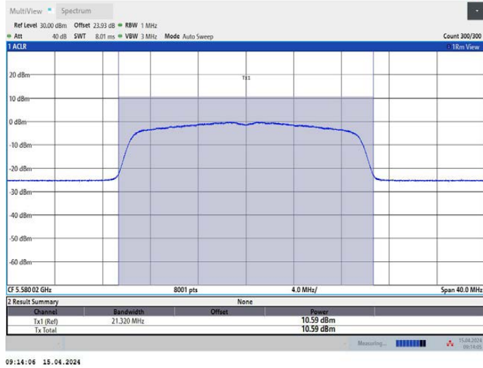
11AX20MIMO_Ant2_5580
