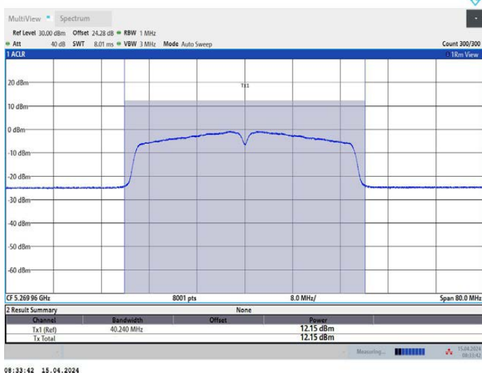
11AC40MIMO_Ant3_5270
