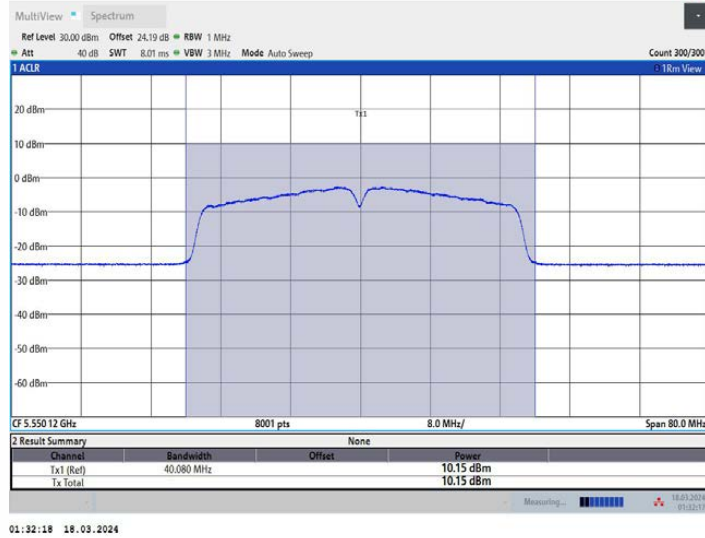
11AC40MIMO_Ant3_5550
