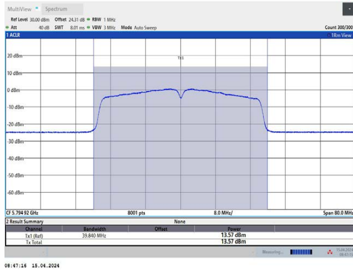
11AC40MIMO_Ant3_5795
