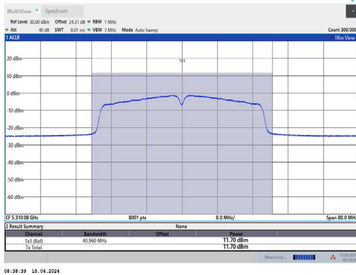
11AC40MIMO_Ant3_5310
