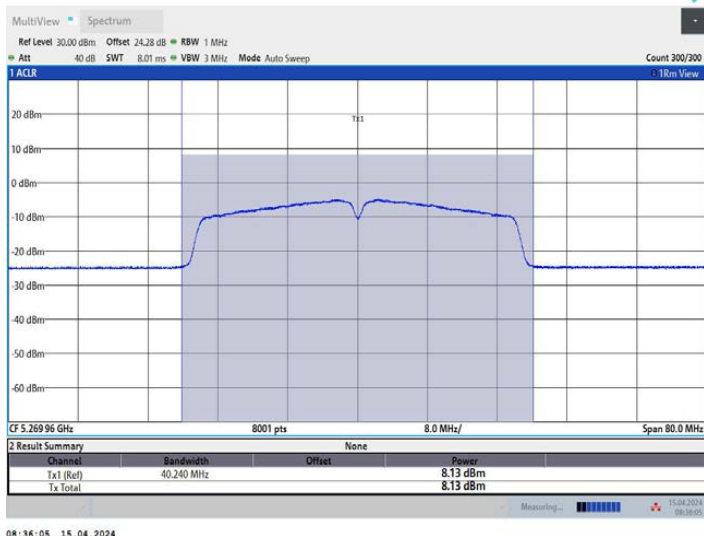
11AC40MIMO_Ant2_5270
