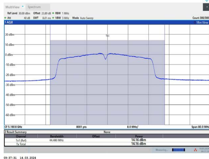
11AC40MIMO_Ant1_5190
