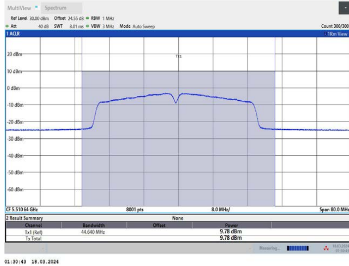
11AC40MIMO_Ant3_5510
