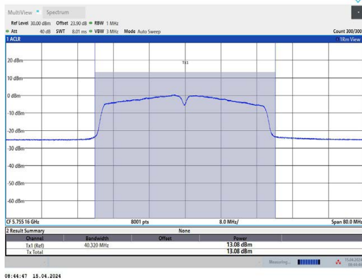
11AC40MIMO_Ant3_5755
