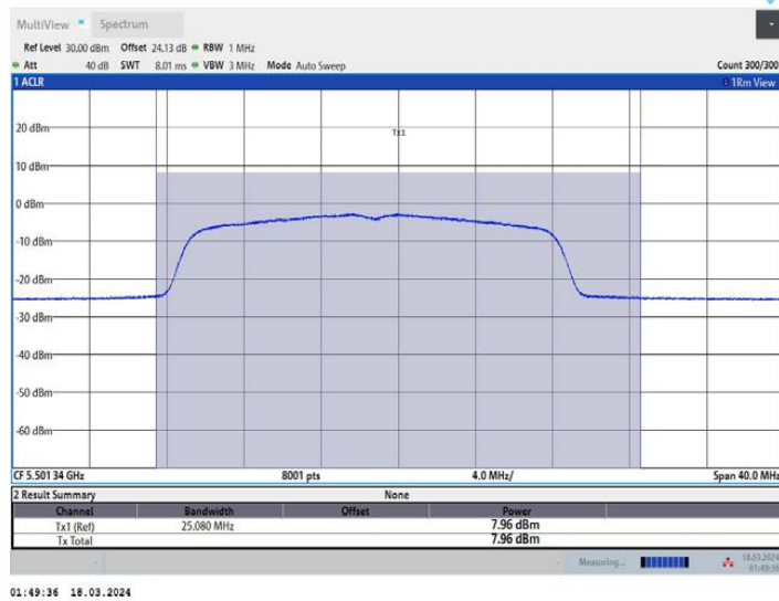
11AX20MIMO_Ant3_5500
