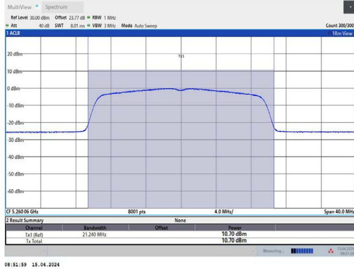
11AX20MIMO_Ant2_5260
