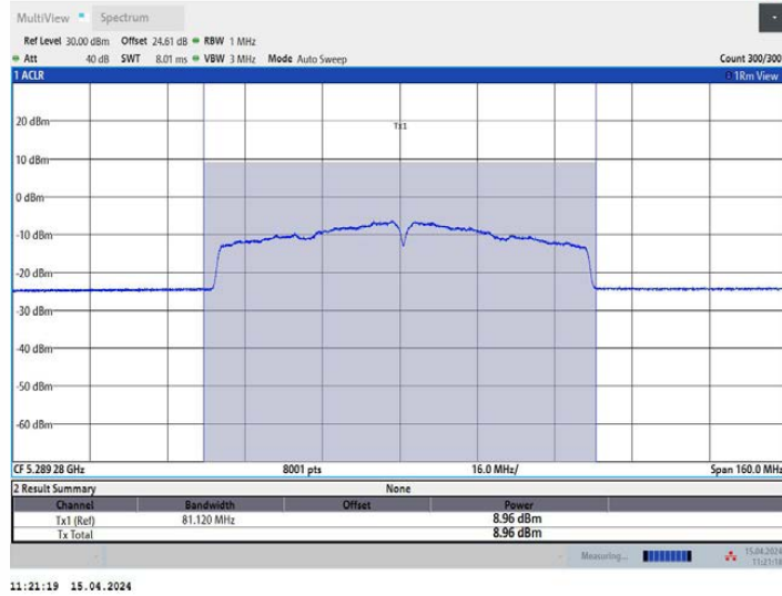
11AC80MIMO_Ant3_5290
