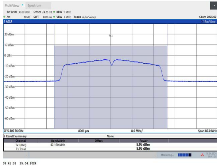
11AC40MIMO_Ant3_5310
