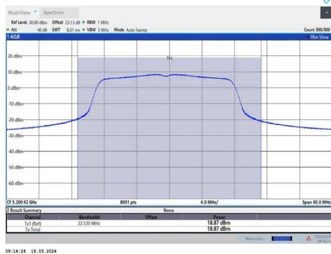
11A_Ant3_5200
