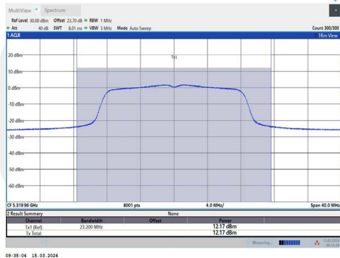
11A_Ant1_5320
