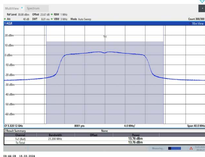
11A_Ant3_5320
