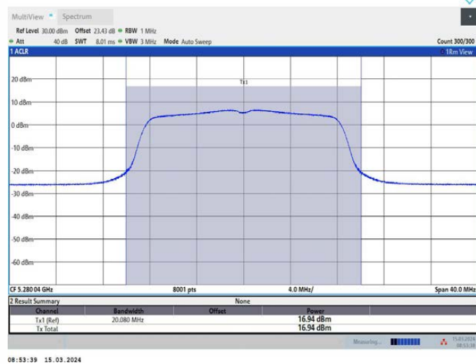
11A_Ant2_5280
