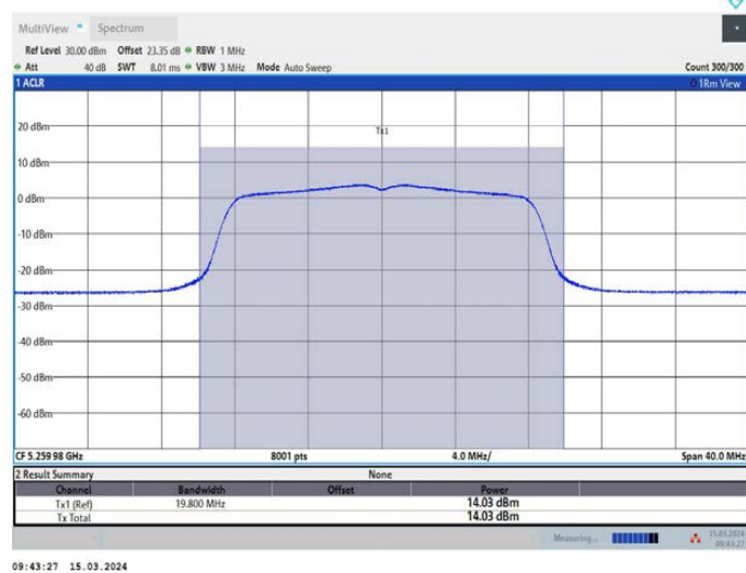
11A_Ant3_5260
