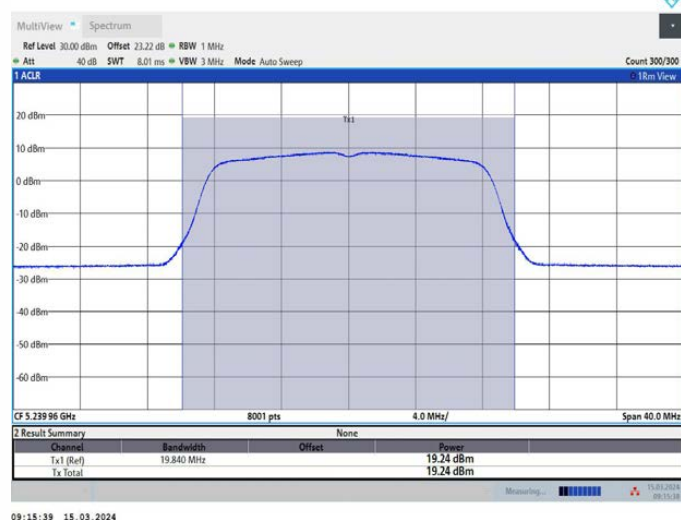
11A_Ant3_5240
