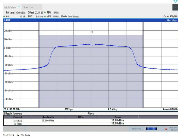
11N20MIMO_Ant3_5200
