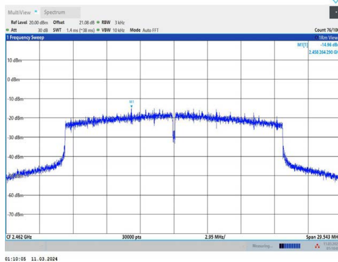
11AX20MIMO_Ant2_2462
