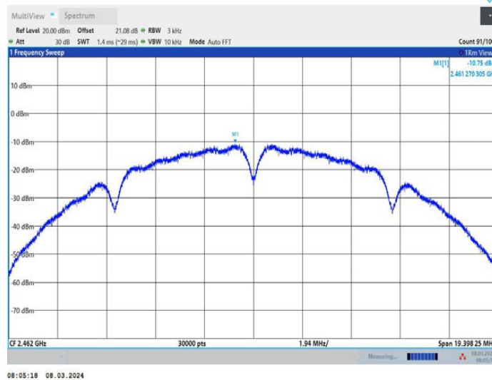
11B_Ant2_2462
