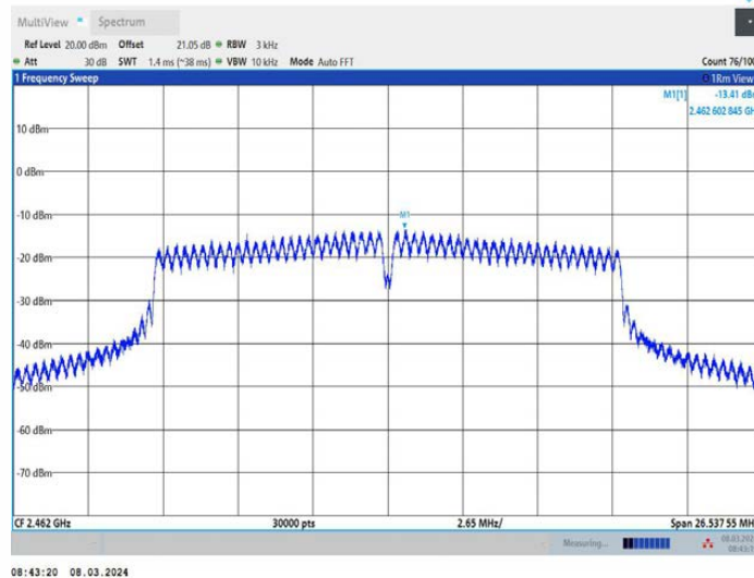
11G_Ant2_2462
