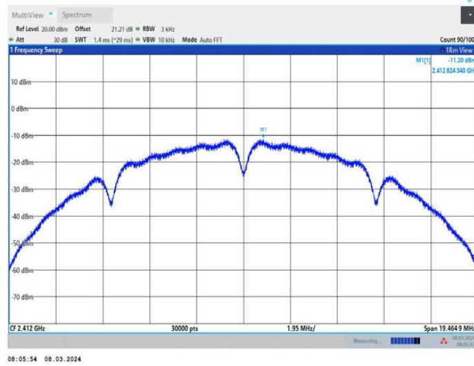
11B_Ant2_2412
