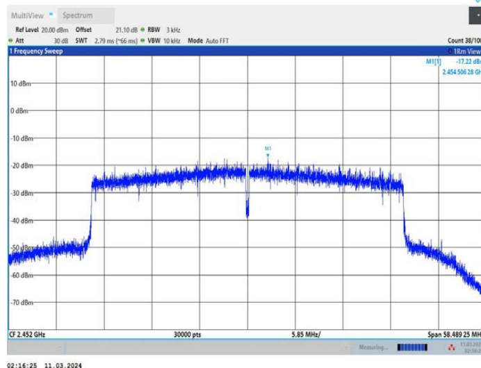
11AX40MIMO_Ant2_2452
