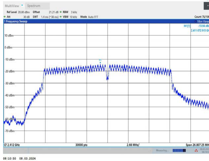
11G_Ant2_2412
