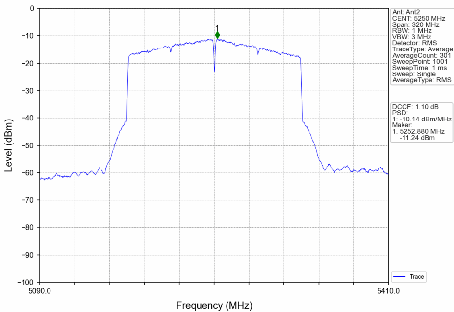
802.11ax(HEW160)_MCH_5250MHz_2xRU996_Left_Ant2_NTNV
