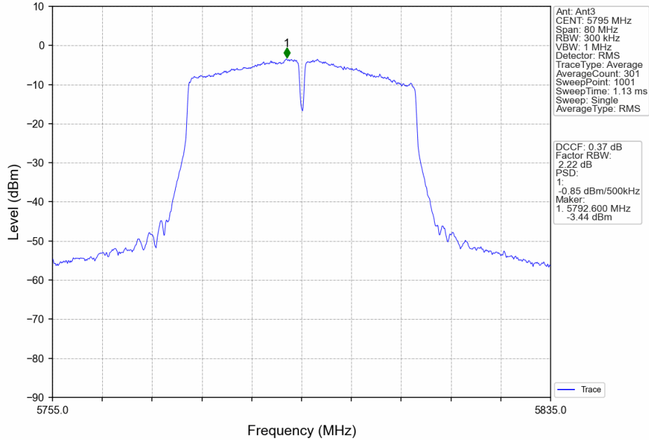
802.11n(HT40)_HCH_5795MHz_MIMO_NTNV
