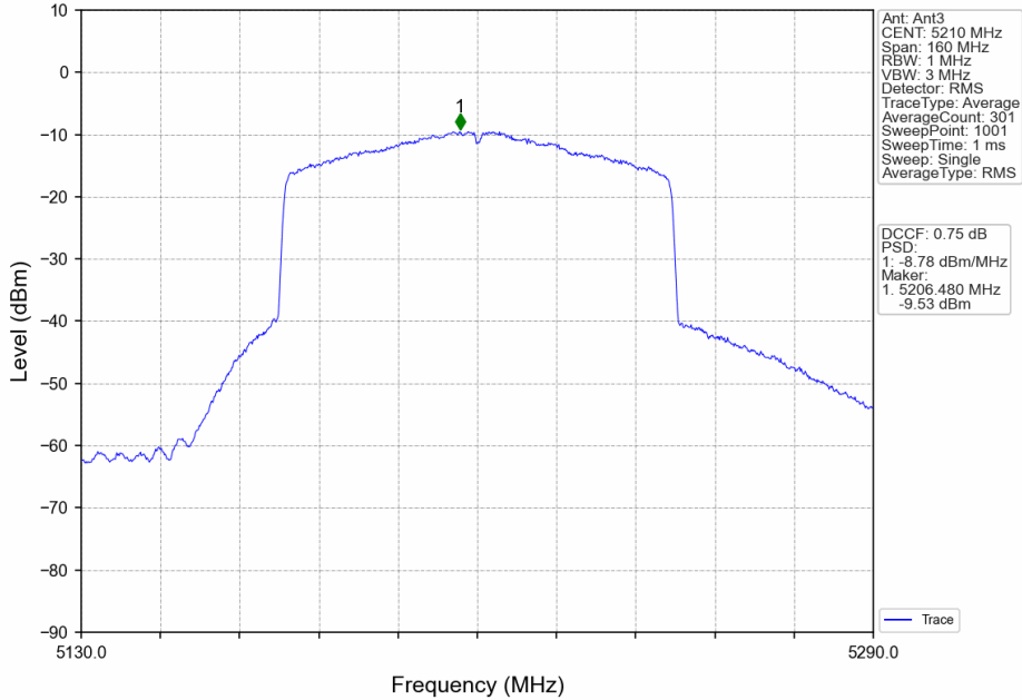
802.11ax(HEW80)_MCH_5210MHz_RU996_Left_MIMO_NTNV
