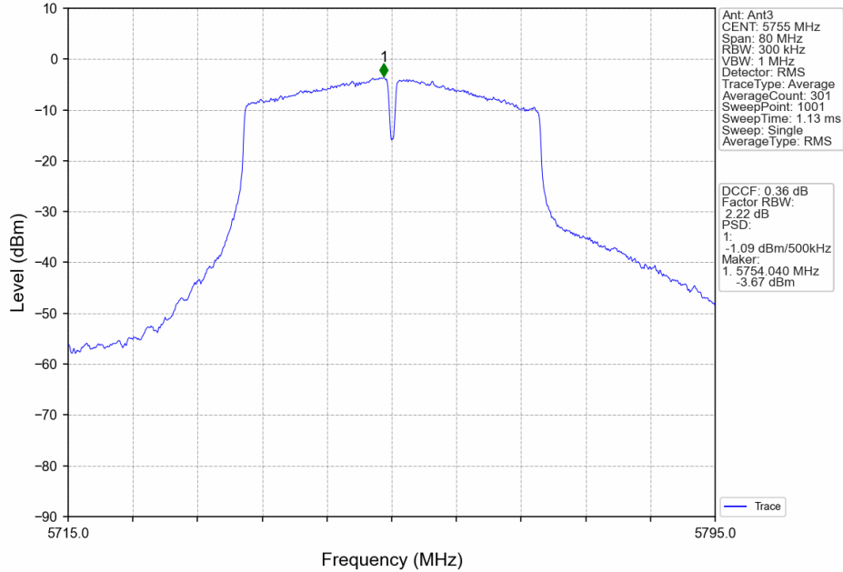
802.11n(HT40)_LCH_5755MHz_MIMO_NTNV
