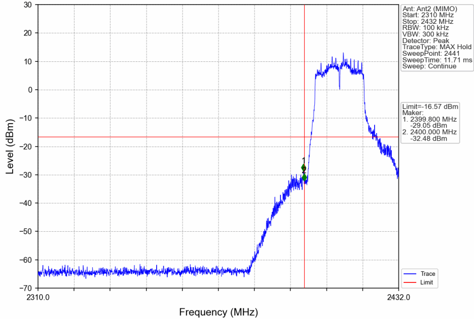
802.11g_LCH_2412MHz_Ant2 (MIMO)_NTNV
