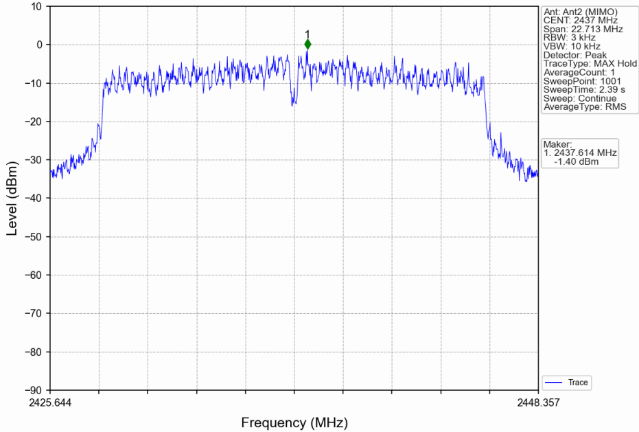
802.11n(HT20)_MCH_2437MHz_MIMO_NTNV
