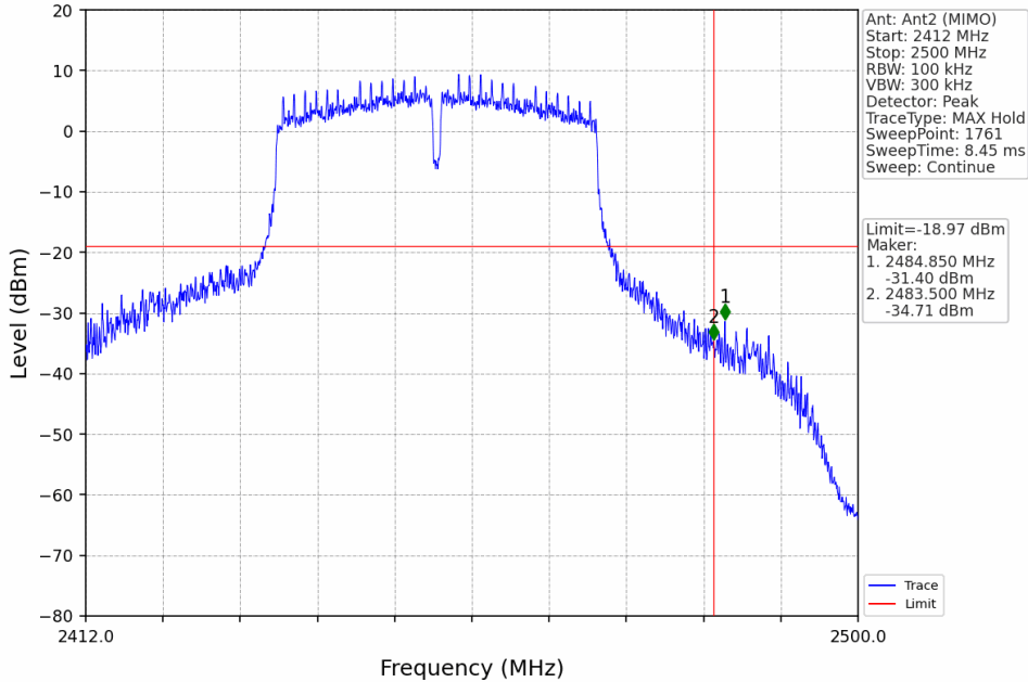
802.11n(HT40)_HCH_2452MHz_Ant2 (MIMO)_NTNV
