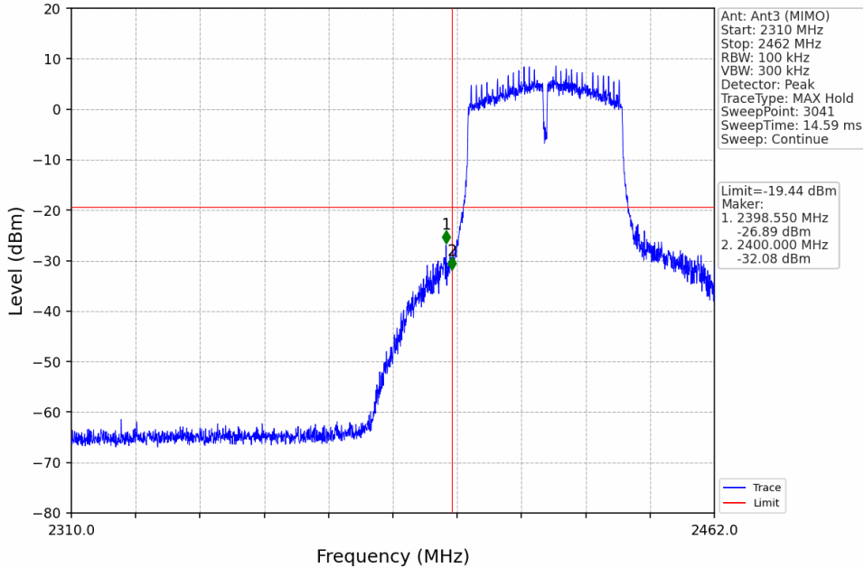
802.11n(HT40)_LCH_2422MHz_Ant3 (MIMO)_NTNV
