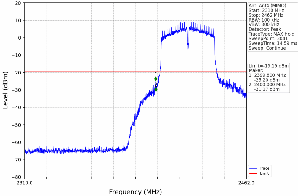
802.11n(HT40)_LCH_2422MHz_Ant4 (MIMO)_NTNV
