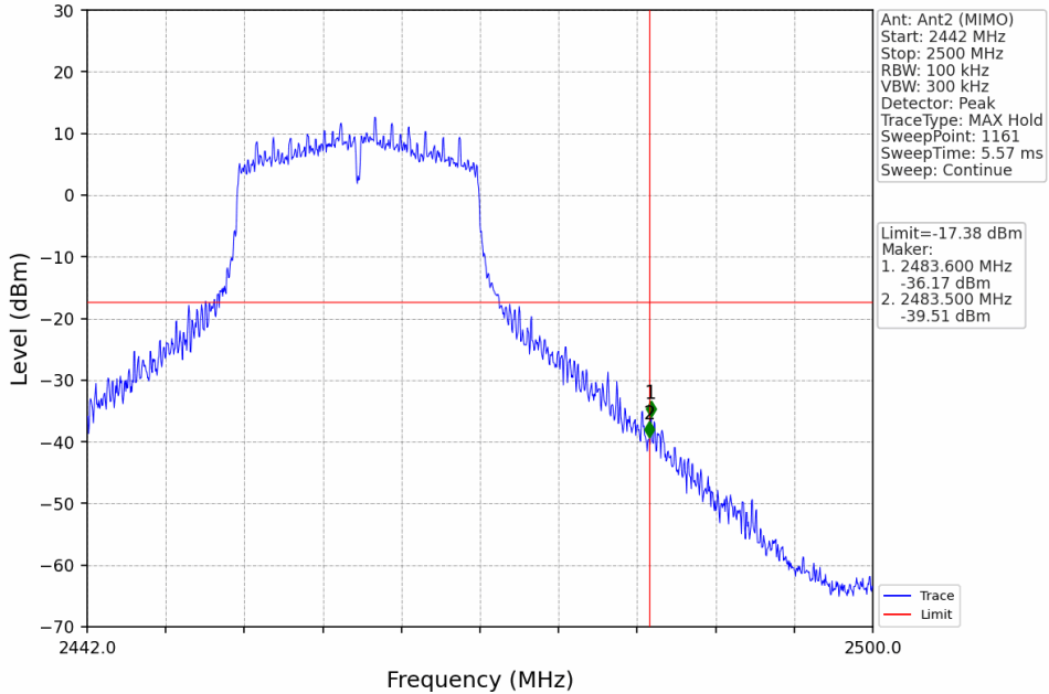
802.11n(HT20)_HCH_2462MHz_Ant2 (MIMO)_NTNV
