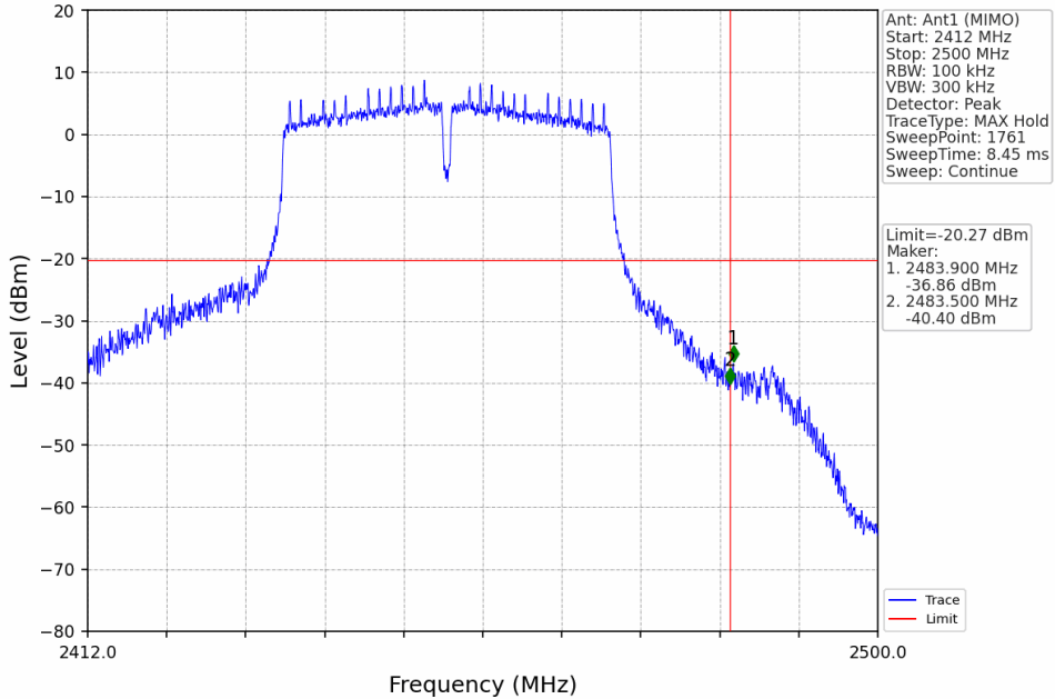
802.11n(HT40)_HCH_2452MHz_Ant1 (MIMO)_NTNV
