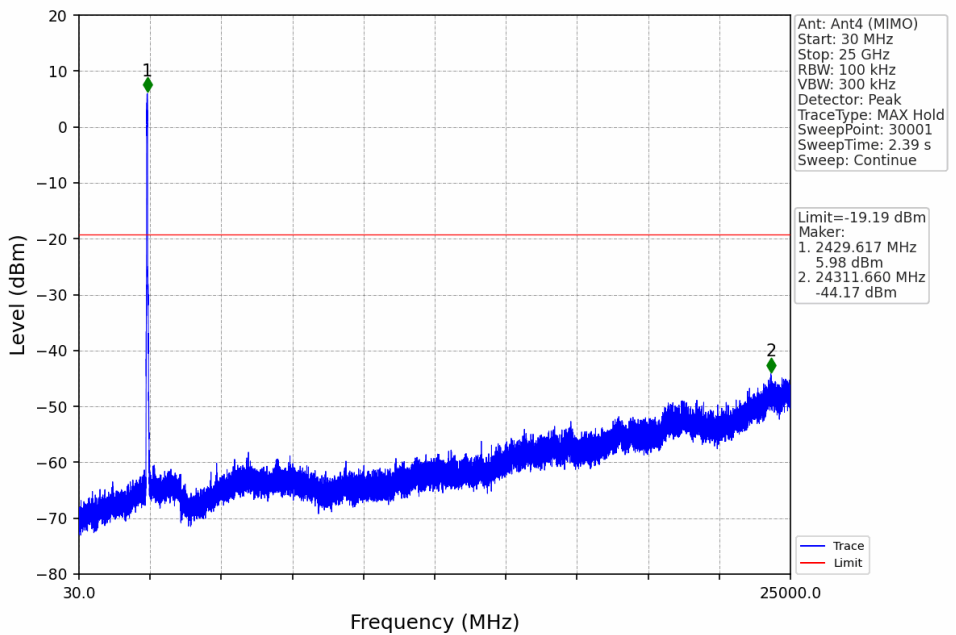
802.11n(HT40)_LCH_2422MHz_Ant4 (MIMO)_NTNV
