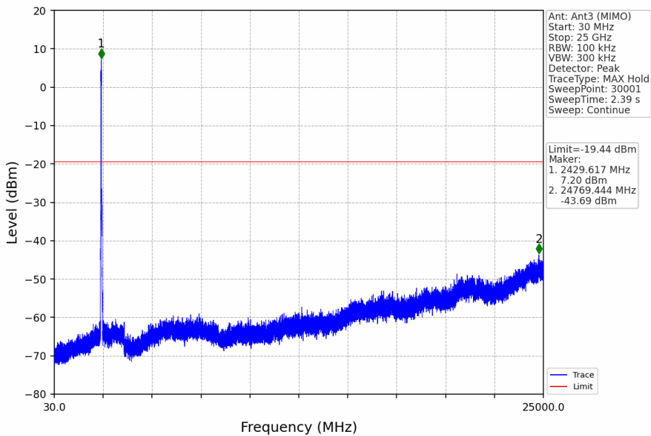
802.11n(HT40)_LCH_2422MHz_Ant3 (MIMO)_NTNV
