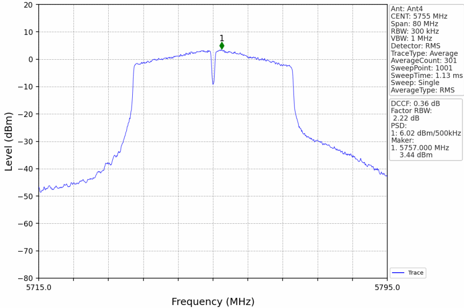
802.11ac(VHT40)_LCH_5755MHz_MIMO_NTNV
