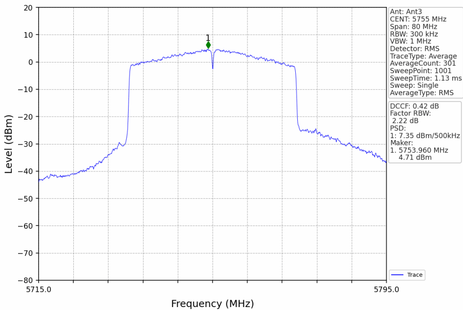
802.11ax(HEW40)_LCH_5755MHz_RU484_Left_Ant3_NTNV
