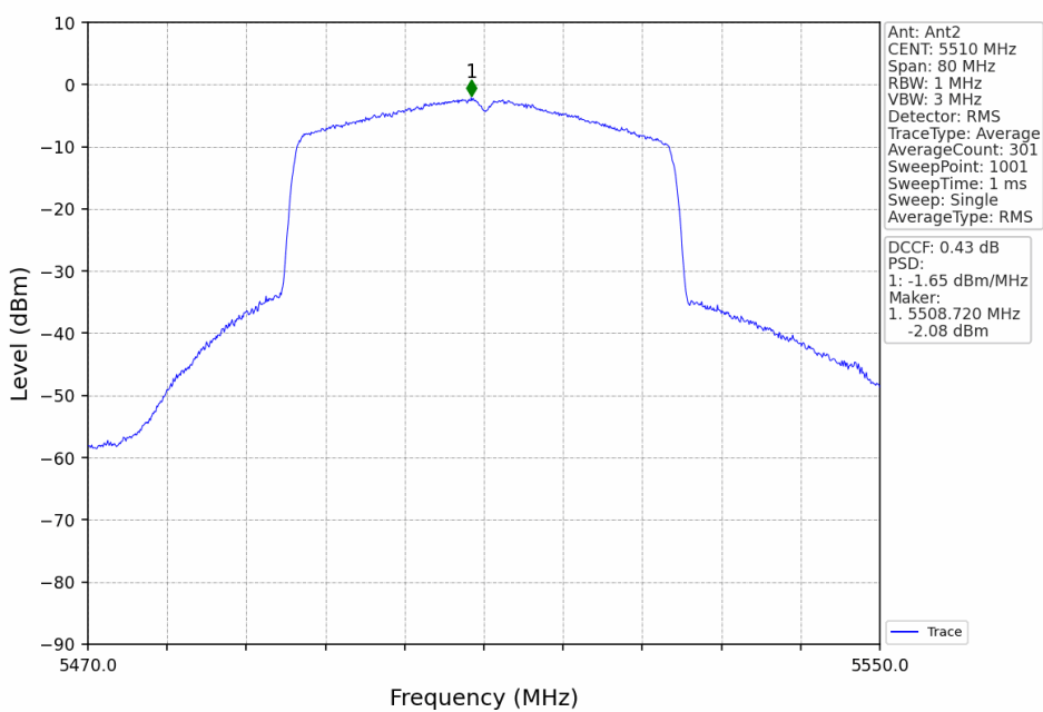
802.11ax(HEW40)_LCH_5510MHz_RU484_Left_Ant2_NTNV
