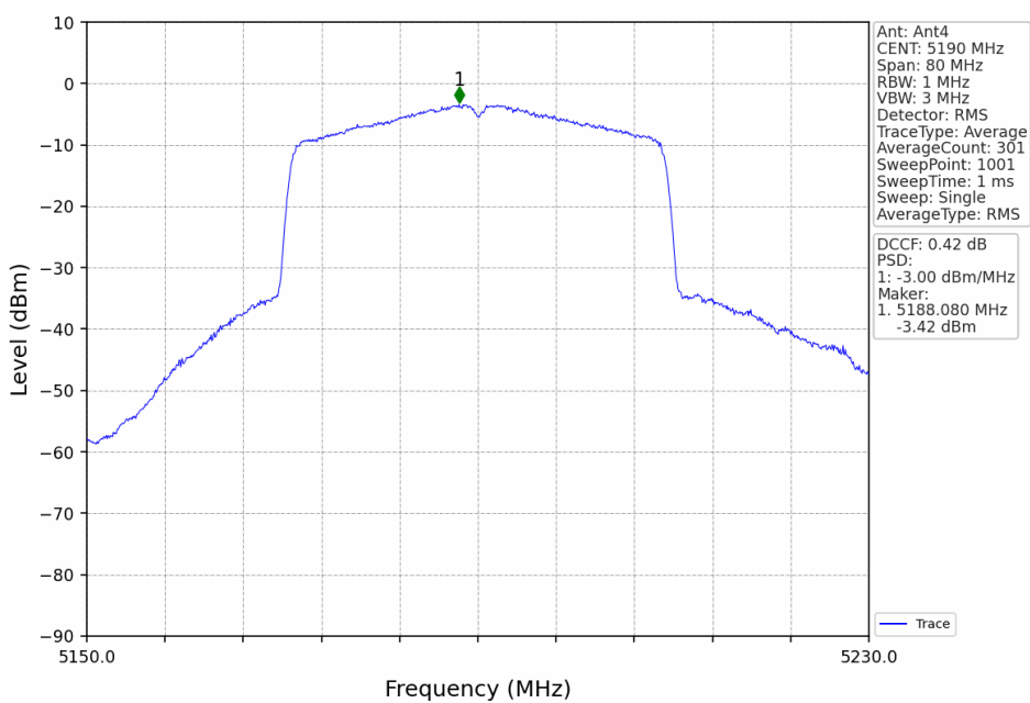
802.11ax(HEW40)_LCH_5190MHz_RU484_Left_Ant4_NTNV
