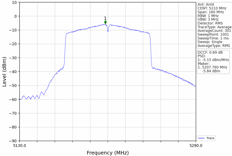
802.11ac(VHT80)_MCH_5210MHz_MIMO_NTNV
