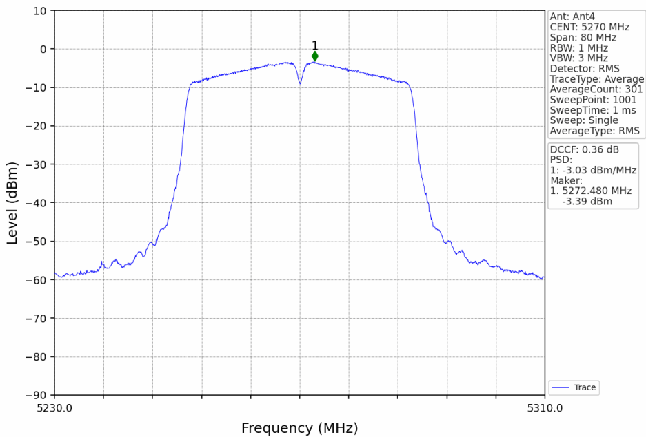
802.11ac(VHT40)_LCH_5270MHz_Ant4_NTNV
