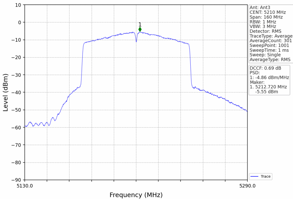
802.11ac(VHT80)_MCH_5210MHz_Ant3_NTNV
