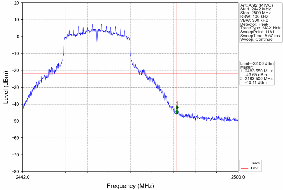
802.11n(HT20)_HCH_2462MHz_Ant2 (MIMO)_NTNV
