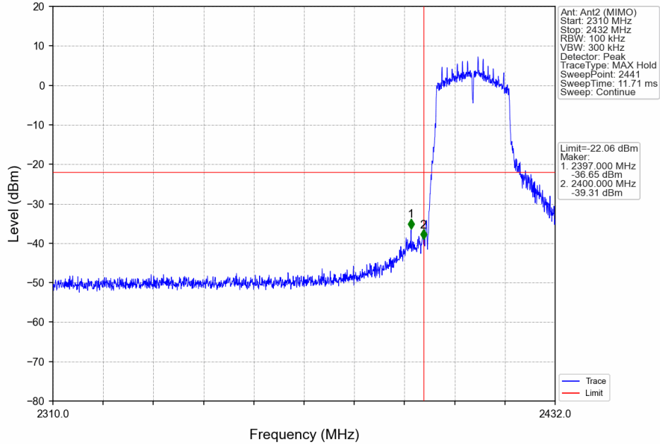
802.11n(HT20)_LCH_2412MHz_Ant2 (MIMO)_NTNV
