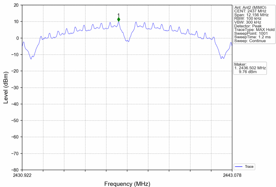
802.11b_MCH_2437MHz_Ant2 (MIMO)_NTNV
