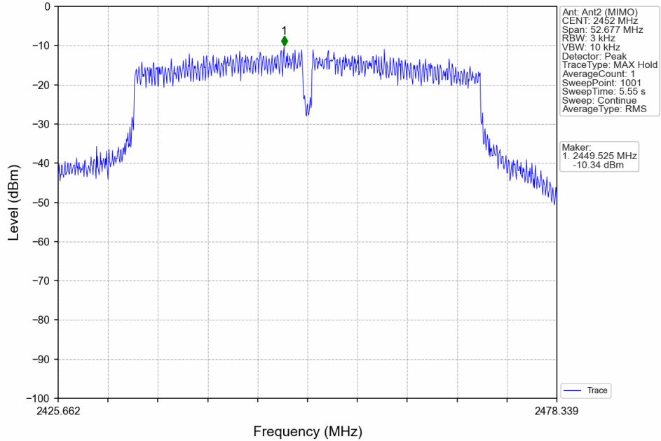
802.11n(HT40)_HCH_2452MHz_MIMO_NTNV
