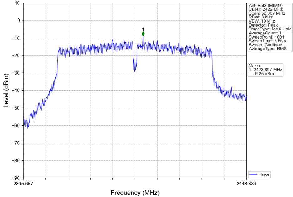
802.11n(HT40)_LCH_2422MHz_MIMO_NTNV
