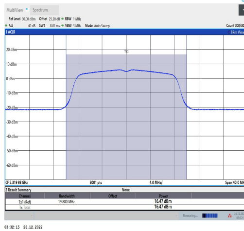
11A-Ant1-5320-TPC L-----16.29-95.86-0.18
