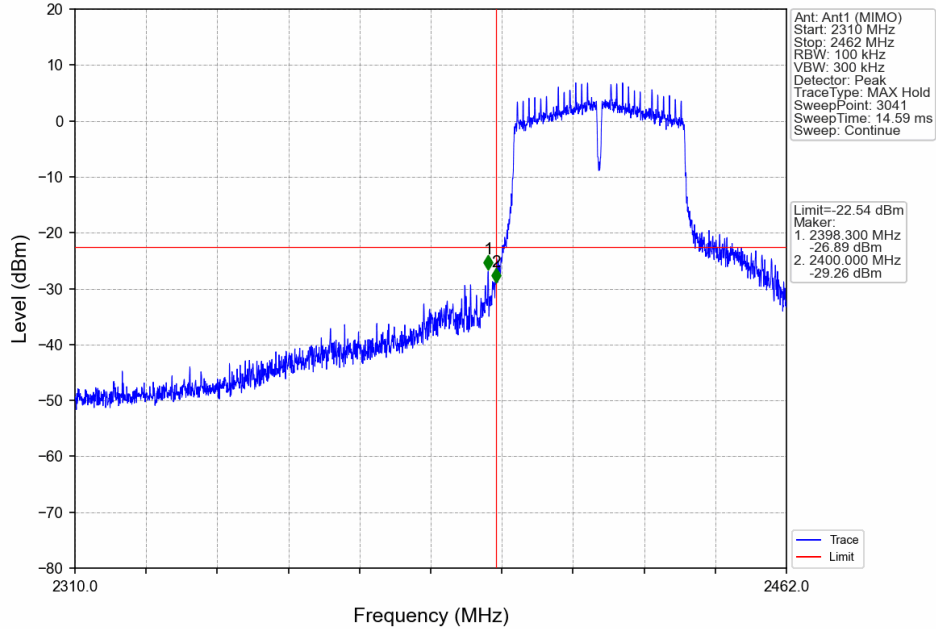
802.11n(HT40)_LCH_2422MHz_Ant1 (MIMO)_NTNV
