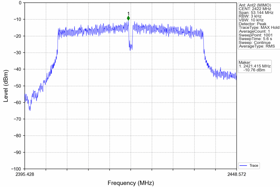
802.11n(HT40)_LCH_2422MHz_MIMO_NTNV
