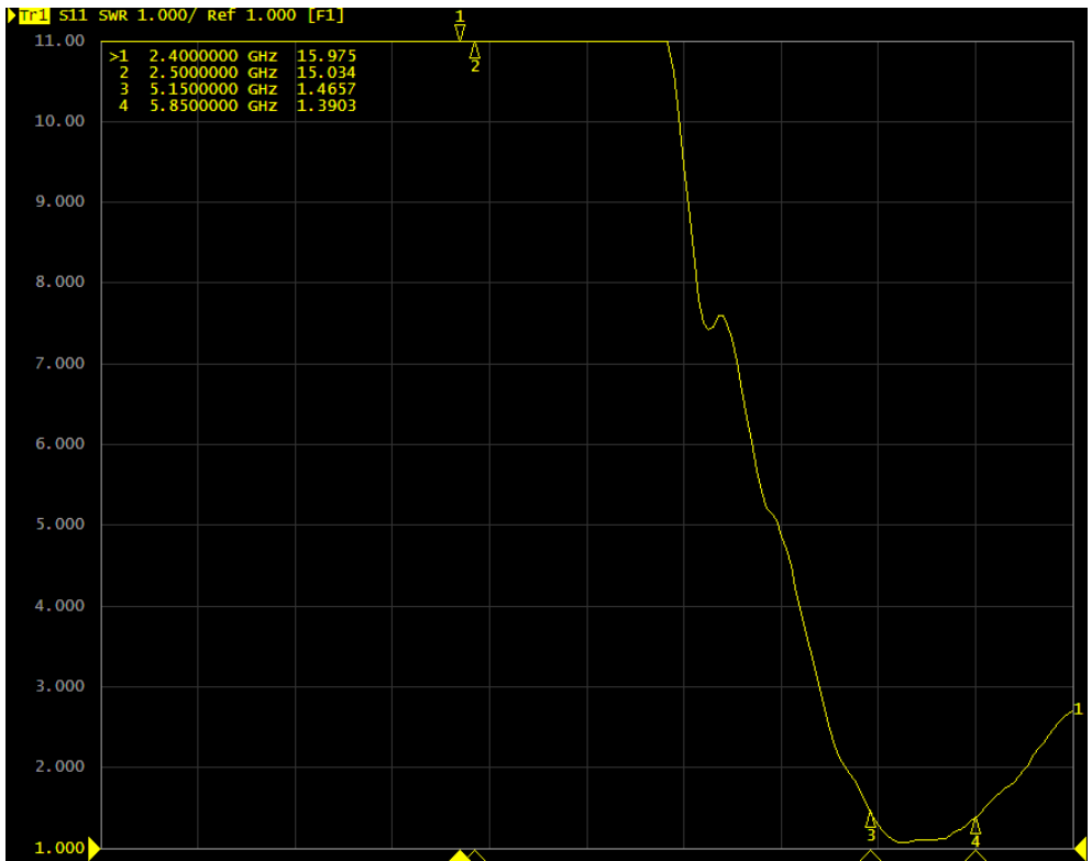
VSWR-3
