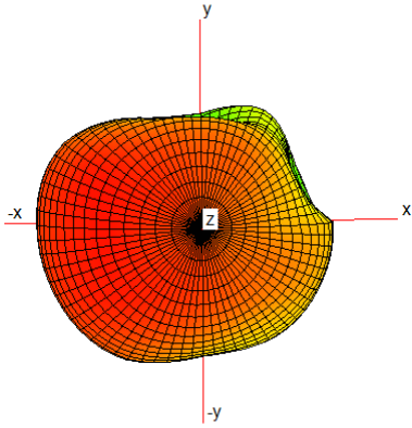
5150MHz
