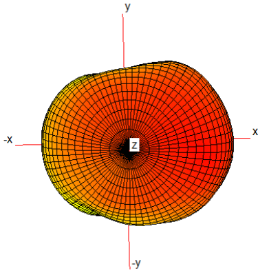
5150MHz
