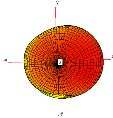
5500MHz
