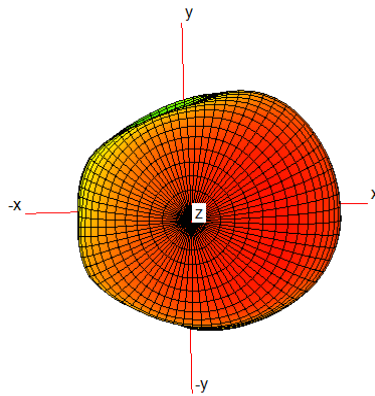
2450MHz
