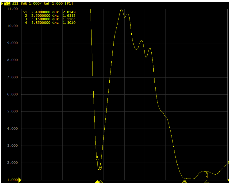
VSWR-2
