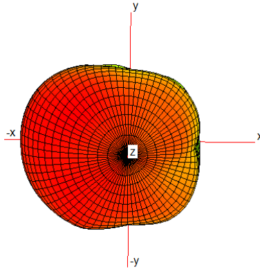
5500MHz
