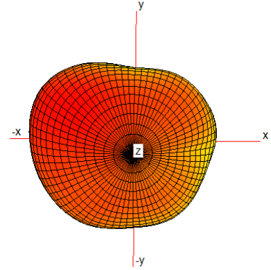
5850MHz
