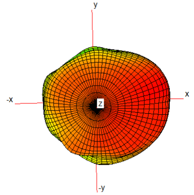
5850MHz
