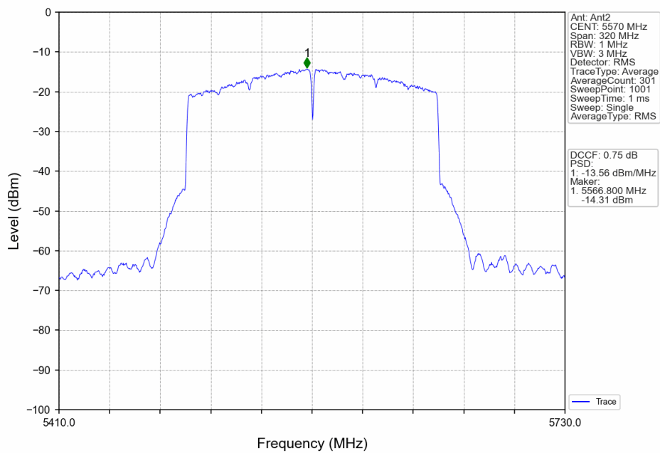
802.11ax(HEW160)_MCH_5570MHz_2xRU996_Left_Ant2_NTNV
