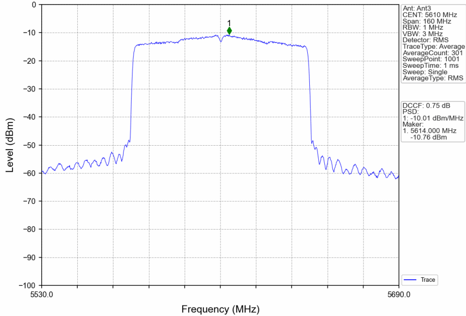
802.11ax(HEW80)_HCH_5610MHz_RU996_Left_MIMO_NTNV
