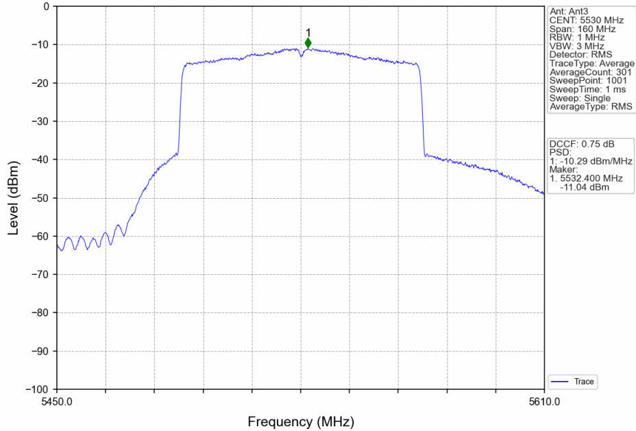
802.11ax(HEW80)_LCH_5530MHz_RU996_Left_MIMO_NTNV
