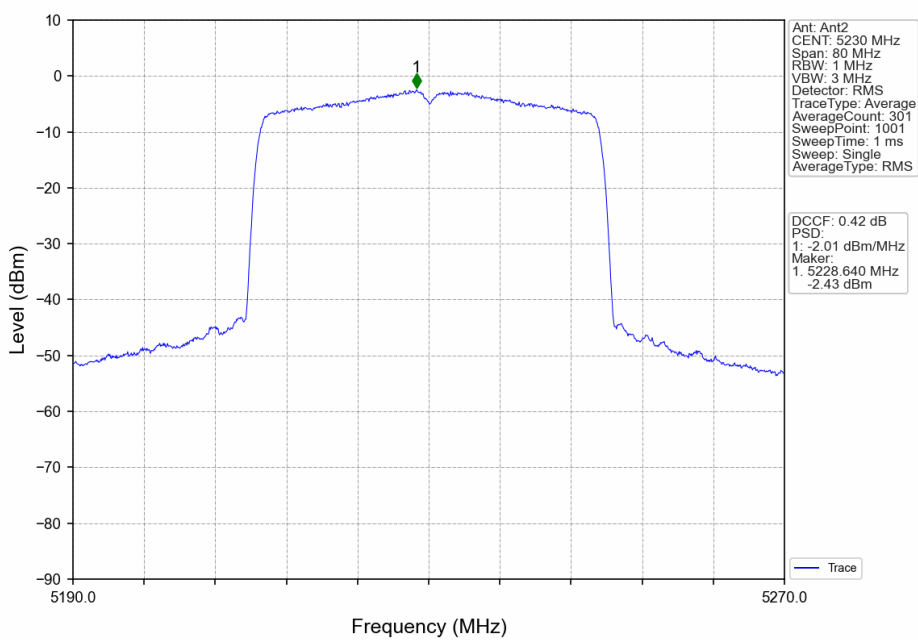
802.11ax(HEW40)_HCH_5230MHz_RU484_Left_Ant2_NTNV
