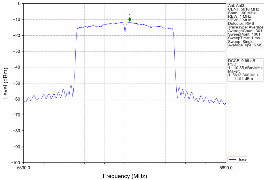
802.11ac(VHT80)_HCH_5610MHz_MIMO_NTNV
