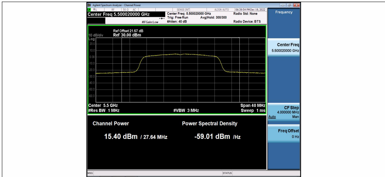
11AC20MIMO_Ant2_5500
