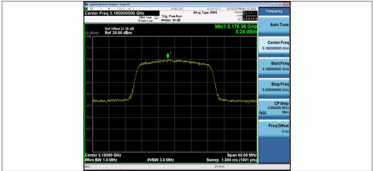
11AC20MIMO_Ant2_5180
