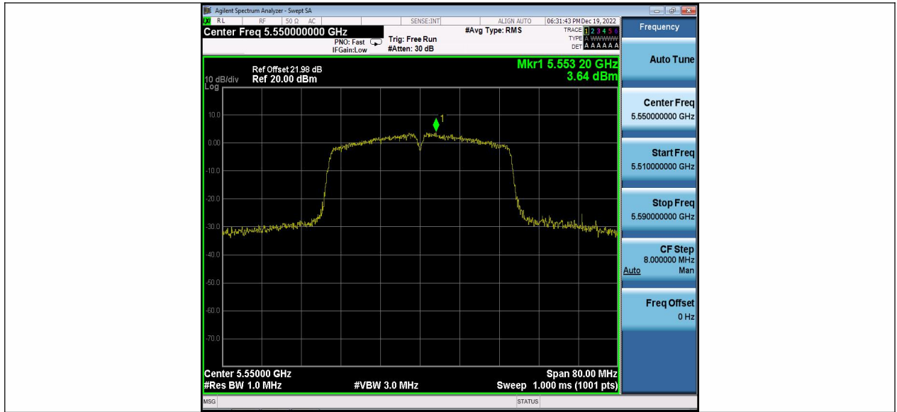
11N40MIMO_Ant2_5550
