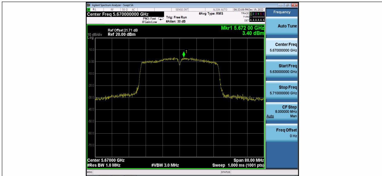
11N40MIMO_Ant2_5670
