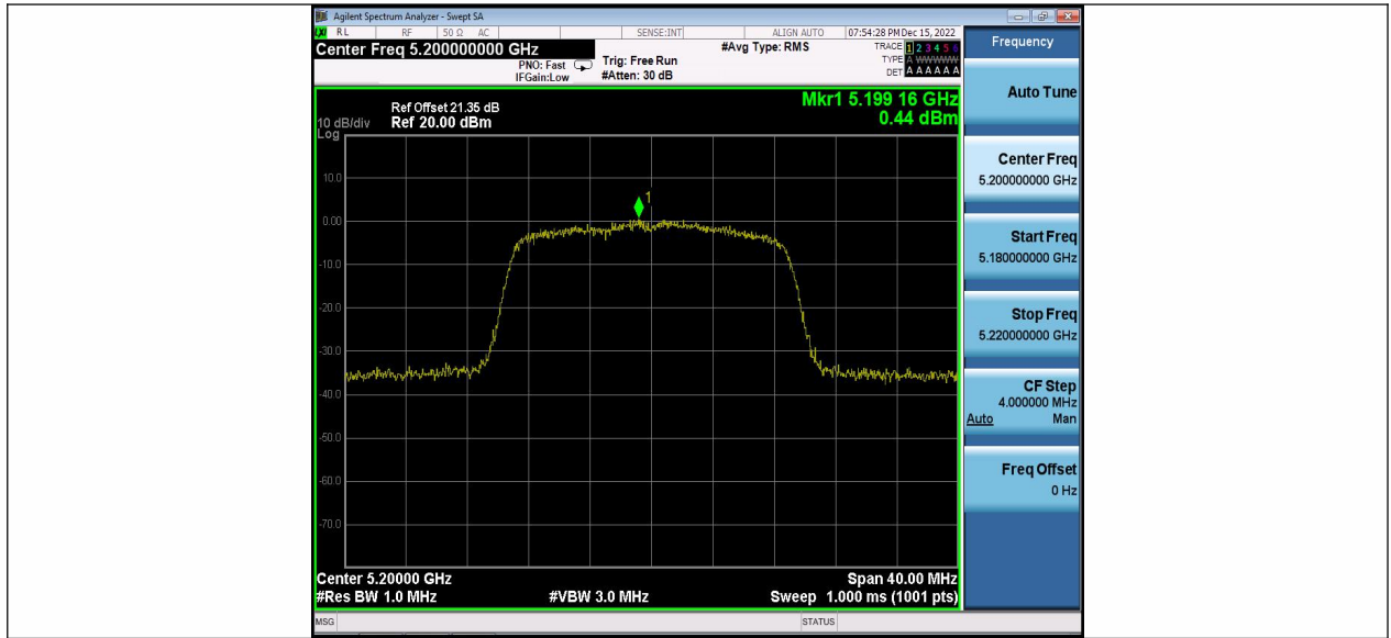
11AC20MIMO_Ant2_5200
