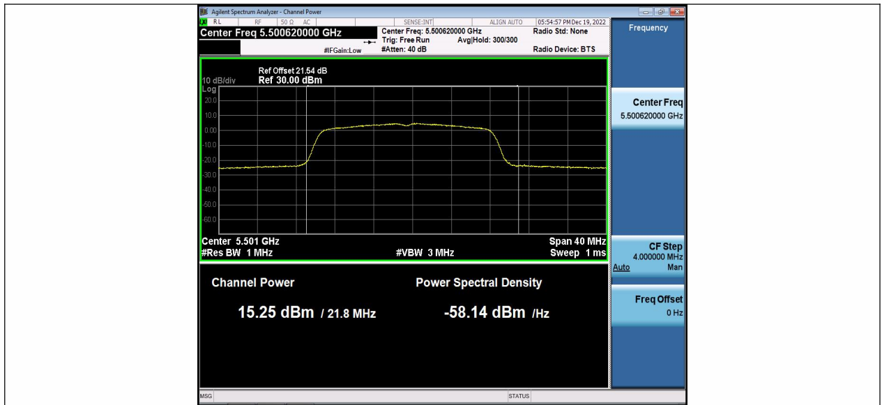
11N20MIMO_Ant2_5500
