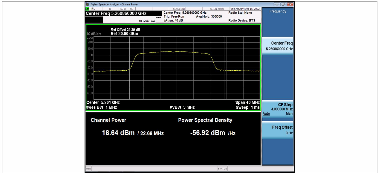
11N20MIMO_Ant2_5260
