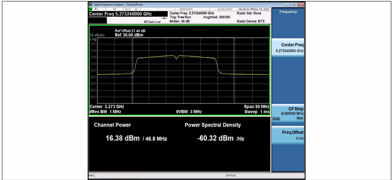
11N40MIMO_Ant2_5270
