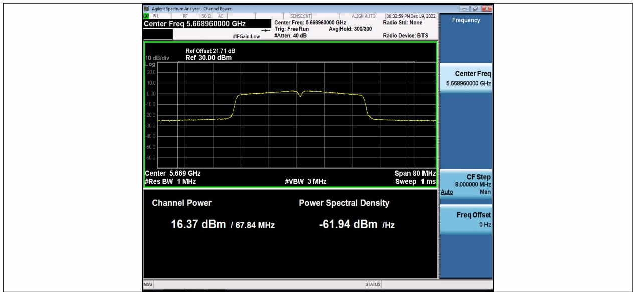
11N40MIMO_Ant2_5670
