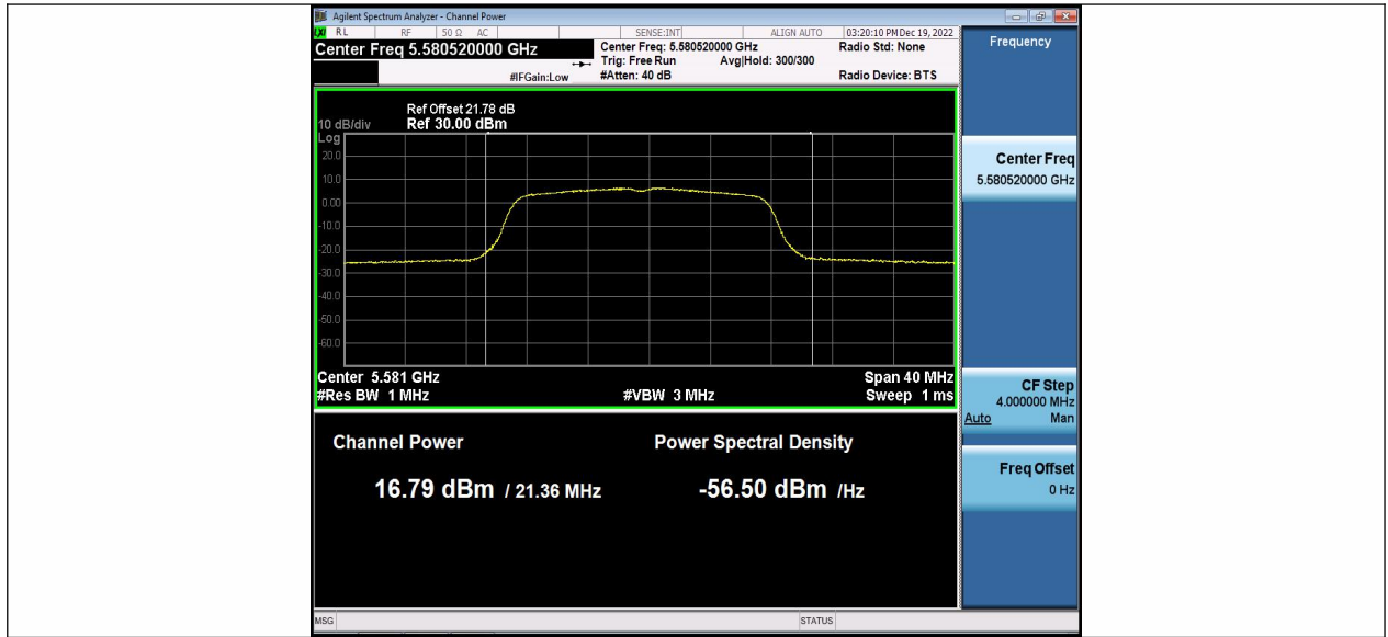
11A_Ant2_5580
