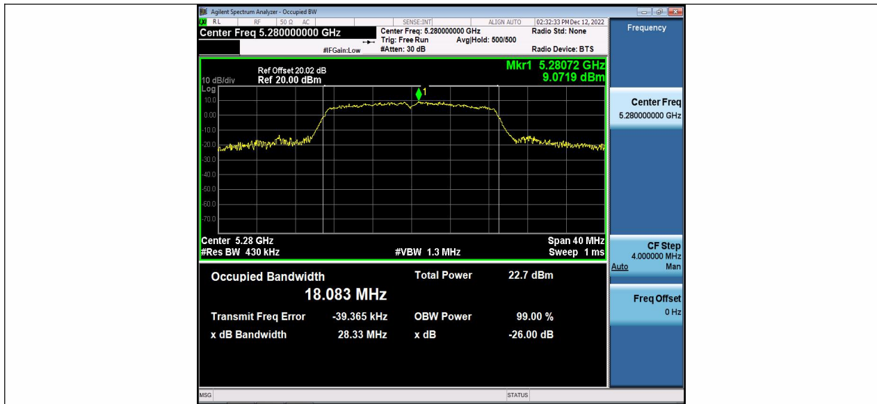
11AC20MIMO_Ant2_5280
