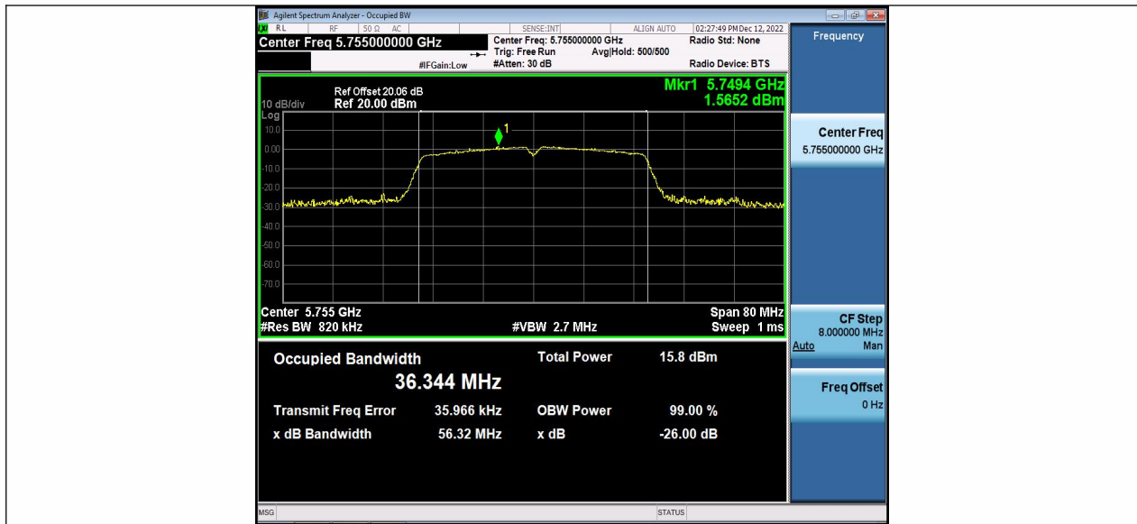
11N40MIMO_Ant2_5755
