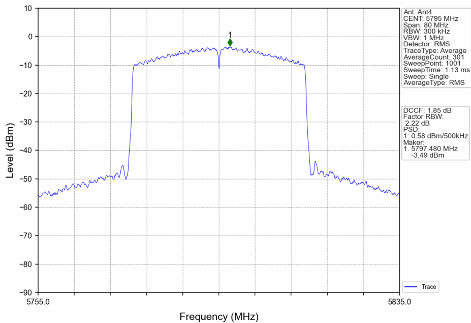
802.11ax(HEW40)_HCH_5795MHz_RU484_Left_Ant4_NTNV
