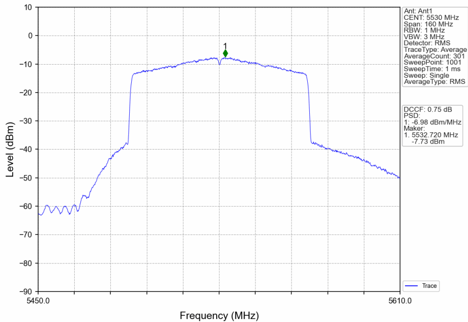
802.11ax(HEW80)_LCH_5530MHz_RU996_Left_Ant1_NTNV
