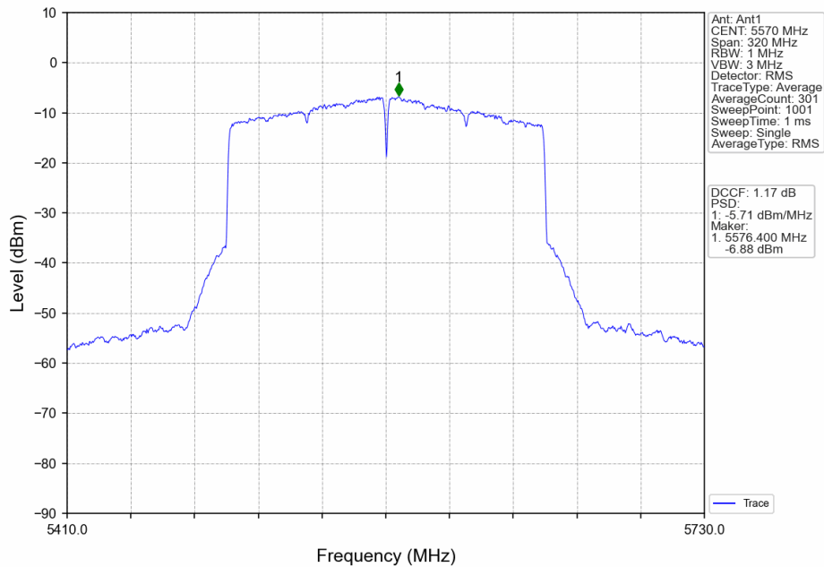
802.11ax(HEW160)_MCH_5570MHz_2xRU996_Left_Ant1_NTNV
