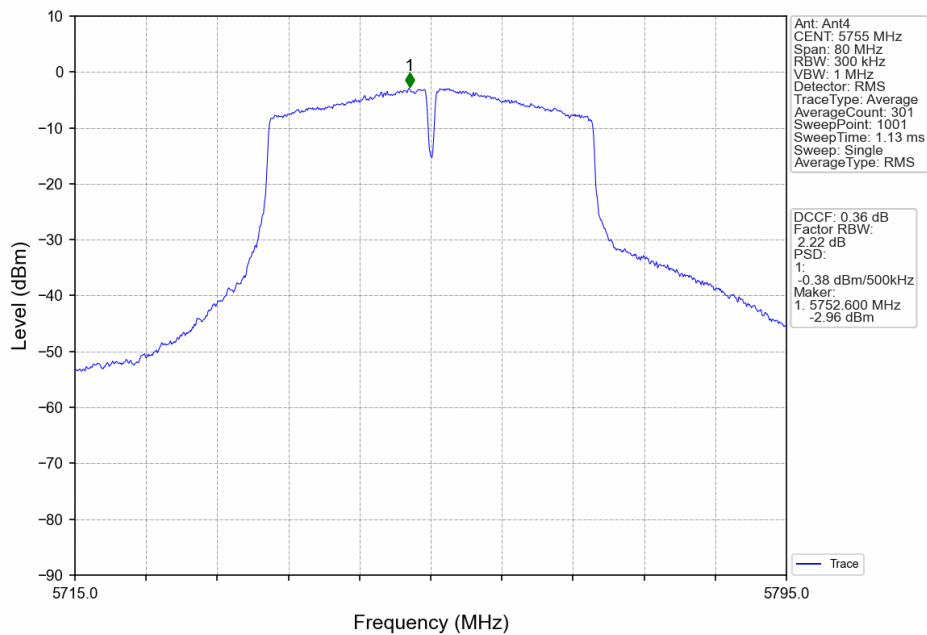
802.11n(HT40)_LCH_5755MHz_Ant4_NTNV
